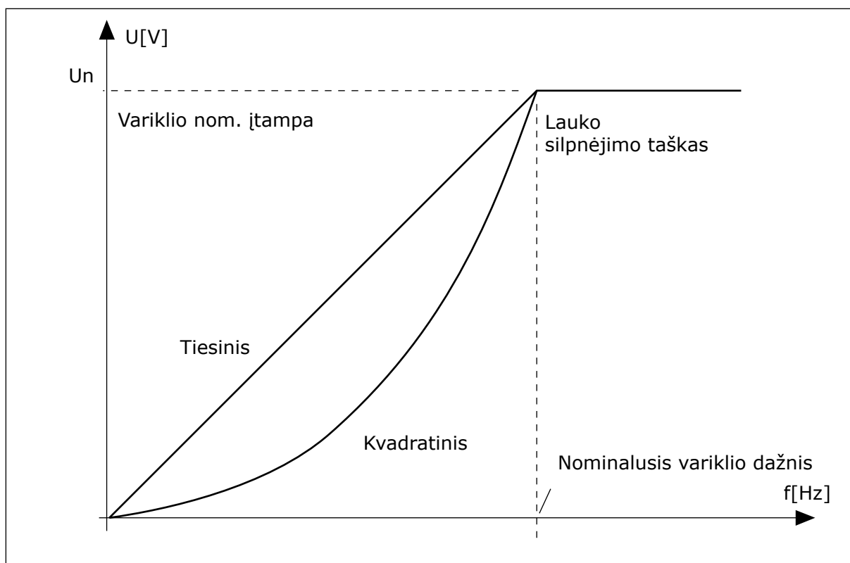
Pav. 13: Variklio įtampos kitimas tiesiniu ir kvadrato principu
