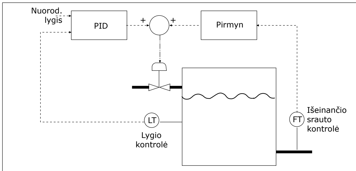
Pav. 40: Tiesioginės eigos (tiekimo) valdymas
