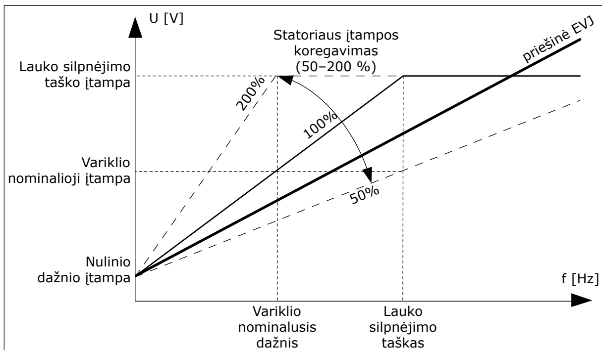
Pav. 14: Statoriaus įtampos koregavimas
