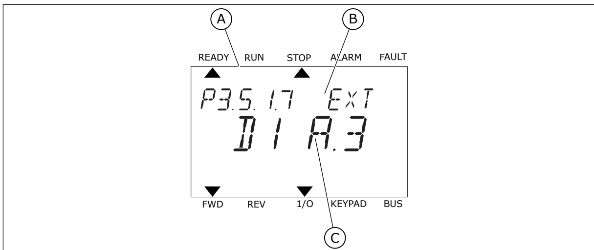
图 24: 文本显示屏中的“数字输入”菜单
