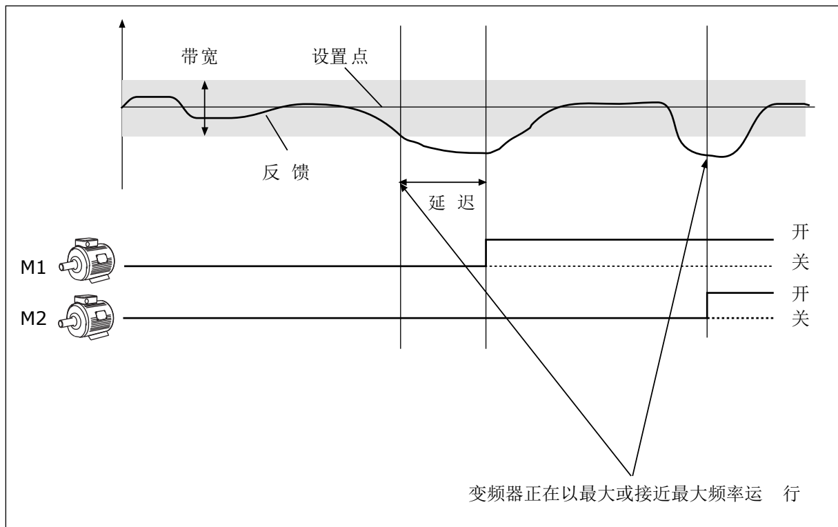
图 44: 多泵功能
