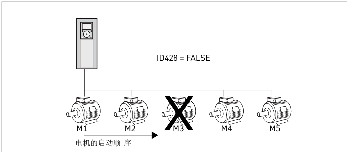
图 46: 互锁逻辑 2
