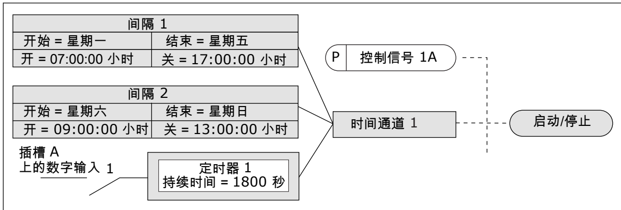
图 36: 时间通道 1 ( 而非数字输入 ) 用作启动命令的控制信号
