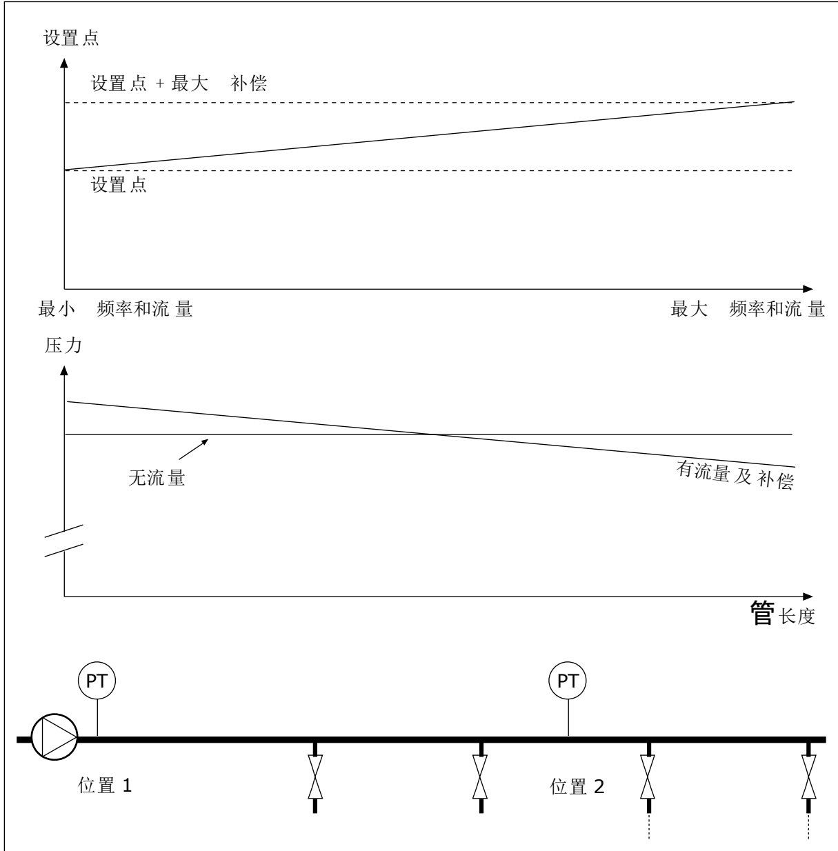
图 43: 压力损失补偿的启用设置点 1
