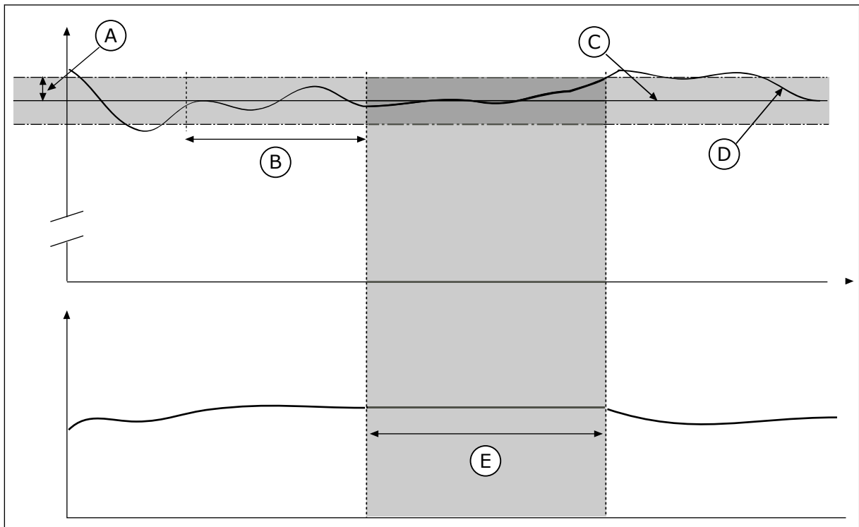
图 37: 死区功能
