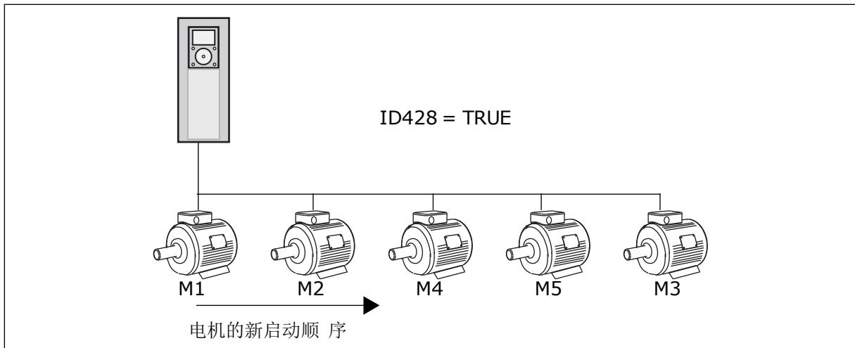
图 47: 互锁逻辑 3
