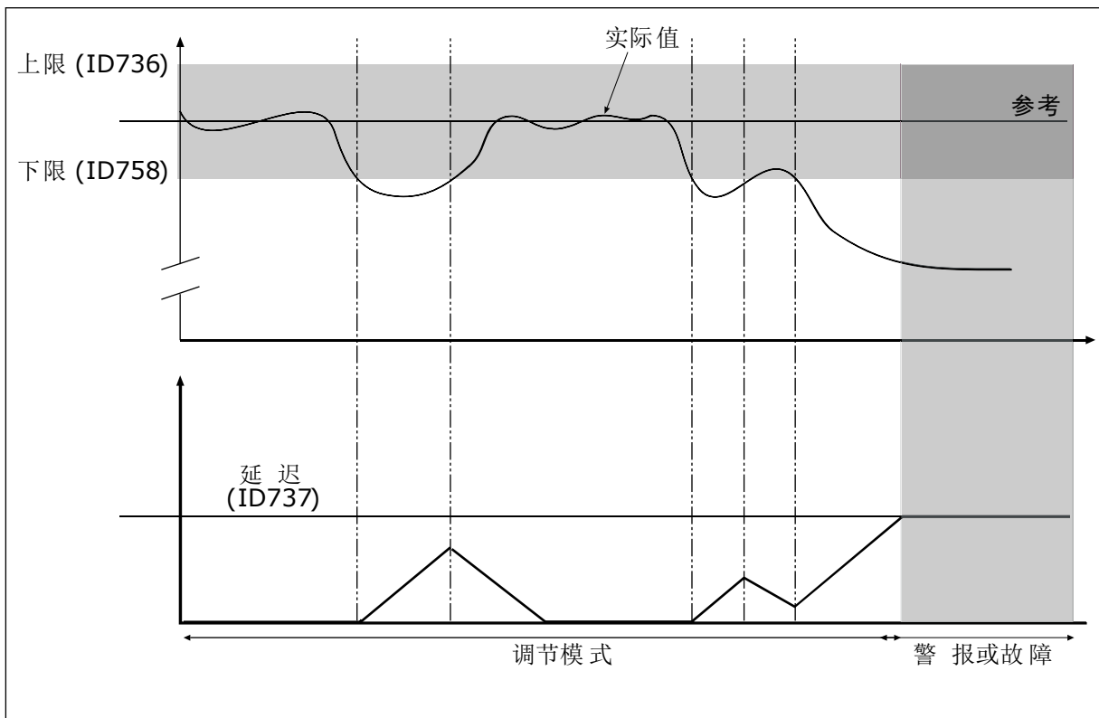
图 41: 反馈监控功能
