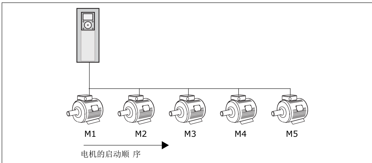
图 45: 互锁逻辑 1
