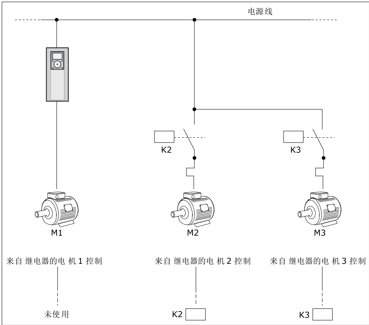
图 48: 选择 0
