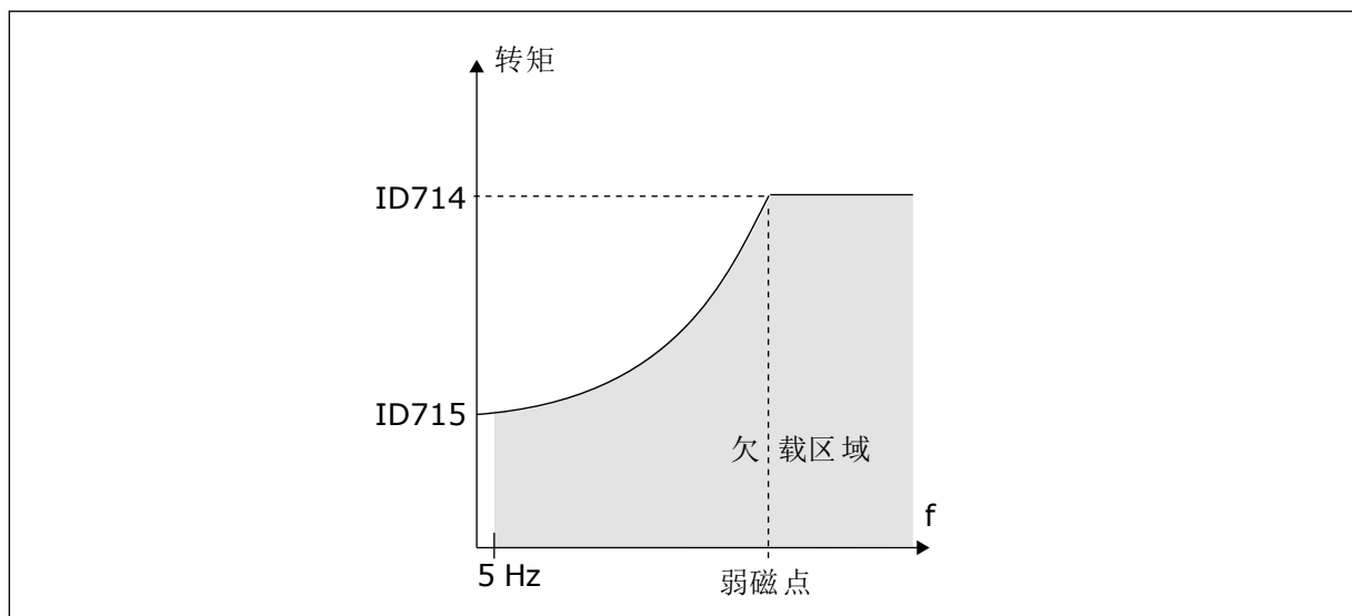
图 31: 设置最小负载
