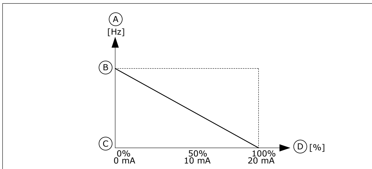
Afb. 52: A11-siginaalinversie bij parameterwaarde 1
