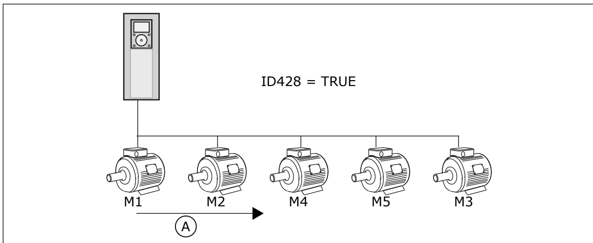
Afb. 83: Vergrendelingslogica 3
