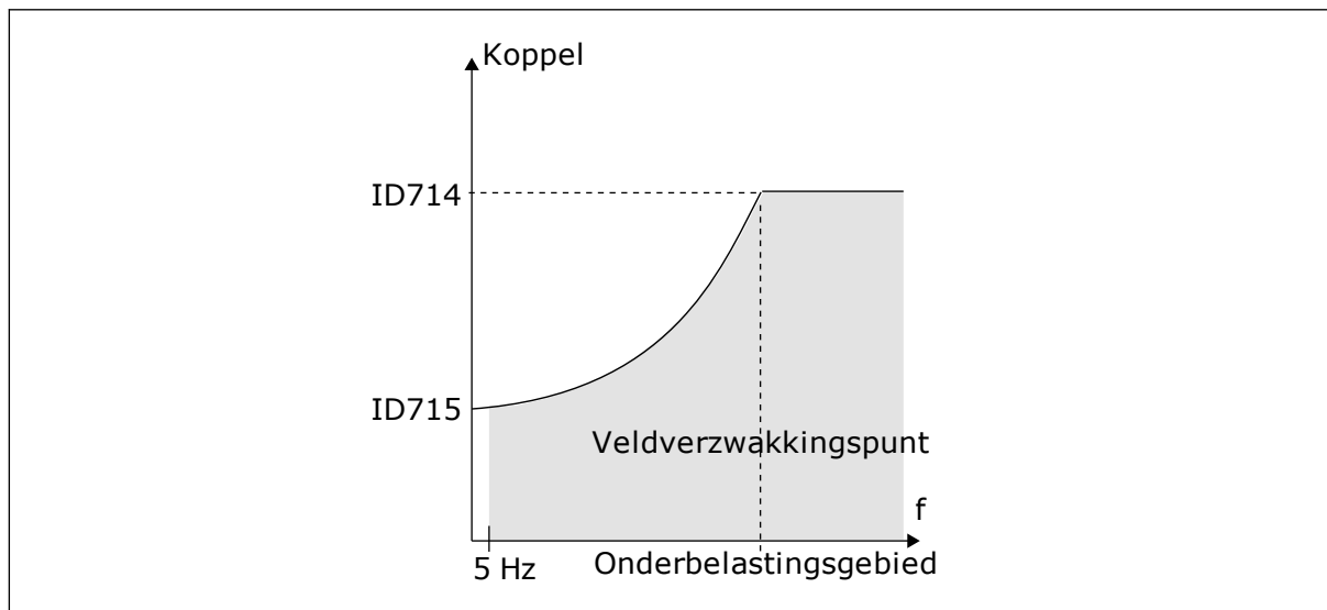
Afb. 60: De minimumbelasting instellen
