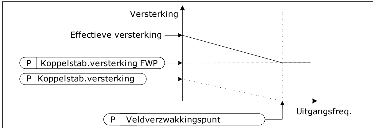
Afb. 26: De koppelstabilisatieversterking
