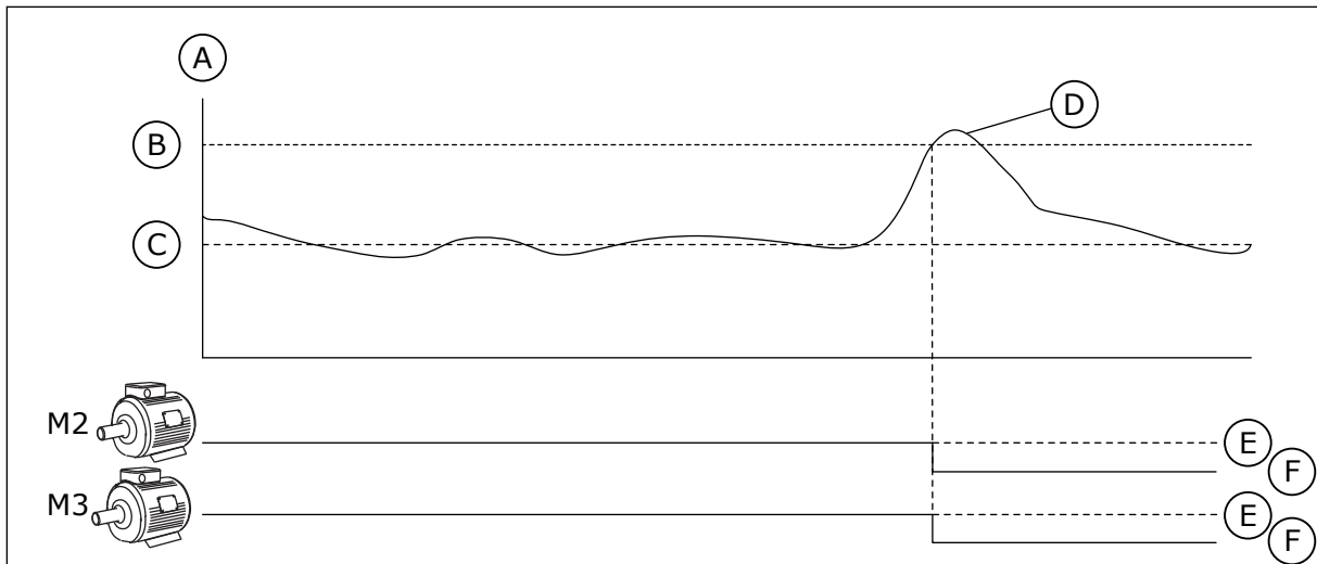
Afb. 86: De functie Overdrukbevaking
