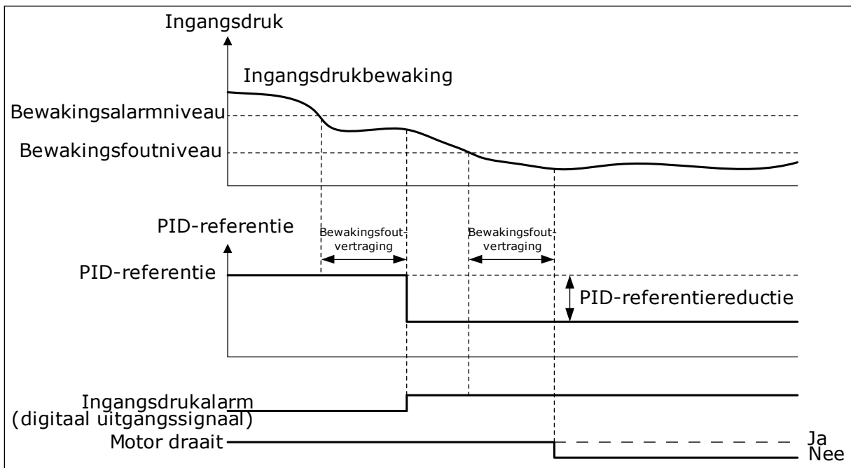
Afb. 79: De functie Ingangsdruk bewaking
