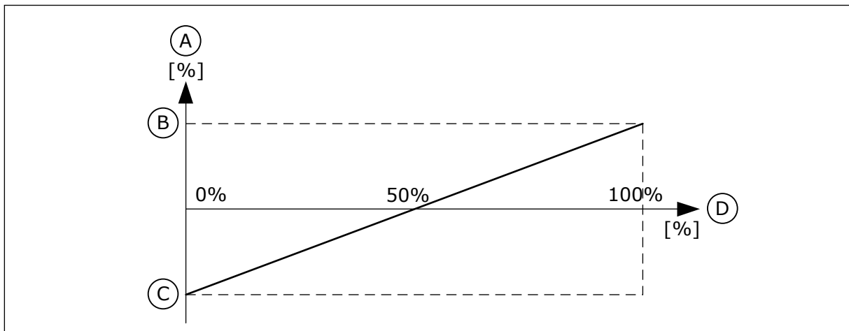
Afb. 34: Schaling van het koppelreferentiesignaal
