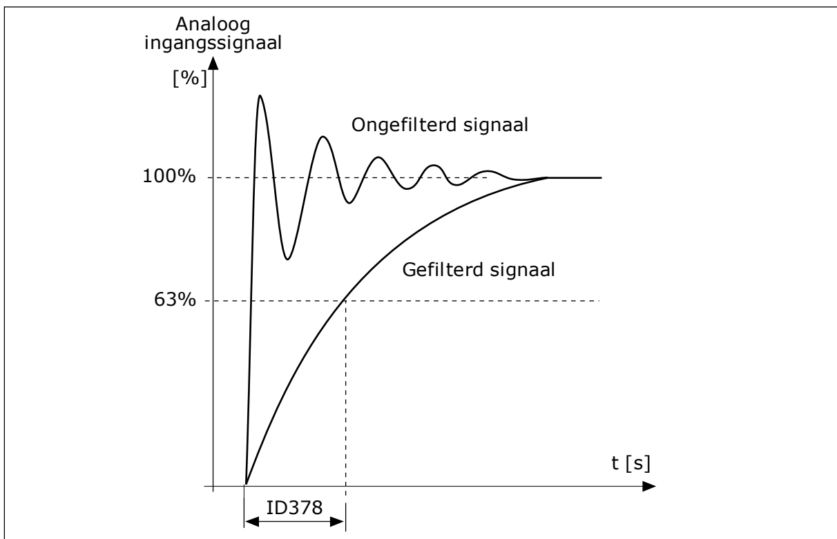
Afb. 47: Het AI1-signaalfilter
