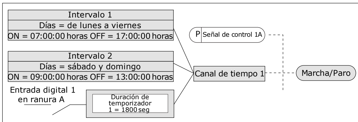
Imag. 69: El canal de tiempo 1 se utiliza como señal de control para la orden de marcha en lugar de una entrada digital
