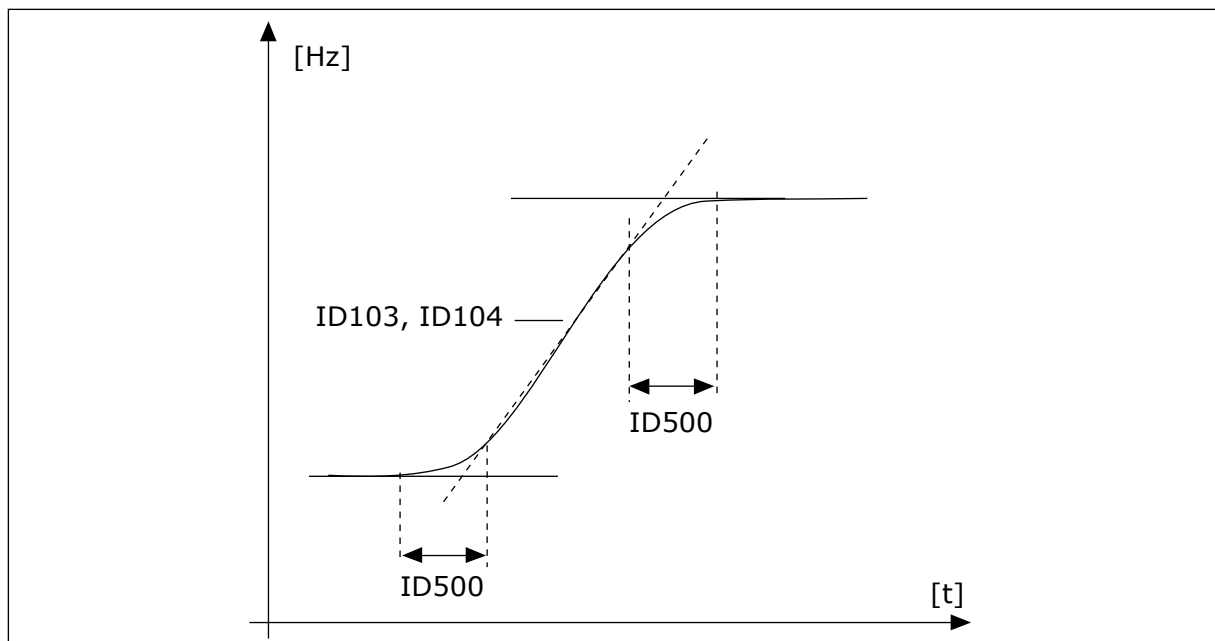
Bild 40: Acceleration/retardation (S-formad)
