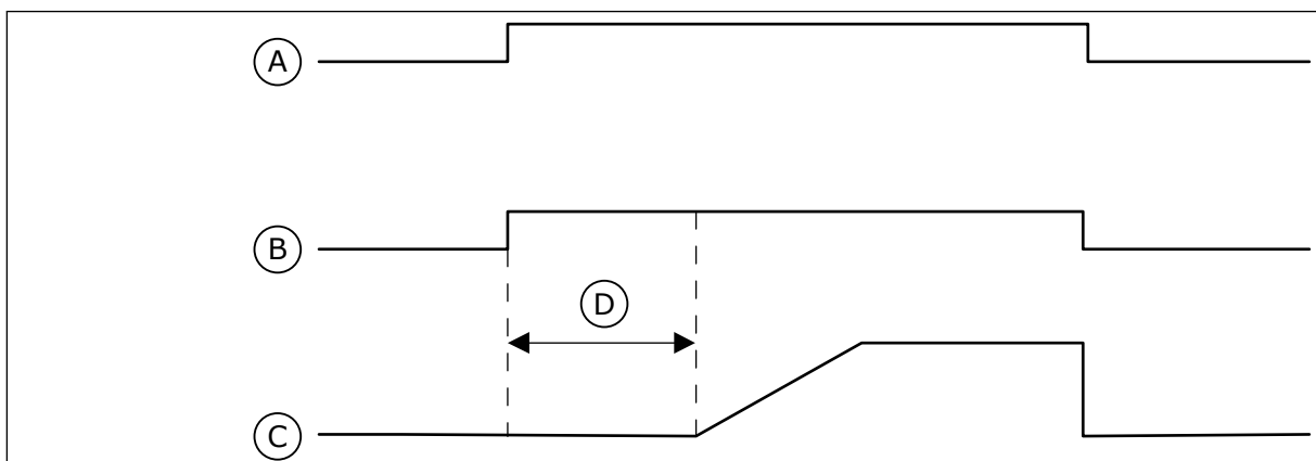
Bild 93: Primingpumpfunktionen
