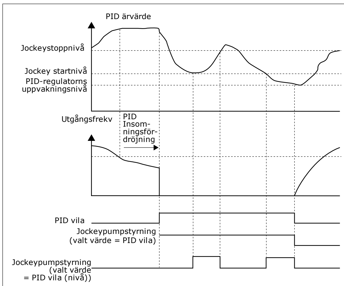
Bild 92: Jockeypumpfunktionen
