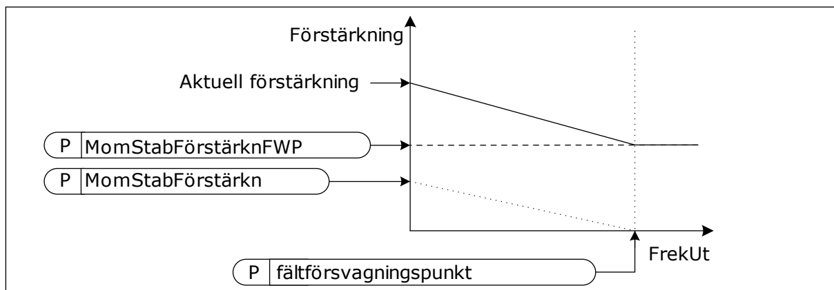
Bild 26: Momentstabilisatorförstärkningen
