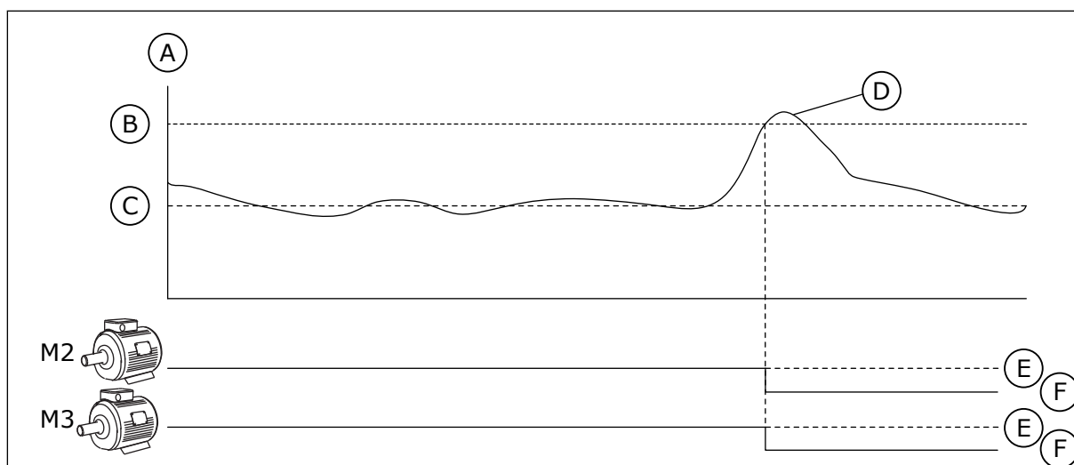
Bild 86: Övertrycksfunktionen
