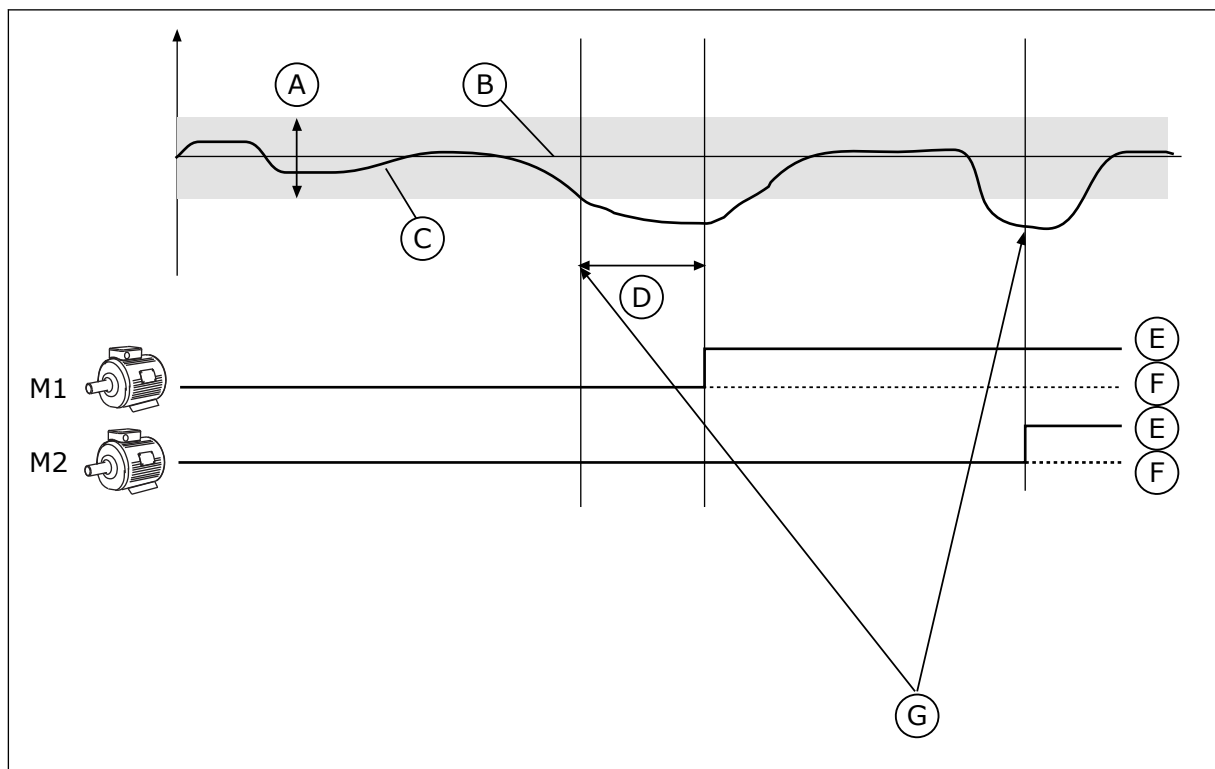
Obr. 80: Funkce multi-čerpádlá
