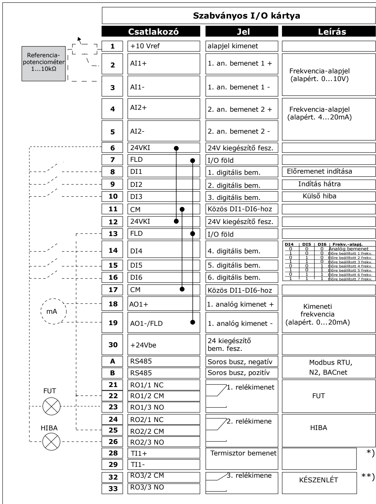
Ábra 8: A Több lépcsős sebesség alkalmazás alapértelmezett vezérlőcsatlakozásai
