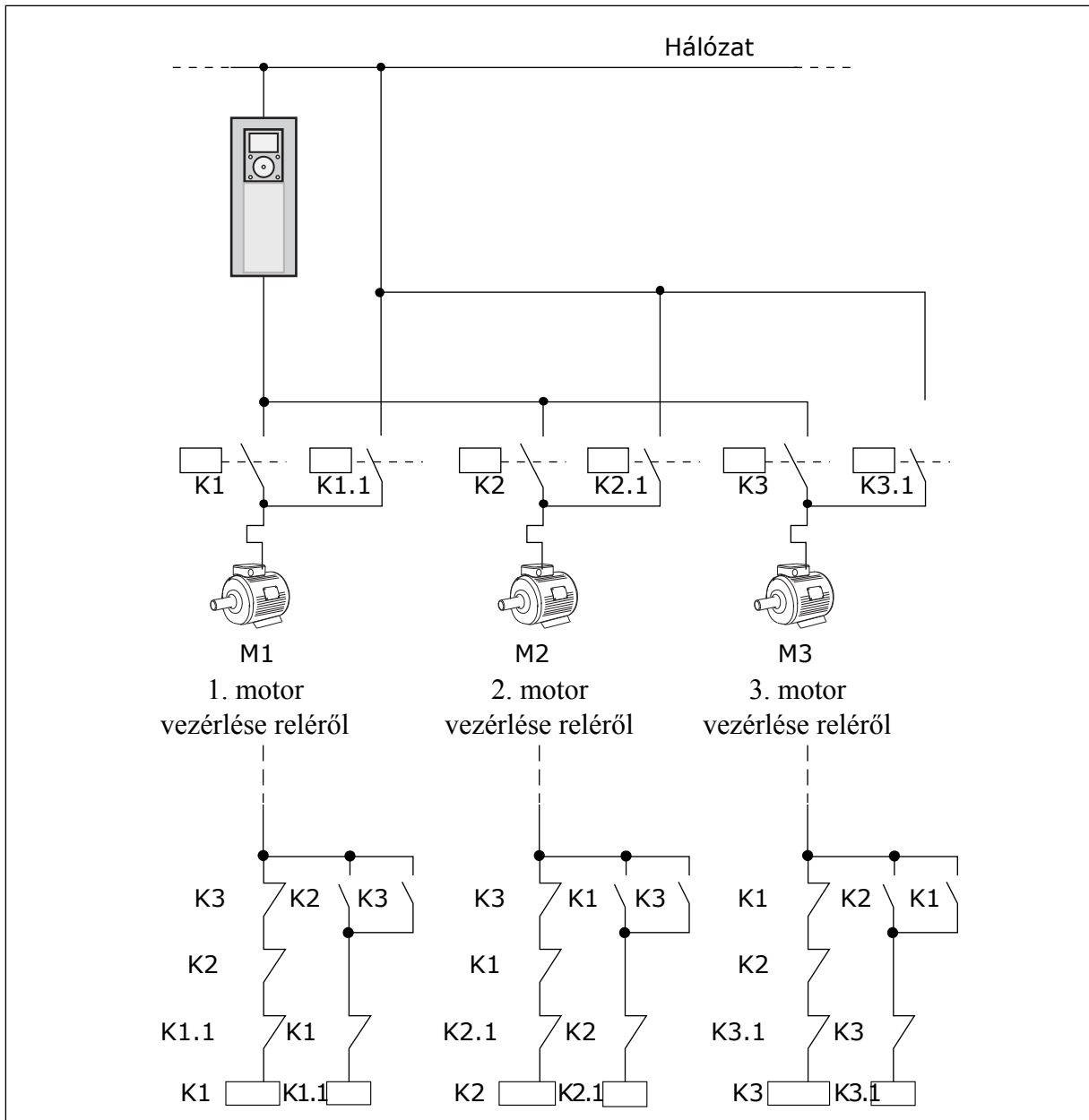
Ábra 85: 1 beállítva
