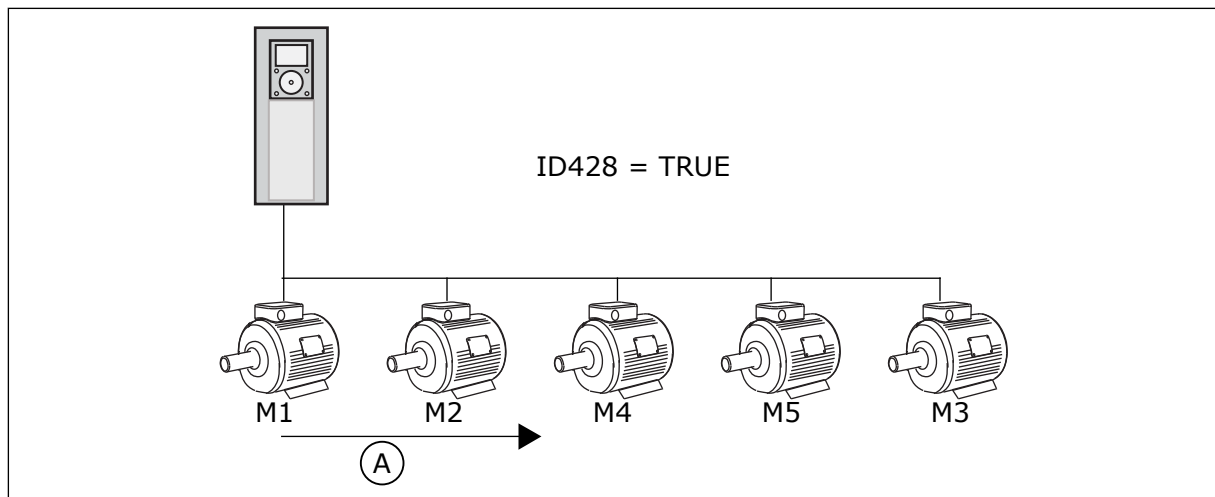
Ábra 83: Az 3. reteszlogika
