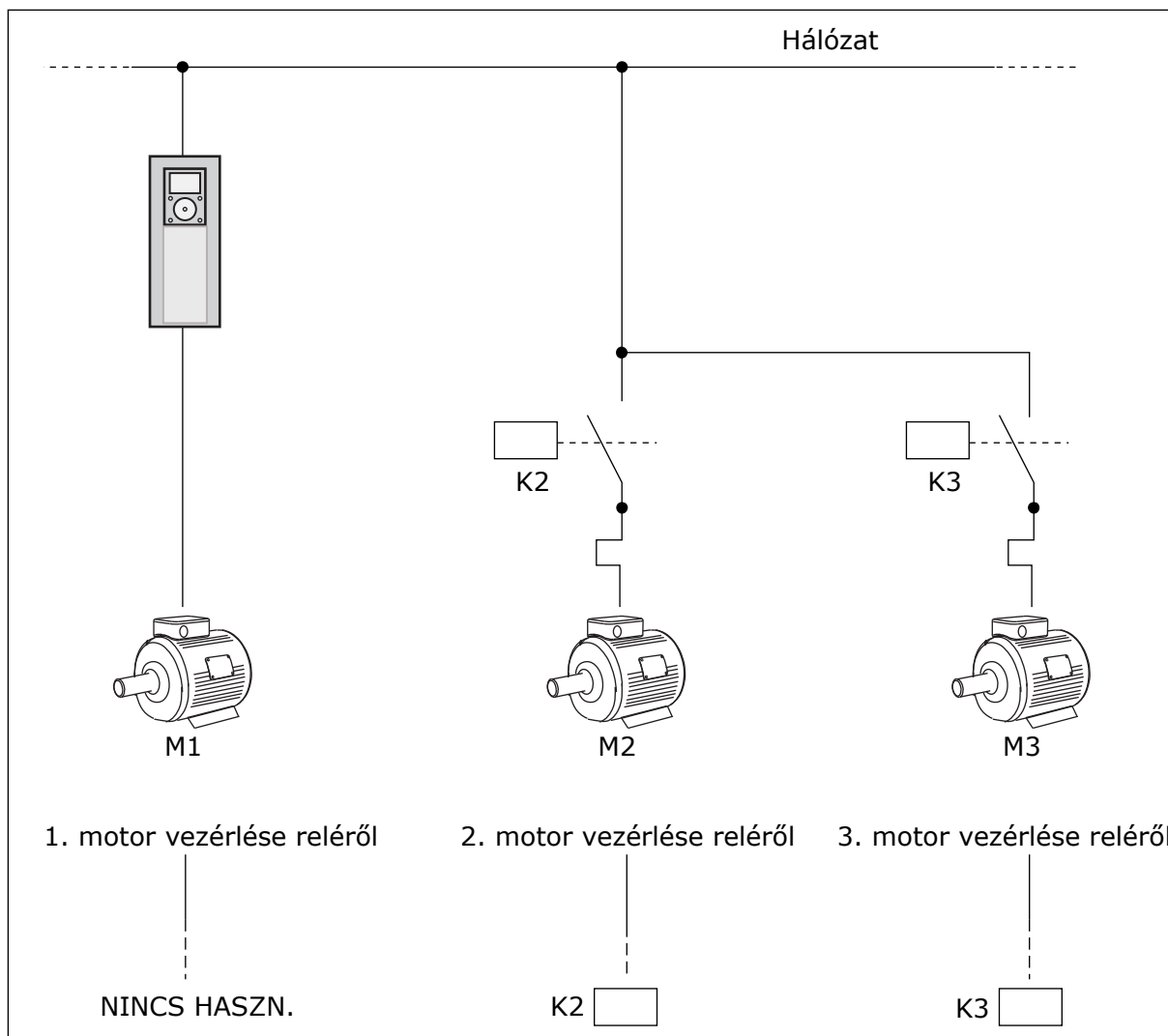
Ábra 84: 0 beállítva
