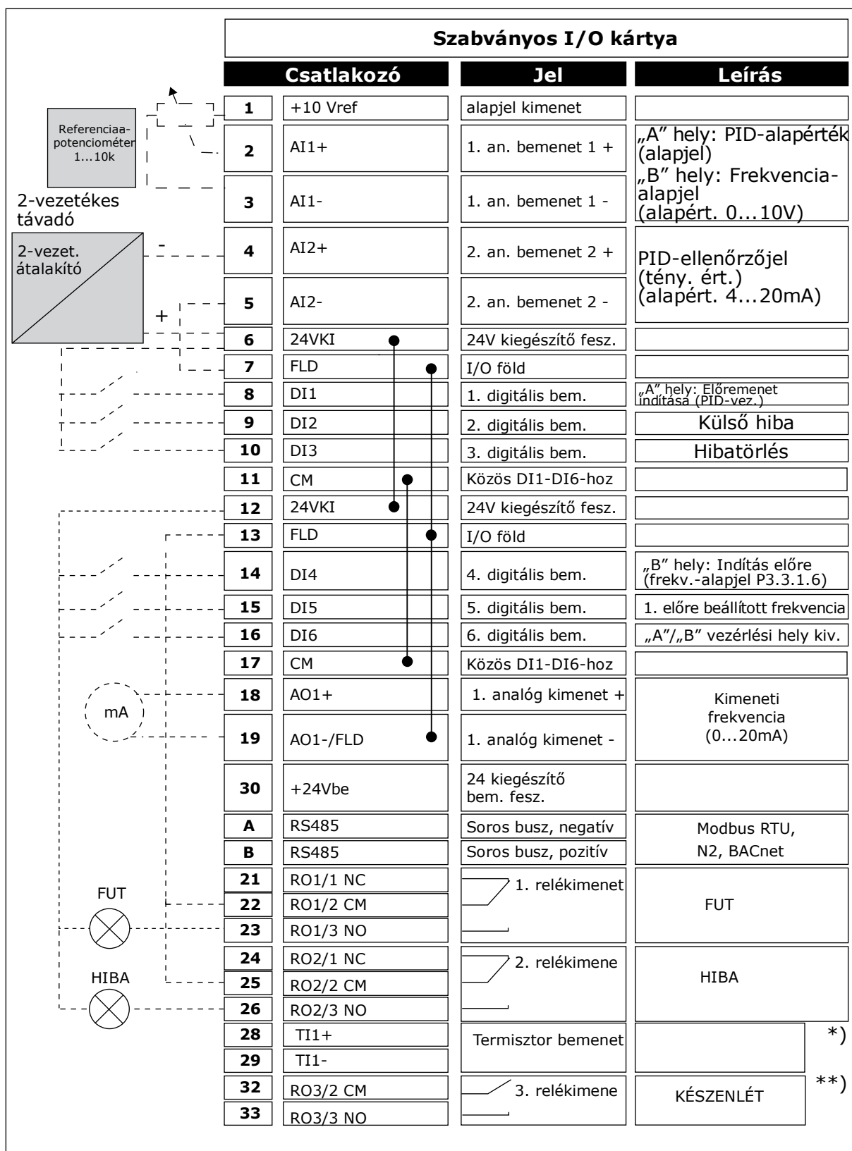
Ábra 10: A PID-szabályzó alkalmazás alapértelmezett vezérlőcsatlakozásai
