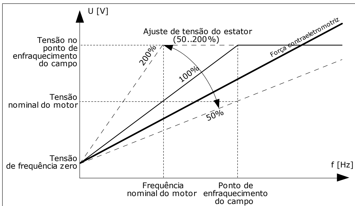
Fig. 22: O ajuste de tensão do estator
