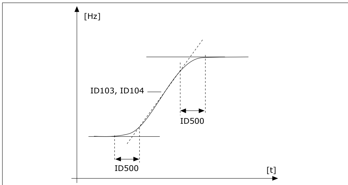
Fig. 41: A curva de aceleração/desaceleração (em forma de S)
