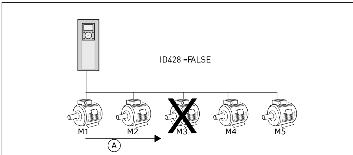
Fig. 82: A lógica de travamento 2
