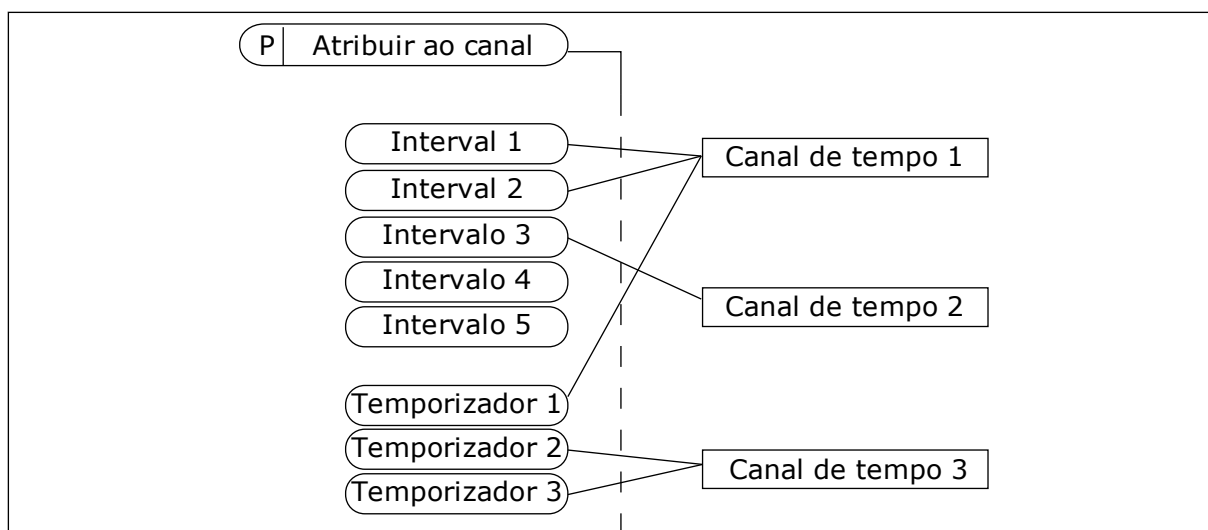
Fig. 64: A atribuição de intervalos e temporizadores aos canais de tempo é flexível. Cada intervalo e temporizador tem um parâmetro com o qual você pode atribuí-lo a um canal de tempo.
