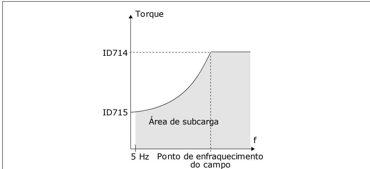
Fig. 60: Configuração da carga mínima
