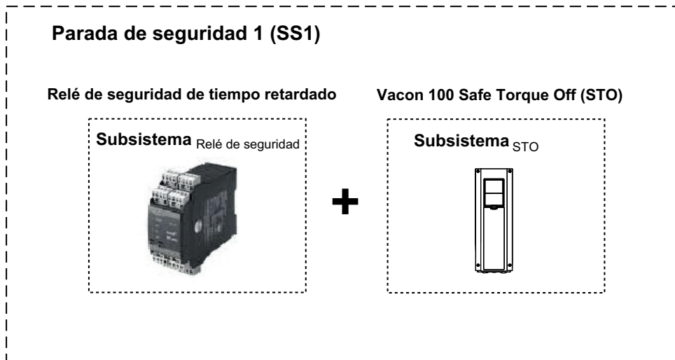
Figura 7. Función de seguridad Parada de seguridad 1 (SS1)
