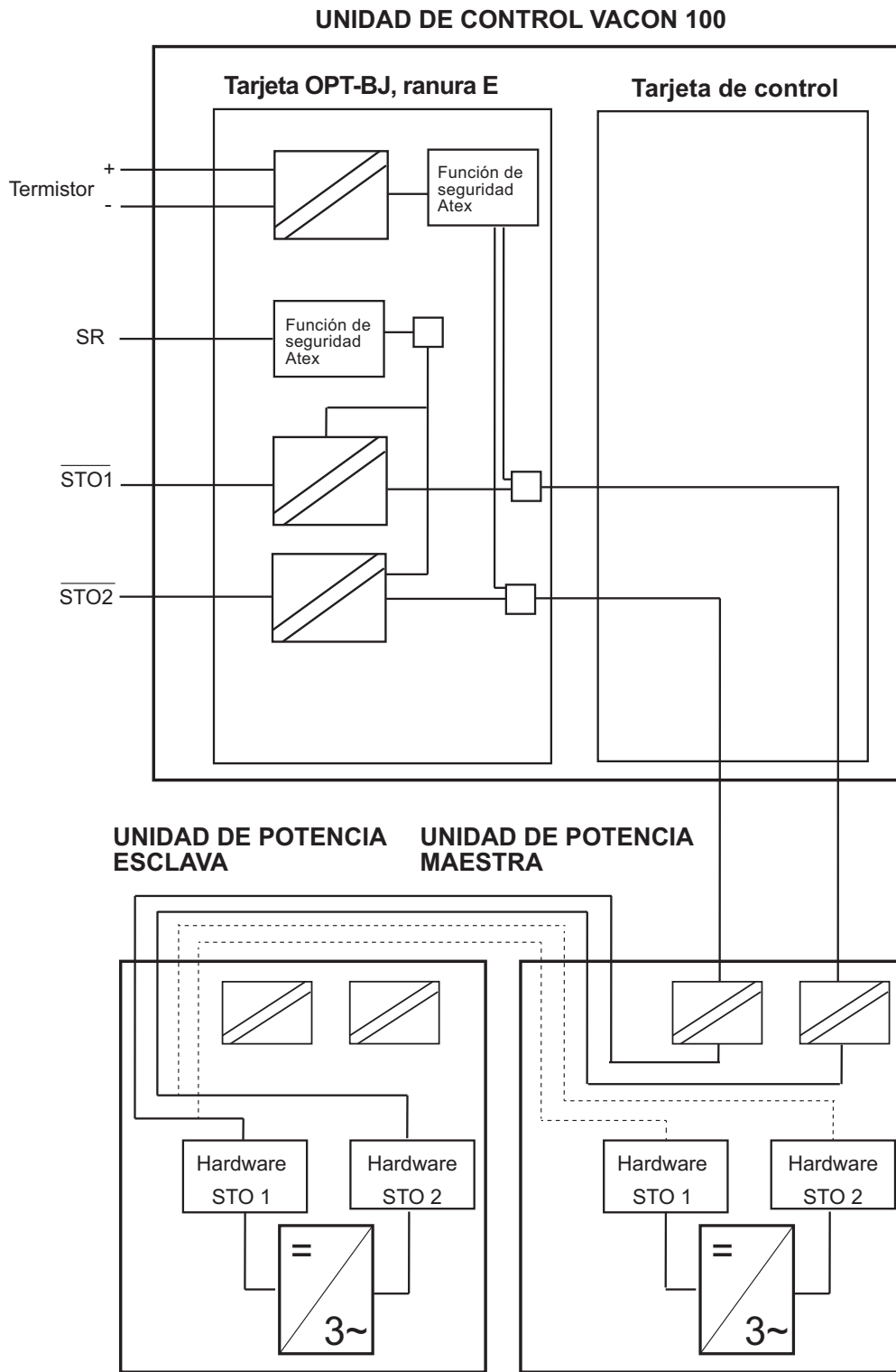
Figura 5. Principio de STO con la tarjeta OPTBJ y la tarjeta de control Vacon 100, MR12
