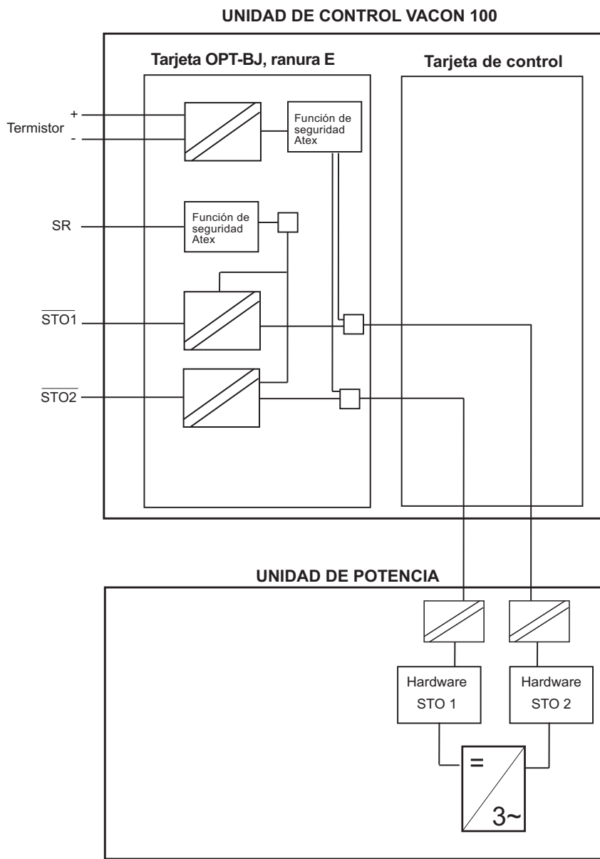
Figura 9. Principio de la función del termistor en el convertidor de frecuencia Vacon 100 con la tarjeta OPTBJ, MR4-10
