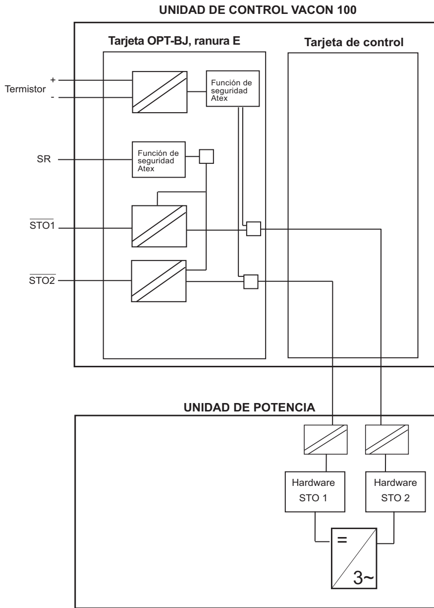
Figura 4. Principio de STO con la tarjeta OPTBJ y la tarjeta de control Vacon 100, MR4-10
