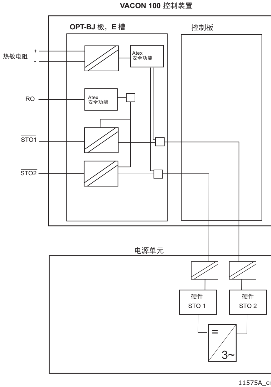
图 9. 在配备 OPTBJ 板 MR4-10 的 Vacon 100 交流变频器中，热敏电阻的功能原理
