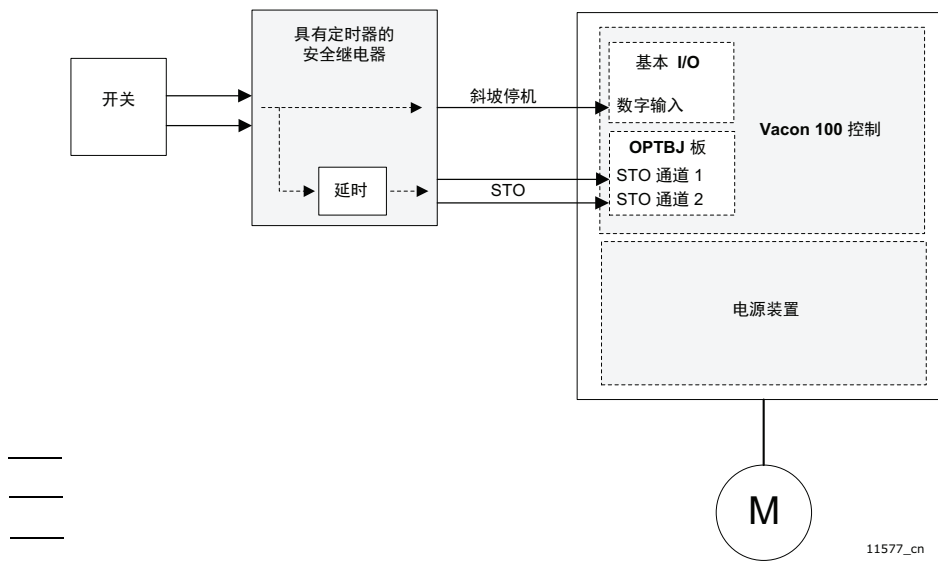
图 8. 安全停机 1 (SS1) 的连接原理
