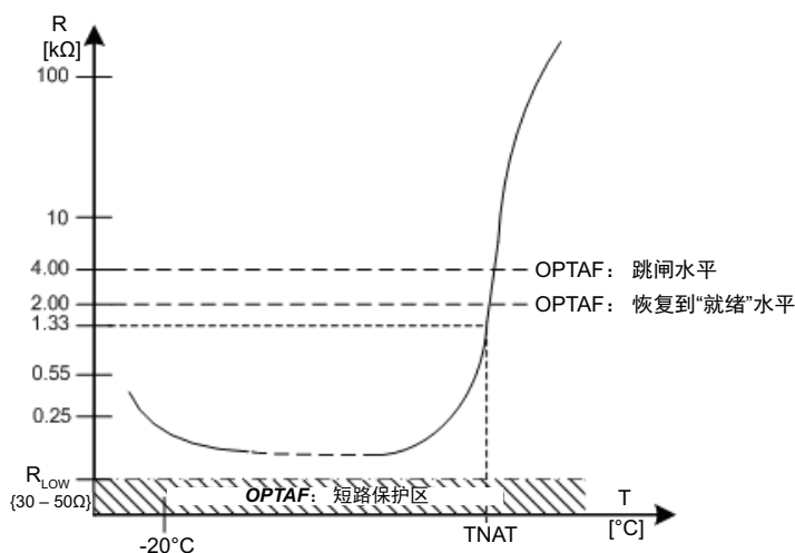
图 11. 有关电机保护传感器的典型特征，请参见 DIN 44081/DIN 440 中的规定
