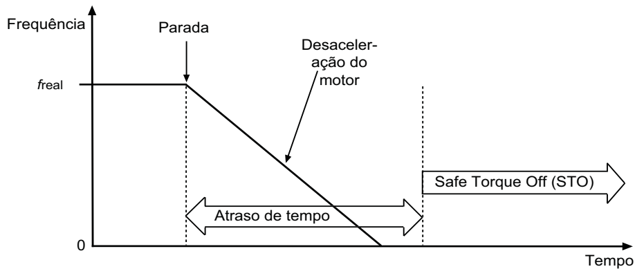
Figura 6. Princípios do Safe Stop 1 (EN 61800-5-2, SS1 tipo c)
