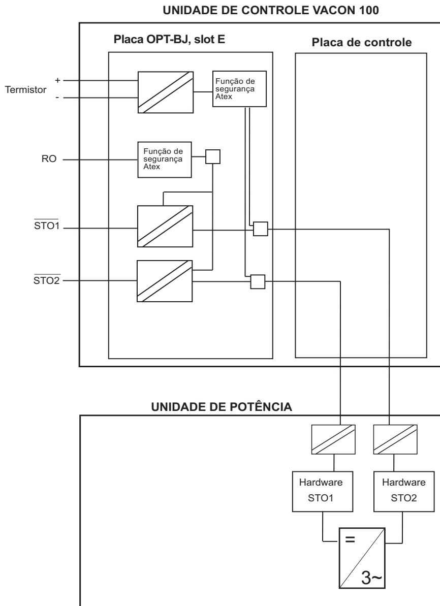
Figura 9. Princípios de funcionamento do conversor de frequência Vacon 100 com a placa OPTBJ, MR4-10
