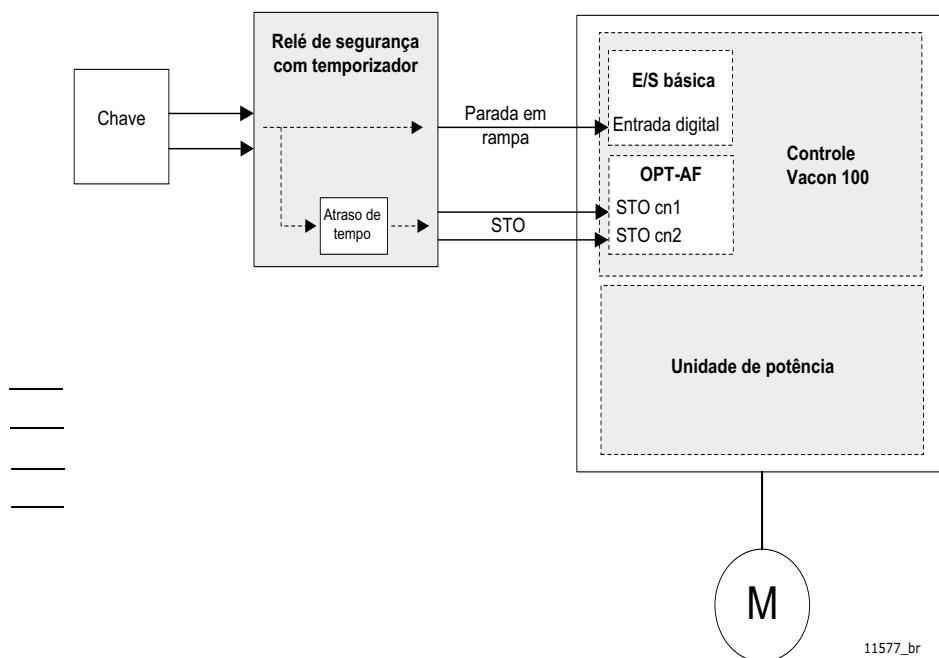
Figura 8. Princípios de conexão do Safe Stop 1 (SS1)
