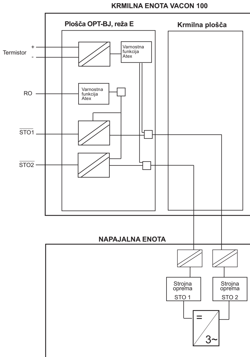
Slika 9. Termistorsko načelo delovanja v frekvenčnem pretvorniku Vacon 100 s ploščo OPTBJ, MR4-10
