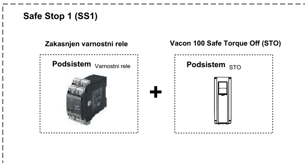
Slika 7. Varnostna funkcija Safe Stop 1 (SS1)
