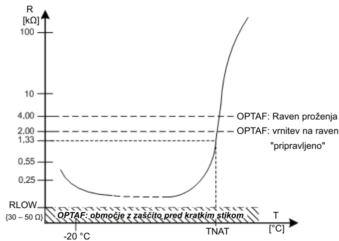
Slika 11. Tipične značilnosti senzora za zaščito motorja, kot je določeno v standardu DIN 44081/DIN 440
