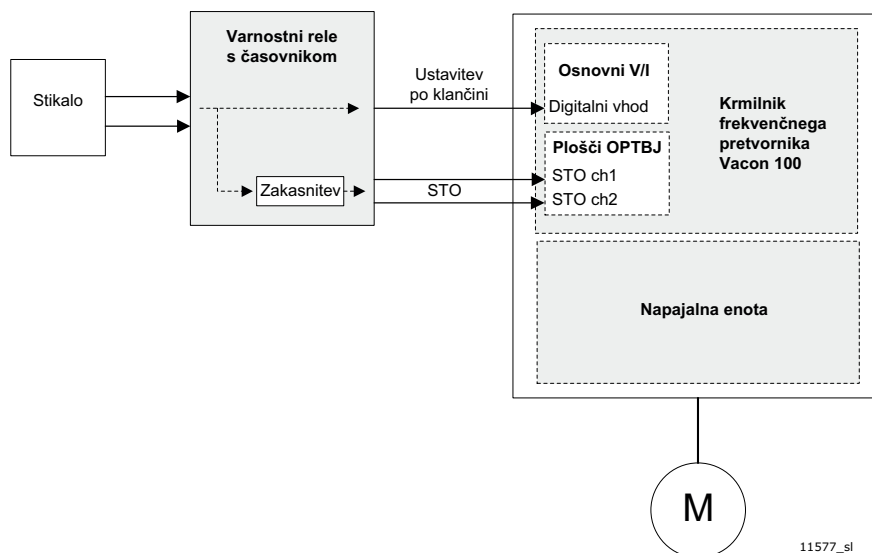
Slika 8. Načelo priključitve funkcije Safe Stop 1 (SS1)
