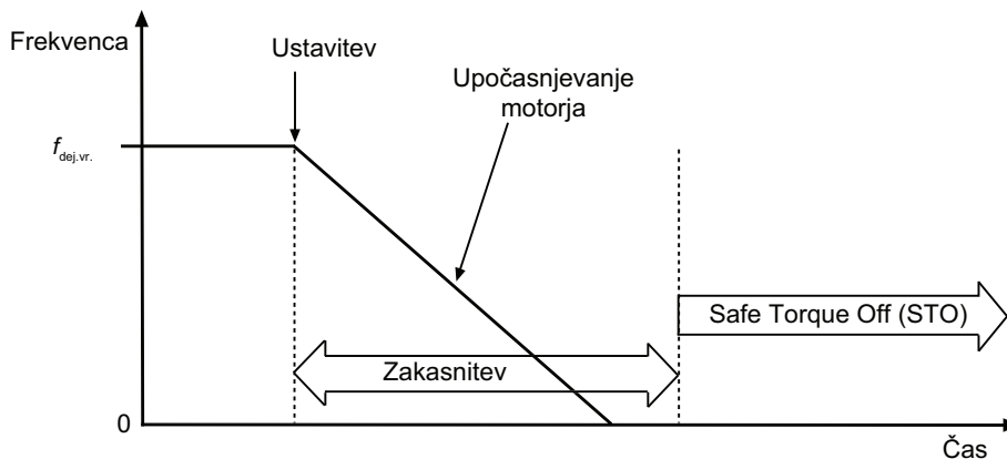
Slika 6. Načelo Safe Stop 1 (EN 61800-5-2, SS1 vrste c)
