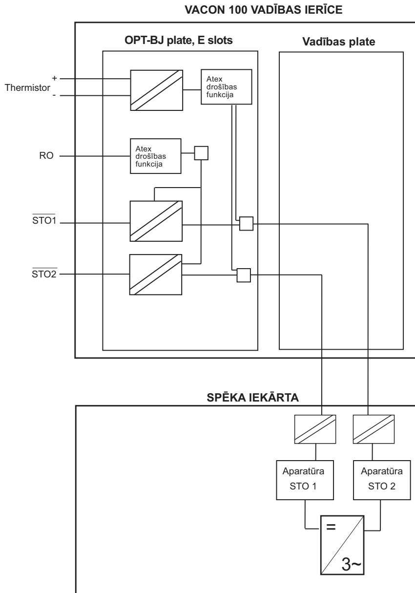
9. attēls. Termistora funkcijas princips Vacon 100 frekvences pārveidotājā ar OPTBJ paneli, MR4-10
