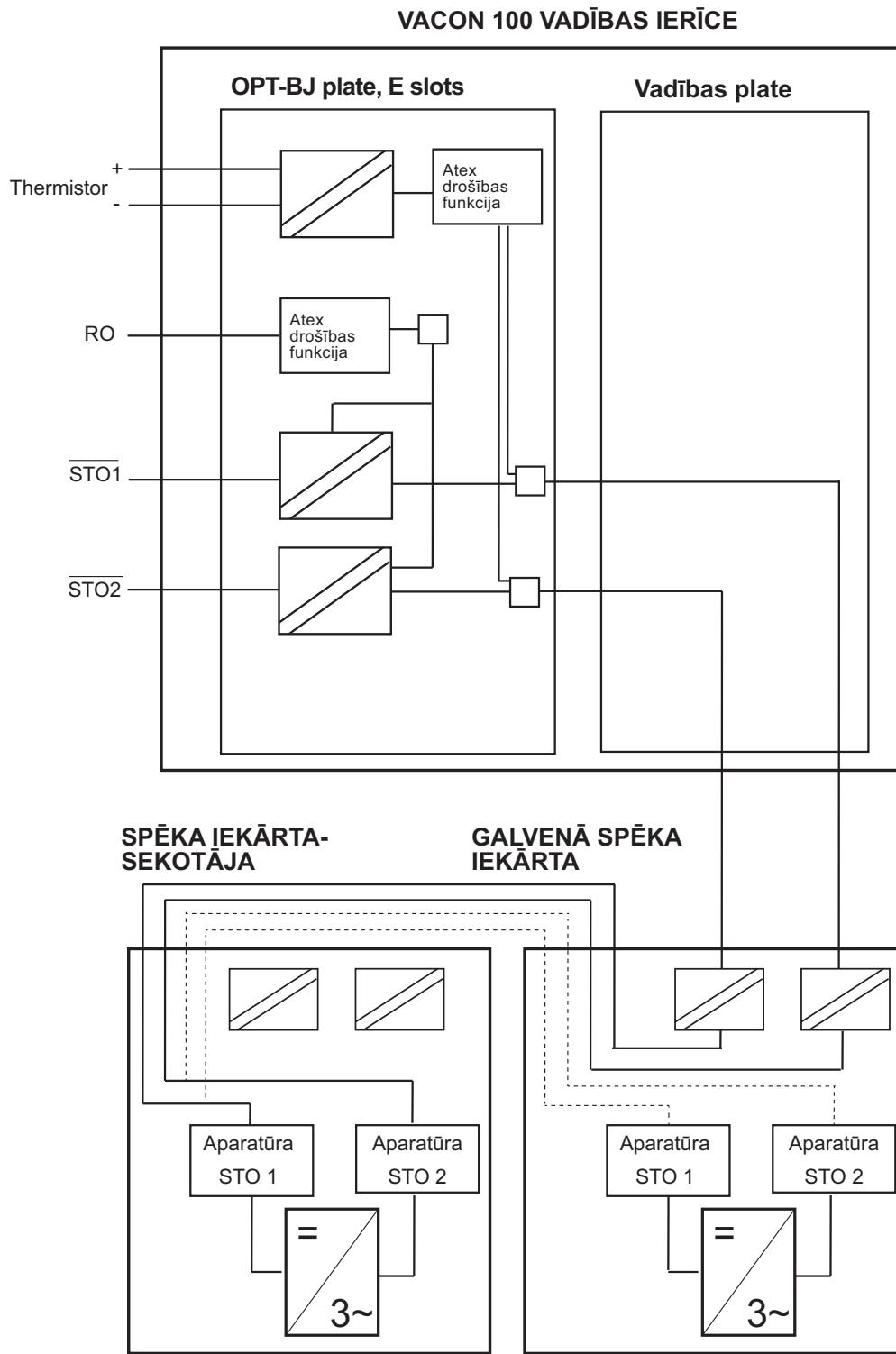
5. attēls. STO princips ar OPTBJ paneli un Vacon 100 vadības paneli MR12
