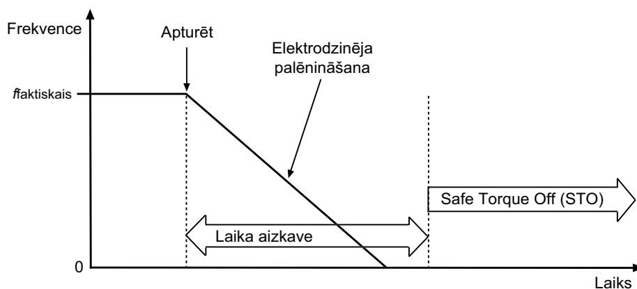
6. attēls. Safe Stop 1 princips (EN 61800-5-2, SS1 tips c)
