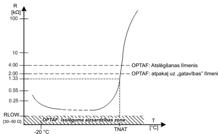
11. attēls. Elektrodzinēja aizsardzības sensora tipiskie raksturlielumi, kā norādīts standartā DIN 44081/DIN 440
