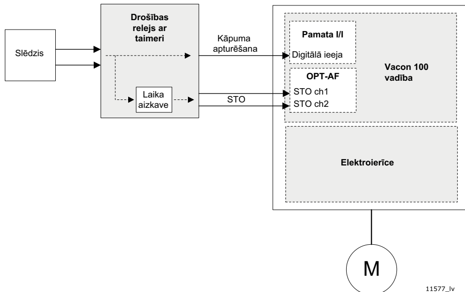
8. attēls. Safe Stop 1 savienojuma princips (SS1)
