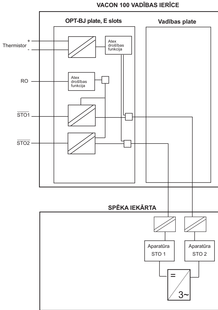
4. attēls. STO princips ar OPTBJ paneli un Vacon 100 vadības paneli MR4-10
