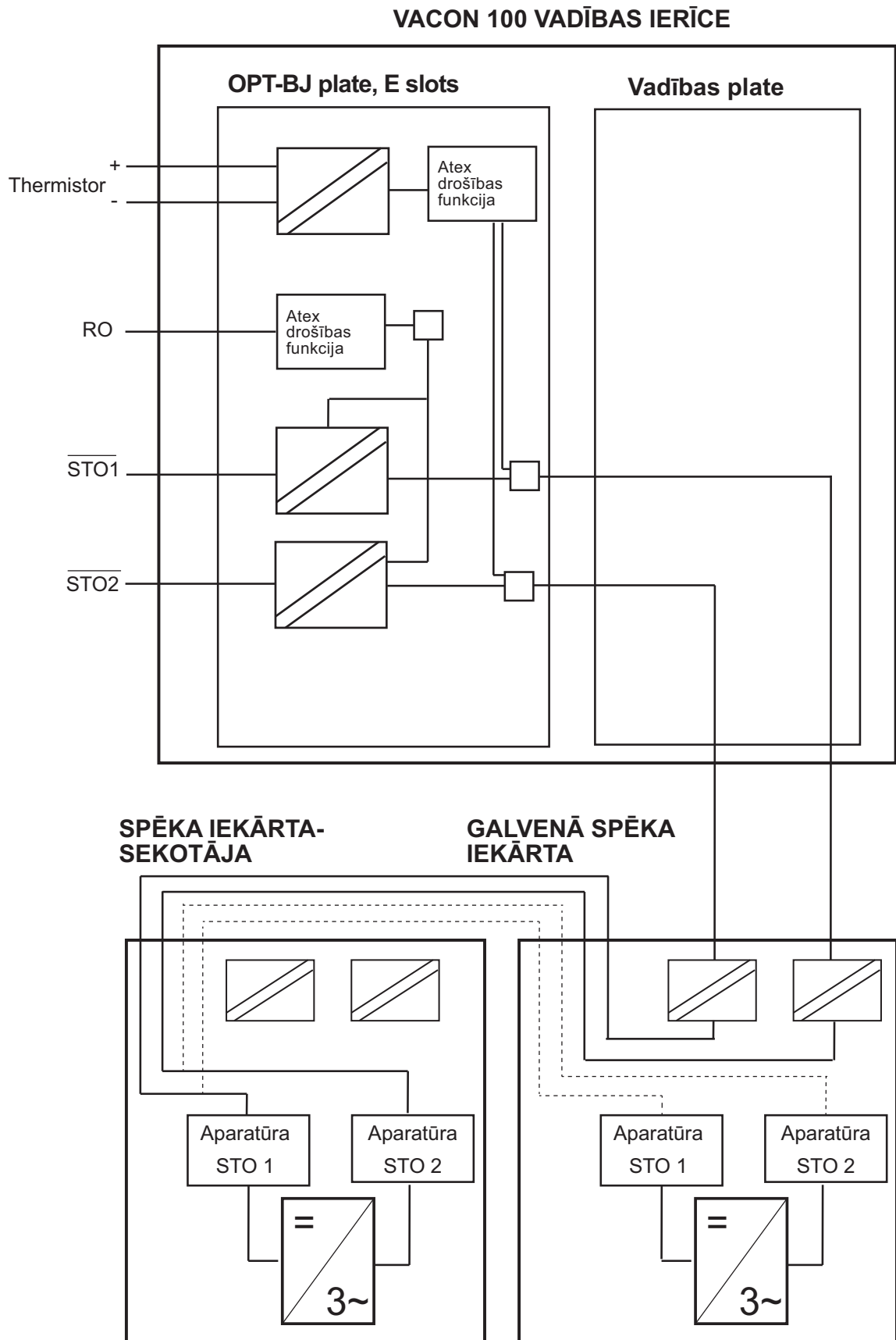
10. attēls. STO princips ar OPTBJ paneli un Vacon 100 vadības paneli MR12
