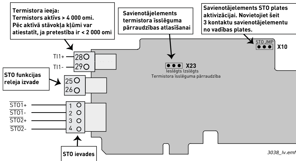
1. attēls. OPTBJ paneļa izkārtojums
