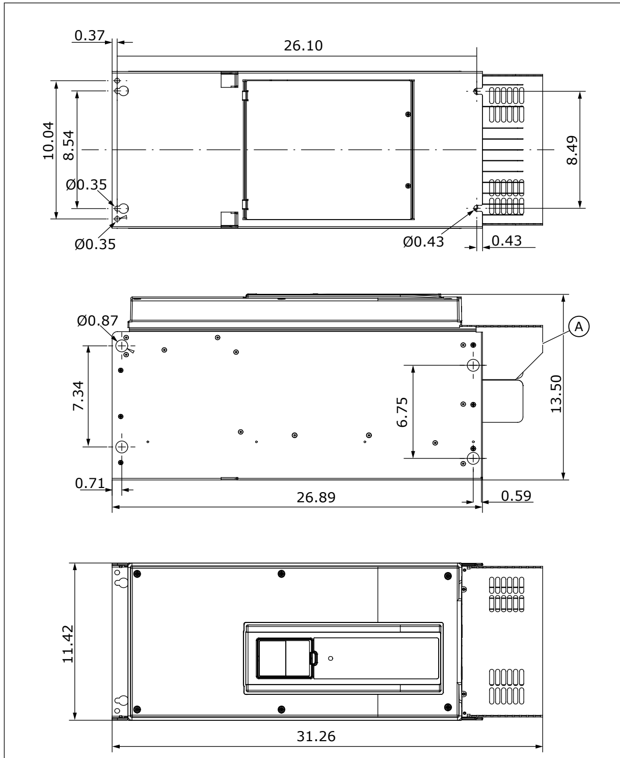
图 15: 交流变频器的尺寸 [in]，MR8，UL 开放型
