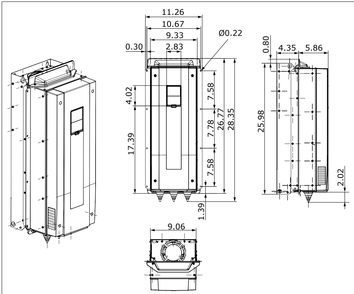
Σχ. 30: Οι διαστάσεις του ρυθμιστή στροφών AC, στερέωση σε φλάντζα, MR7 [in]
