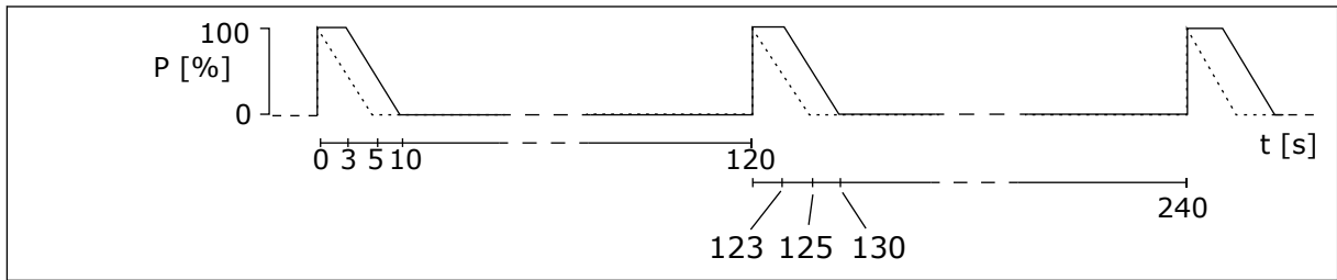
Şekil 49: LD ve HD palslerinin görev döngüleri
