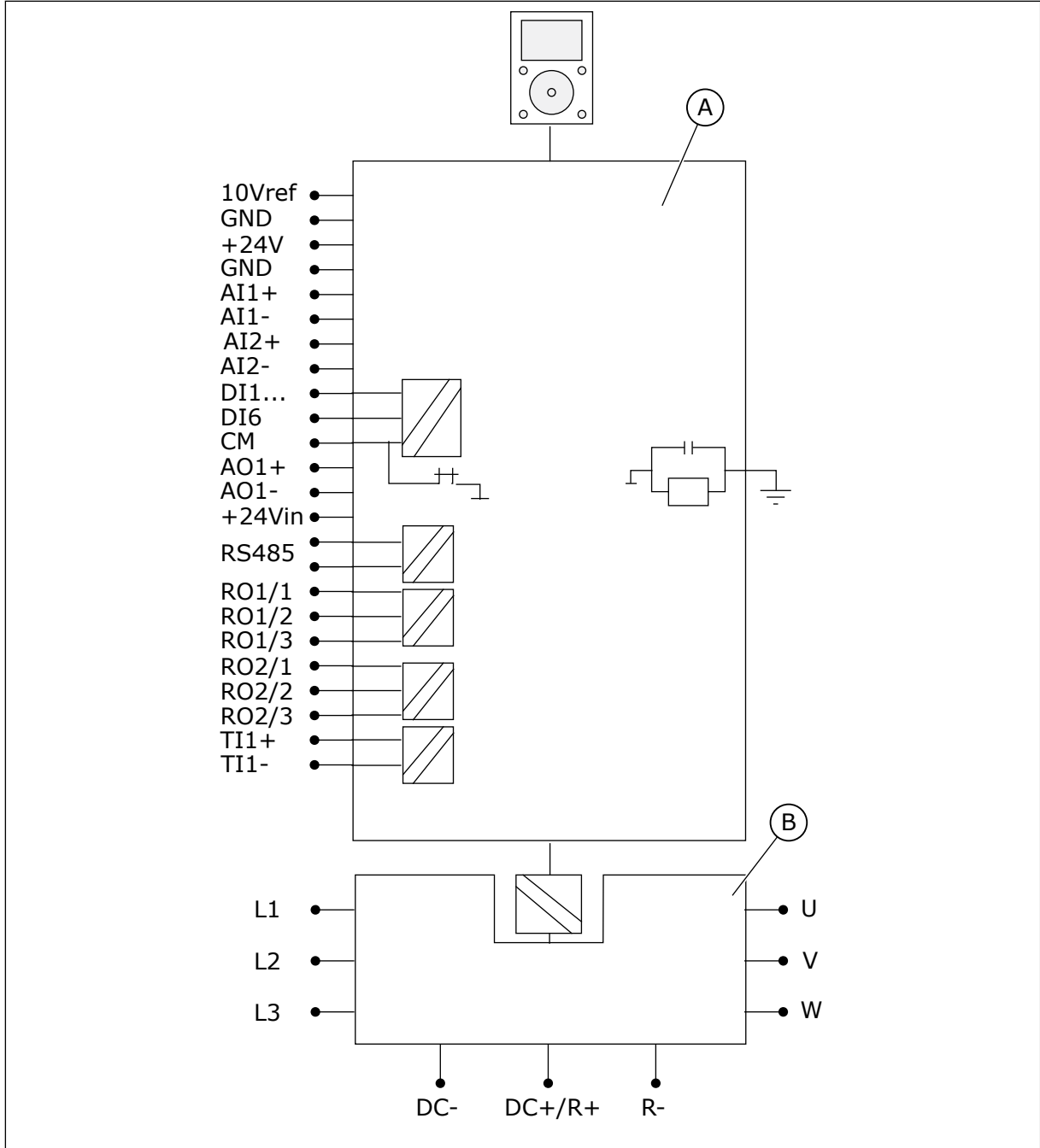
Şekil 45: Galvanik yalıtım bariyerleri
