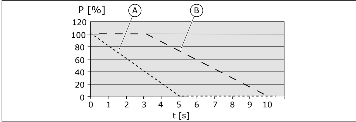
Şekil 48: LD ve HD palsleri, P = fren gücü
