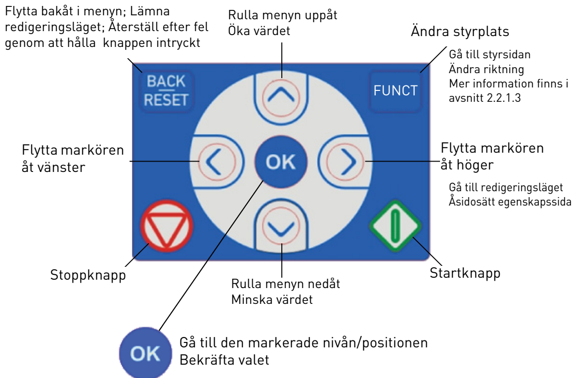
Figur 1. Manöverpanelens knappar
