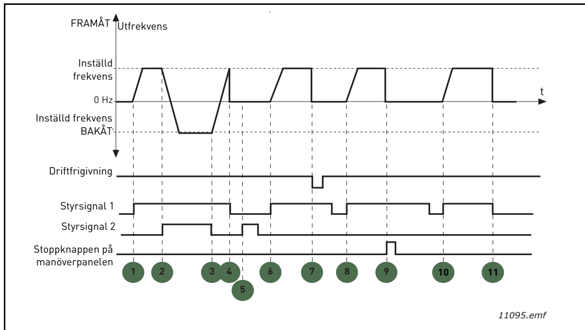
Figur 23. Start/stopp-logik för I/O A = 4
