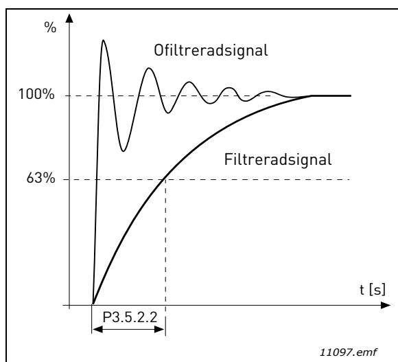
Figur 25. AI1 signalfiltrering
