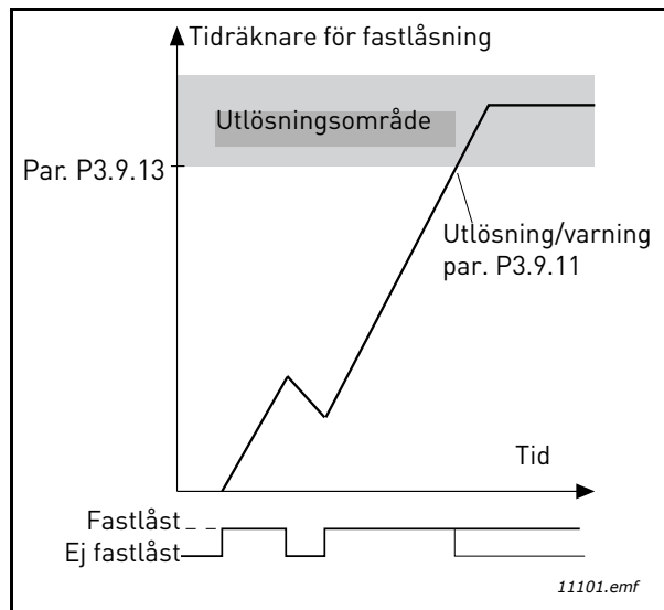
Figur 29. Tidräkning för fastlåsning
