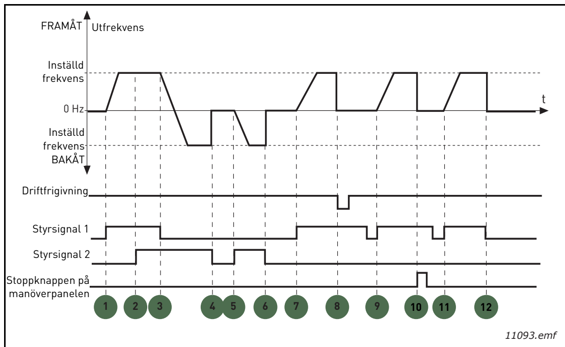
Figur 21. Start/stop-logik för I/O A = 2
