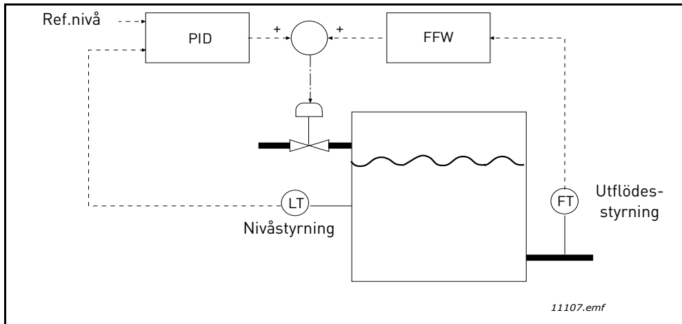
Figur 35. Framkopplingsstyrning
