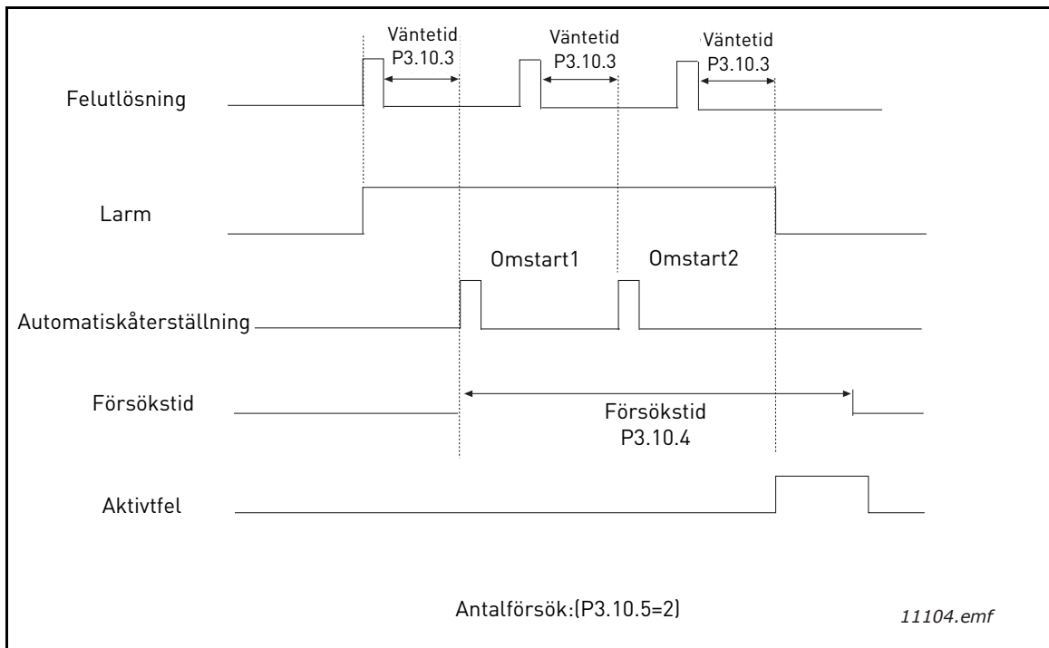
Figur 32.Funktionen automatisk återställning
