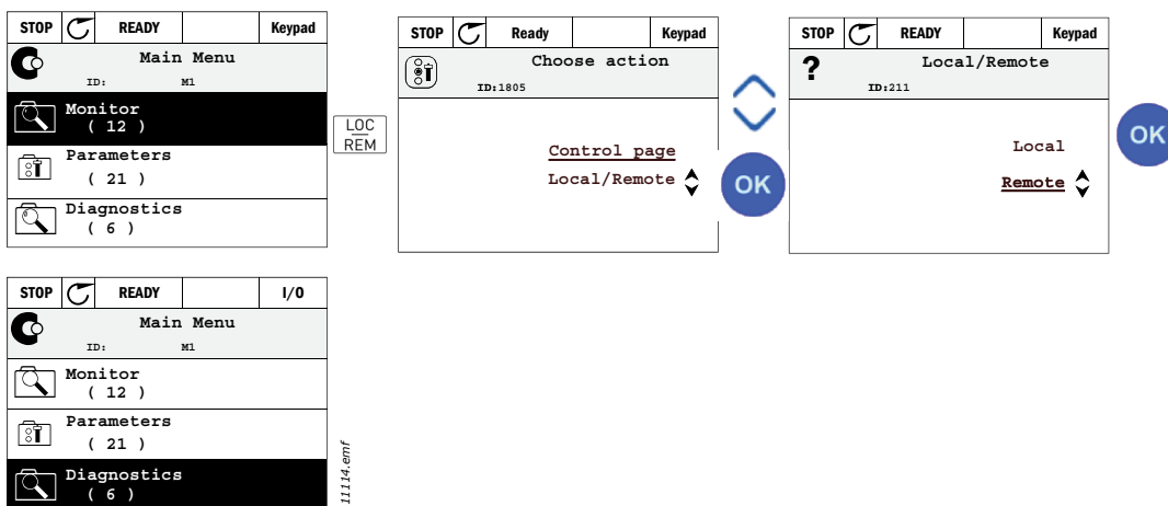
Рис. 4. Переключение между источниками управления
