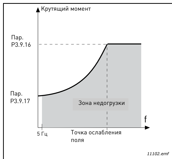
Рис. 30. Установка минимальной нагрузки
