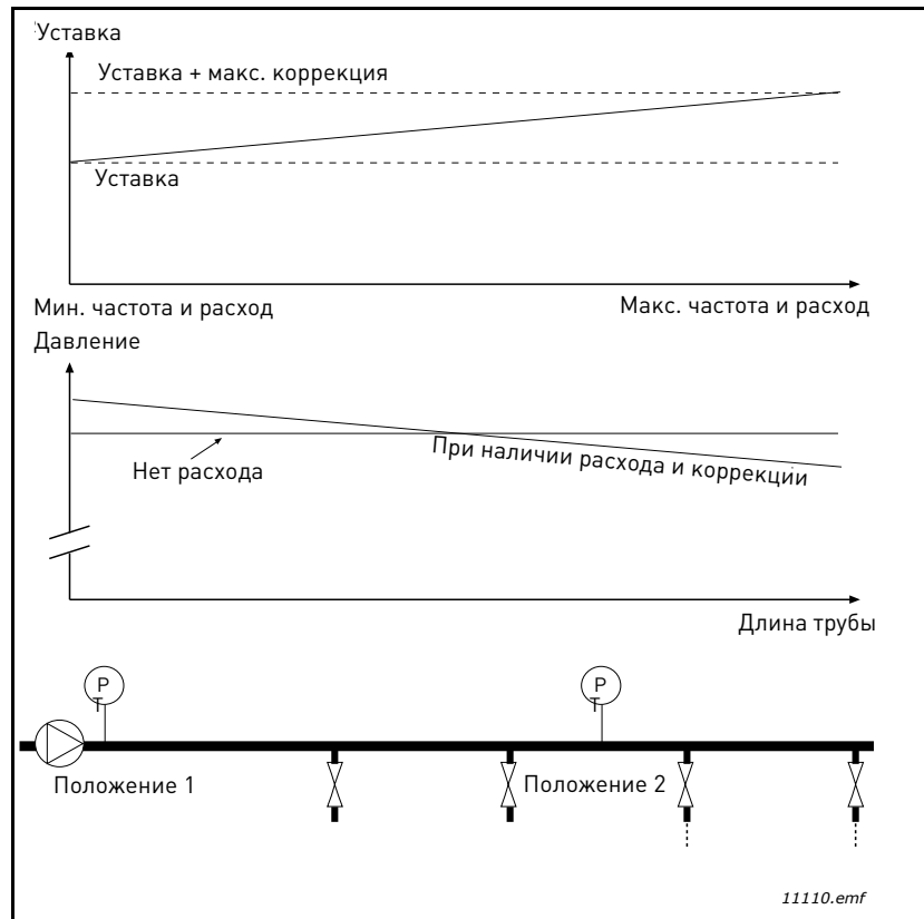
Рис. 38. Разрешает уставку 1 для коррекции падения давления
