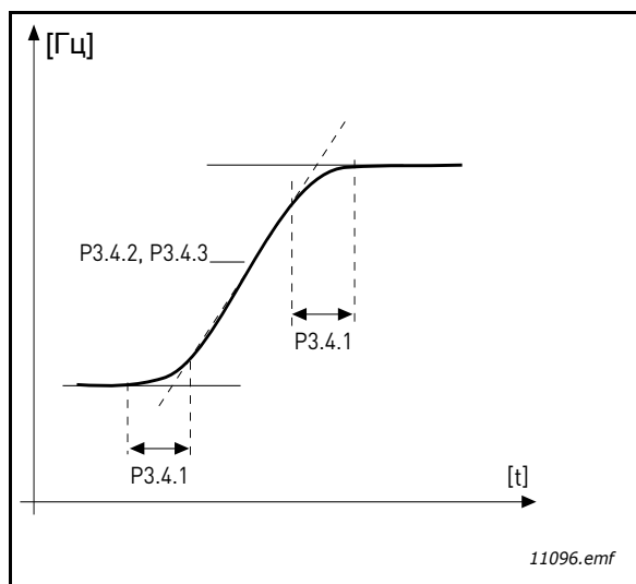
Рис. 24. Разгон/замедление (S-образная характеристика)
