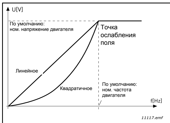
Рис. 18. Линейное и квадратичное изменение напряжения двигателя
