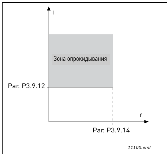
Рис. 28. Настройка характеристик опрокидывания
