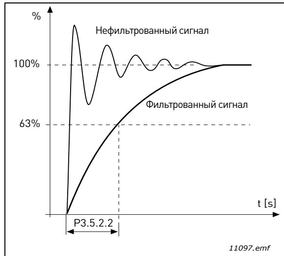
Рис. 25. Фильтрация сигнала АВХ1
