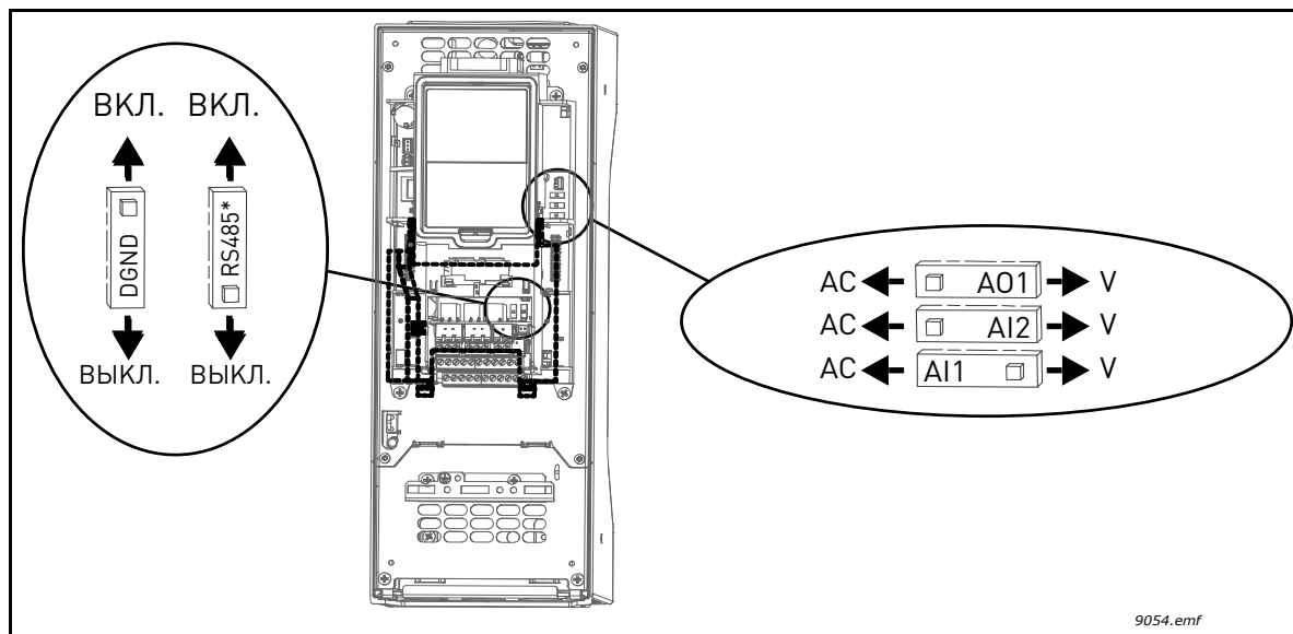
Рис. 13. DIP-переключатели и их настройки по умолчанию. * Согласующий резистор шины
