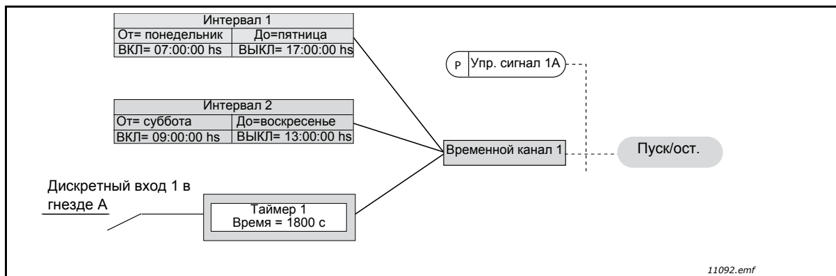
Рис. 17. Окончательная конфигурация, в которой временной канал 1 используется как сигнал управления для запуска вместо дискретного входа.
