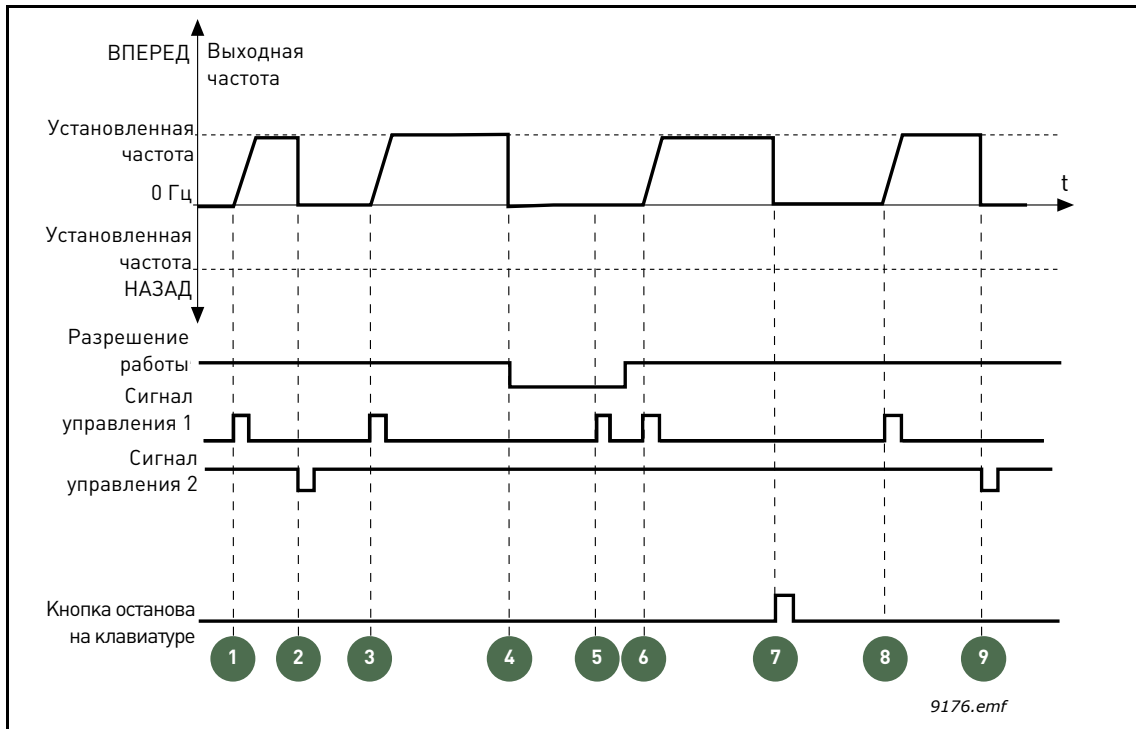
Рис. 20. Логика пуска/останова от платы ввода/вывода A = 1
