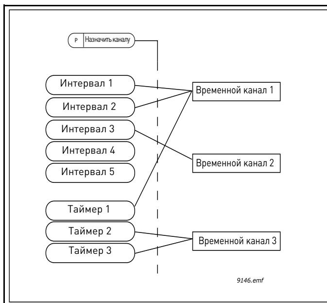
Рис. 15. Имеется возможность гибкого назначения интервалов и таймеров для временных каналов. Каждый интервал и таймер имеет собственный параметр для назначения временному каналу.
