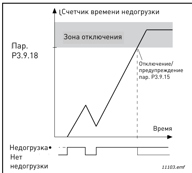
Рис. 31. Функция счетчика недогрузки
