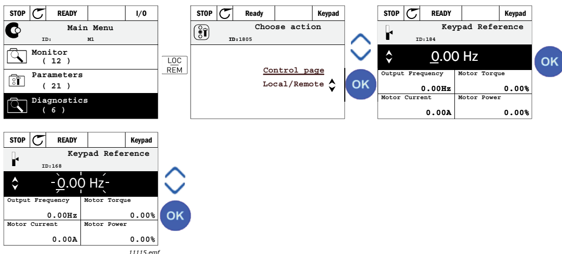
Рис. 5. Вызов страницы управления
