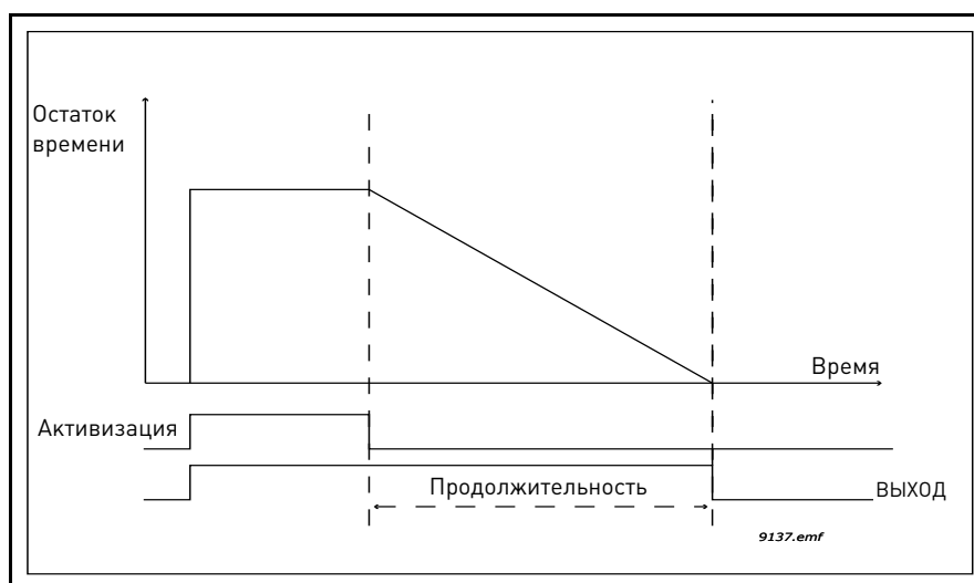
Рис. 16. Сигнал активизации поступает от дискретного входа или виртуального дискретного входа, а именно временного канала. Таймер начинает обратный отсчет от нижнего края сигнала.
