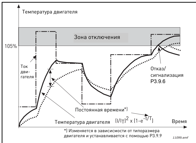
Рис. 27. Расчет температуры двигателя
