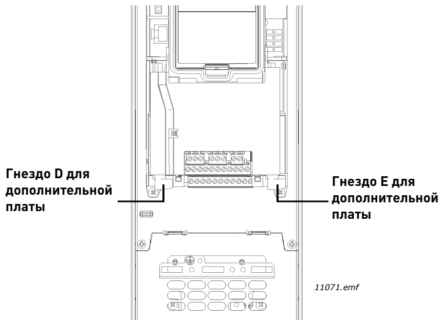
Рис. 14. Гнезда для дополнительных плат
