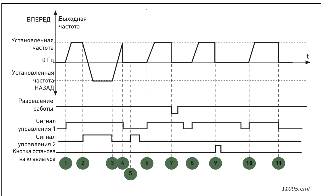
Рис. 23. Логика пуска/останова от платы ввода/вывода А = 4
