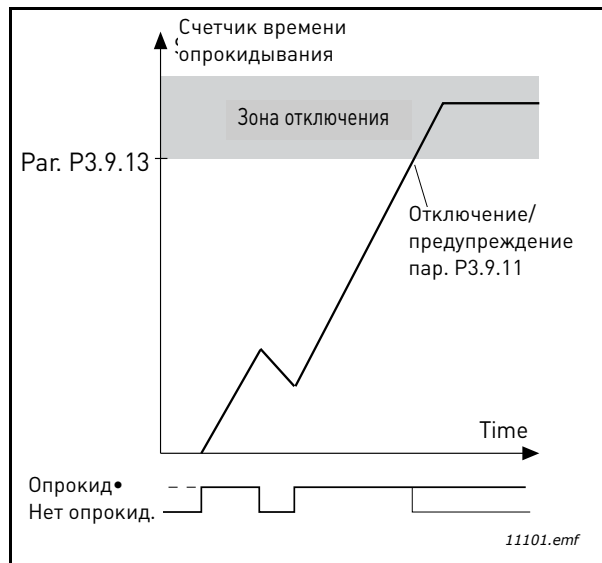
Рис. 29. Счет времени опрокидывания
