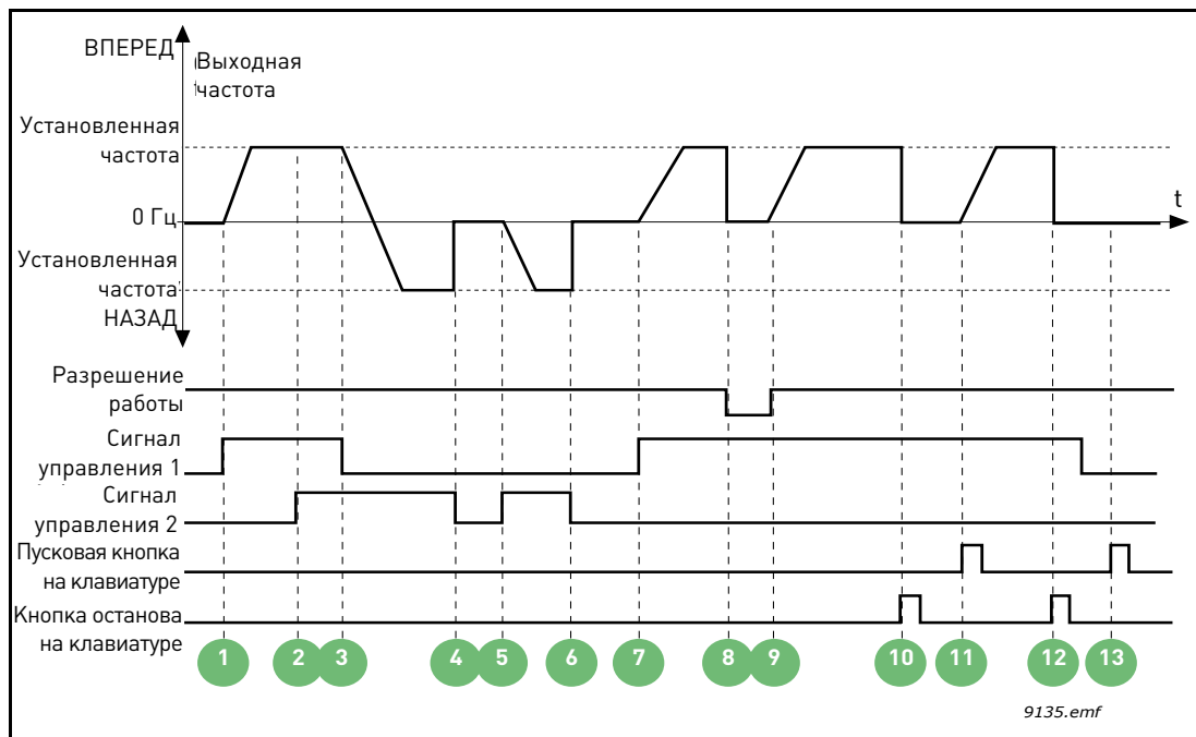
Рис. 19. Логика пуска/останова от платы ввода/вывода A = 0
