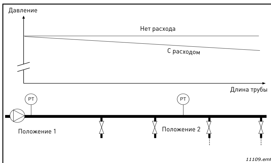
Рис. 37. Размещение датчика давления
