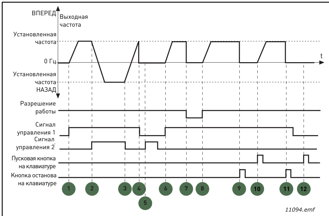
Рис. 22. Логика пуска/останова от платы ввода/вывода A = 3
