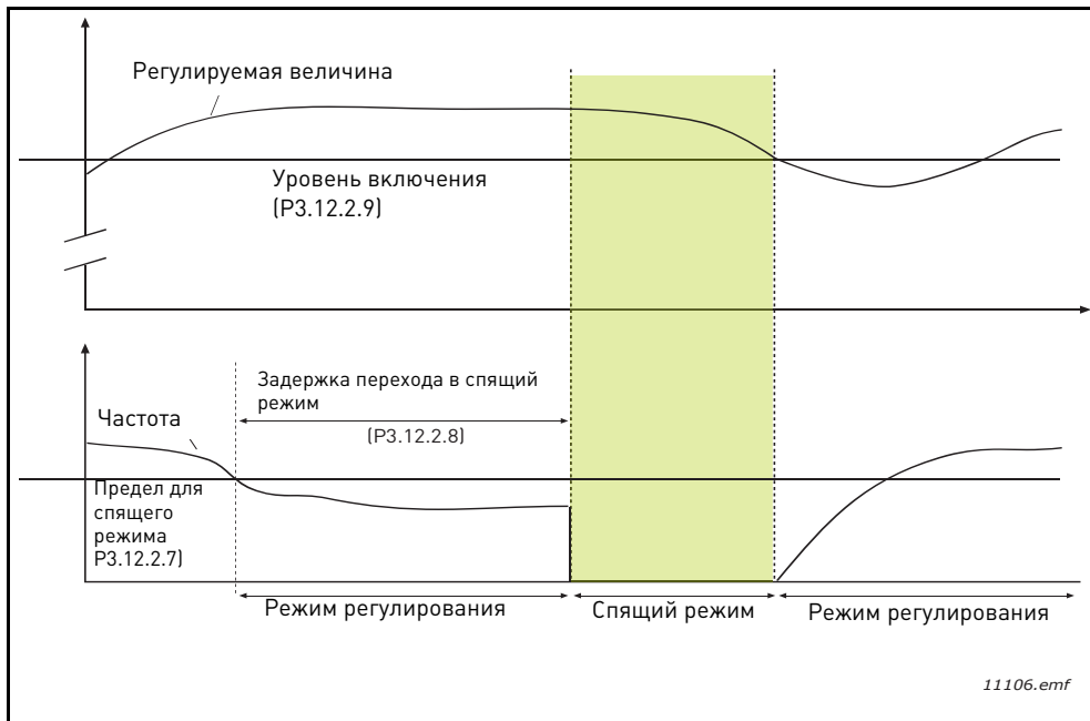
Рис. 34. Предел и задержка для перехода в спящий режим, порог включения
