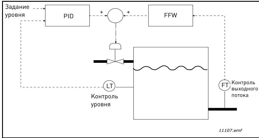
Рис. 35. Регулирование с прямой связью
