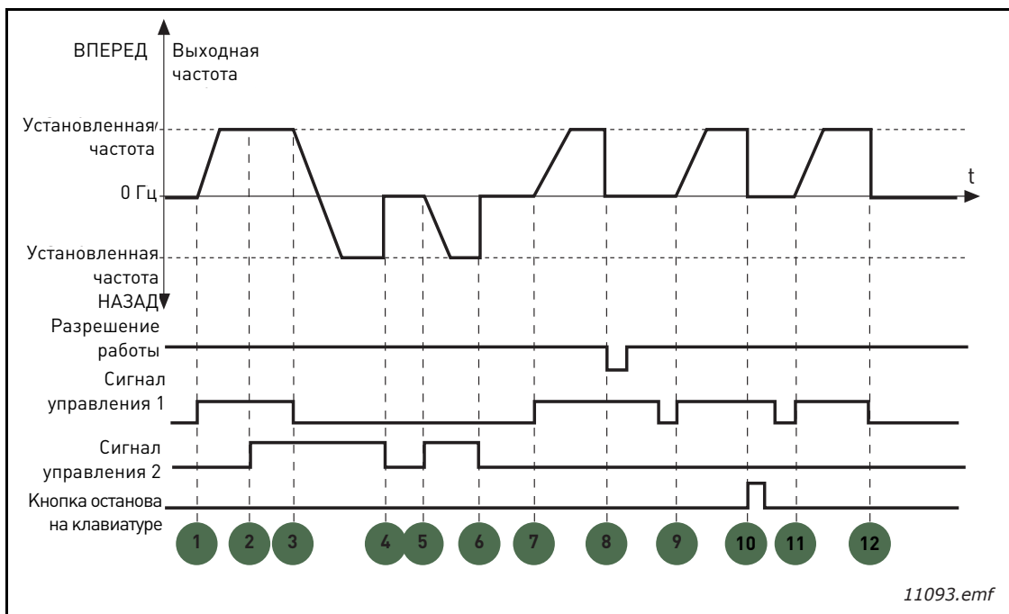
Рис. 21. Логика пуска/останова от платы ввода/вывода A = 2
