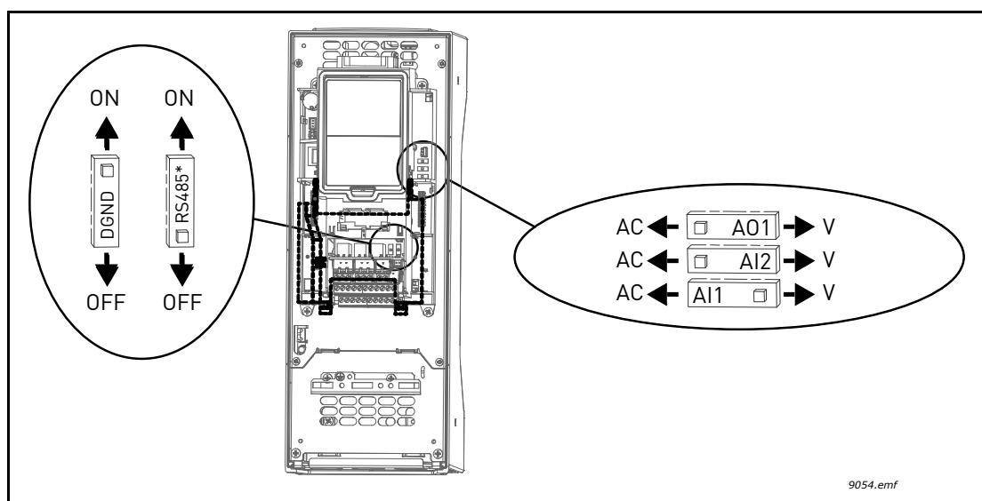
Figure 50. Interrupteurs DIP à leurs positions par défaut, * Résistance de terminaison du bus
