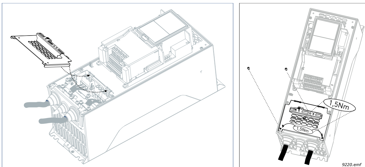
Figure 31. Remontage de l'écran de séparation des câbles
