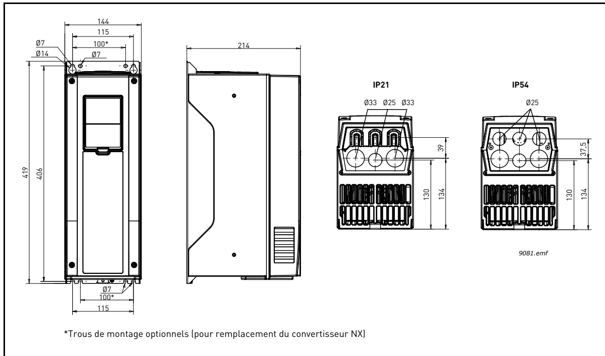
Figure 5. Dimensions du convertisseur de fréquence Vacon, MR5, montage mural
