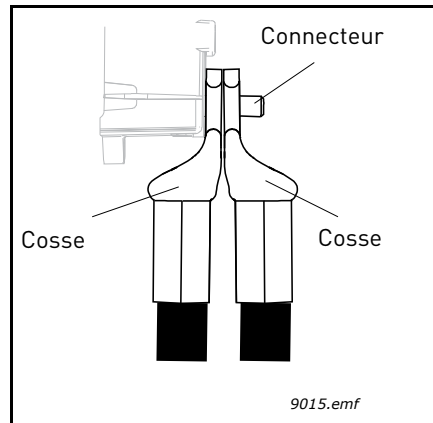
Figure 43. Placement de deux cosses l'une sur l'autre
