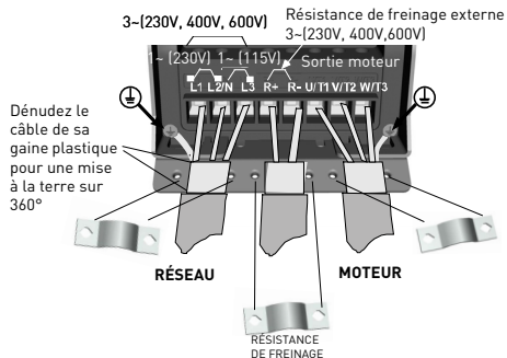
Figure 3.18: Raccordements de puissance Vacon 20, MI2 - MI3
