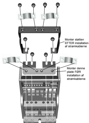
Figur 8: Fastgørelse af PE-pladen og API-kabelstøtten, MI1-MI3
