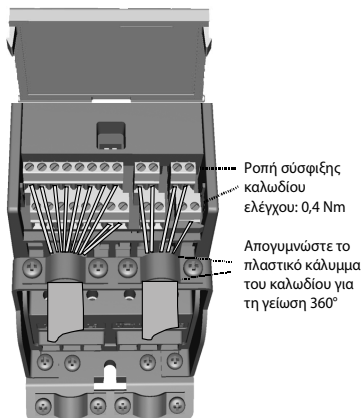
Εικόνα 13: Τοποθετήστε τα καλώδια ελέγχου, MI1 - MI3
