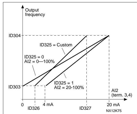
Figure 8-21. 아날로그 입력 AI2 검출
