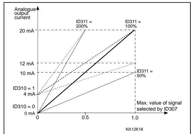
Figure 8-15. 아날로그 출력 검출
