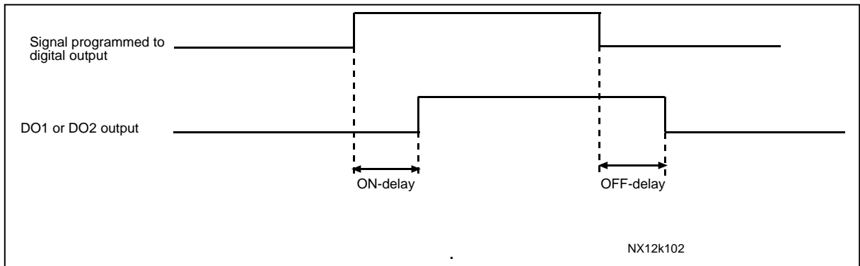
Figure 8-41. 디지털 출력 지연 on/off-설정
