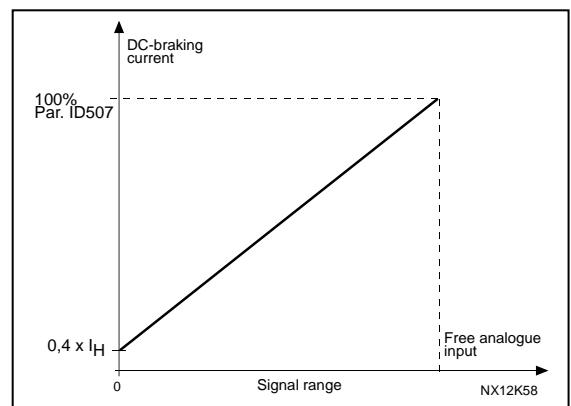
Figure 8-27. 제동 전류의 감소
