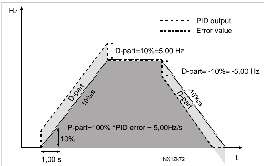
Figure 8-5. 예 3의 값을 가진 PID 출력
