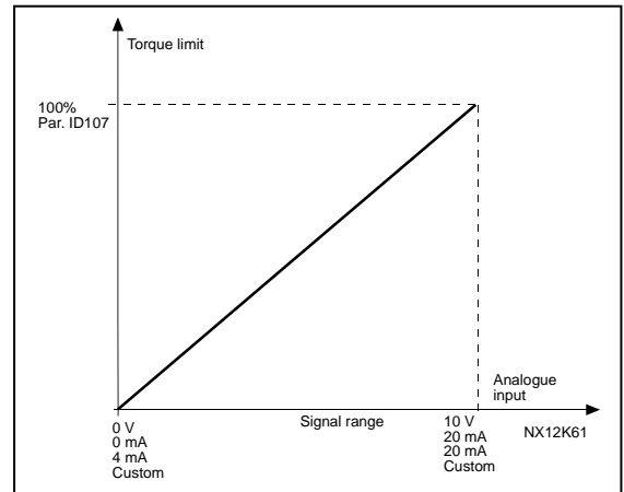
Figure 8-26. 최대 모터 전류의 검출
