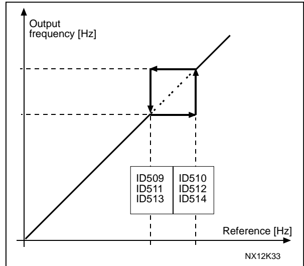
Figure 8-46. 금지 주파수 영역 세팅의 예
