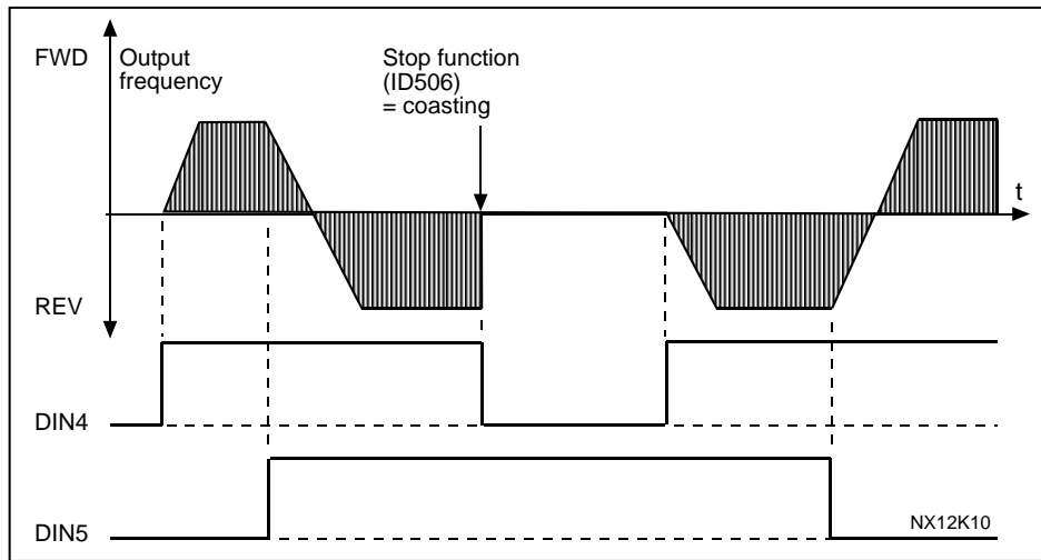
Figure 8-31. 스타트, 정지, 역방향
