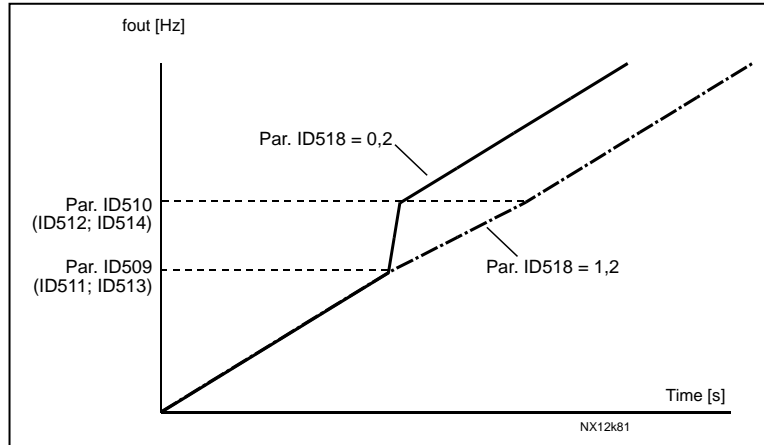
Figure 8-47. 금지주파수간의 램프 속도 검출
