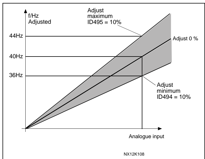
Figure 8-42. 입력 조정의 예
