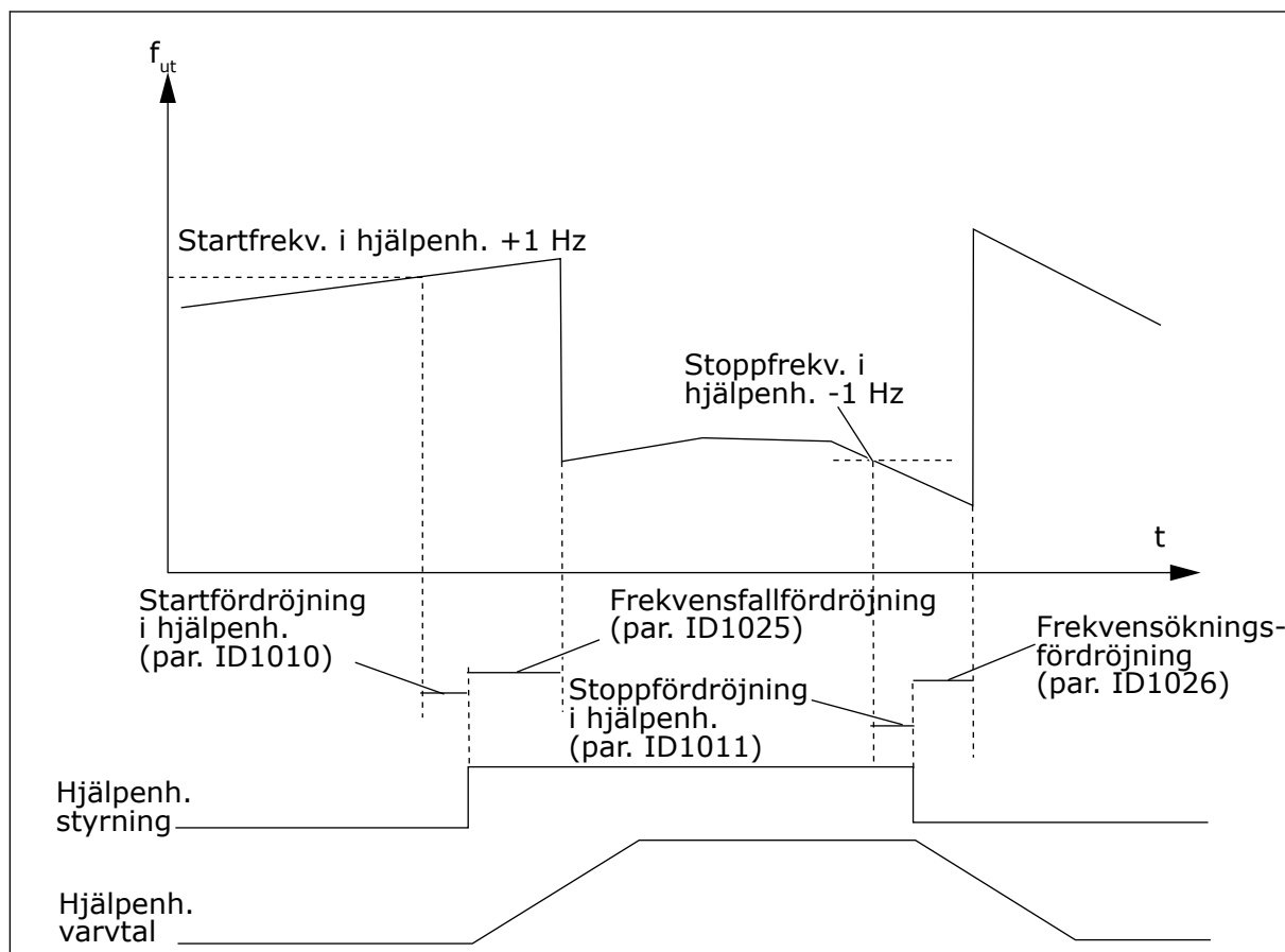
Bild 85: Frekvensfalls- och ökningsfördröjningar
