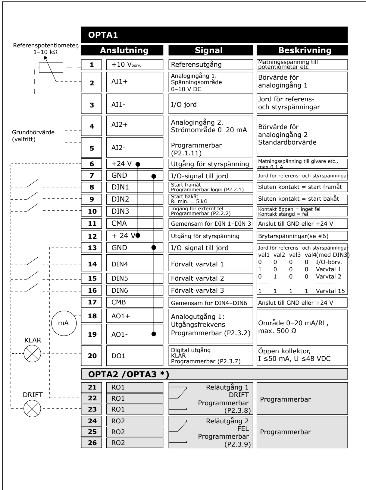
Bild 10: Konstanthastighetsstyrningens I/O-standardkonfiguration
