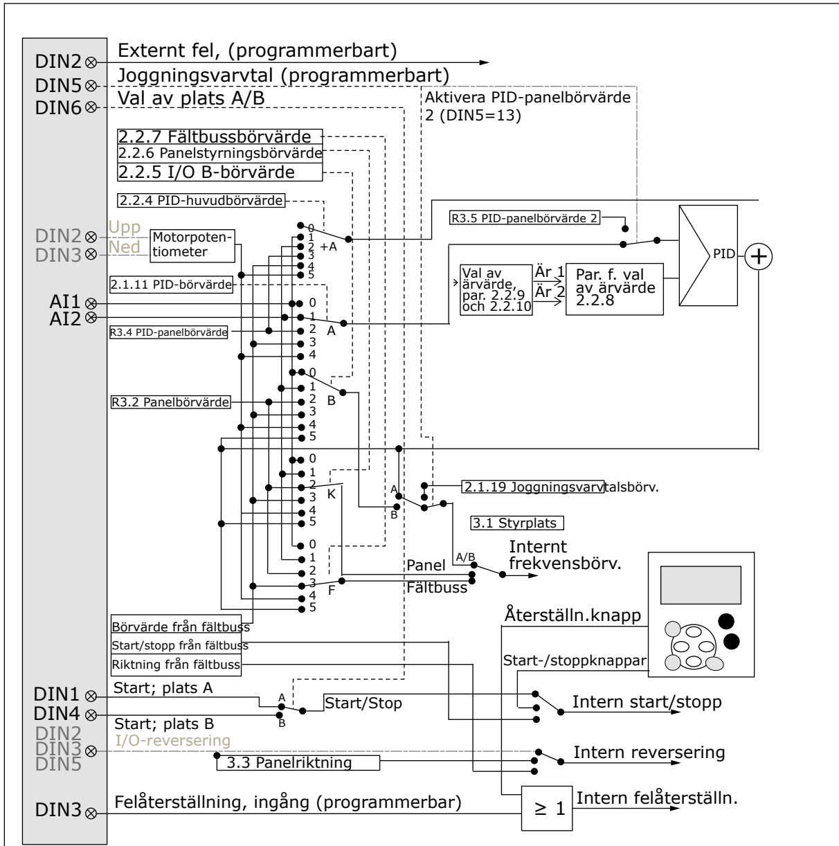
Bild 15: PID-regleringsapplikationens styrsignallogik
