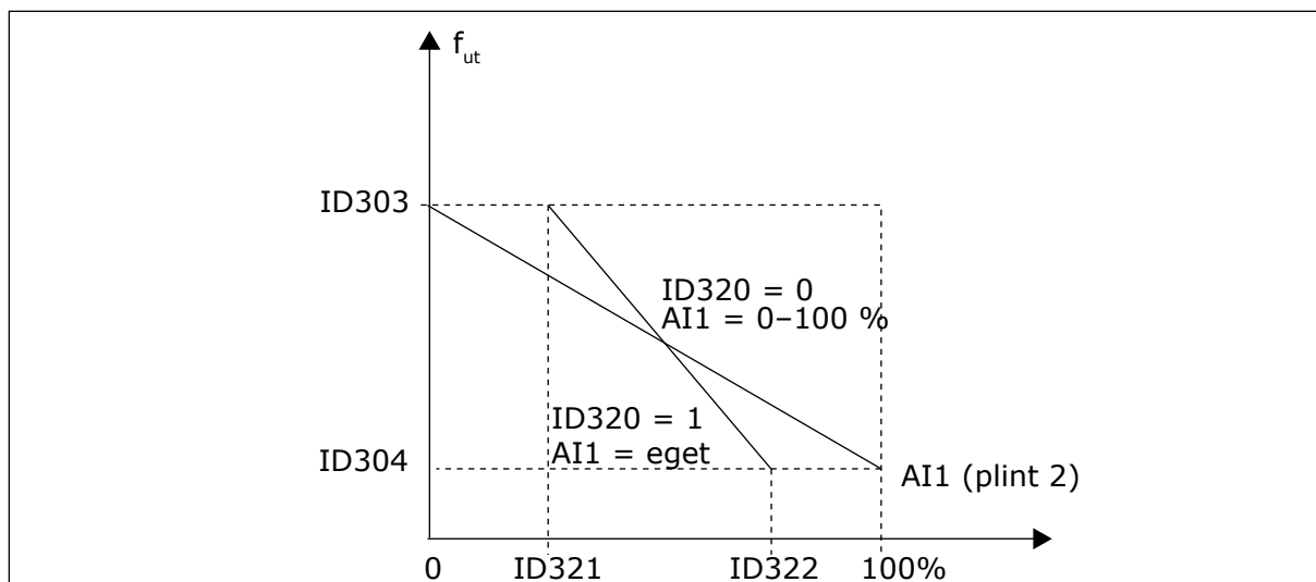
Bild 43: AI1 signalinvert
