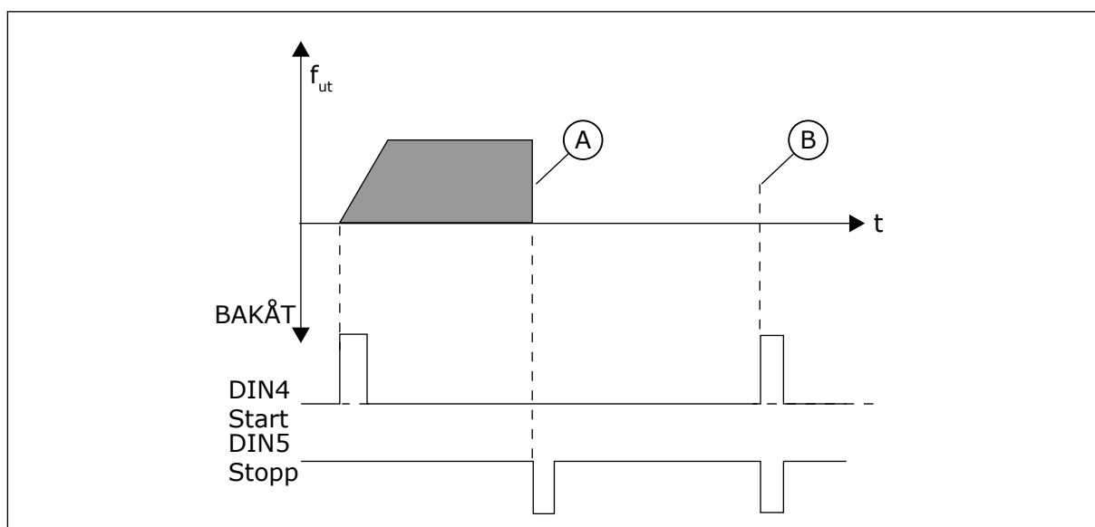
Bild 56: Startpuls/Stoppuls
