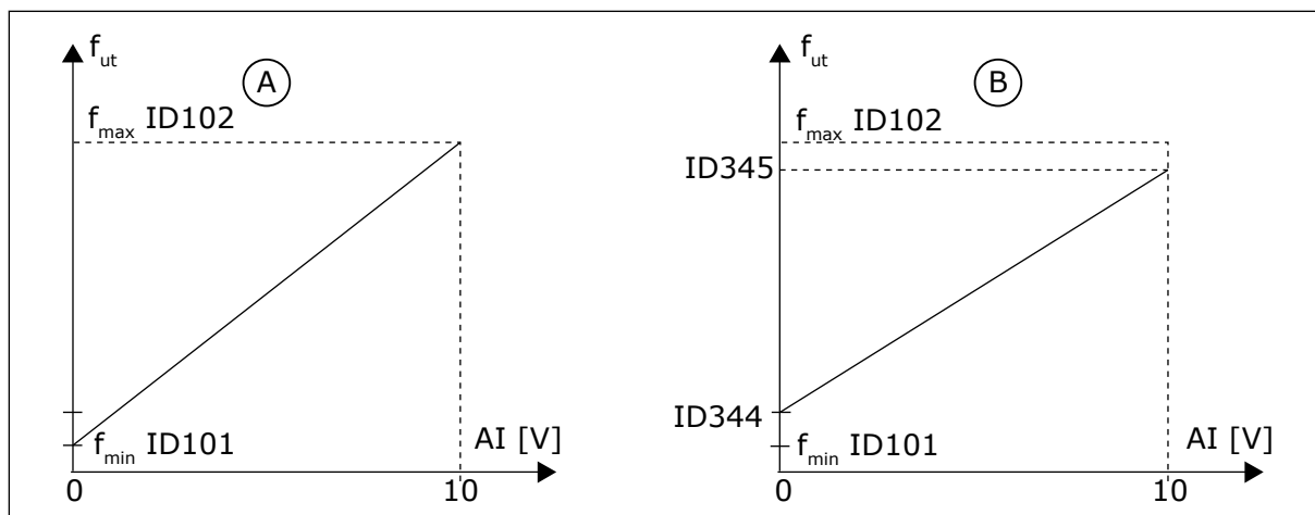
Bild 47: Referensskalning maxvärde
