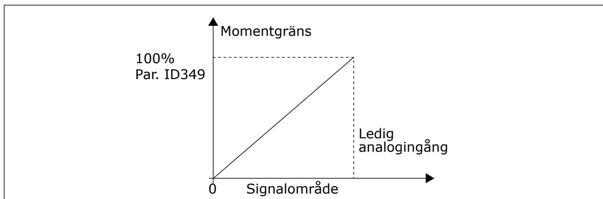
Bild 64: Skalning av motormomentgräns
