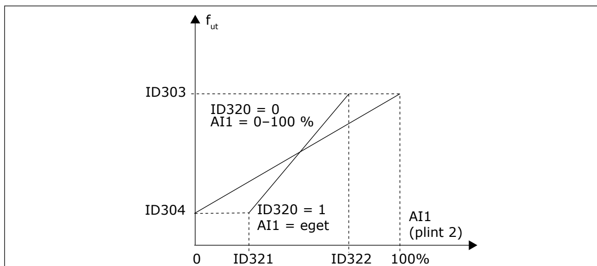
Bild 42: AI1 ingen signalinvertering
