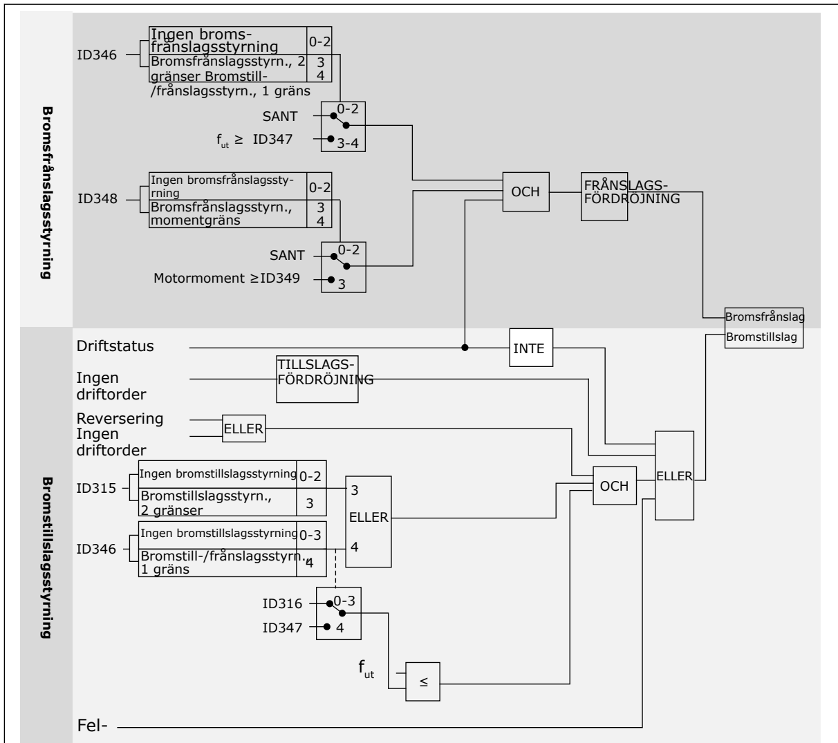
Bild 93: Bromsstyrningslogik
