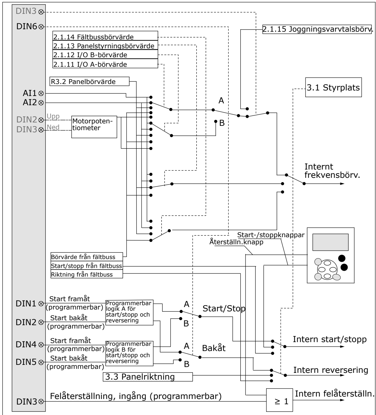
Bild 9: Styrsignallogik i Lokal styrning/fjärrstyrning
