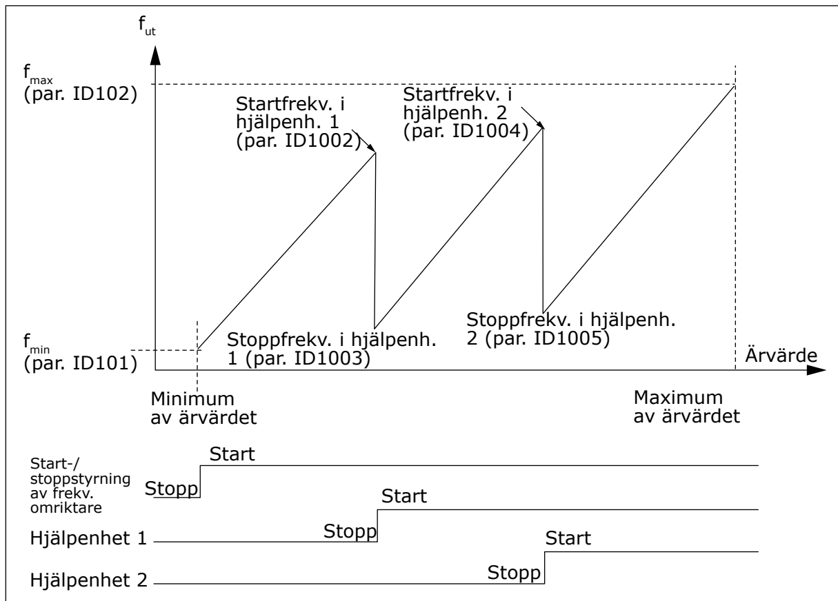
Bild 82: Exempel på omriktare med variabelt varvtal och två hjälpenheter med kringgången PID-regulator
