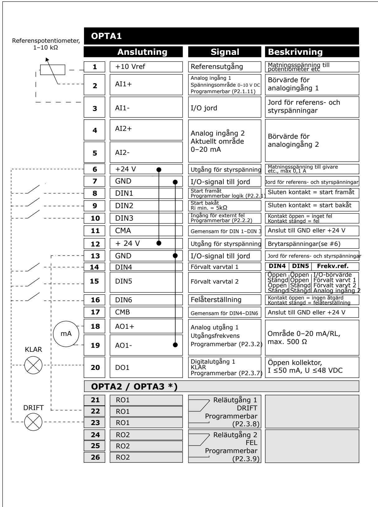
Bild 4: I/O-standardkonfiguration för standardapplikation
