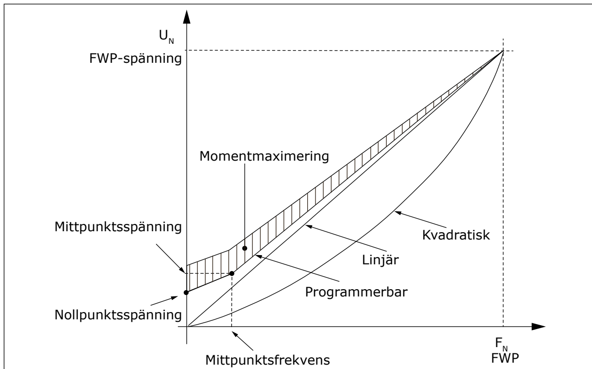
Bild 26: U/f-optimering
