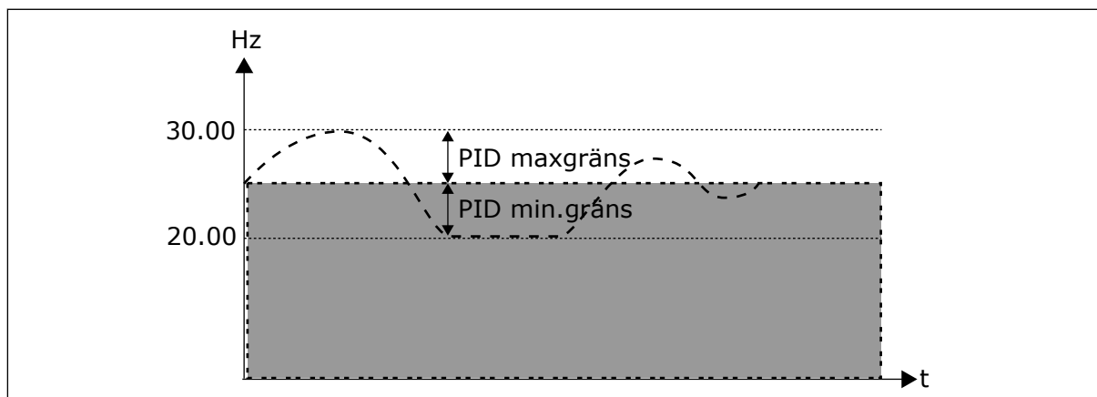
Bild 57: PID-summebörvärde
