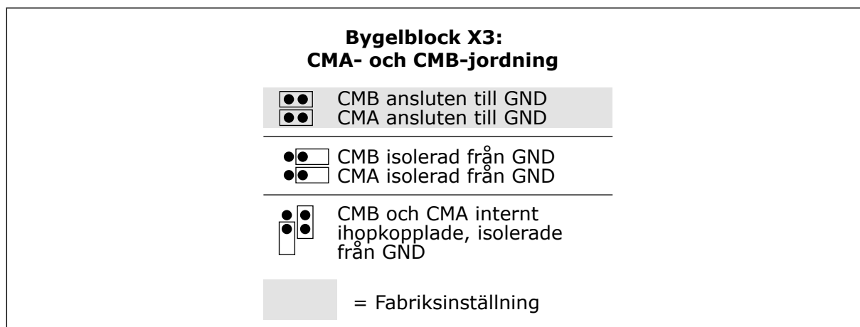
Bild 8: Bygellägen
