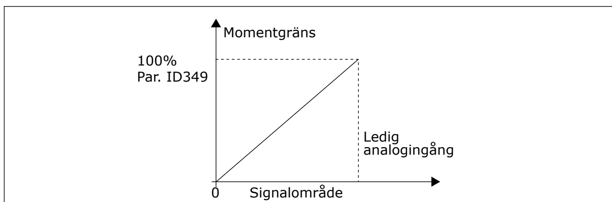
Bild 63: Minska momentövervakningsgränsen
