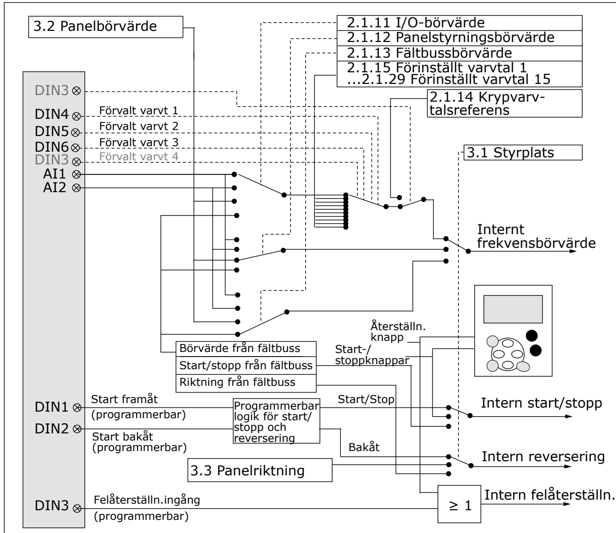
Bild 12: Konstanthastighetsapplikationens styrsignallogik
