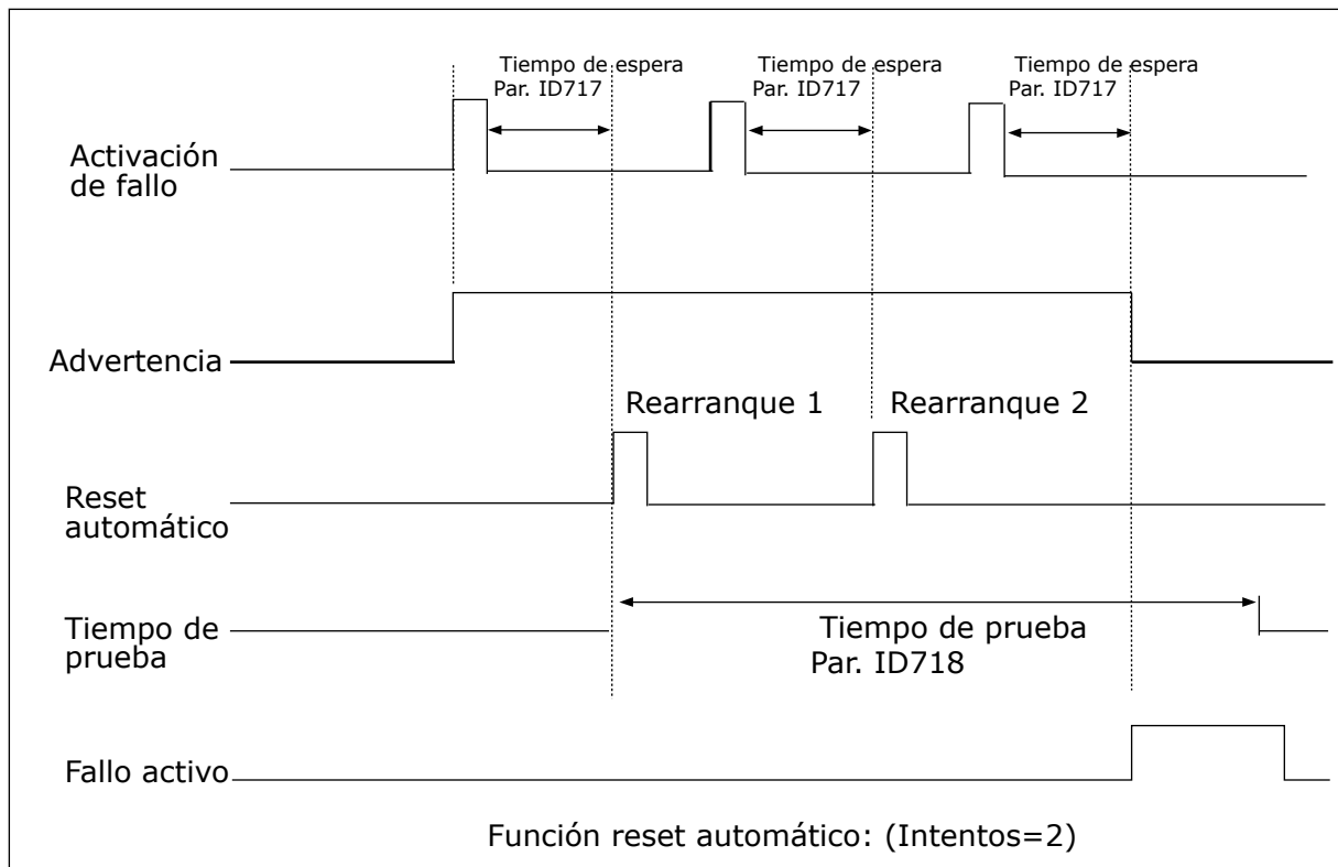
Imag. 78: Ejemplo de re arranques automáticos con dos re arranques
