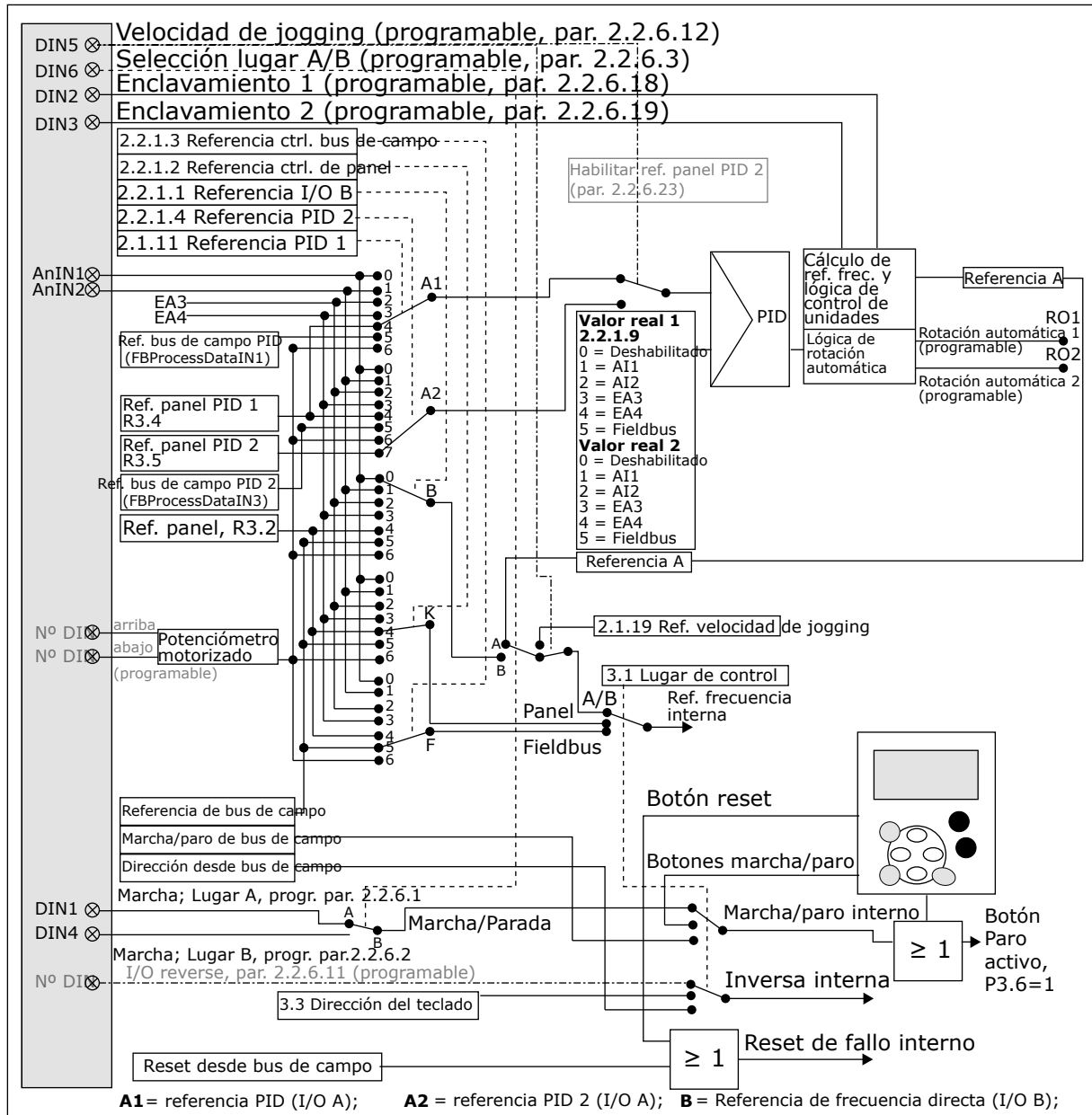
Imag. 23: Lógica de señales de control de la Aplicación de control de bombas y ventiladores
