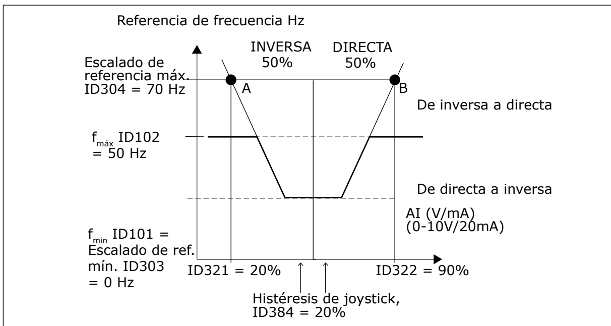
Imag. 60: Histéresis de Joystick con frecuencia mínima en 35 Hz
