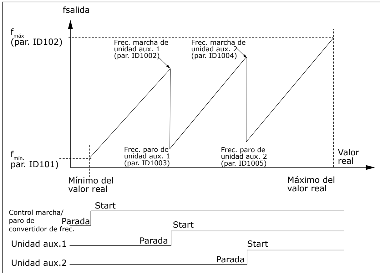
Imag. 82: Ejemplo de unidad de velocidad variable y dos unidades auxiliares con controlador PID derivado
