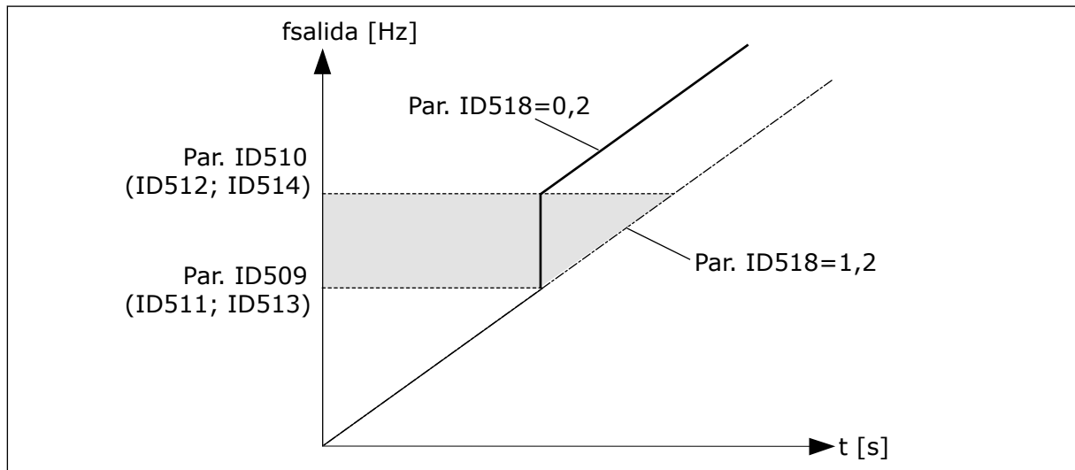
Imag. 71: Escalado de velocidad de rampa entre frecuencias prohibidas
