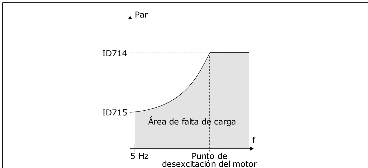
Imag. 76: Ajuste de la carga mínima
