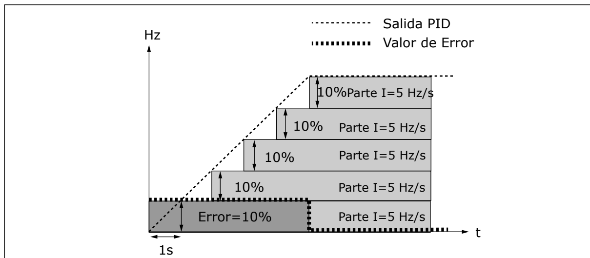
Imag. 27: Función del controlador PID como controlador I
