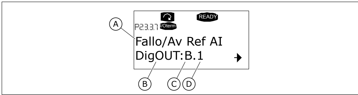
Imag. 94: Definición de una entrada/salida para una función determinada en el panel
