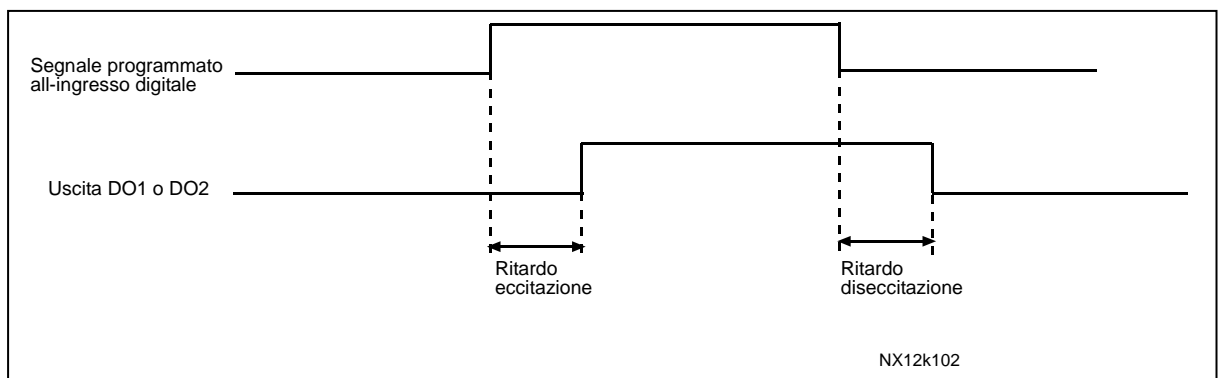
Figura 8-41. Uscite digitali 1 e 2, ritardi di eccitazione e diseccitazione
