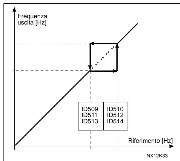
Figura 8-46. Impostazione area di frequenza proibita.
