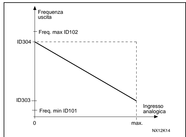
Figura 8-11. Inversione riferimento
