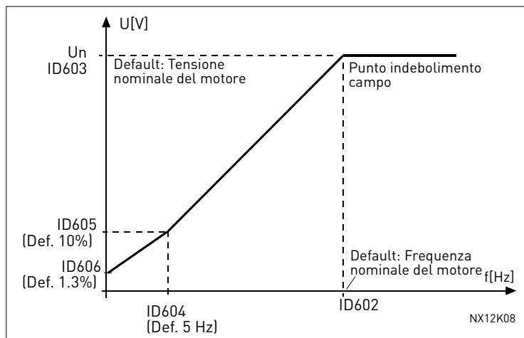
Figura 8-2. Curva V/f programmabile
