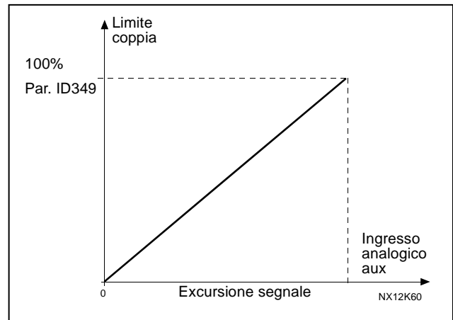
Figura 8-39. Riduzione del limite di supervisione della coppia
