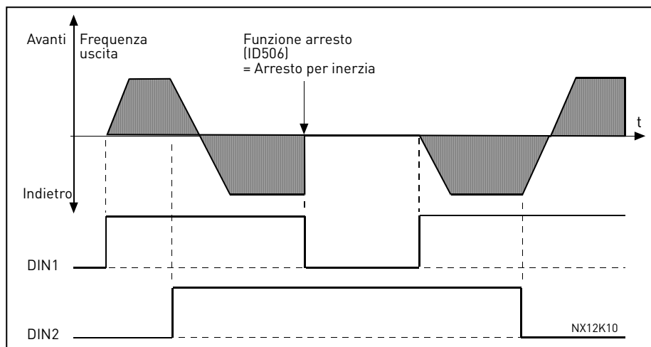
Figura 8-7. Marcia, Arresto, Inversione
