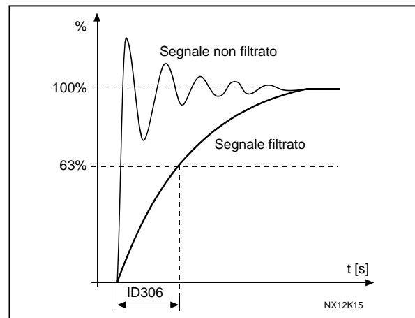
Figura 8-12. Filtraggio di riferimento
