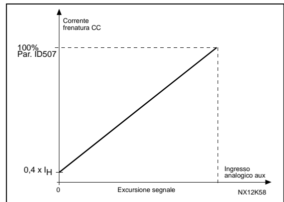
Figura 8-27. Riduzione corrente di frenatura in CC
