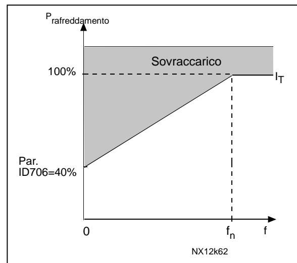
Figura 8-48. Curva corrente termica motore I_T
