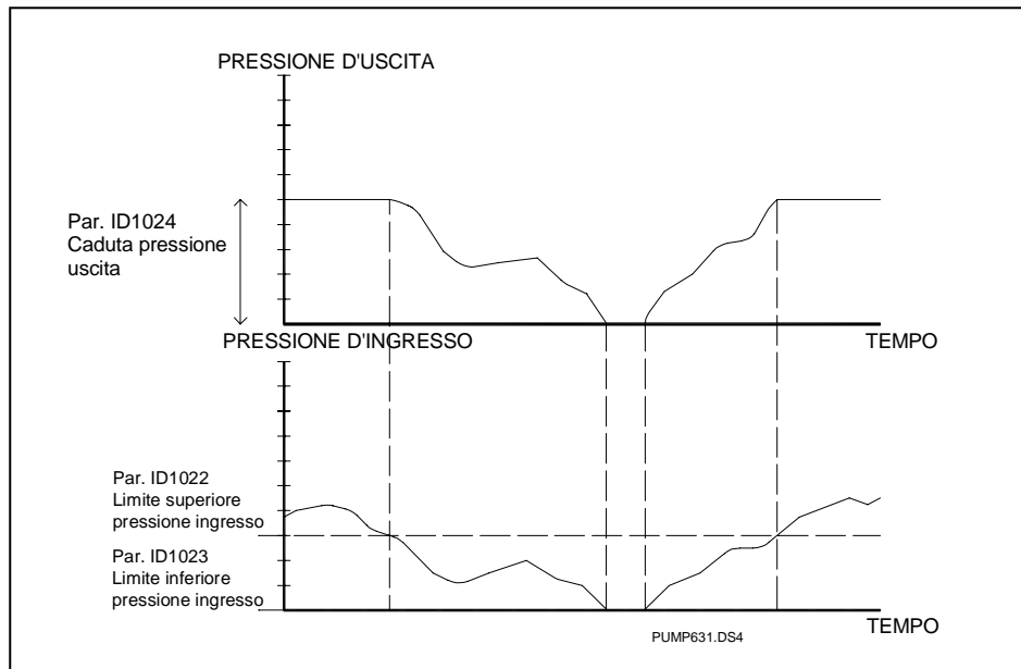
Figura 8-61. Comportamento della pressione d'uscita in base alla pressione d'ingresso e alle impostazioni dei parametri
