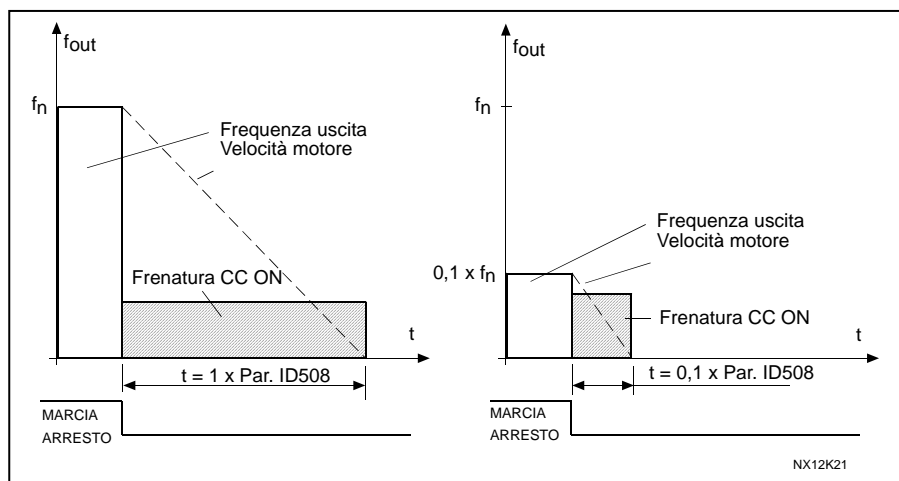
Figura 8-44. Tempo di frenatura in CC nella funzione Arresto = Arresto per inerzia.
