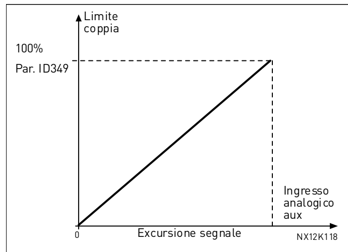
Figura 8-40. Scalatura del limite di coppia motorizzante
