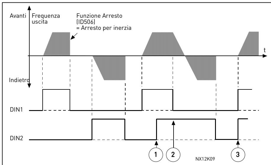
Figura 8-6. Marcia avanti/Marcia indietro
