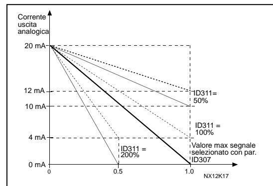
Figura 8-14. Inversione uscita analogica
