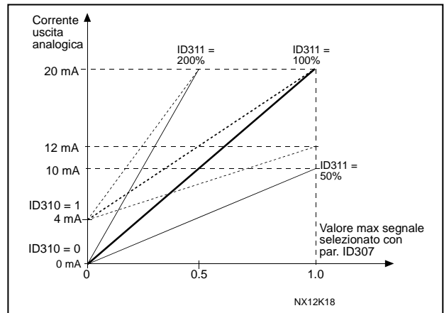
Figura 8-15. Scalatura uscita analogica
