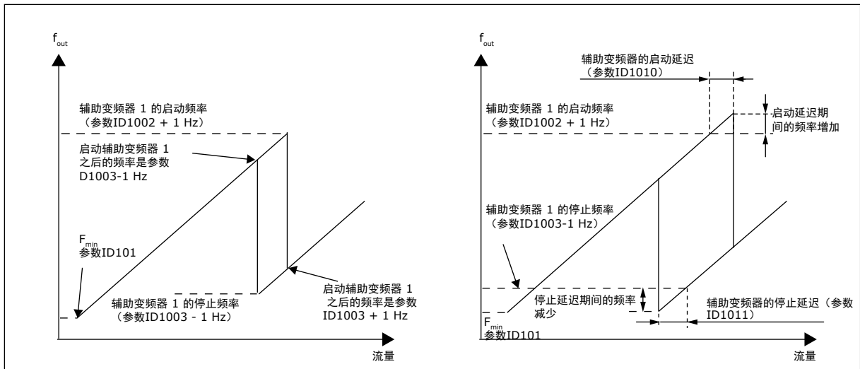
图 79: 参数设置示例；可变速速度变频器和一个辅助变频器
