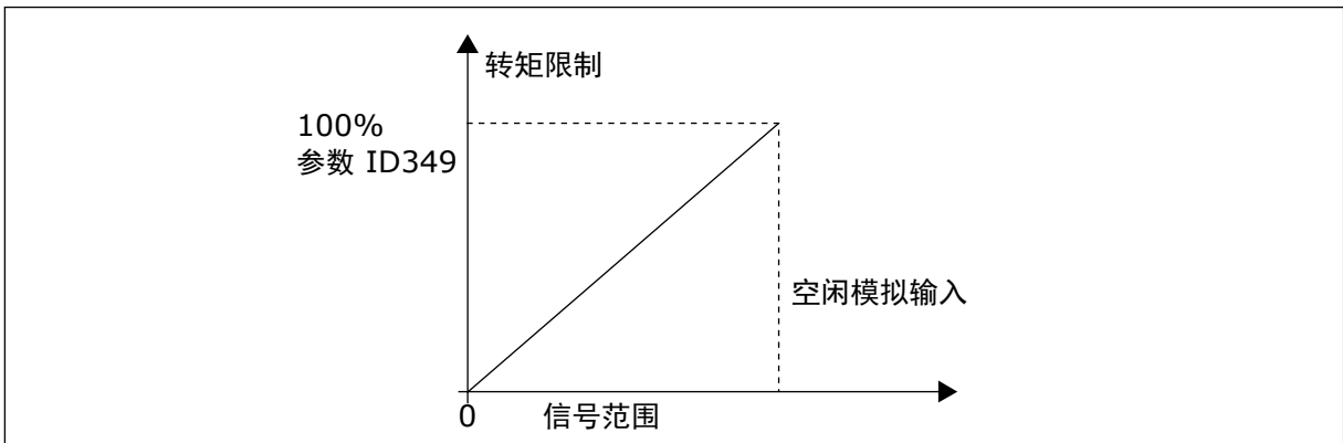
图 53: 降低转矩监控限制
