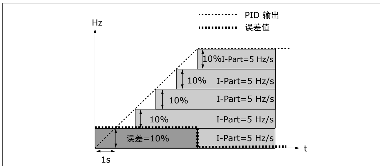
图 27: PID 控制器用作 I 控制器
