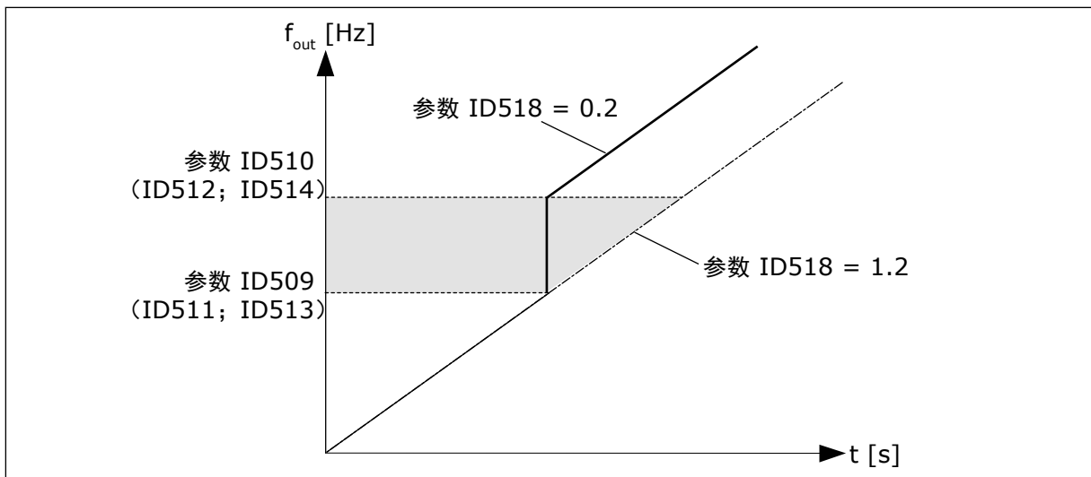
图 71: 禁止频率之间的斜坡速度缩放
