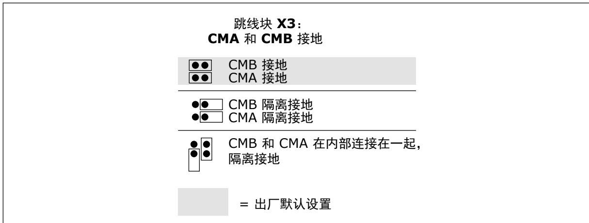
图 11: 跳线选择
