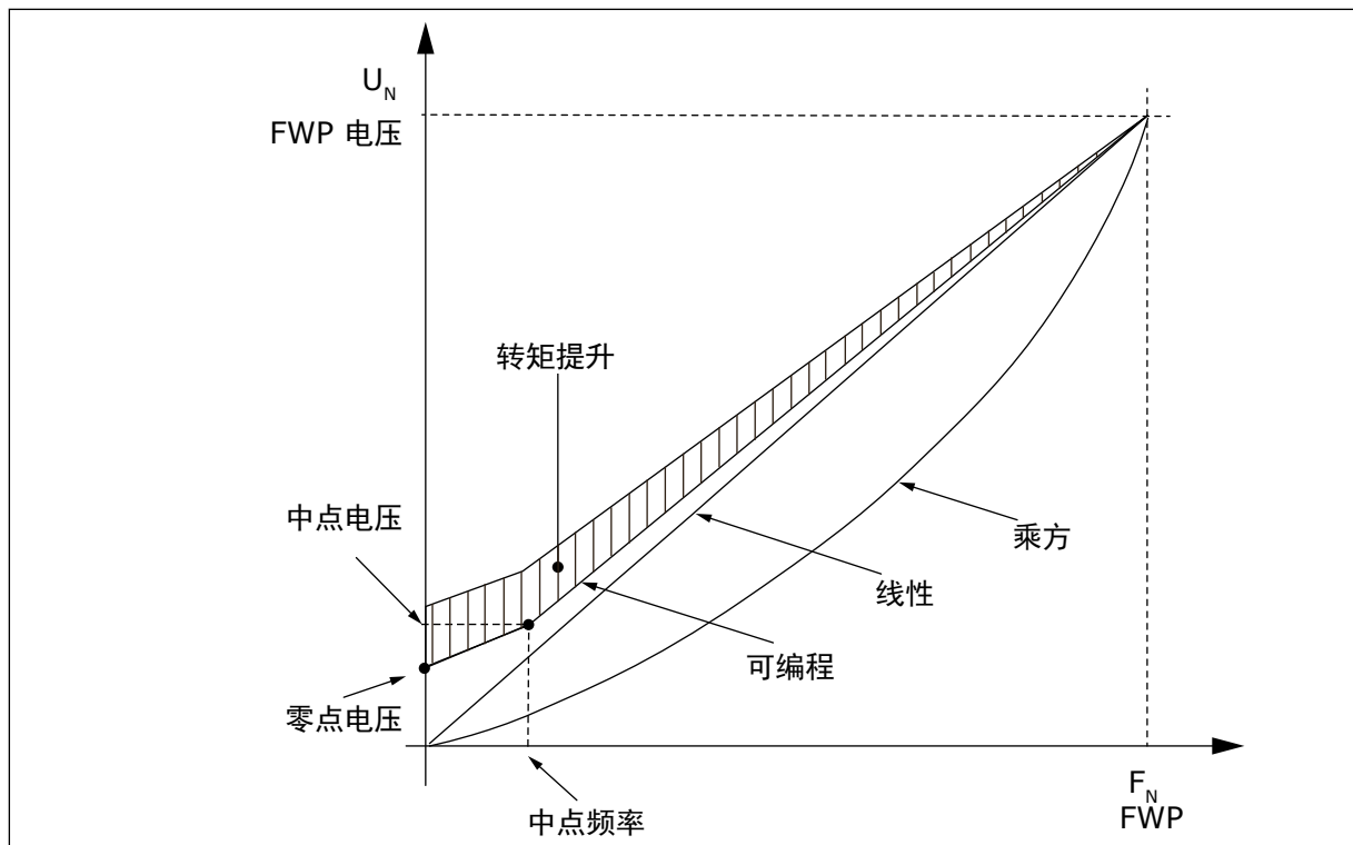
图 26: U/f 优化
