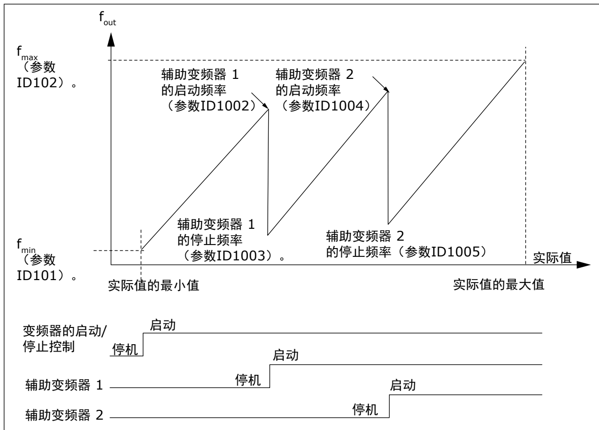
图 82: 可变速变频器 and 两个辅助变频器 (带旁路 PID 控制器) 示例
