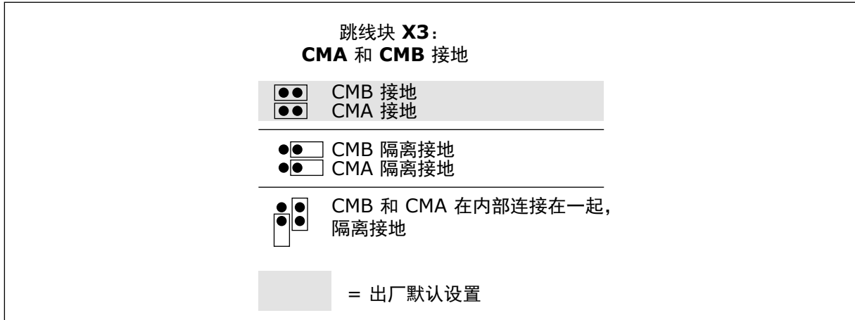
图 20: 跳线选择
