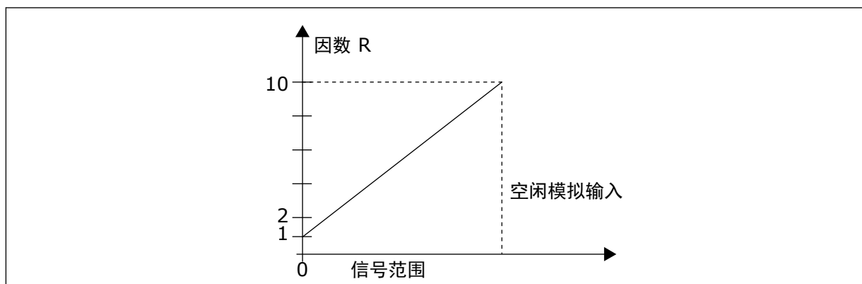
图 62: 减少加速和减速时间
