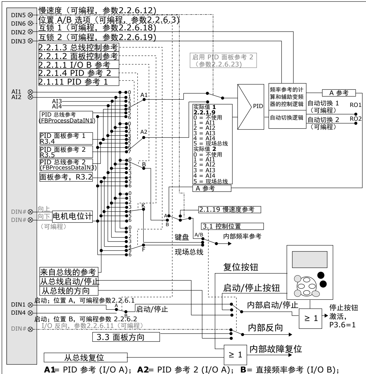
图 23: 泵和风机控制应用程序的控制信号逻辑
