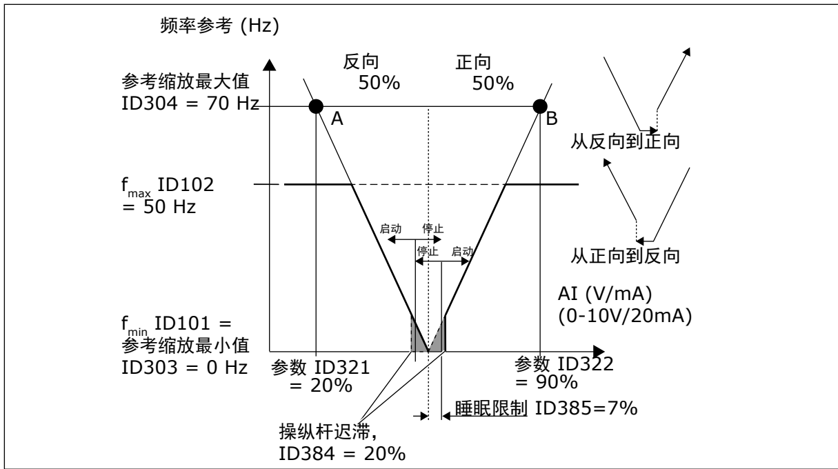
图 59: 睡眠限制功能示例
