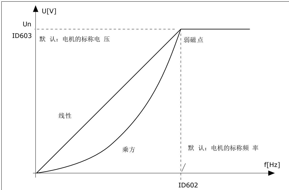
图 24: 电机电压的线性和乘方变化
