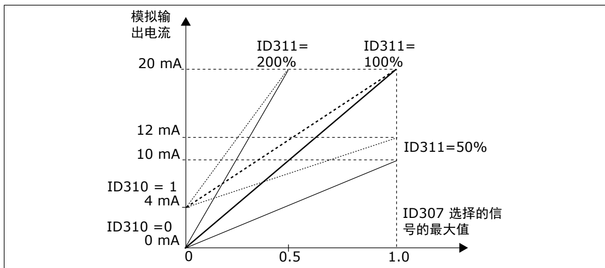
图 39: 模拟输出缩放
