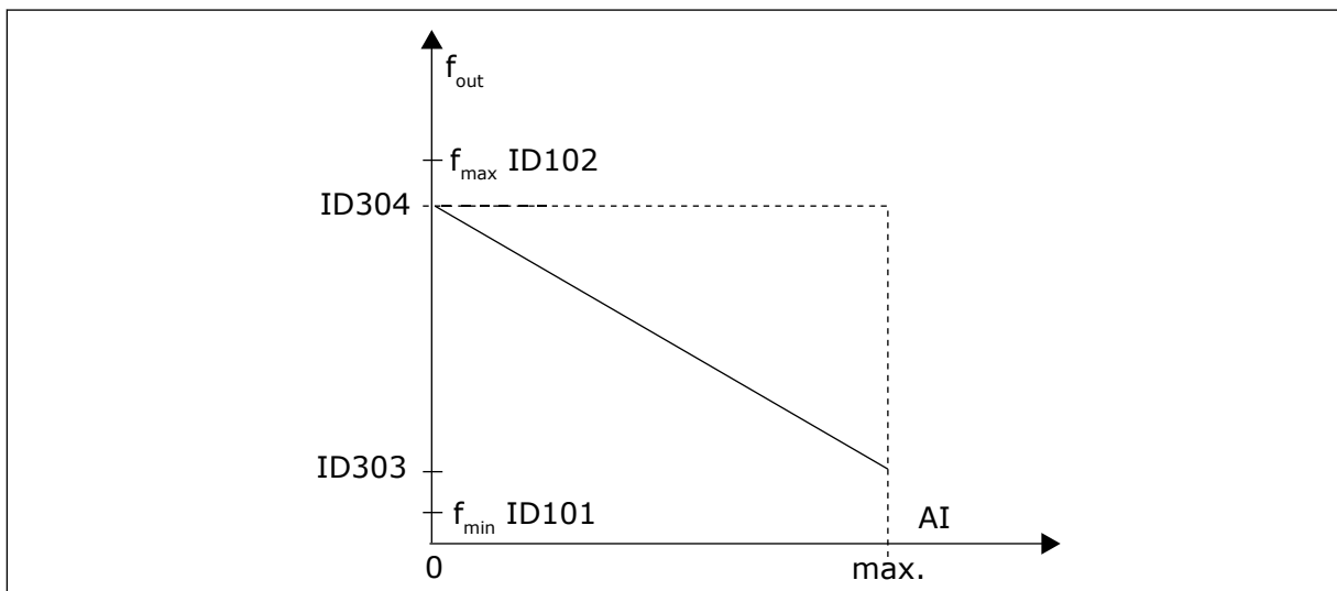
图 35: 参考倒置
