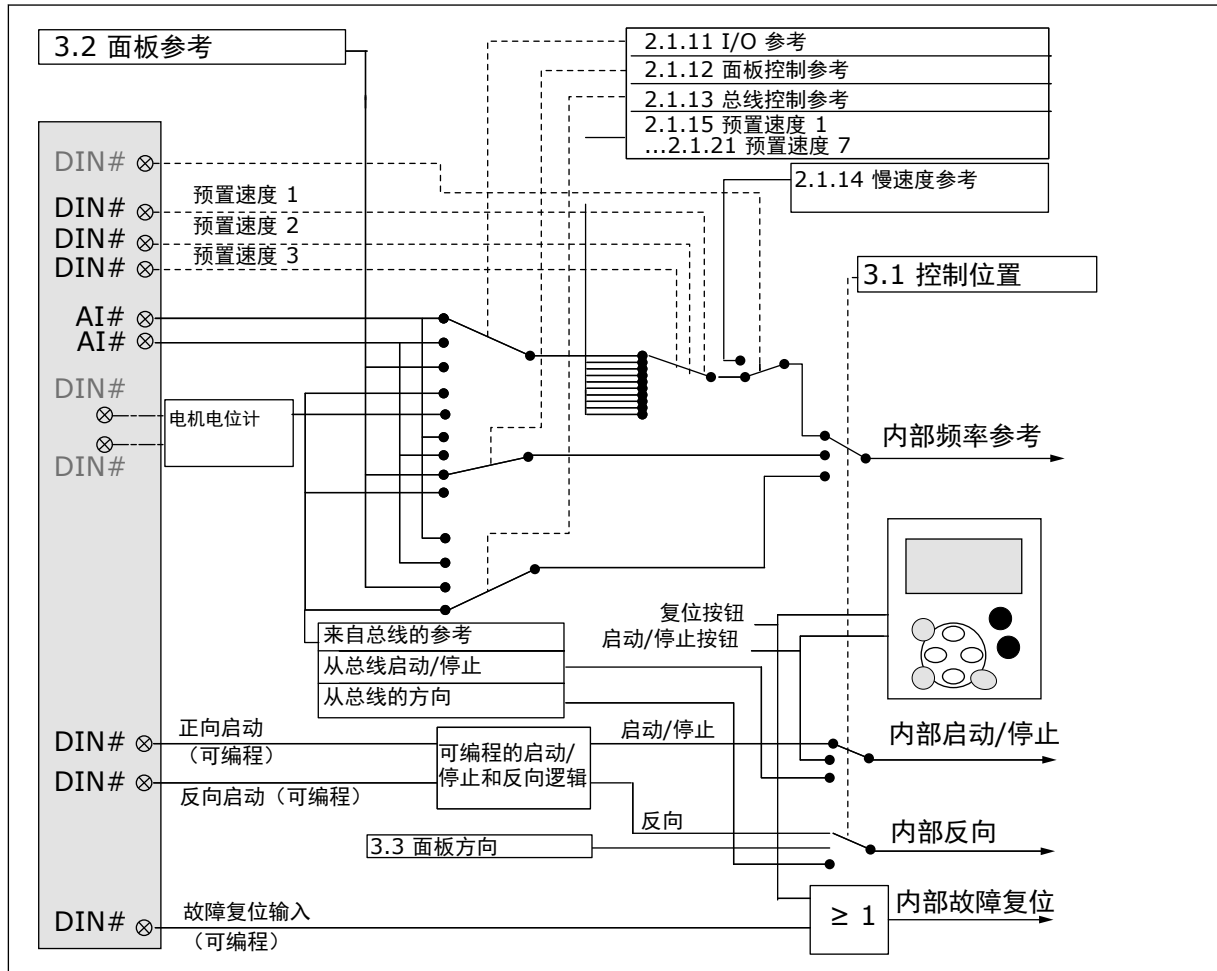
图 18: 多用途控制应用程序的控制信号逻辑
