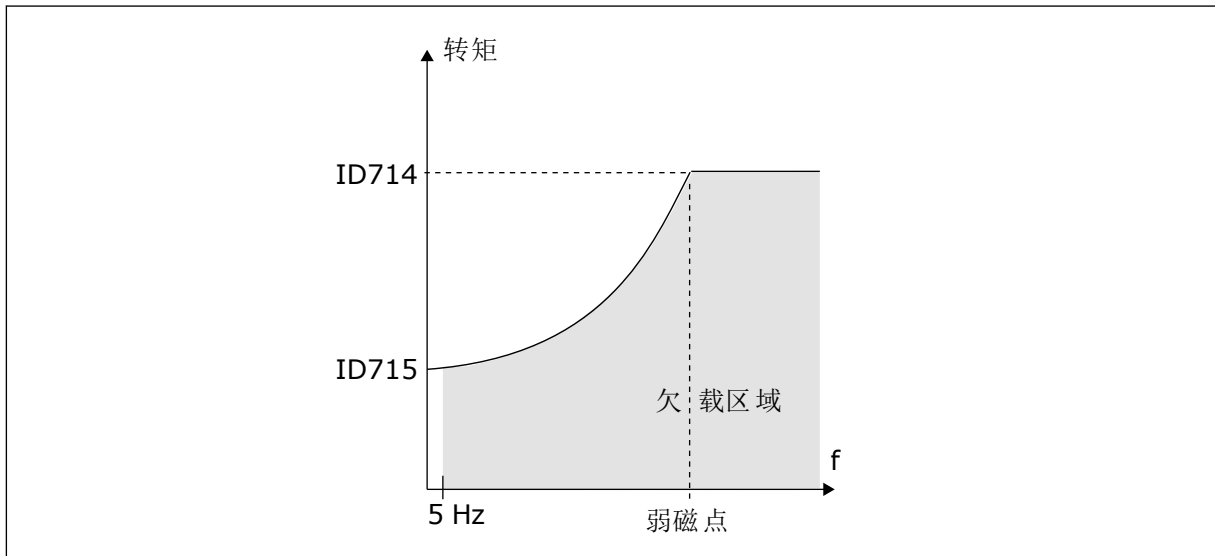
图 76: 设置最小负载
