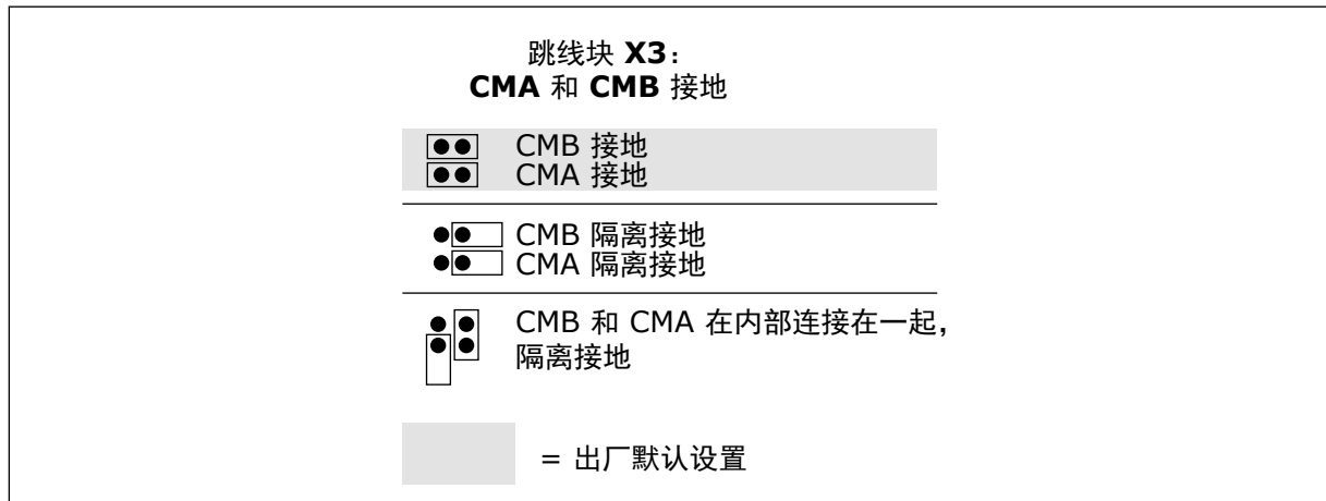
图 5: 跳线选择
