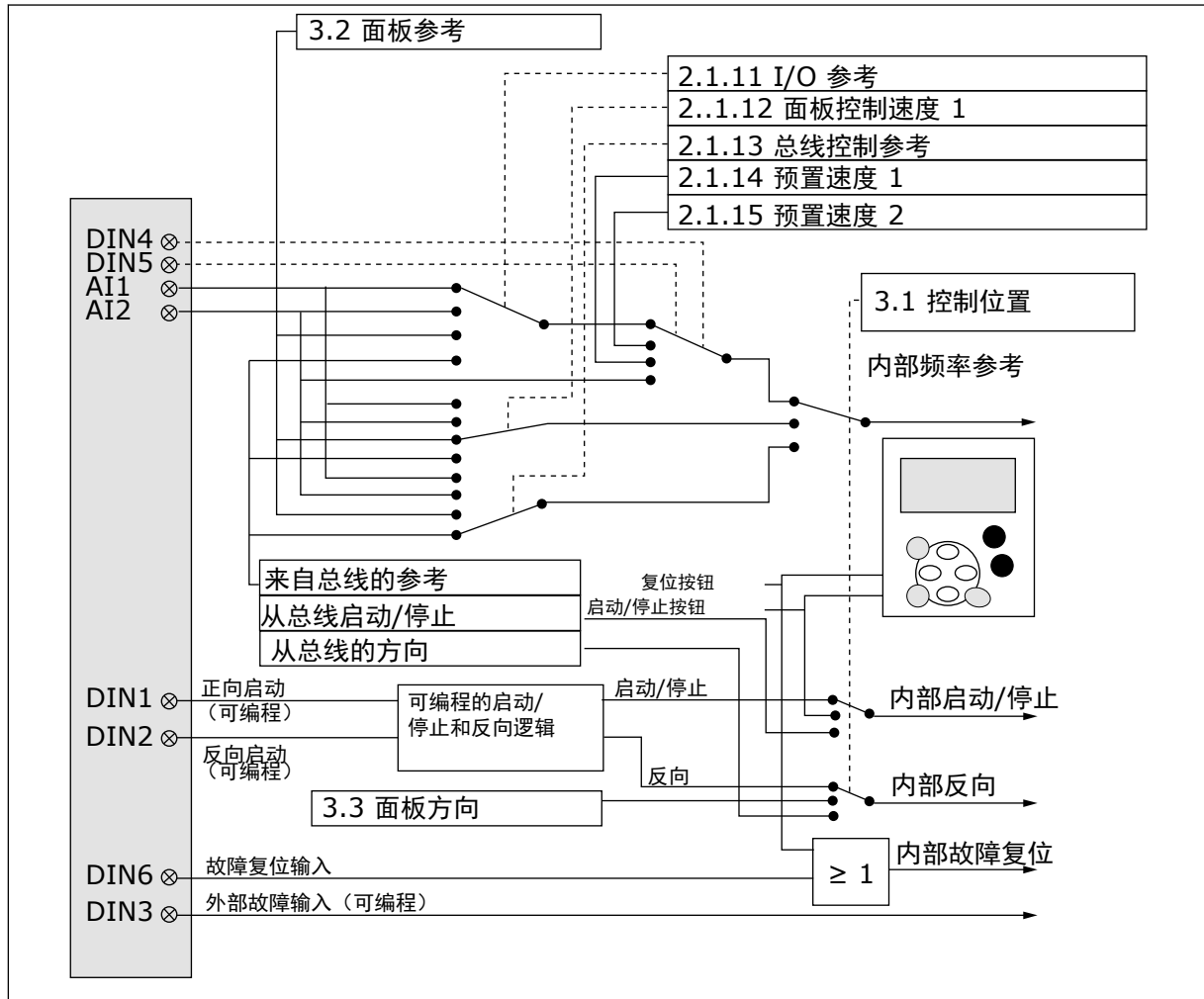
图 6: 标准应用程序的控制信号逻辑
