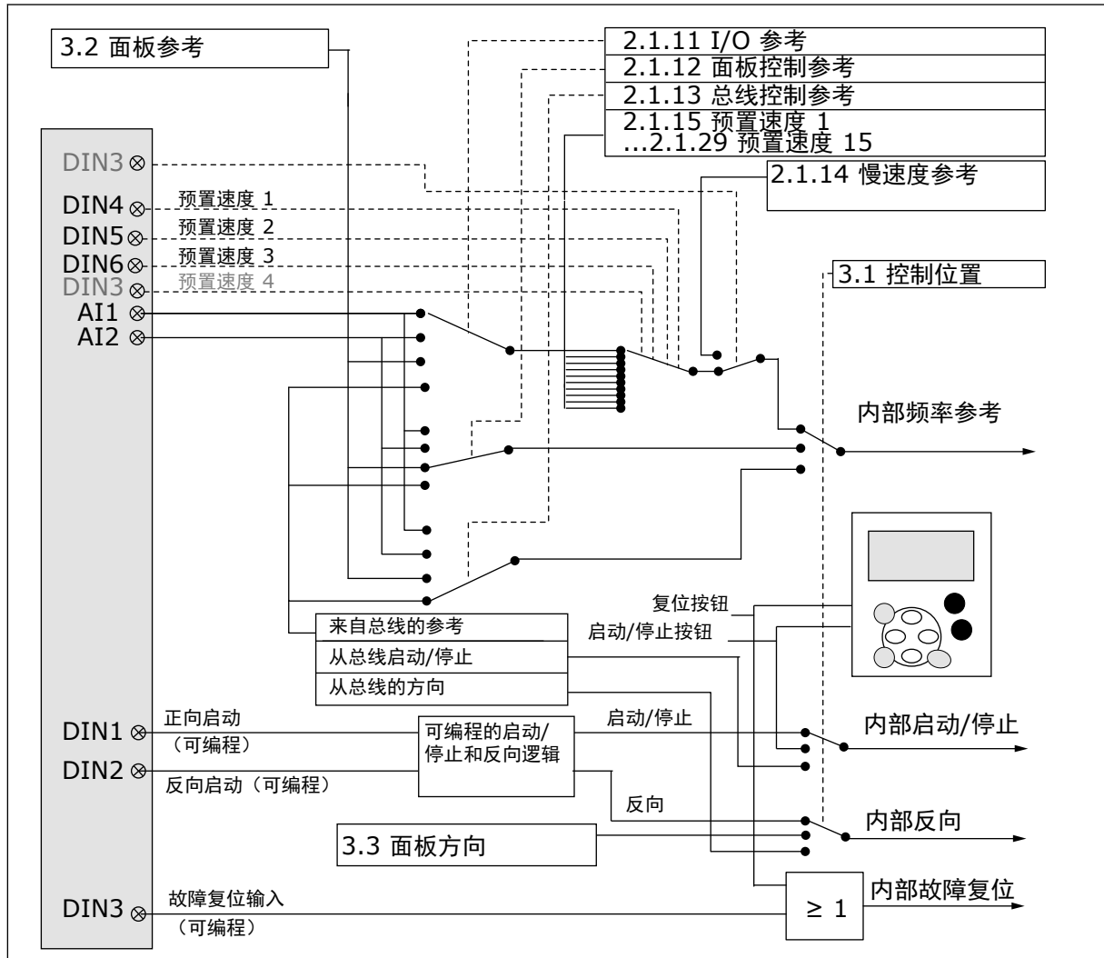
图 12: 多级速度应用程序的控制信号逻辑
