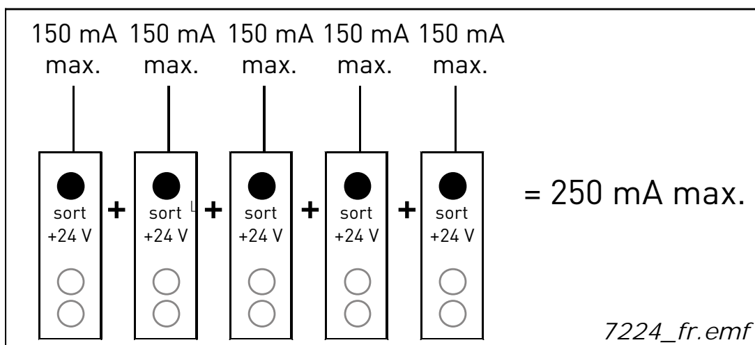
Figure 3. Charges maximales sur la sortie +24 V/EXT+24 V
