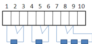
Configuration à deux fils
