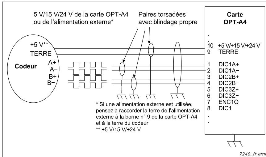
Figure 13. Raccordement d'un codeur de type RS-422 à l'aide d'entrées différentielles
