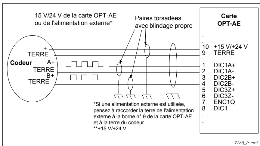
Figure 20. Raccordement d'un codeur de type HTL (source ouverte) à l'aide d'entrées unipolaires
