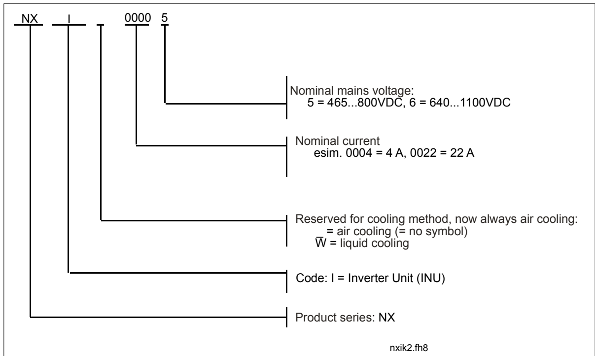
图 3-1 Vacon NX 型号标识码，FR4—FR8
