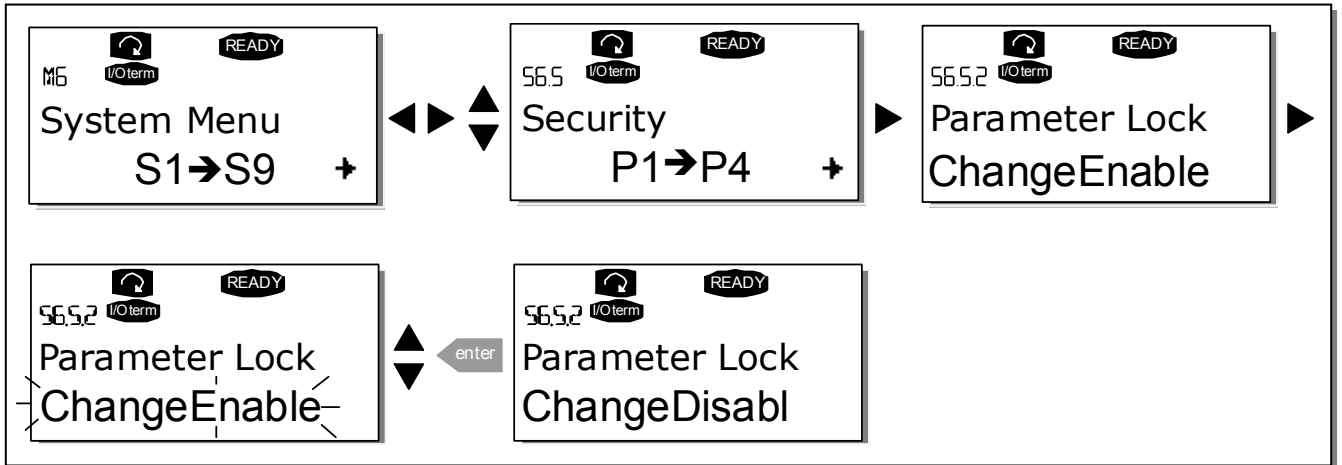
图 7-11， 参数锁定
