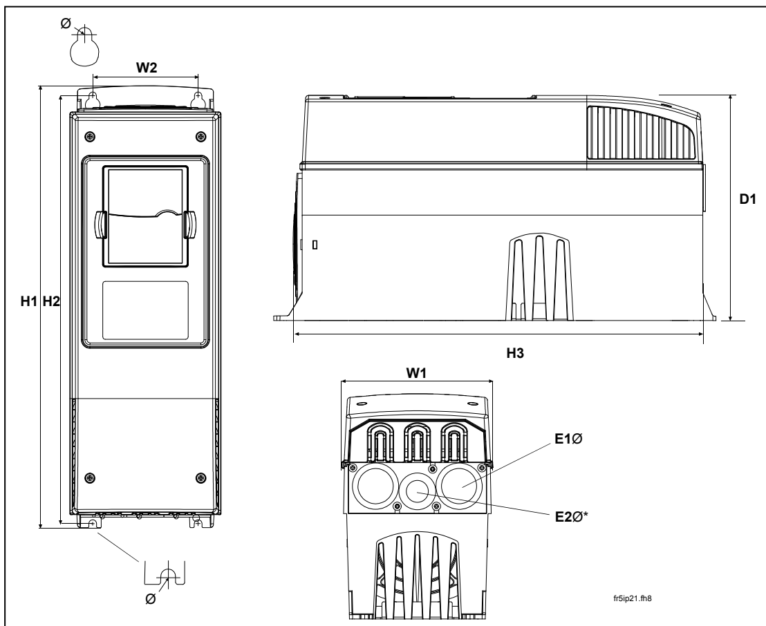
图 5-1, Vacon NX 尺寸
