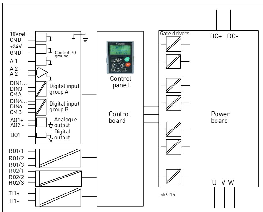
图 6-12，电隔离
