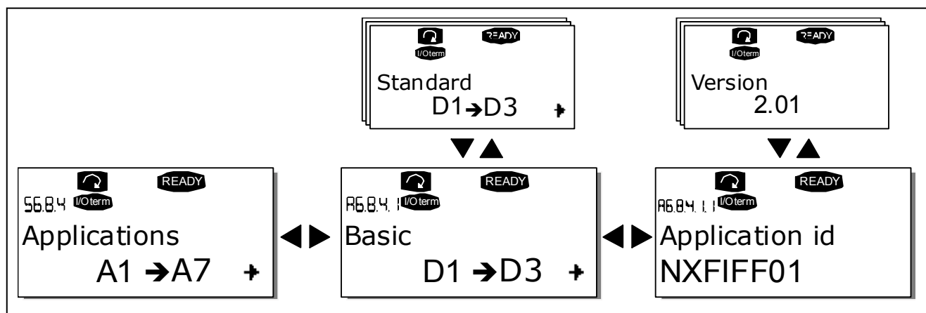
图 7-21, 应用宏信息子菜单
