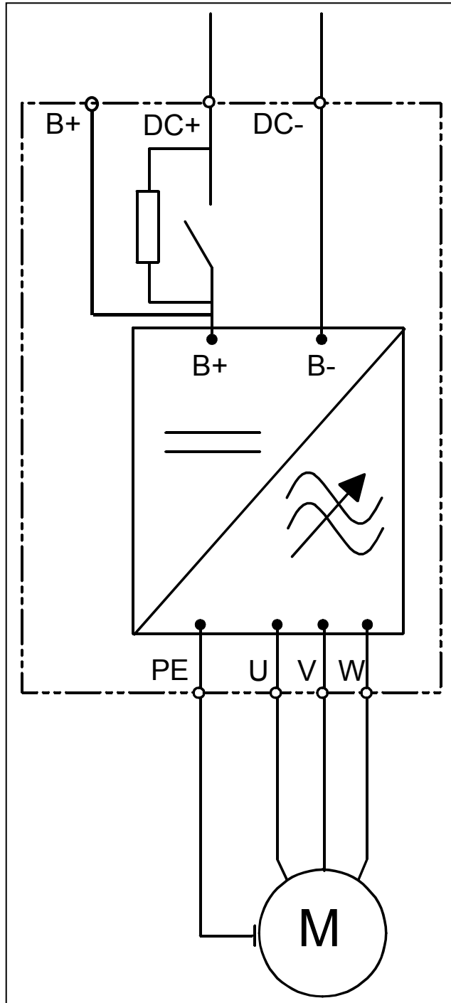
图 6-1, 基本接线图
