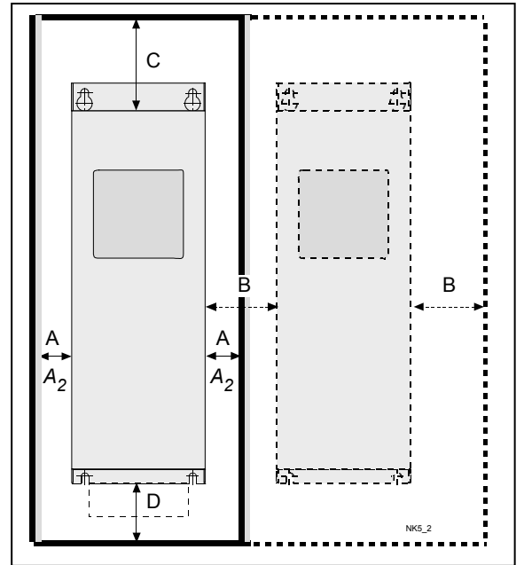
图 5-6, 安装空间
