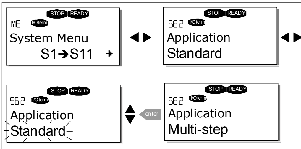
图 7-6，应用宏的变更
