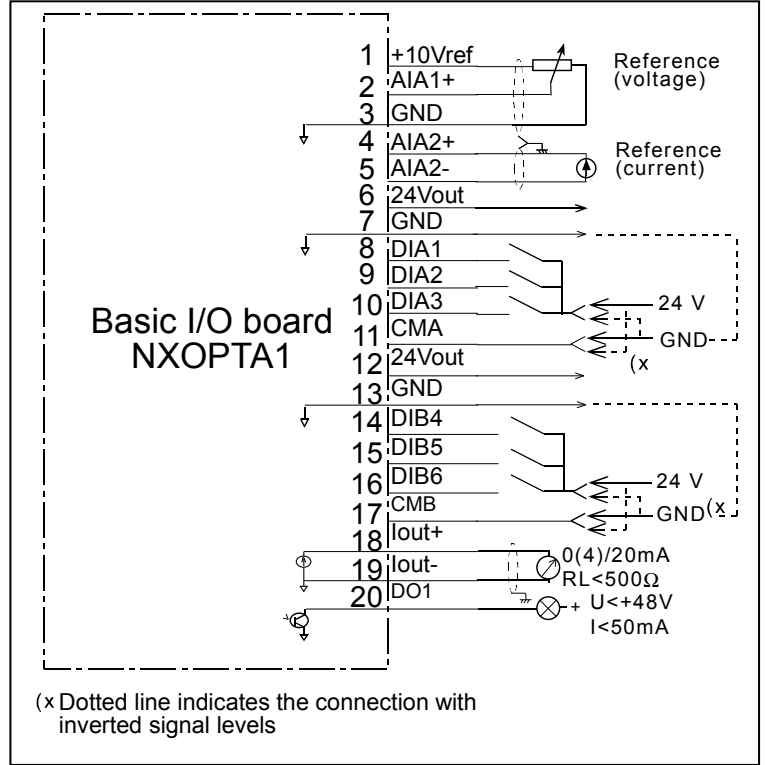
图 6-10, 基本 I/O 板(NXOPTA1)的常规连线
