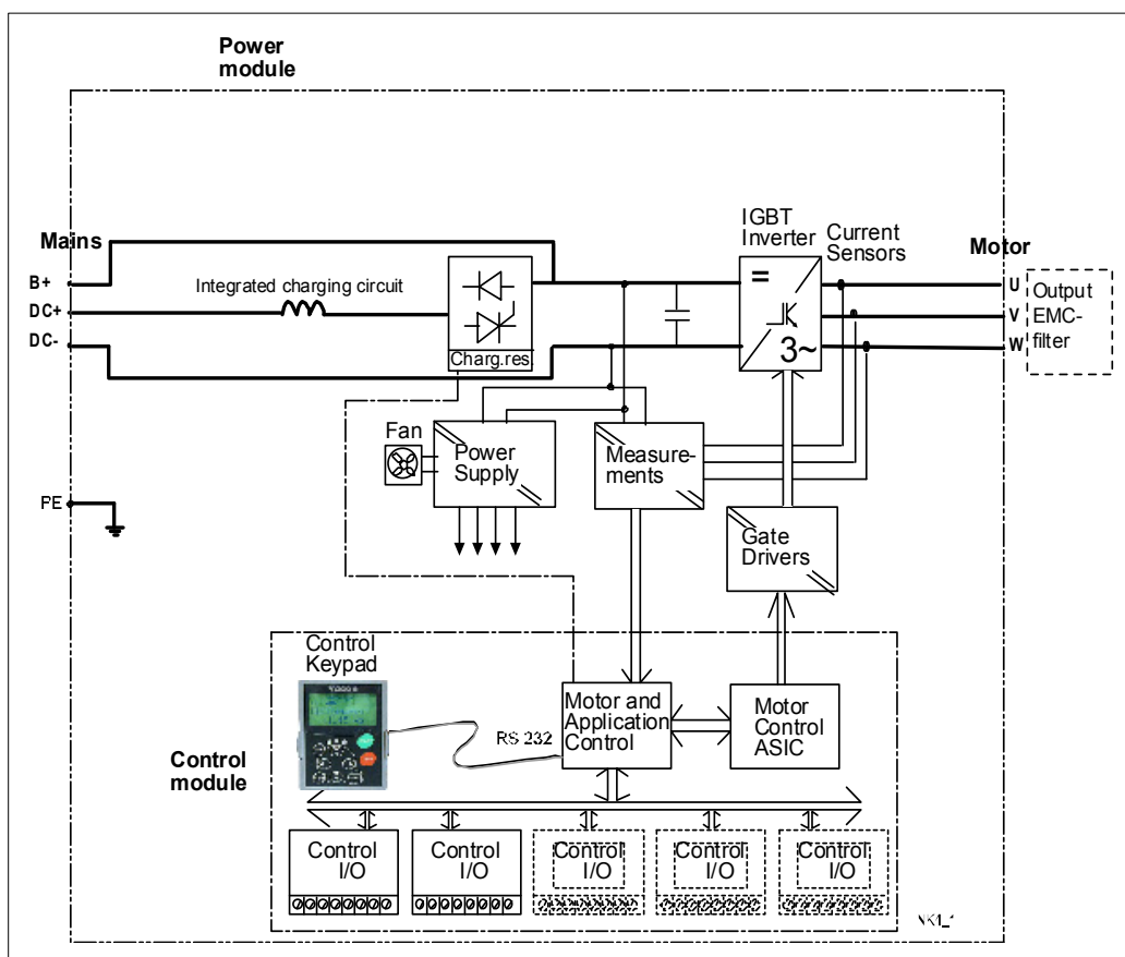
图4-1, Vacon NX 变频器框图
