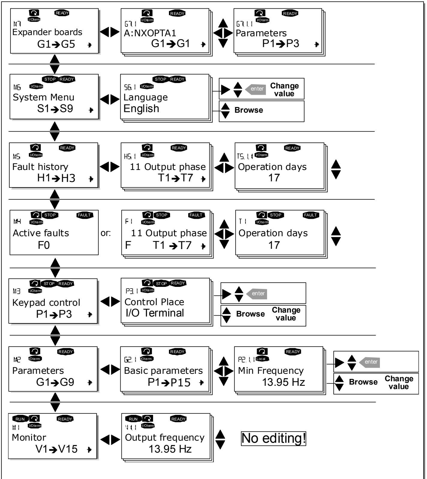
图 7-2. 面板操作导航图
