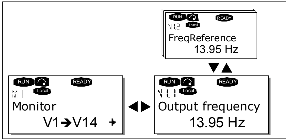
图 7-3, 监控菜单
