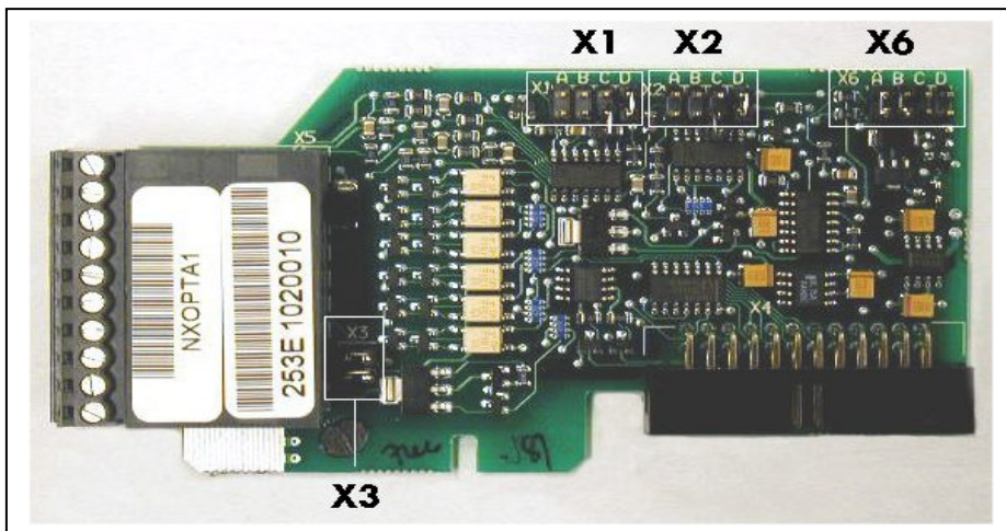
图 6-14, NXOPTA1 板上的跳线块
