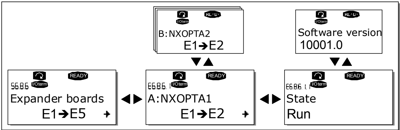
图 7-22, 选件板信息菜单
