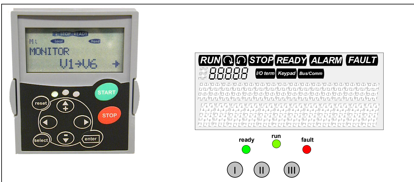
图 7-1, Vacon 控制面板和变频器状态指示
