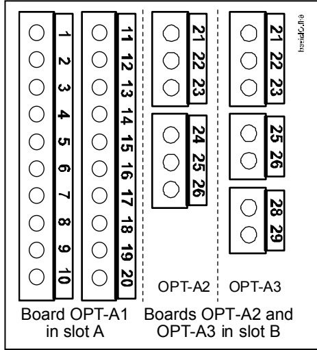
图 6-9, 两块基本板的 I/O 端子
