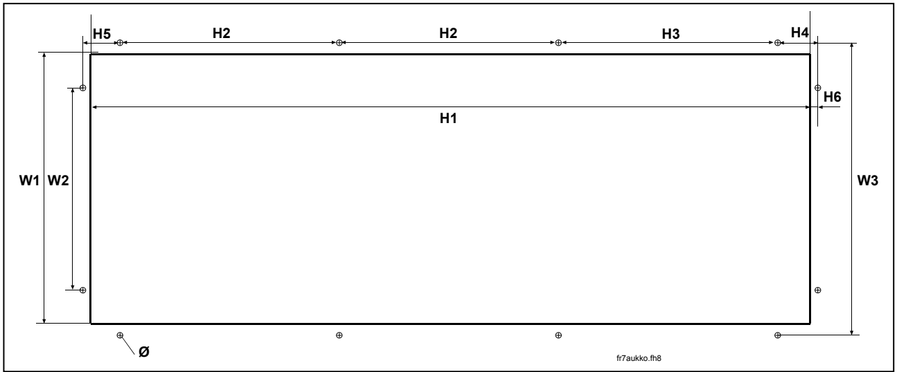
图 5-5, 法兰安装所需开口的尺寸, FR7/FR8。
