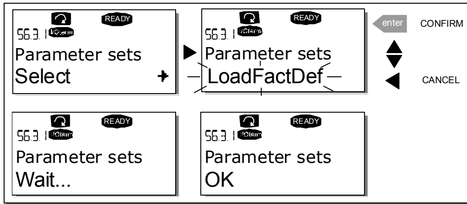
图 7-7，存储和调用参数集
