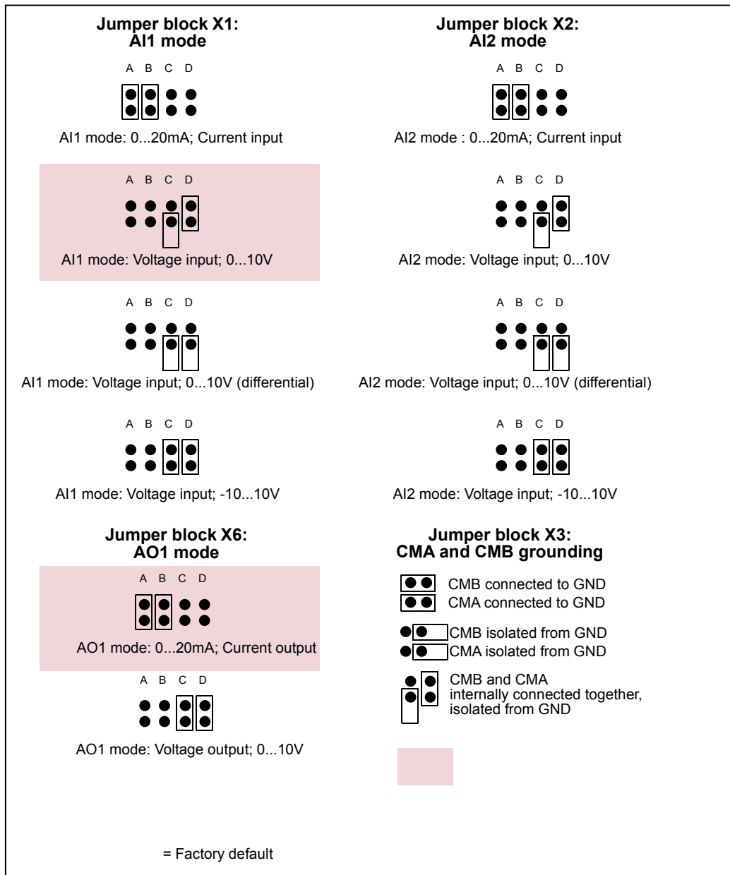
图6-15, NXOPTA1 板上的跳线选择
