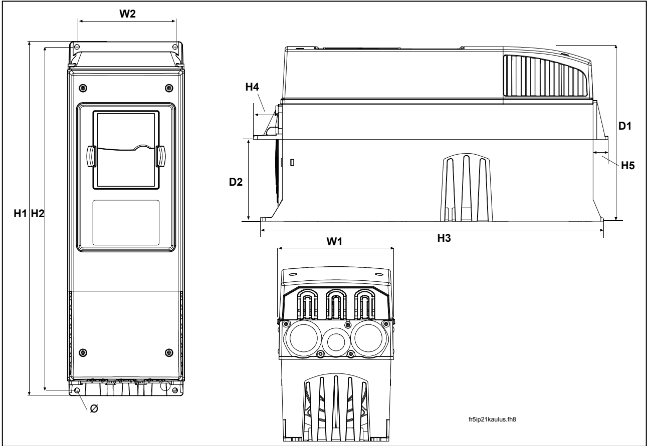
图 5-2, Vacon NX 尺寸 FR4 和 FR6，法兰安装。
