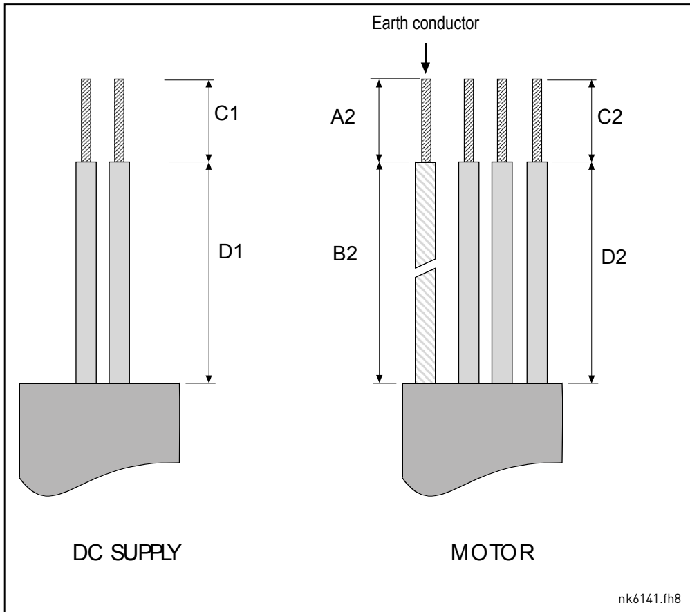
图 6-2，剥除电缆绝缘层。
