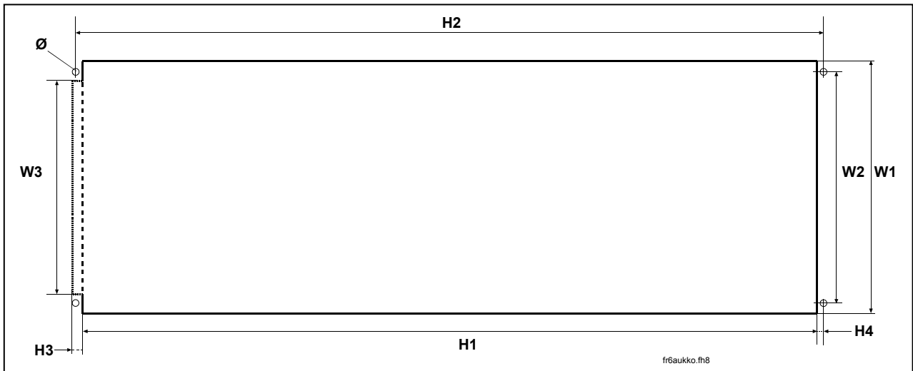
图 5-3，法兰安装所需开口的尺寸，FR4 和 FR6。
