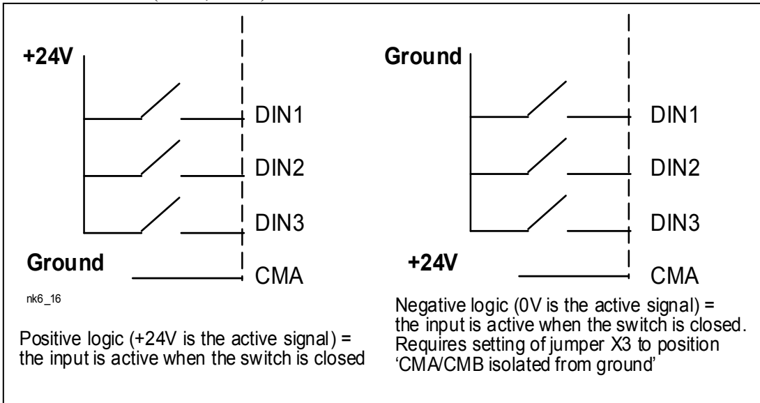
图 6-13, 正/负逻辑
