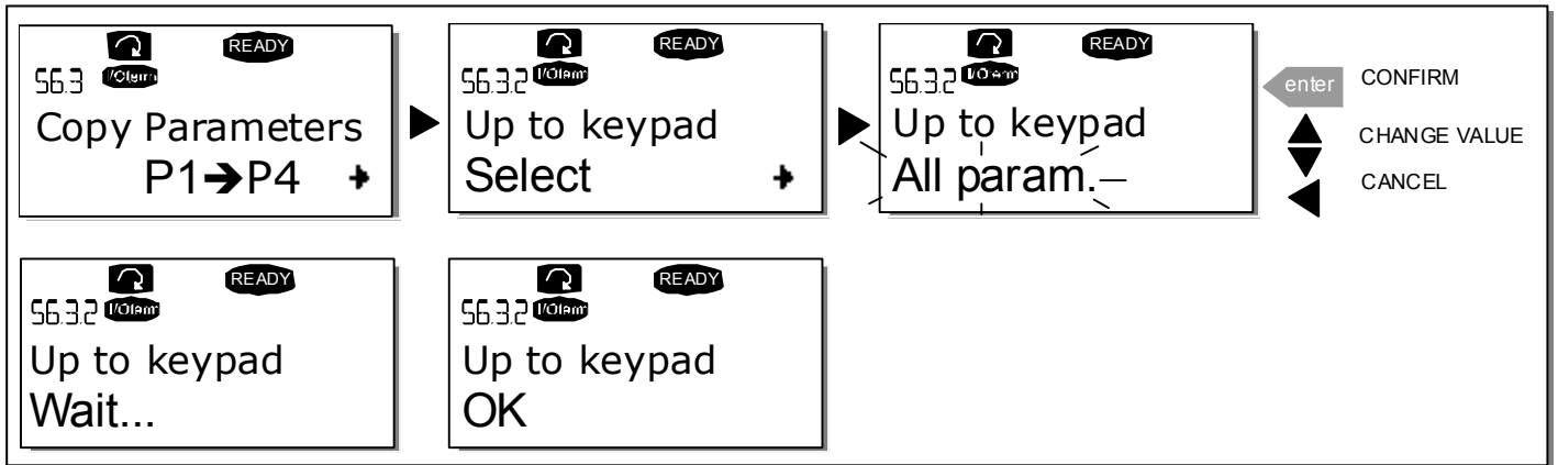
图 7-8，上传参数到控制面板
