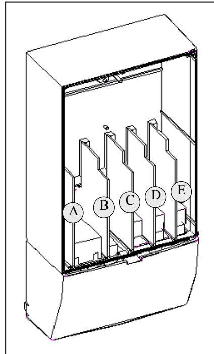
图 6-8, 基本板和选件板与控制板的连接
