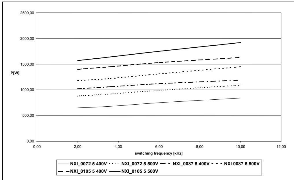
图 5-7，功率损失取决于开关频率; NXI 0061...0105 5
