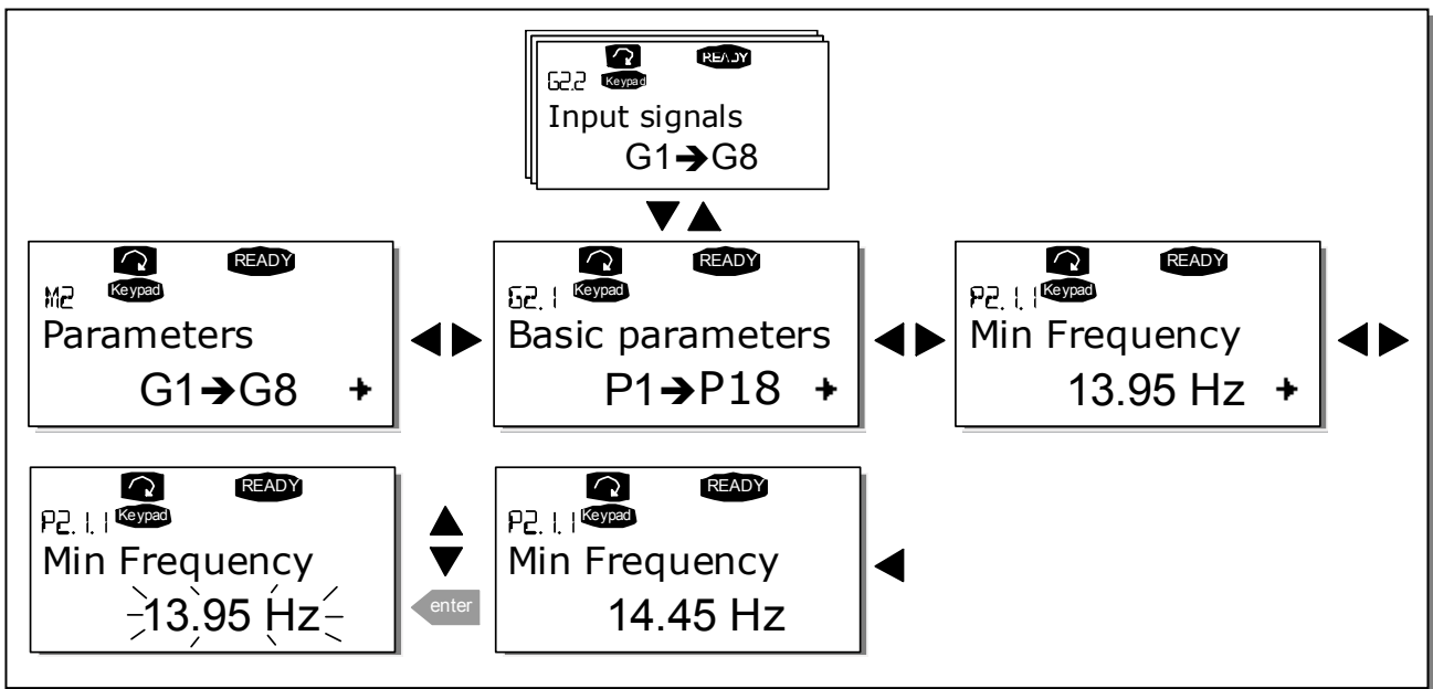
图 7-1. 参数值修改过程
