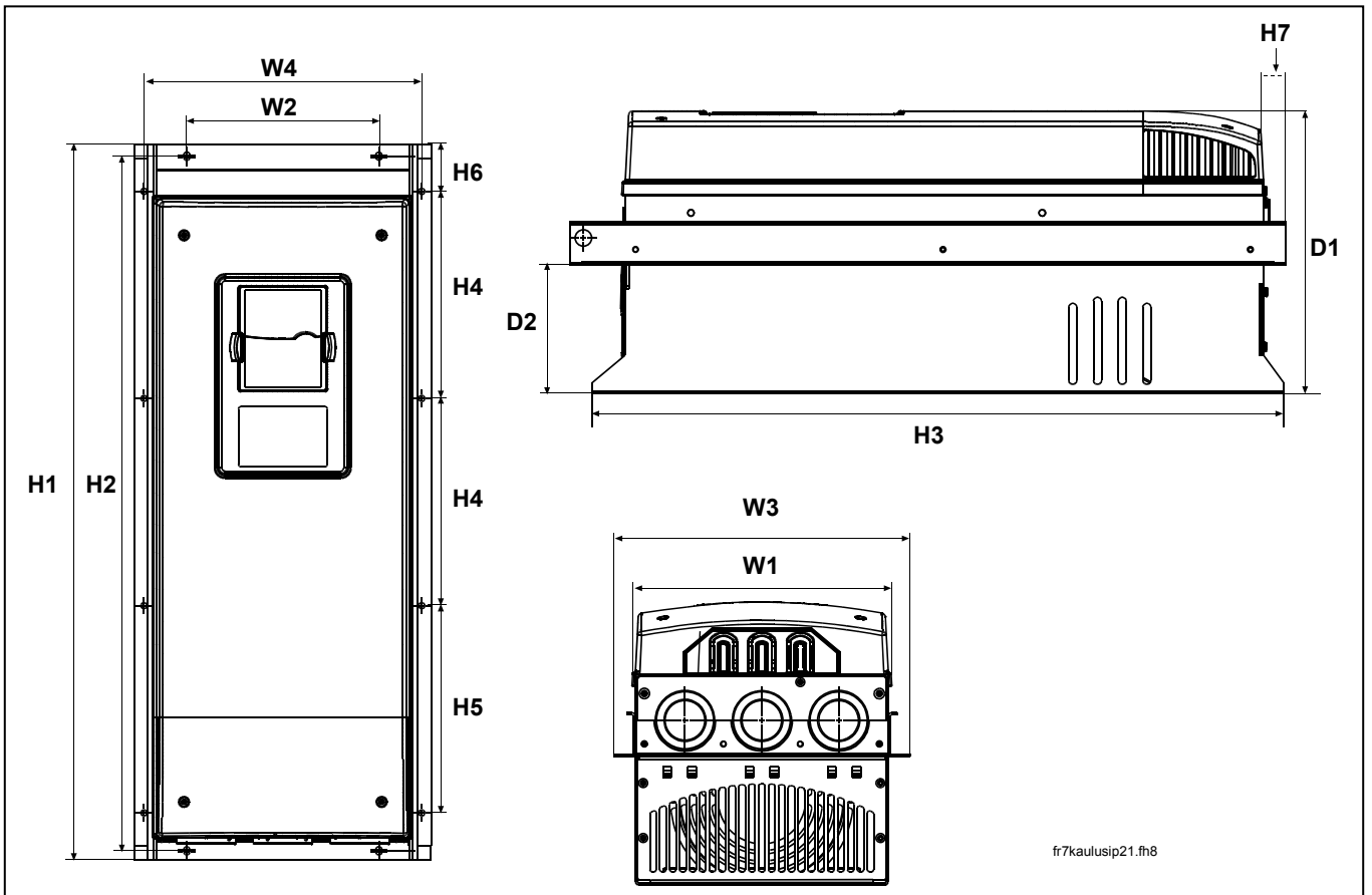
图 5-4, Vacon NX 尺寸 FR4 -FR6 , 法兰安装
