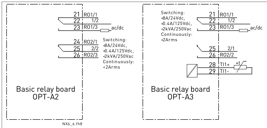
图 6-11, 基本继电器输出板(NXOPTA2/NXOPTA3)的常规连线图
