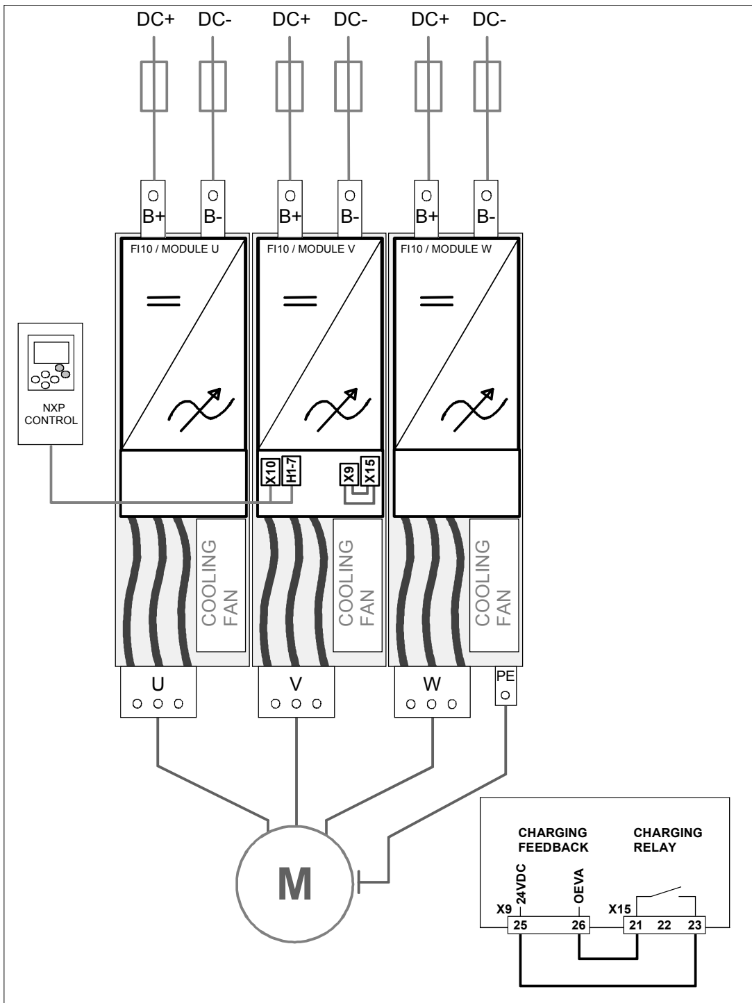
图 6-5 FI13 无充电基本接线图
