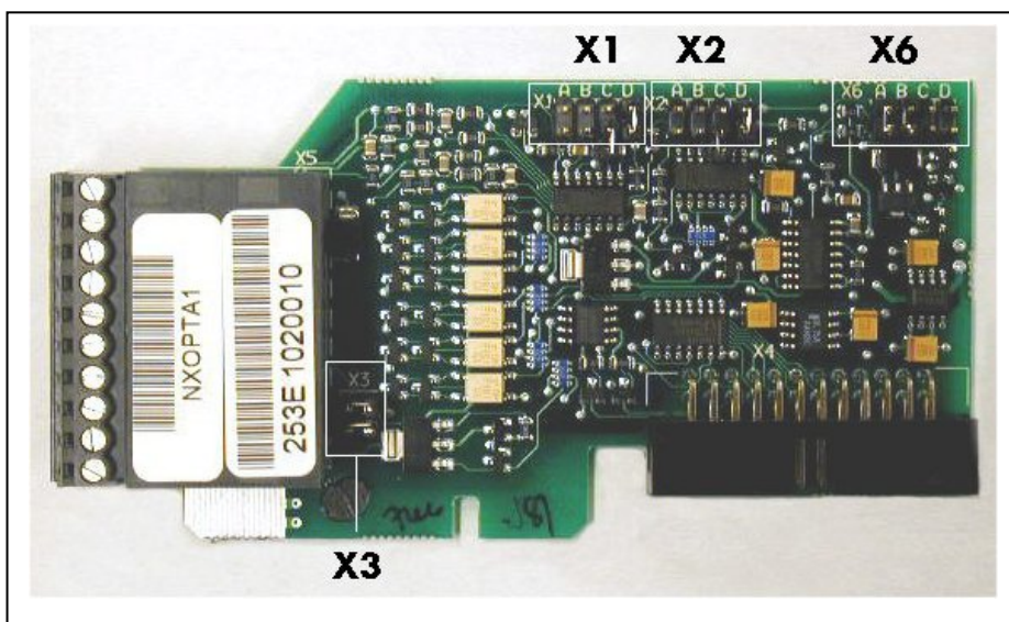
图 6-20 OPT-A1 上的跳线块
