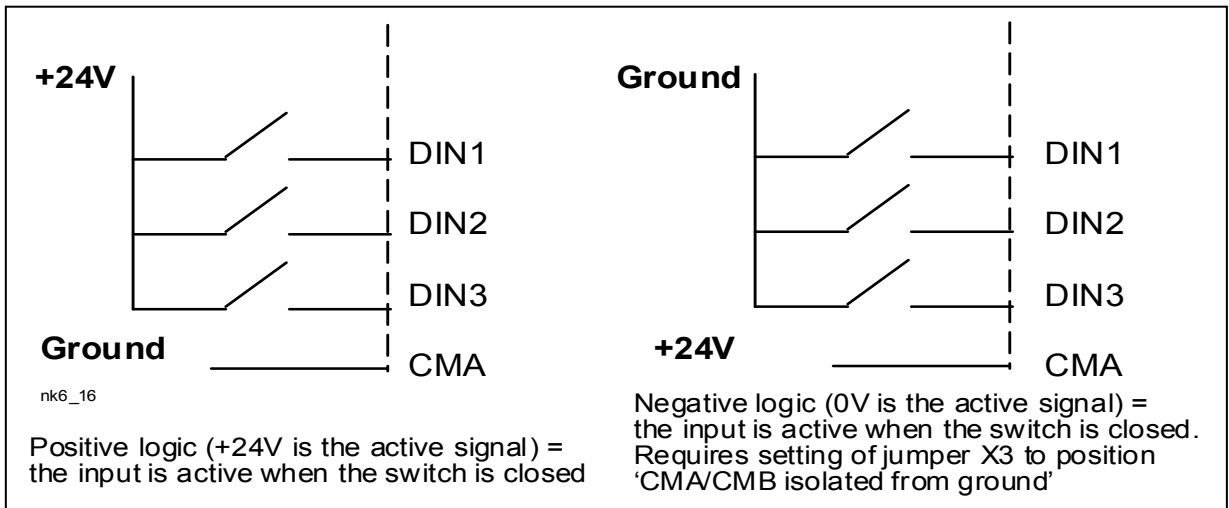
图 6-19 正/负逻辑
