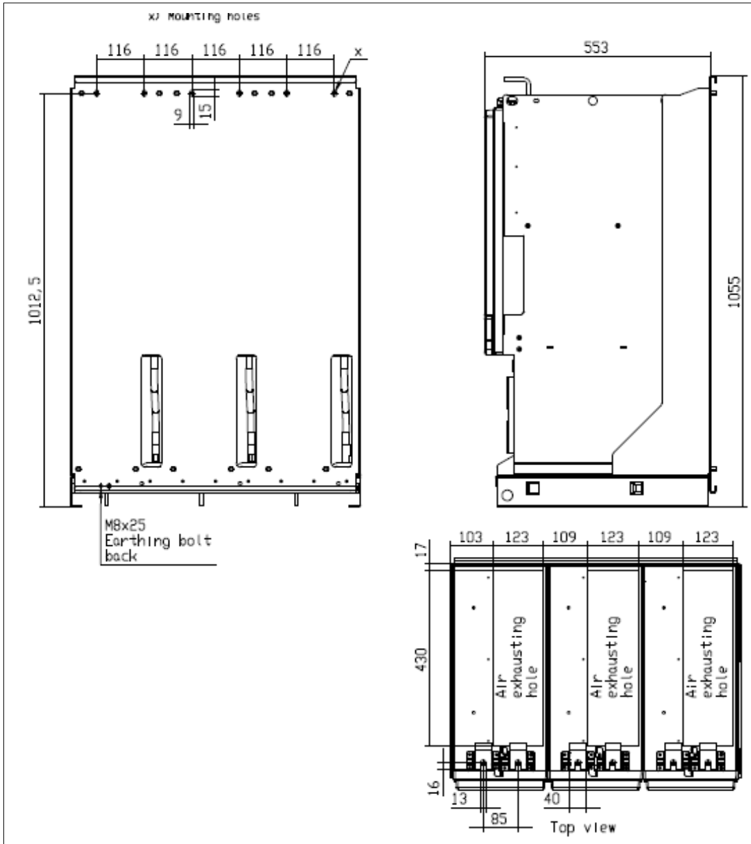
图 5-5 Vacon NXI 尺寸, FI13 背视图, 注, FI14 是两个 FI13
