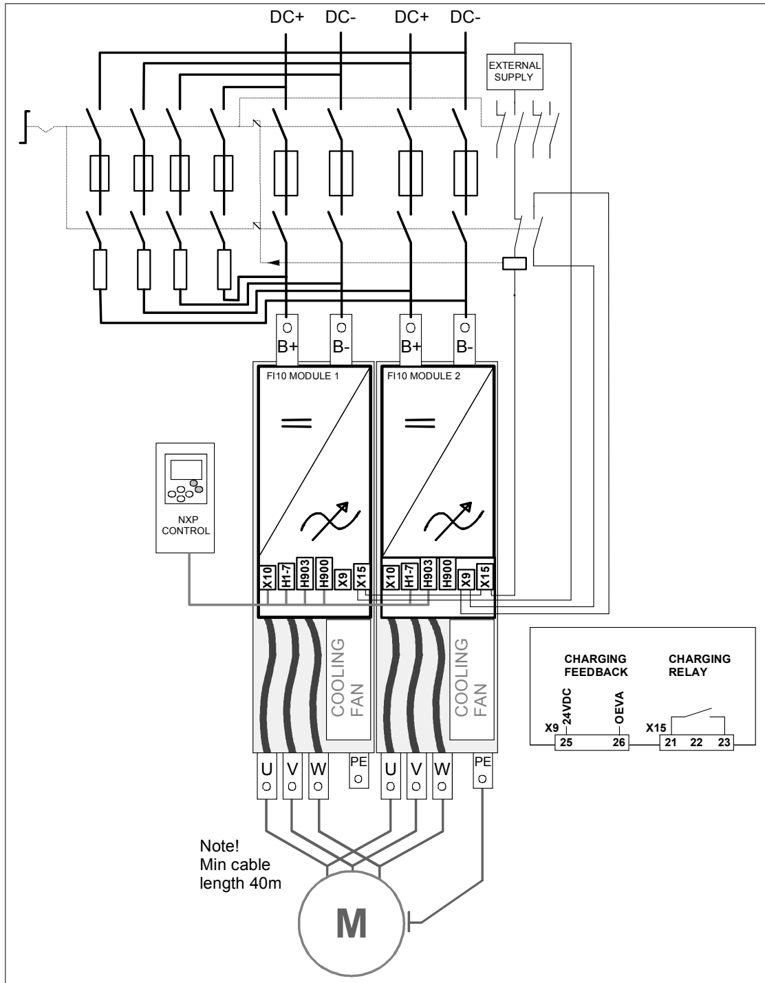
图 6-4 FI12 充电基本接线图
