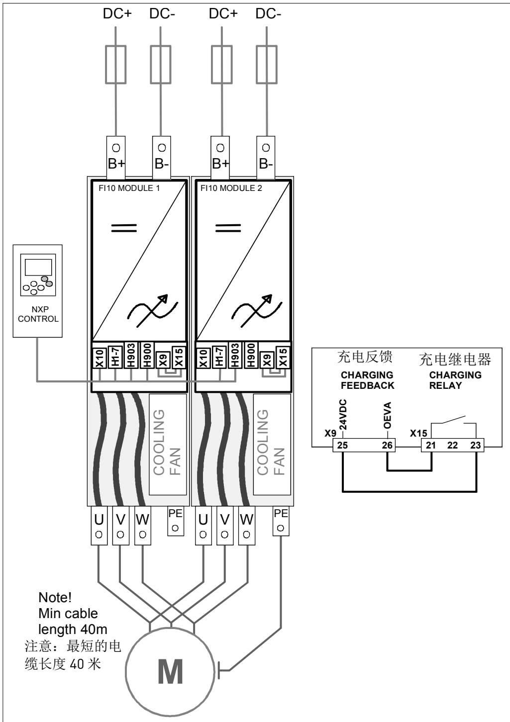
图 6-3 FI12 无充电的基本接线图
