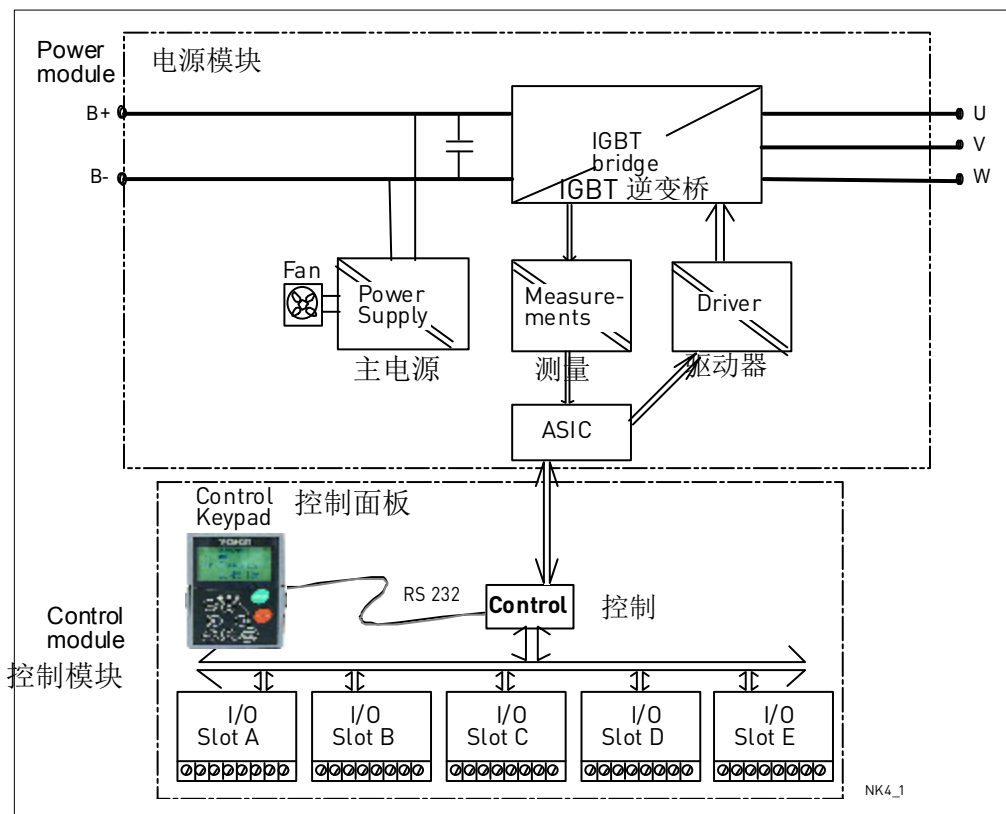
图 4-1 Vacon NXI 变频器的框图
