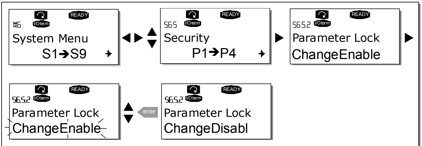
图 7-11 参数锁定
