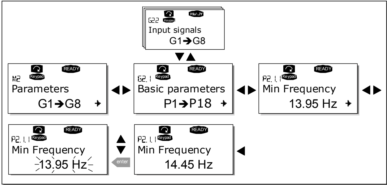
图 7-4 参数值修改流程
