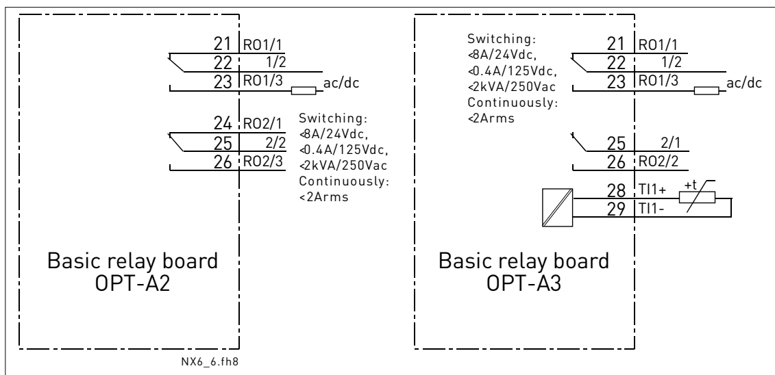
图 6-17 基本继电器板的常规接线图
