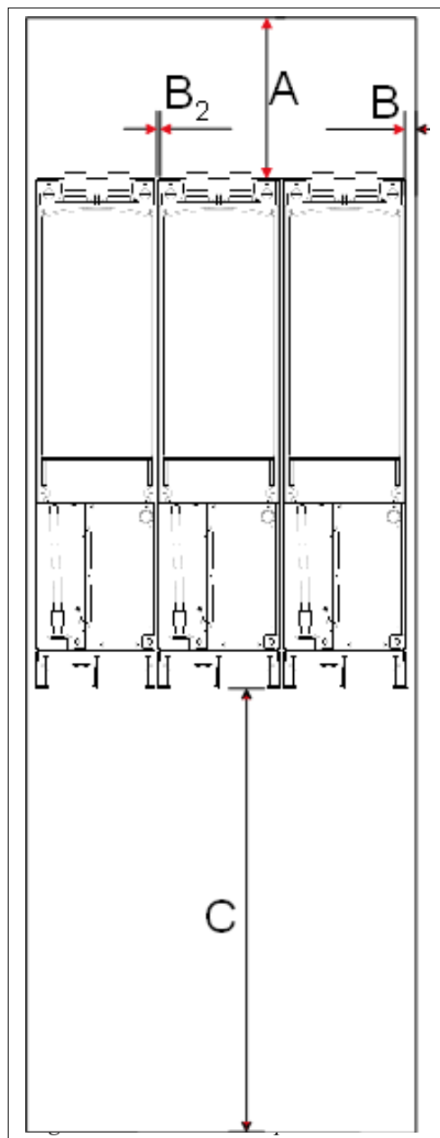
图 5-7 安装空间
