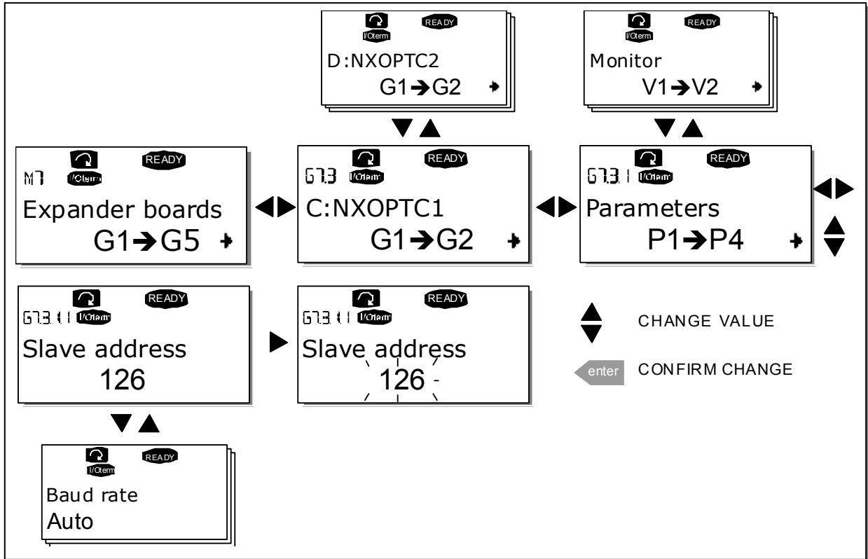
图 7-23 扩展板信息菜单
