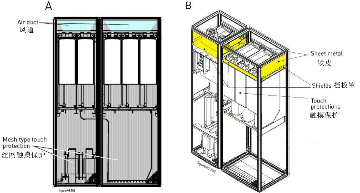
图 5-9 控制柜冷却气流指示
