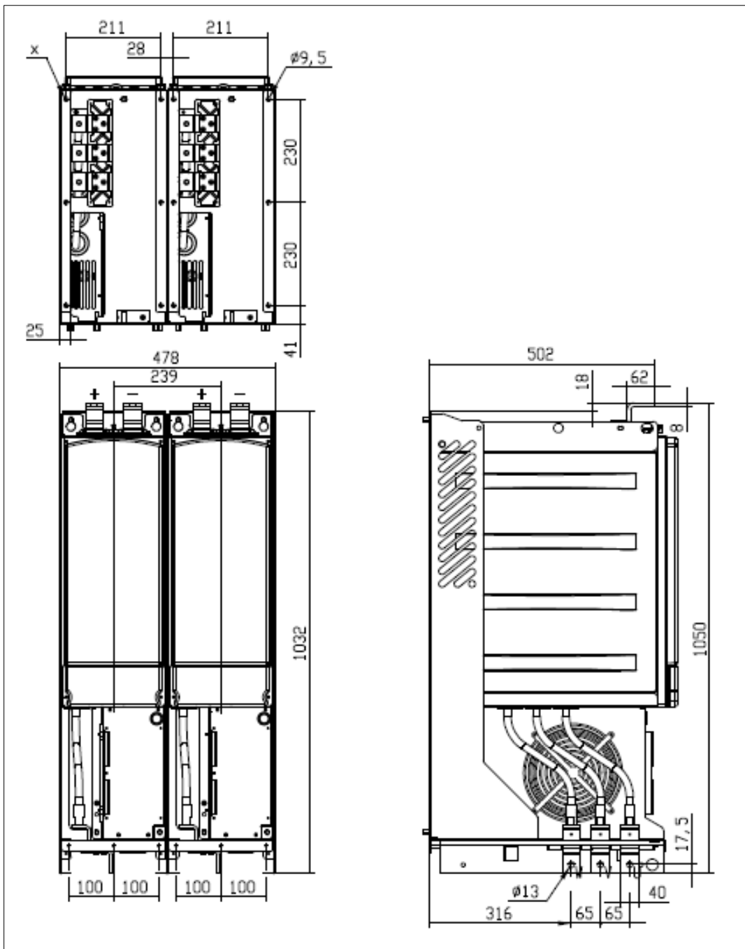
图 5-4 Vacon NXI 尺寸, FI12 正视图
