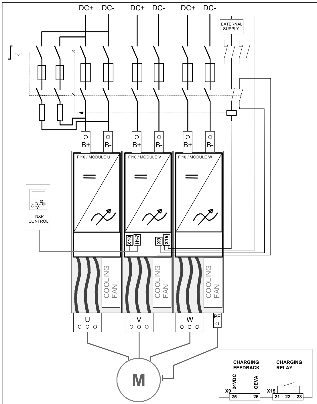
图 6-6 FI13 充电基本接线图
