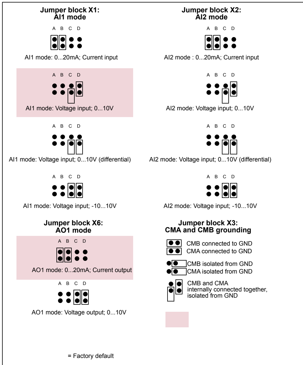
图 6-21 OPT-AI 跳线选择
