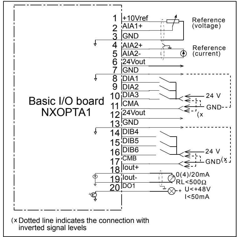
图 6-16 基本 I/O 板的常规接线图
