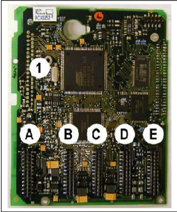
图6-13.控制板
