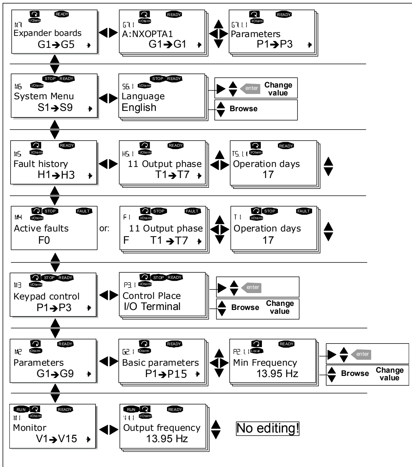
图7-2 面板导航表
