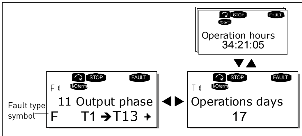
图 7-3 故障显示
