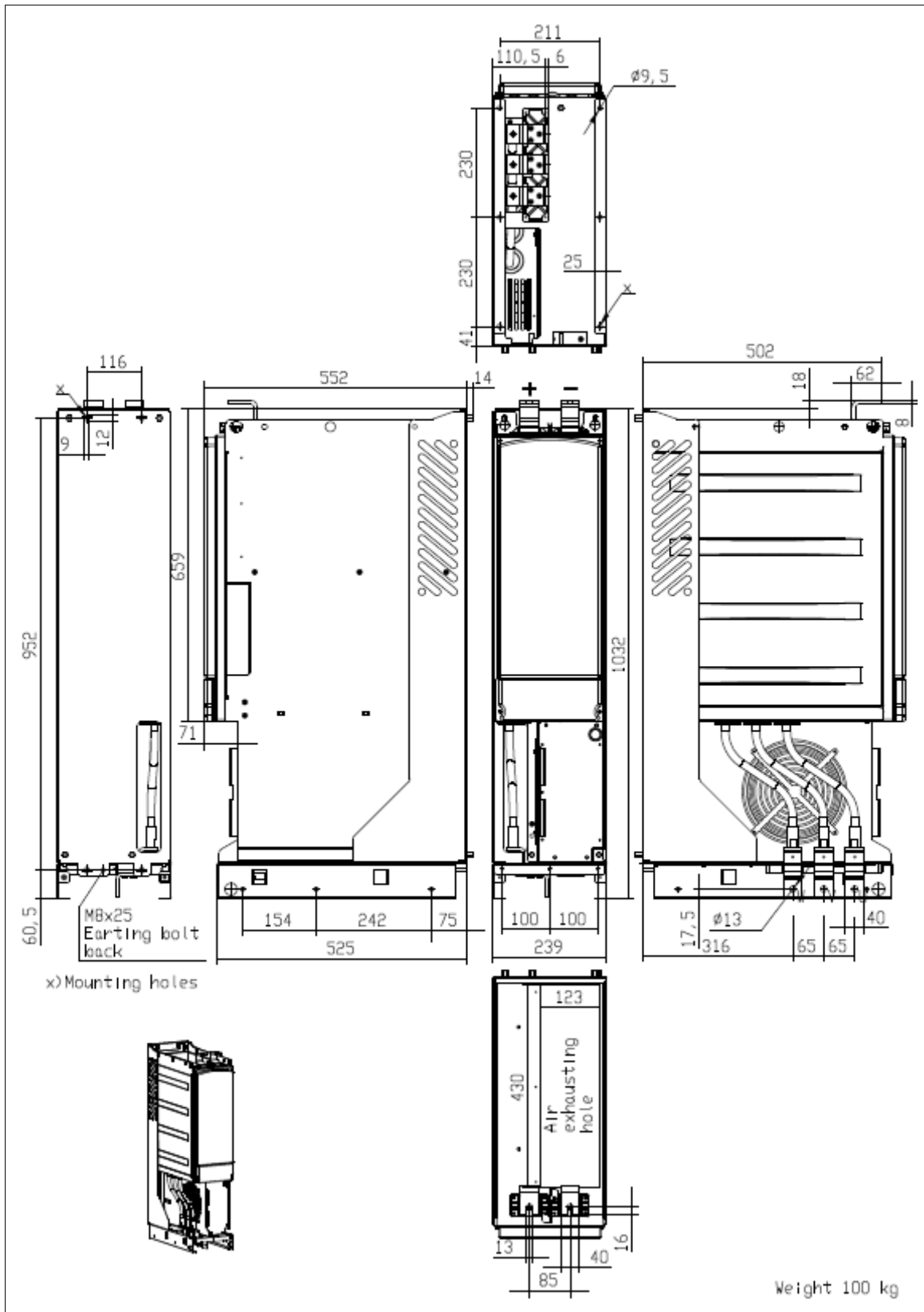
Vacon NXI 尺寸, F110
