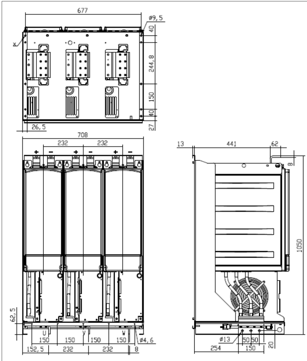
图 5-6 Vacon NXI 尺寸，FI13 正视图，注意，FI14 是两个 FI13
