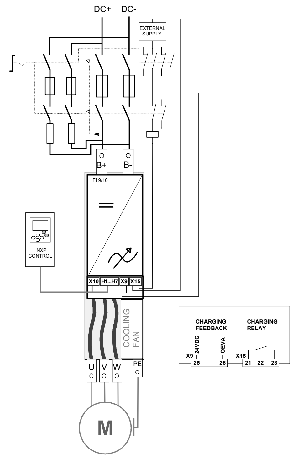
图6-2 F19/10 充电的基本接线图
