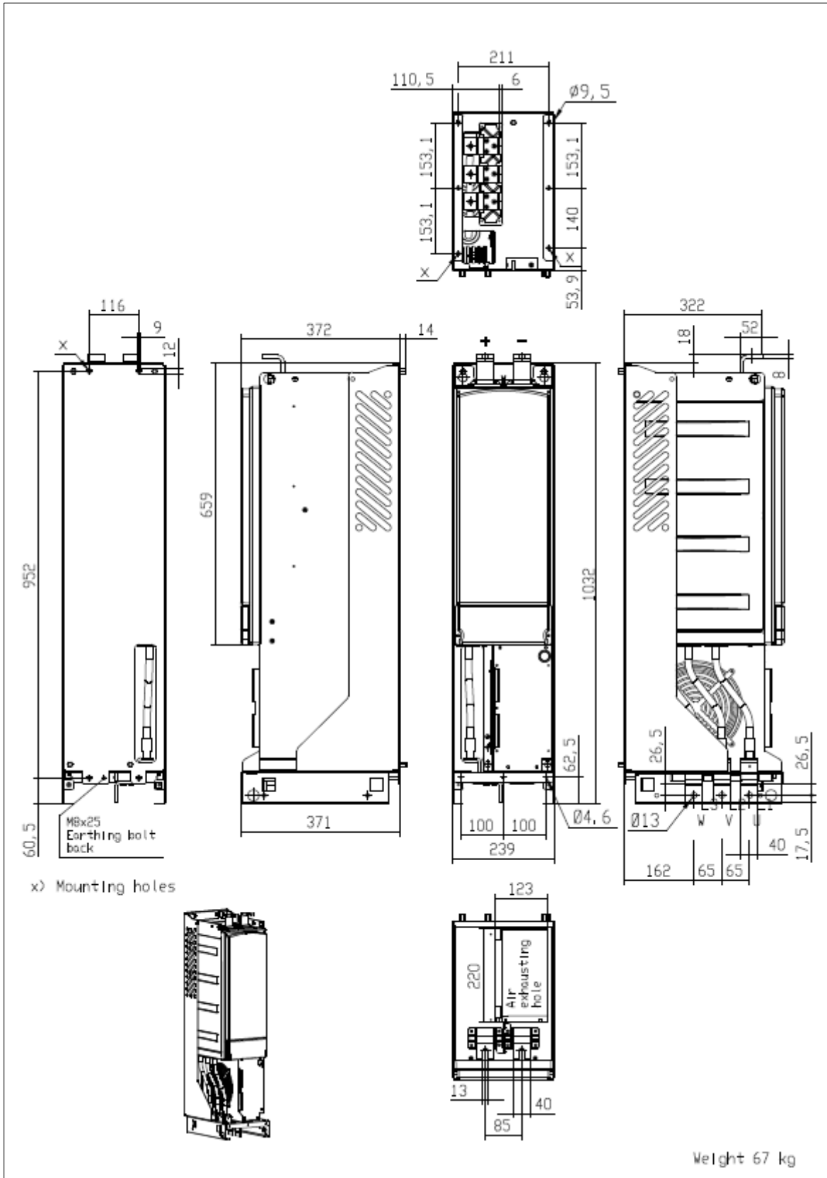
图5-1 Vacon NXI FI9 尺寸
