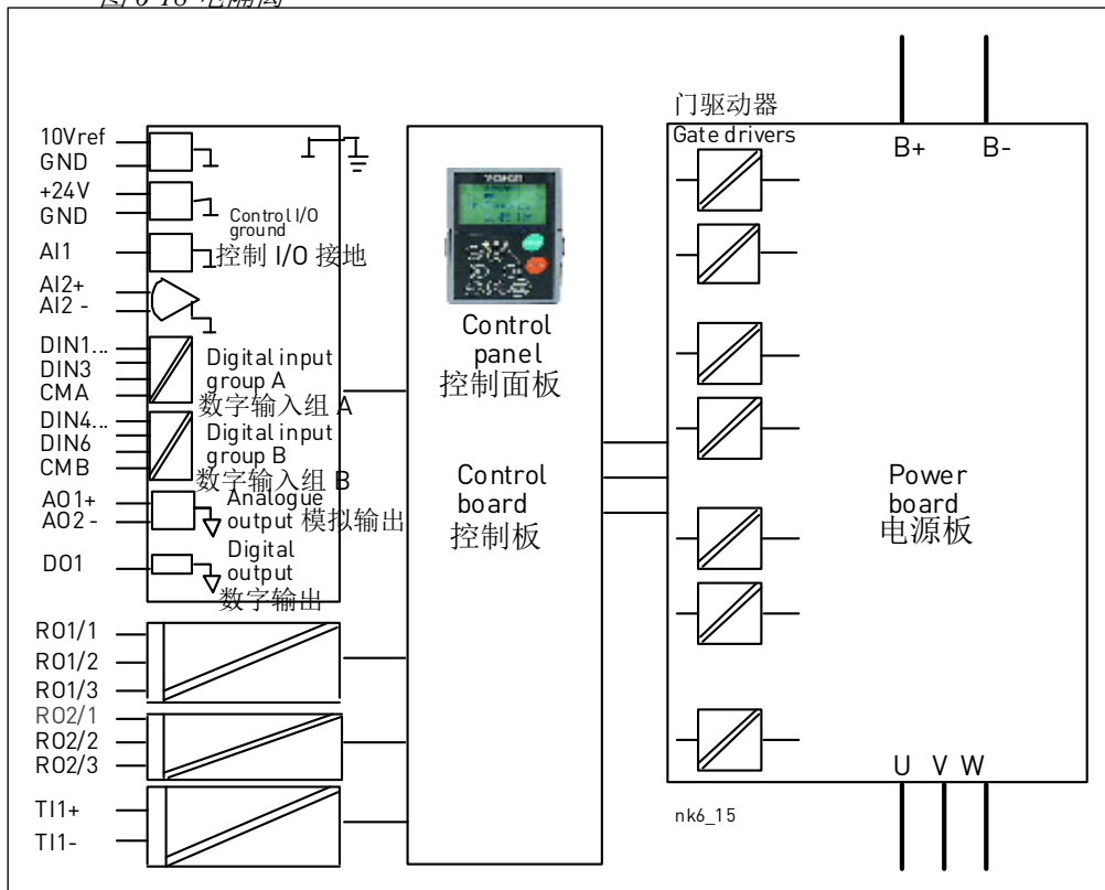
图 6-18 电隔离
