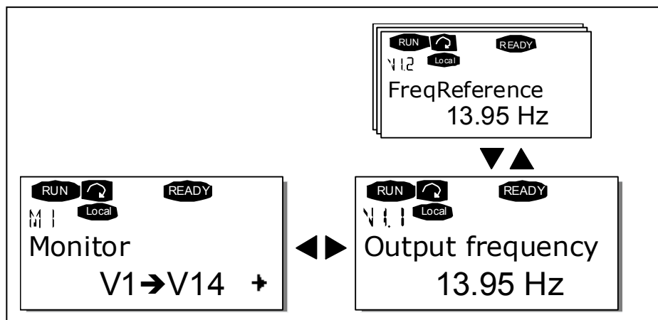
图 7-3 监测菜单
