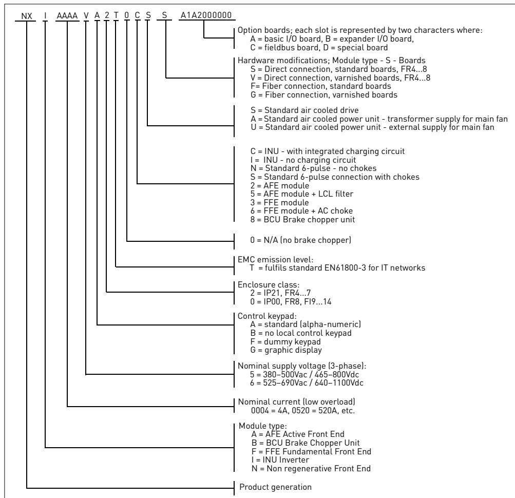
图 3-1 Vacon NX FI9 – FI14 型号标识码
