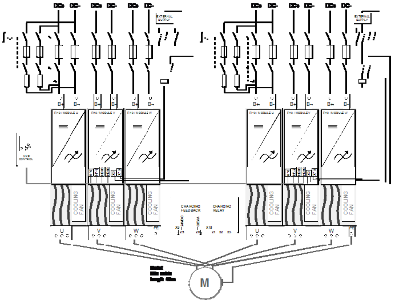
图6-8 FI14 充电基本接线图
