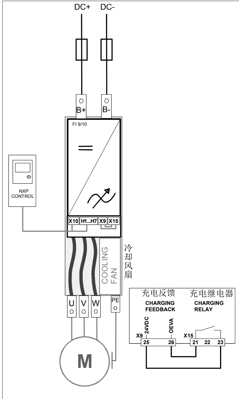
图 6-1 FI9/10 无充电的基本接线图
