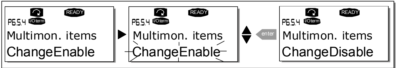
图 7-13 禁止多监控项内容变化
