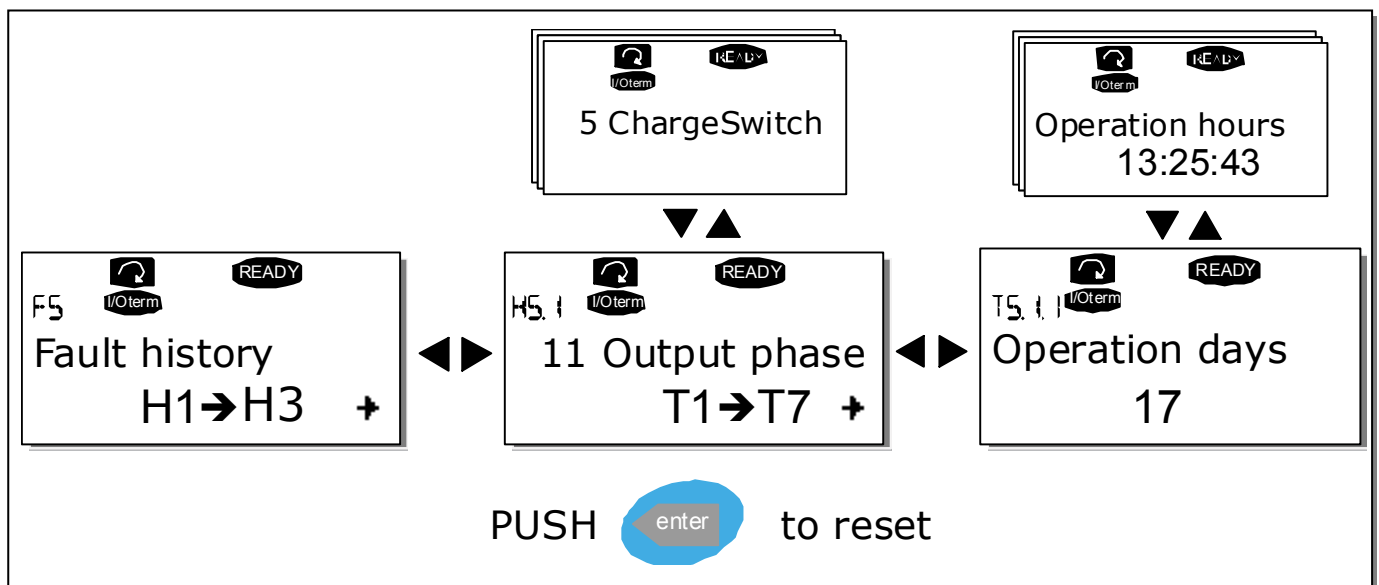
图 7-4 故障历史菜单
