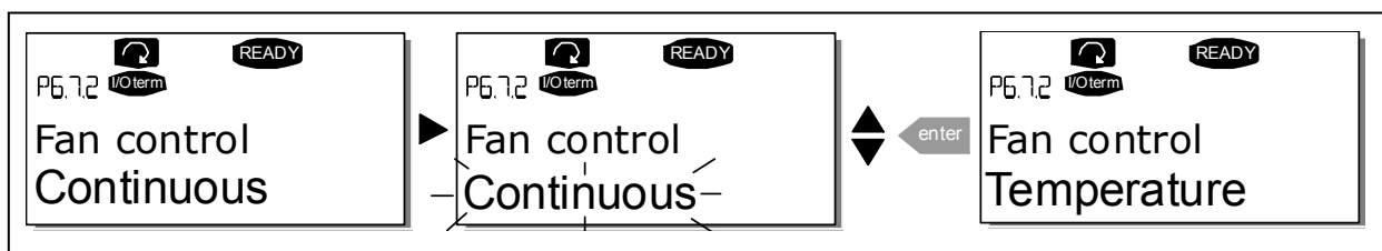
图 7-18 风扇控制功能
