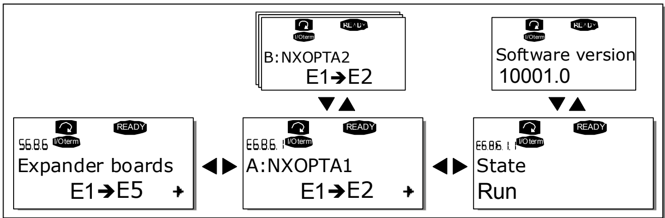
图 7-22, 扩展板信息菜单
