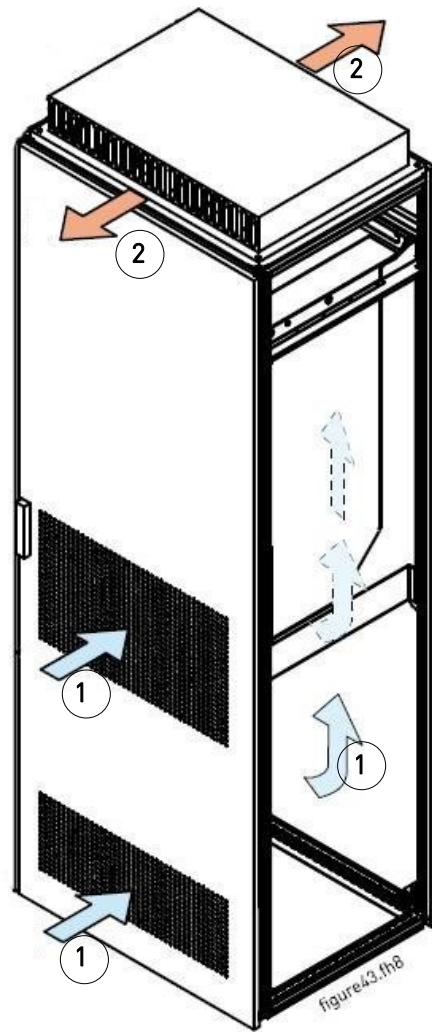
图5-8 控制柜冷却开口
