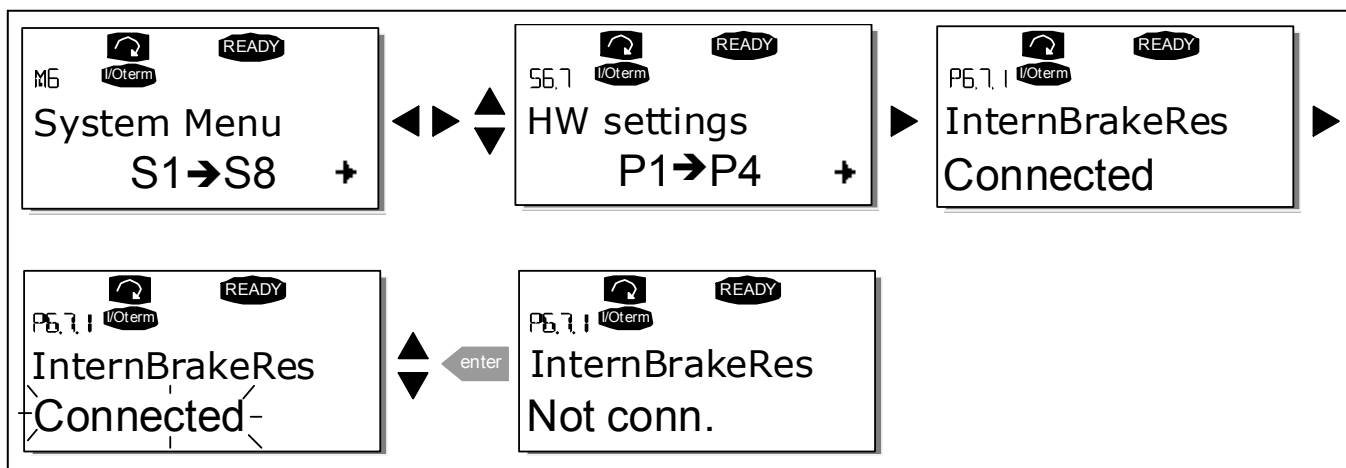
图 7-17，内部制动电阻的连接
