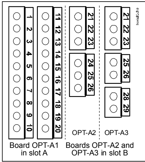
图 6-15 两个基本板的 I/O 端子
