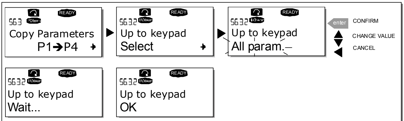
图 7-8 参数复制到面板
