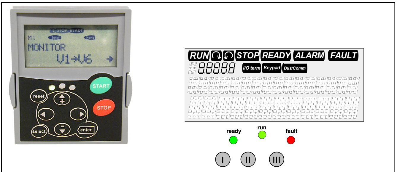
图 7-1 Vacon 控制面板和变频器状态显示
