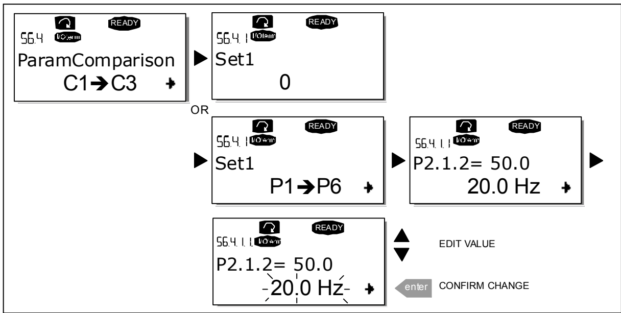
图 7-9 参数比较
