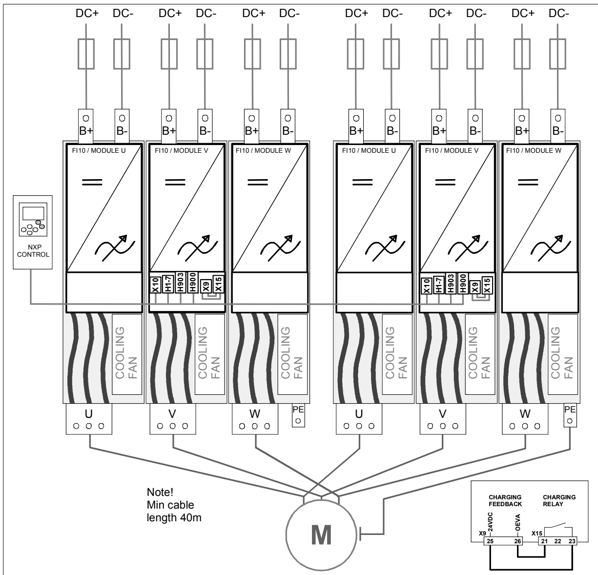
图 6-7 FI14 无充电基本接线图
