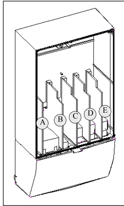
图6-14.控制板上的基本板和选件板连接
