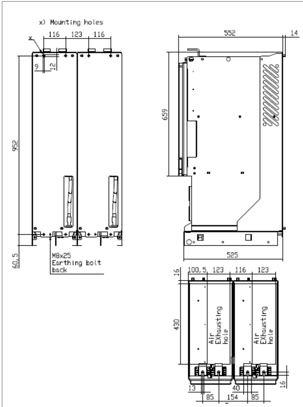
图5-3 Vacon NXI 尺寸, FI12 后视图
