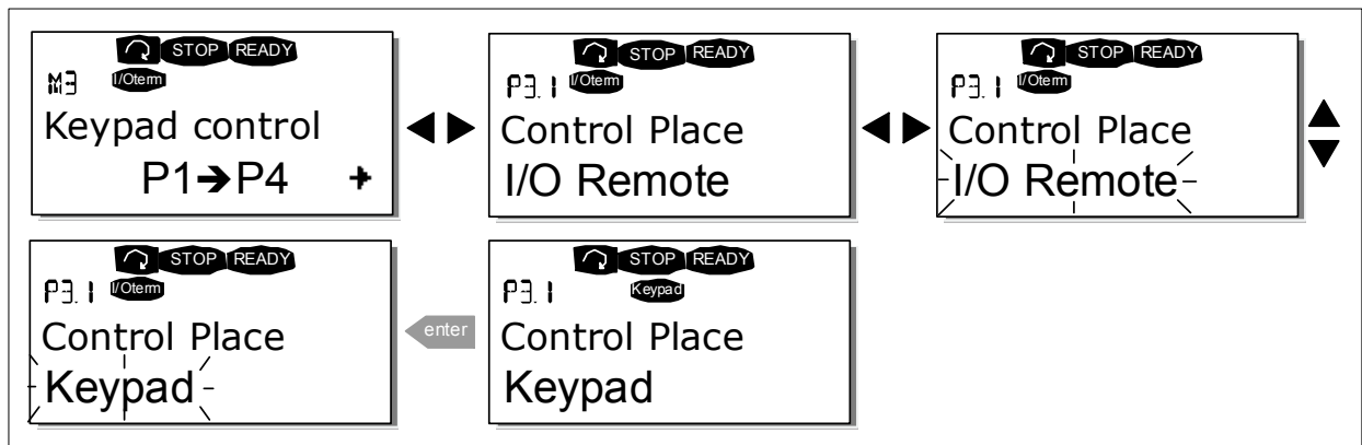
图7-5 控制信号源的选择
