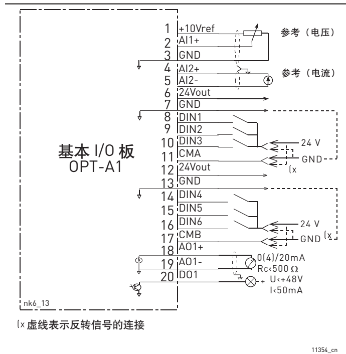
图 44. 基本 I/O 板 (OPT-A1) 的一般接线图
