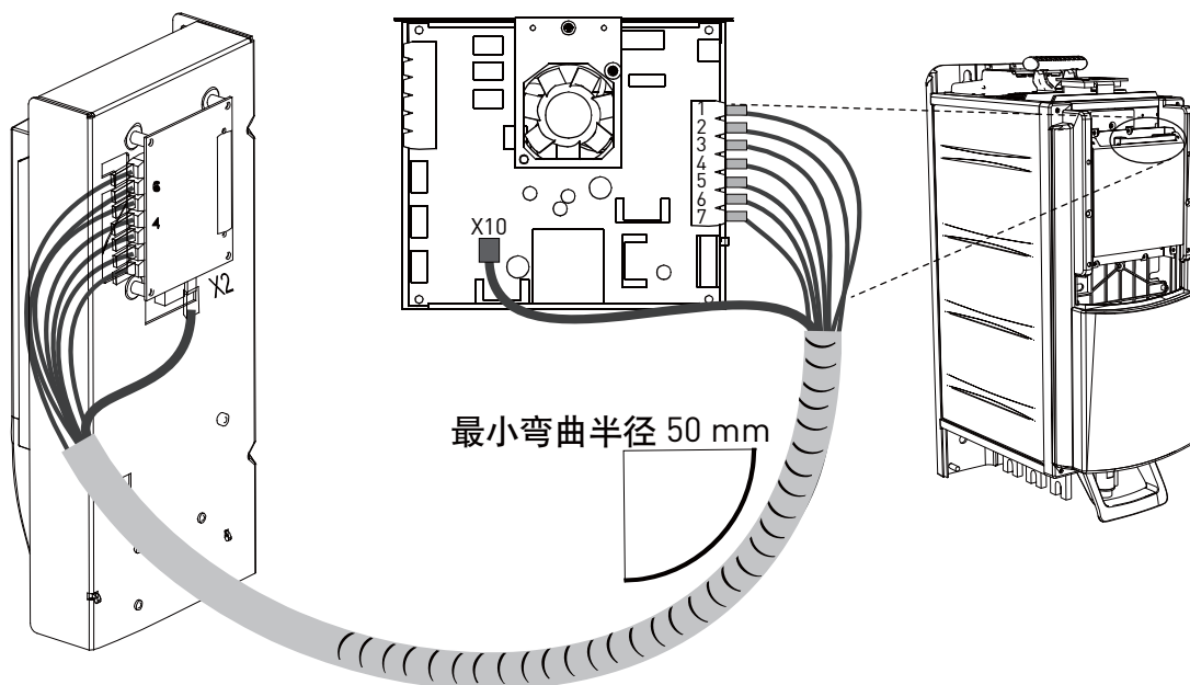
图 56. 将电源和控制电缆连接到控制单元，Ch6x
