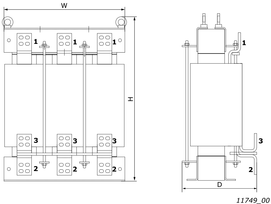
图 104. CHK1030N6A0 电抗器示例
