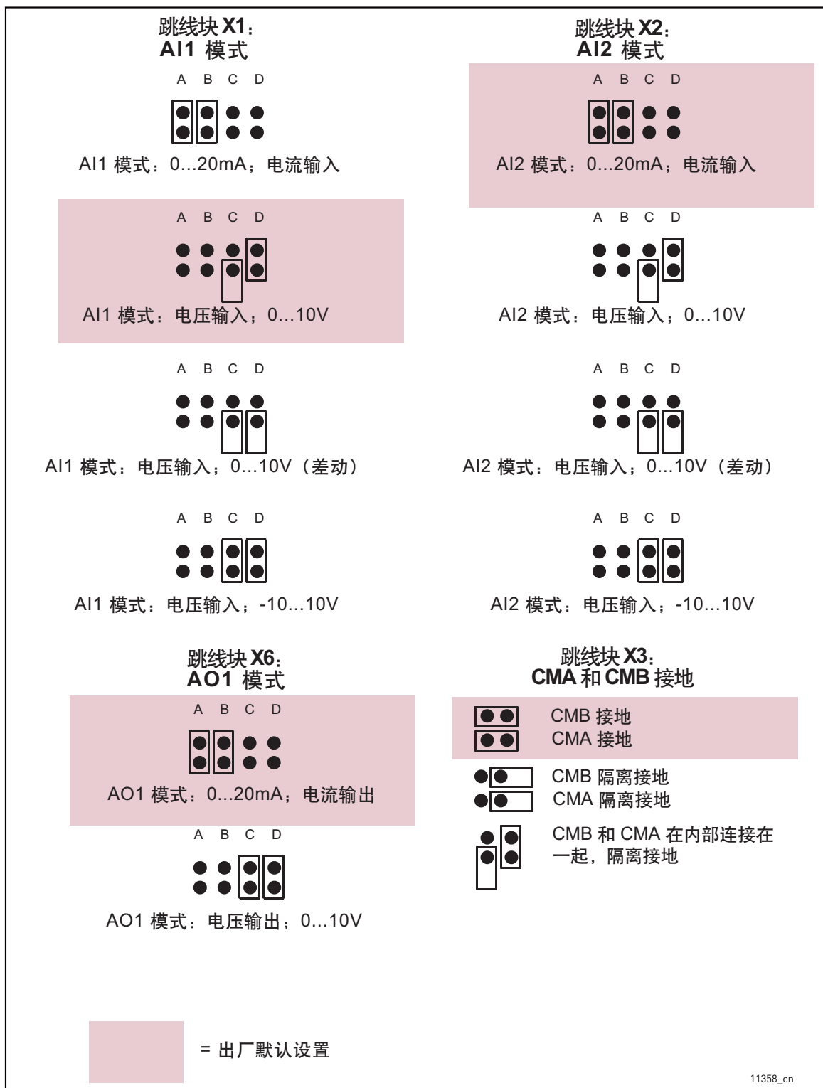
图 49. OPT-A1 的跳线选择
