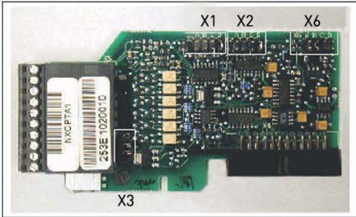
图 48.OPT-A1 上的跳线块
