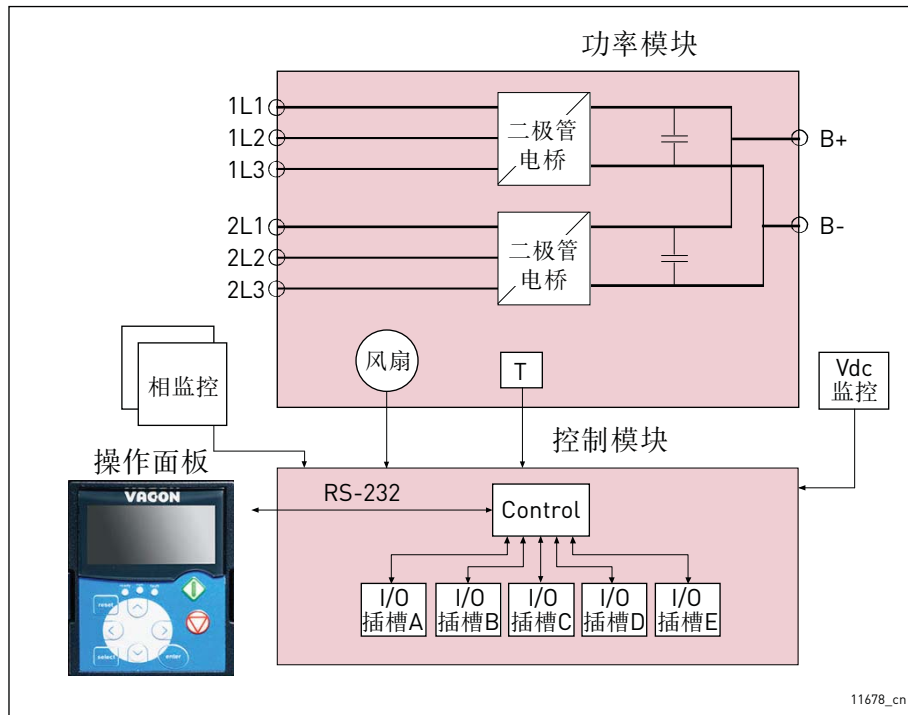
图 102. 无回馈前端模块示意图
