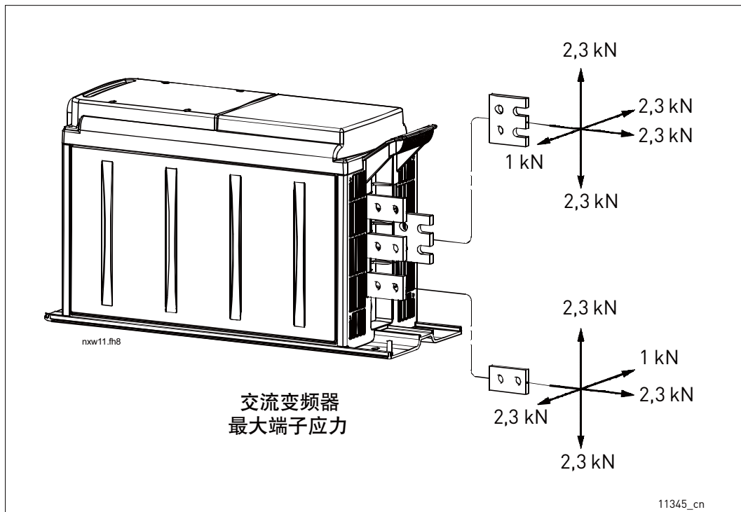
图 37. 最大端子应力
