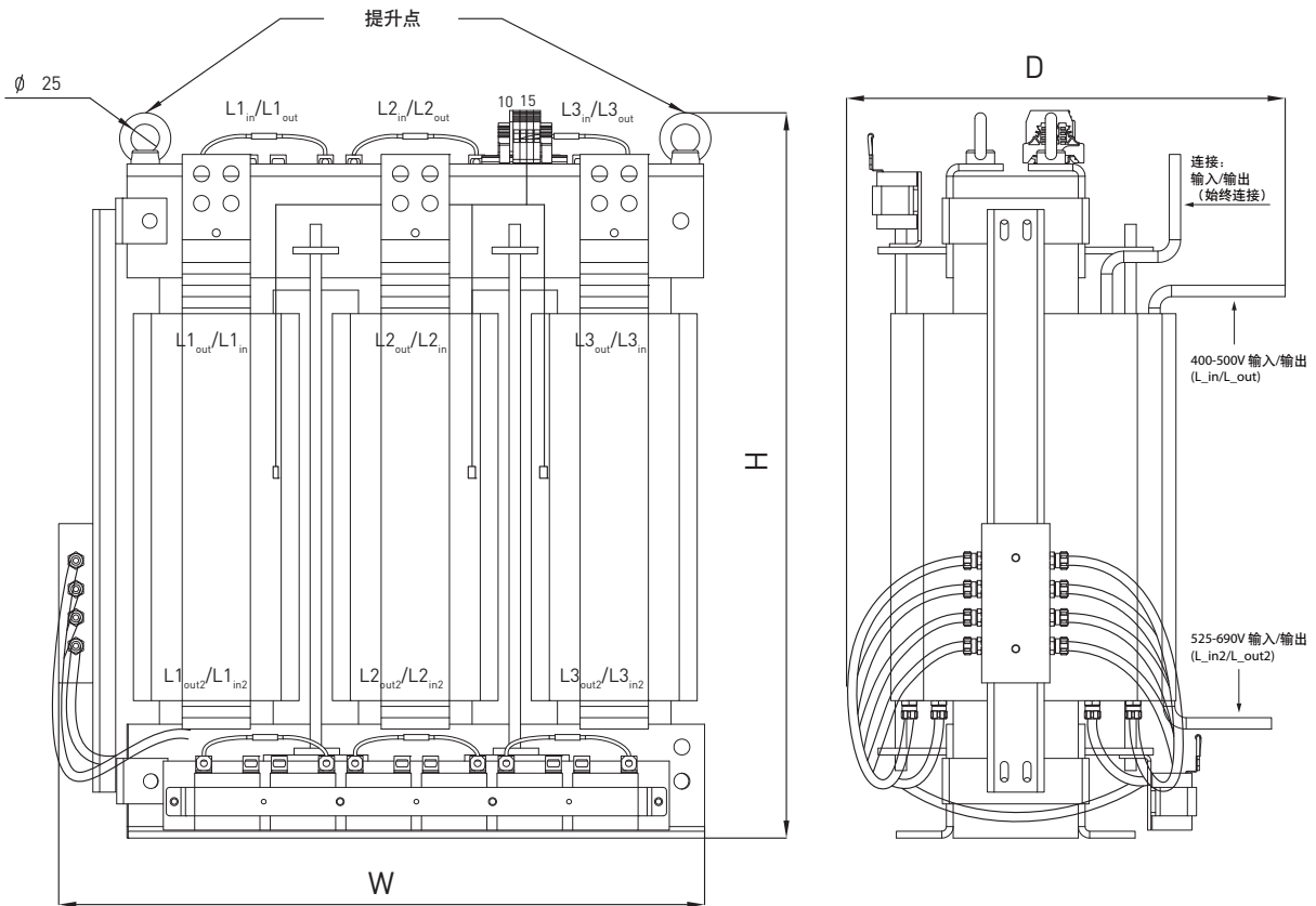
图 88. VACON® RLC 滤波器 L_{net} 电抗器的示例
