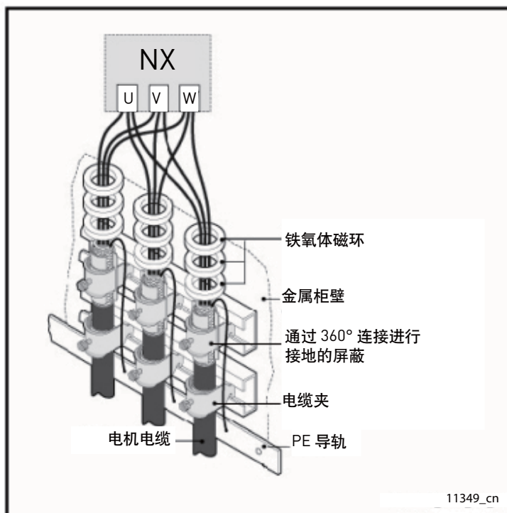
图 40. 铁氧体磁环的安装
