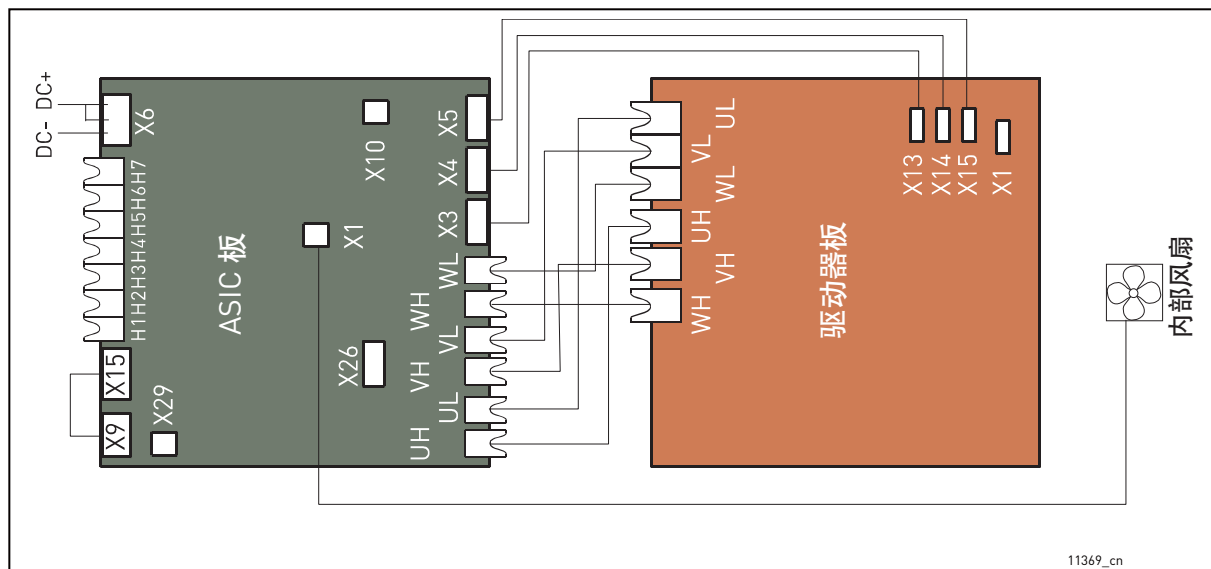
图 52. ASIC 和驱动板 ( CH61、CH62 和 CH72 ) 之间的端子和连接
