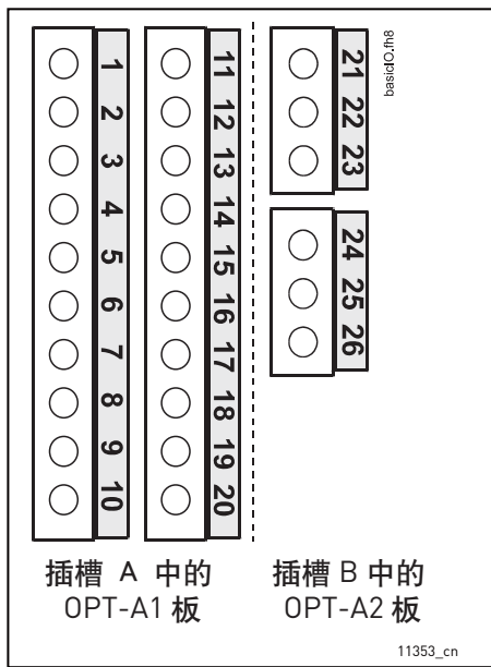
图 43. 两个基本板的 I/O 端子
