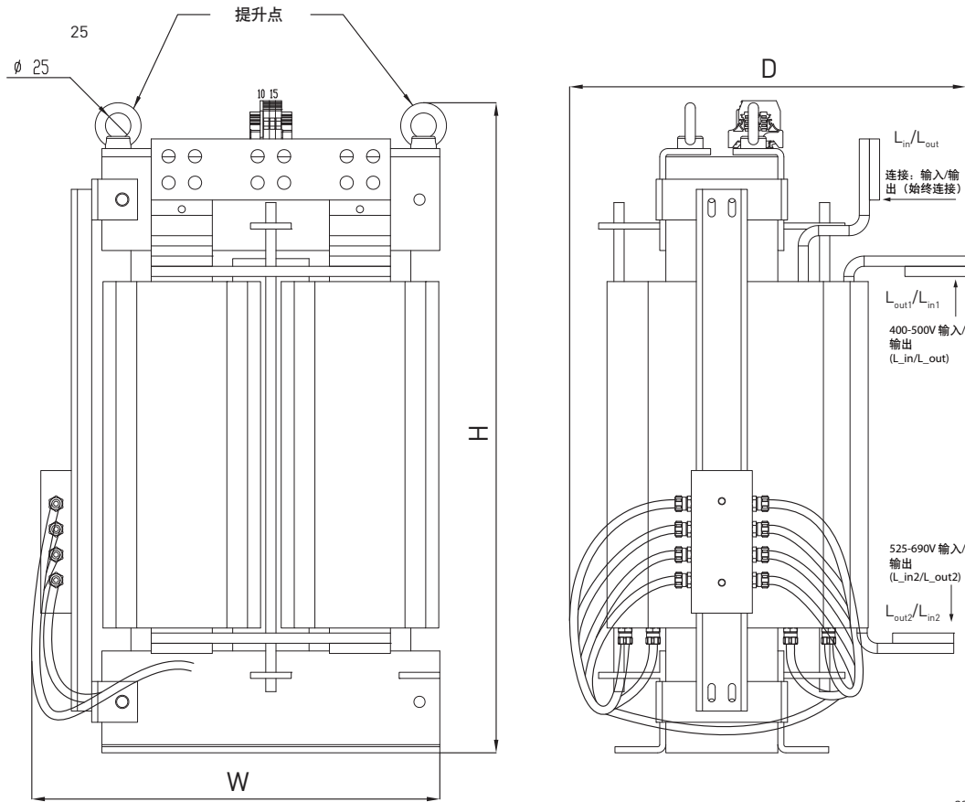
图 89. VACON® RLC 滤波器 L_{afe} 电抗器的示例
