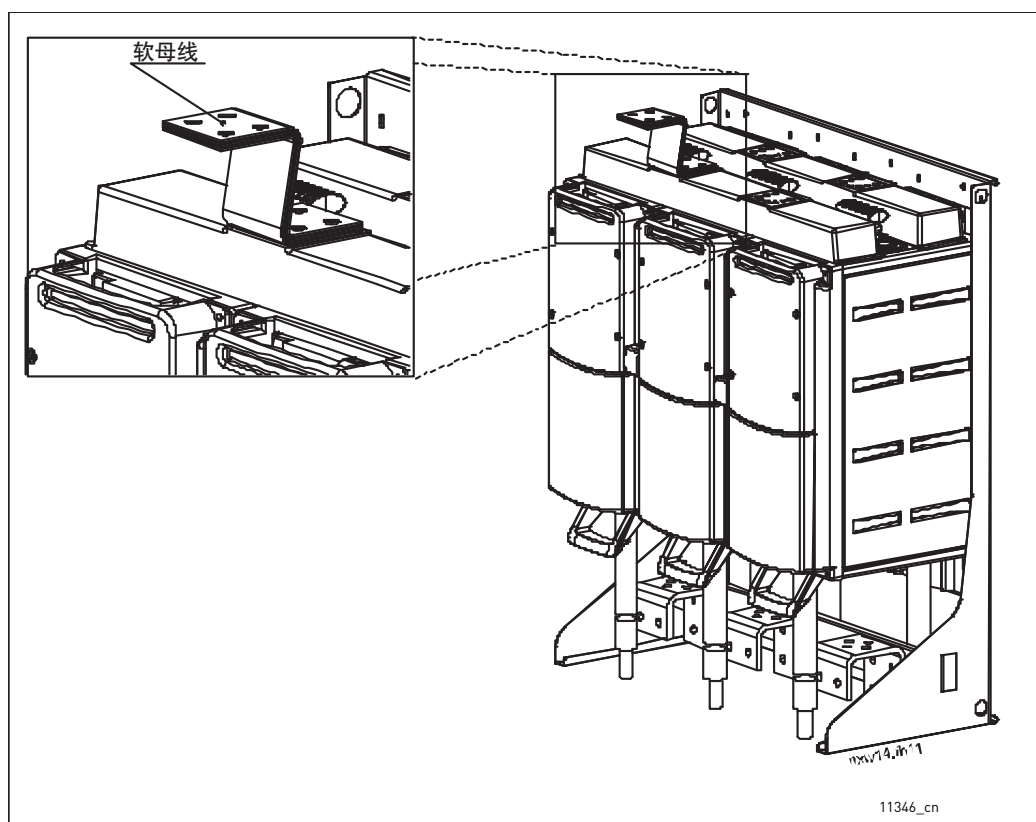
图 38. 柔性母线的安装
