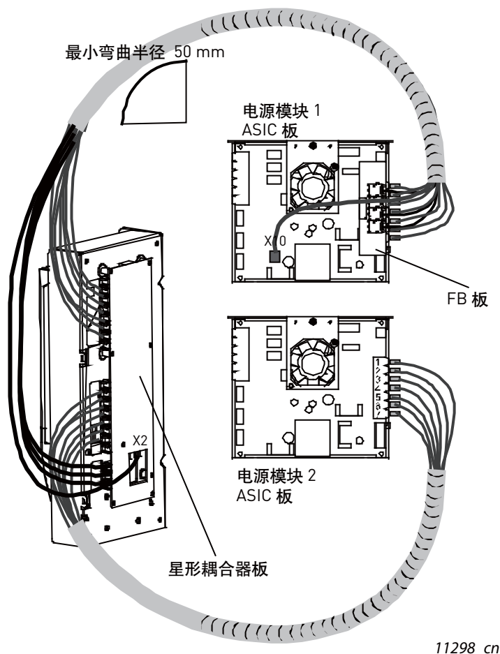
图 58. 将电源和控制电缆连接到控制单元， 2xCh64 和 2xCH74
