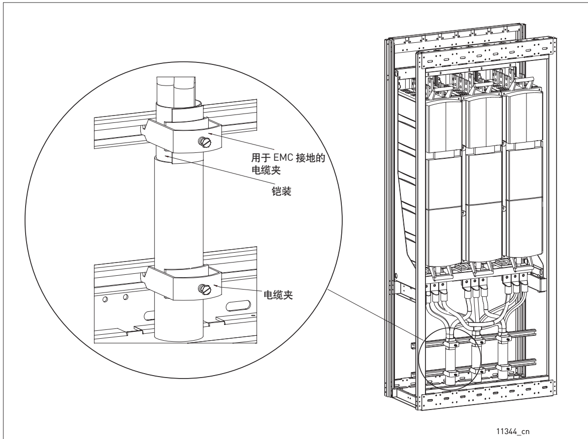
图 36. 将电机电缆夹到柜架上
