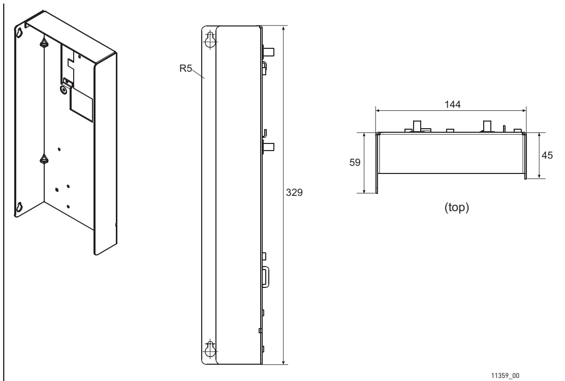
图 50. 控制单元安装盒尺寸
