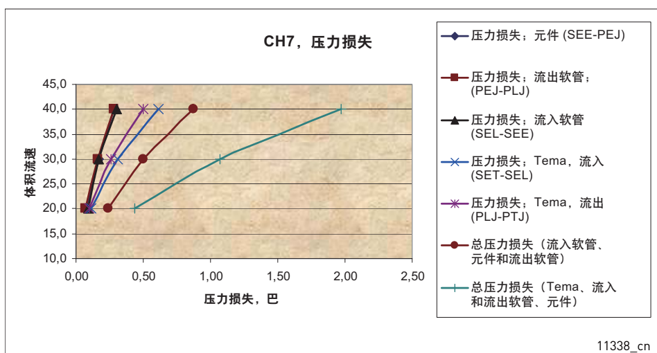
图 30. 压力损失，CH7x
