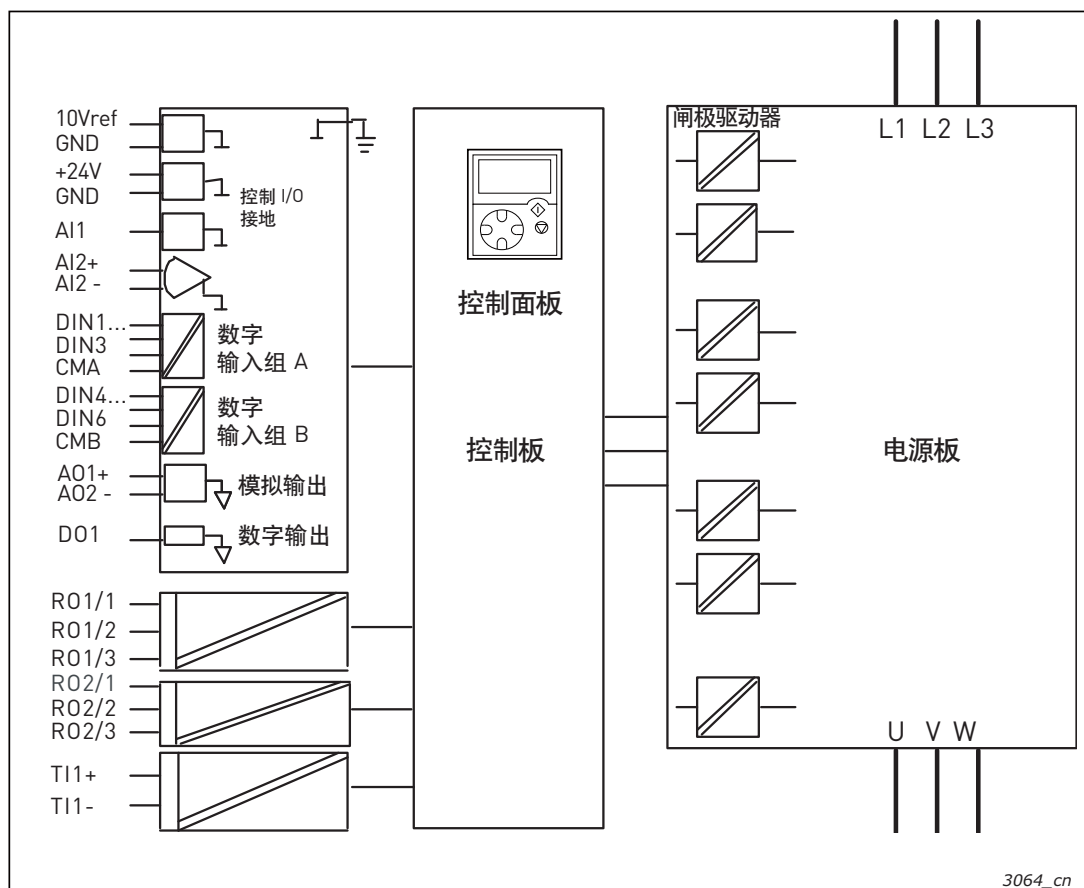
图 46. 电隔离
