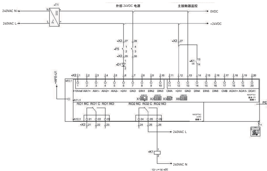
图 95. 控制单元接线图
