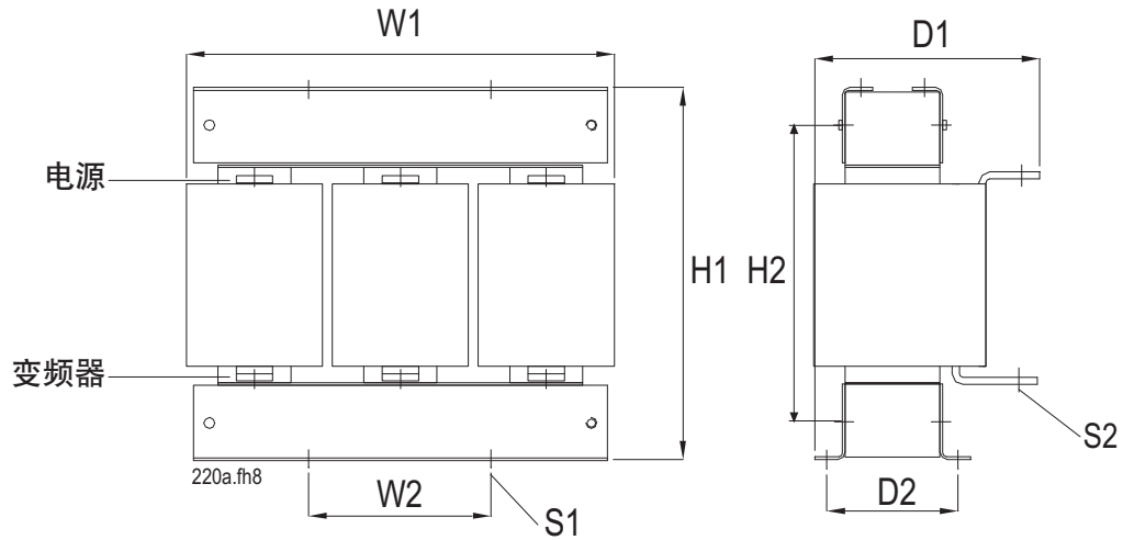
图 34. VACON® NX 水冷变频器的输入电抗器示例。尺寸 87 A...145 A 和 590 A
