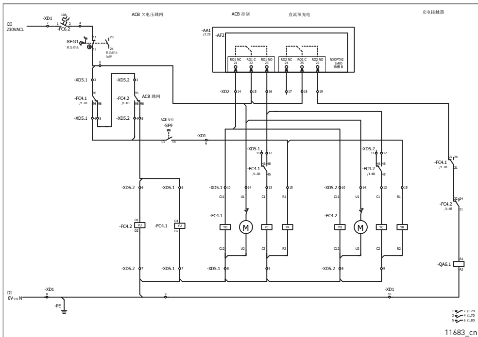
图 101. 控制接线图，OPTA2
