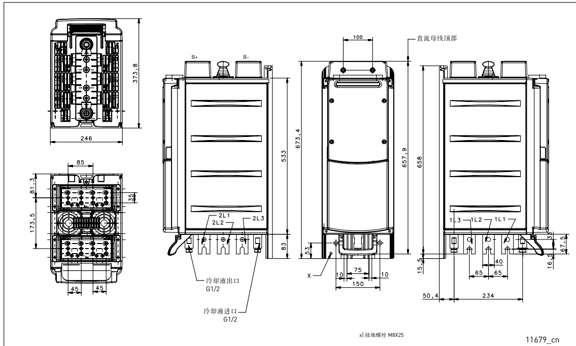
图 103. VACON® 水冷无回馈前端，CH60
