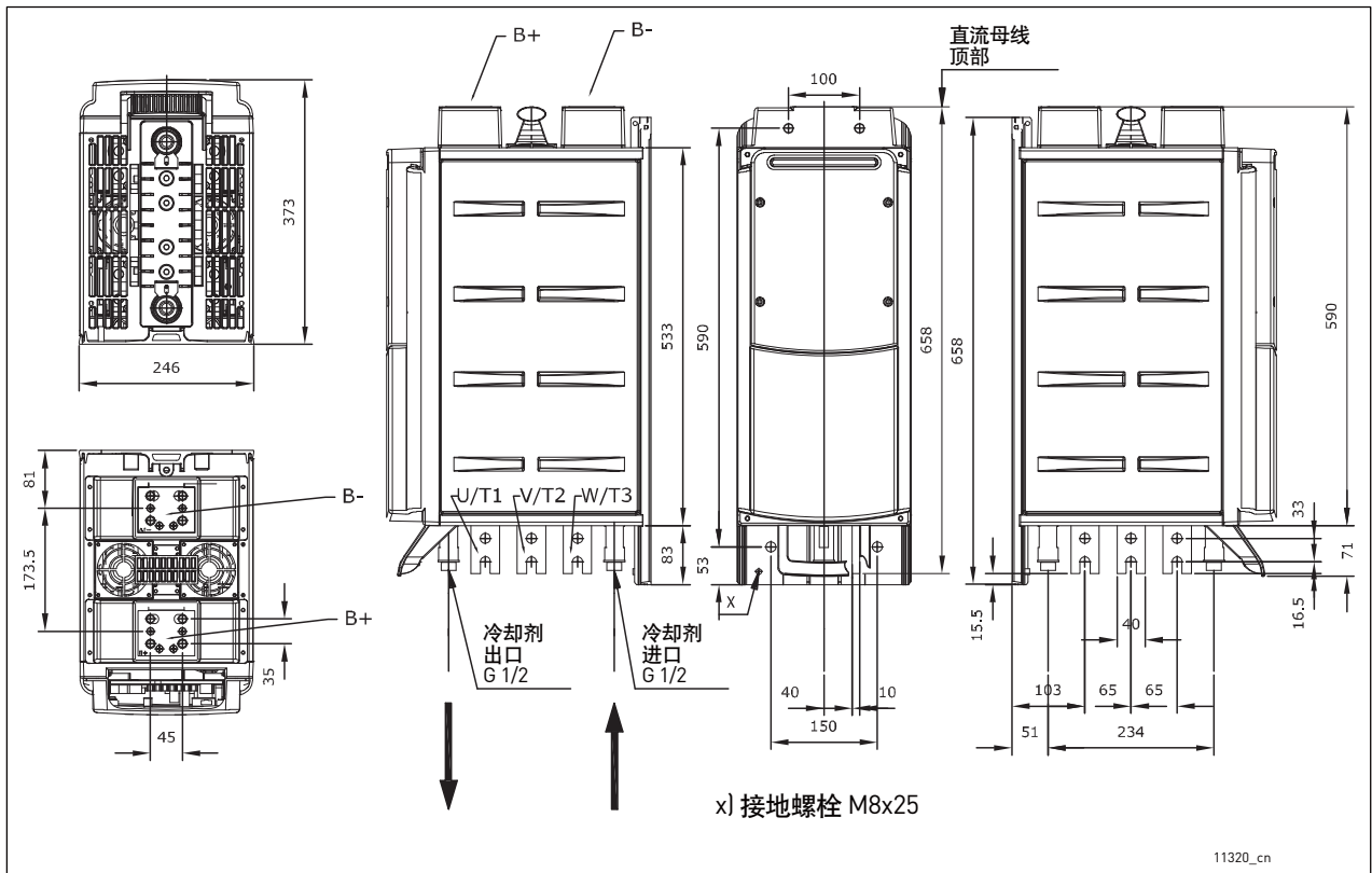
图 12. VACON® 水冷逆变器，CH61
