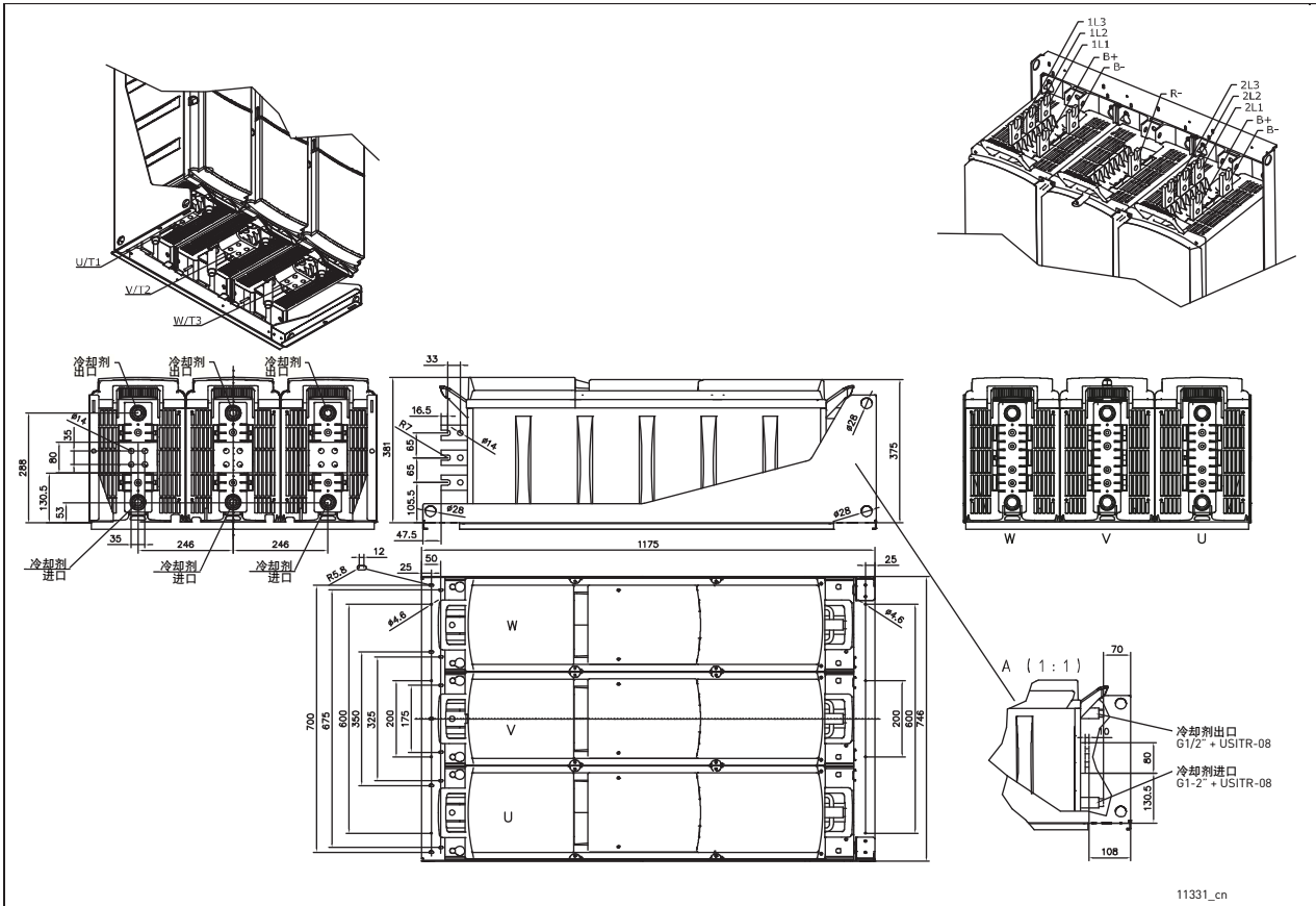
图 23. 带有内部制动斩波器的 VACON® NX 水冷交流变频器（12 脉冲）尺寸，CH74，IP00
