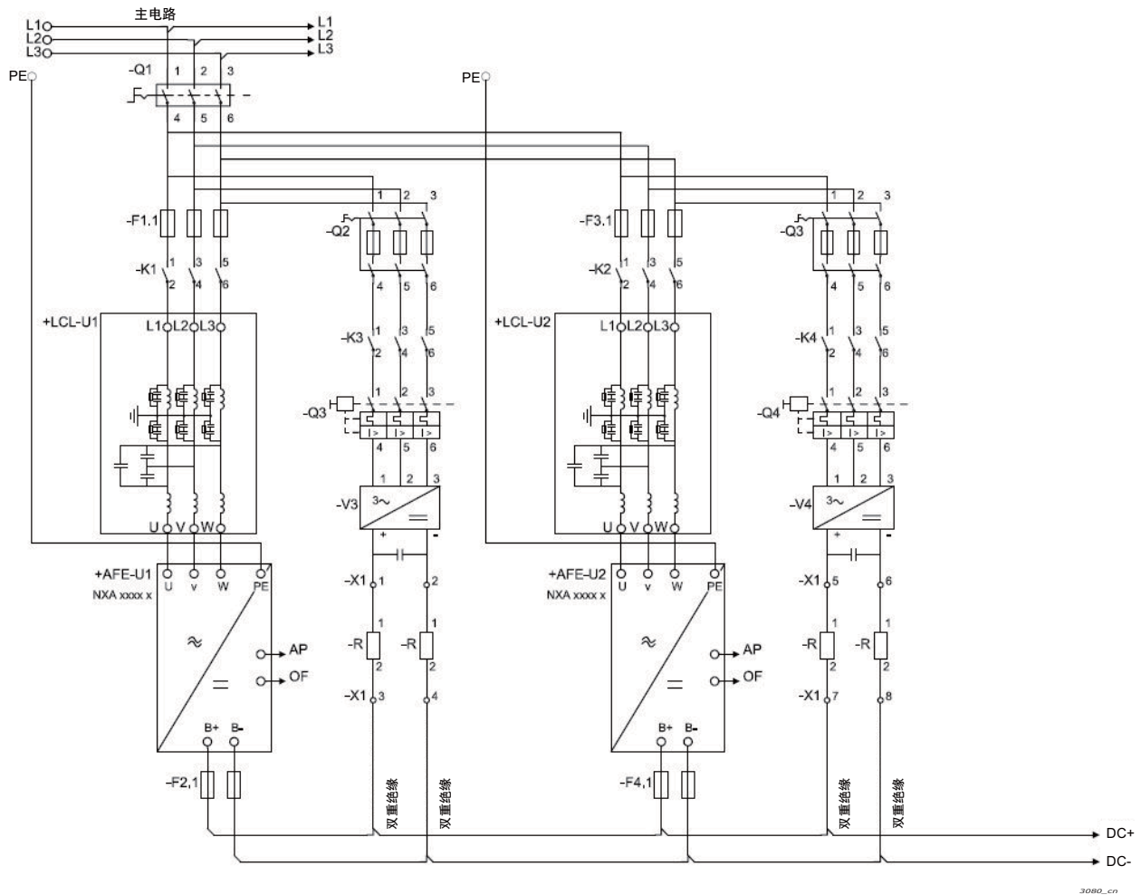
图 97. 有源前端单元并联，具有各自的预充电电路
