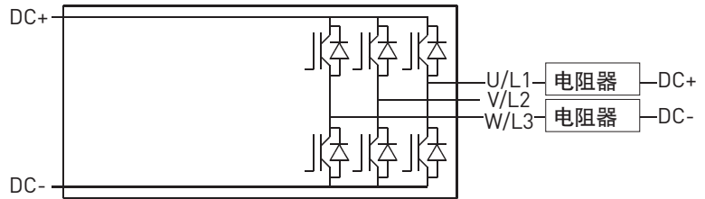
图 107. 制动斩波器单元拓扑
