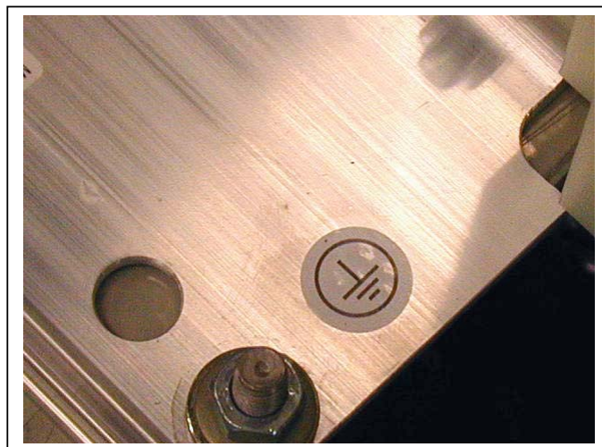
图 39. 安装板上的接地端子
