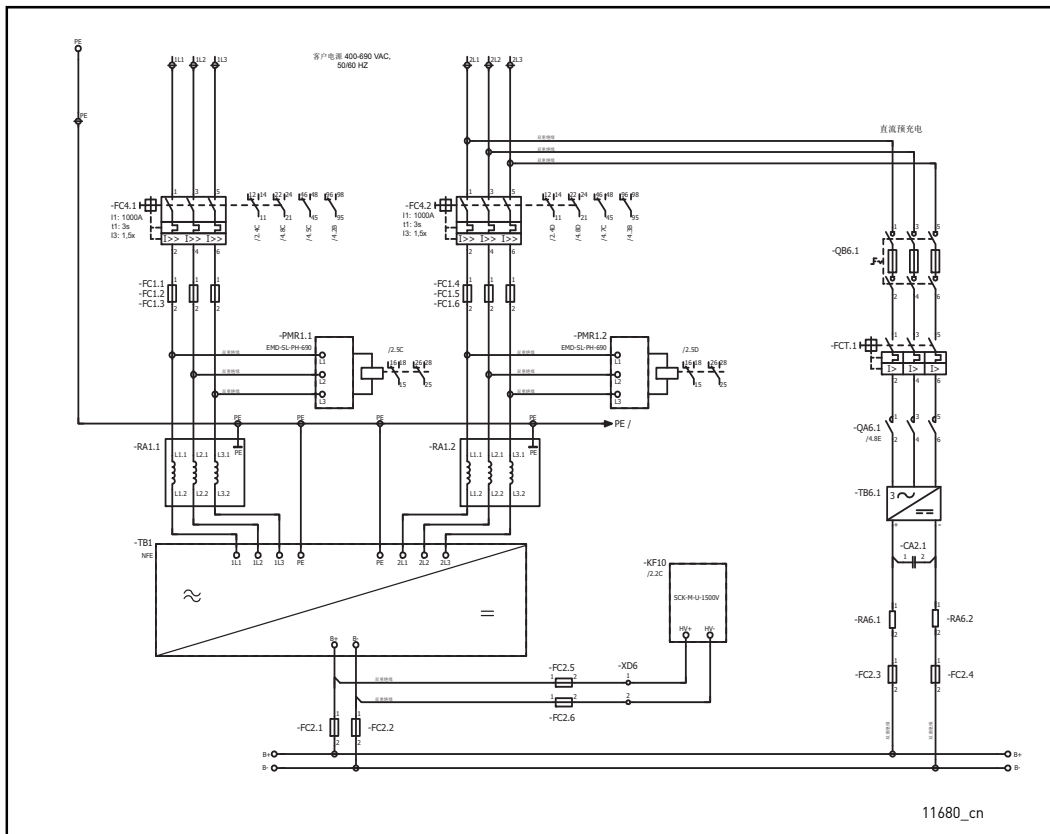
图 98. NFE 单元接线图
