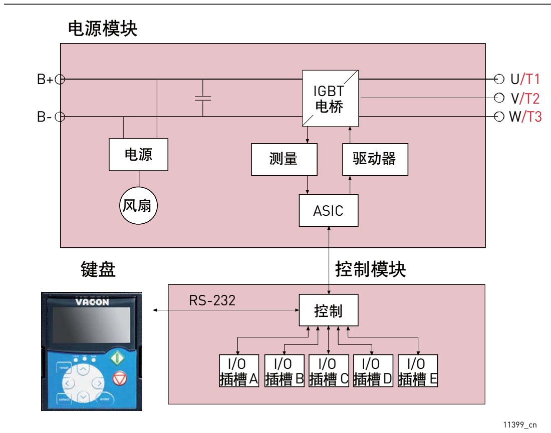
图 106. BCU 块示意图
