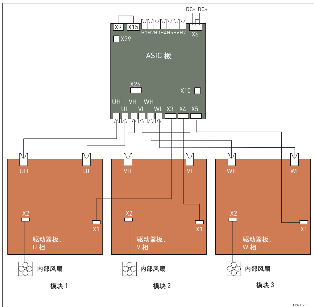
图 54.ASIC 和驱动板 ( CH64 和 CH74 ) 之间的端子和连接
