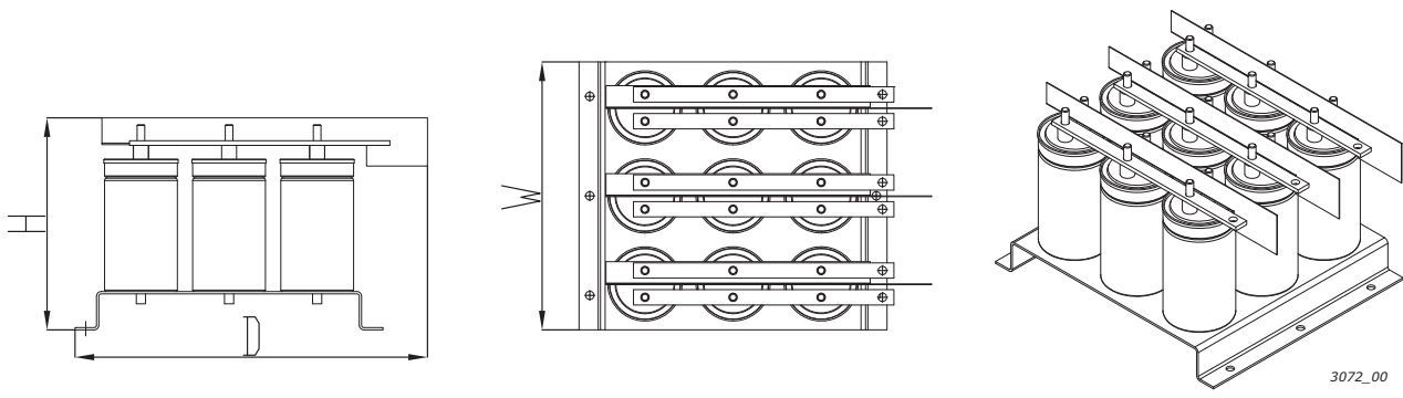
图 90. VACON® RLC 滤波器电容器组 ( C_{bank} ) 的示例
