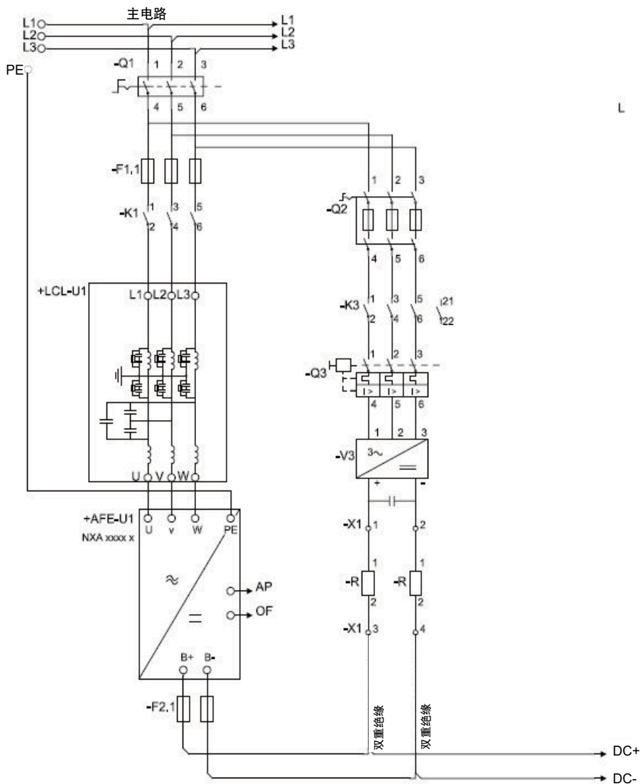
图 85. 有源前端配置
