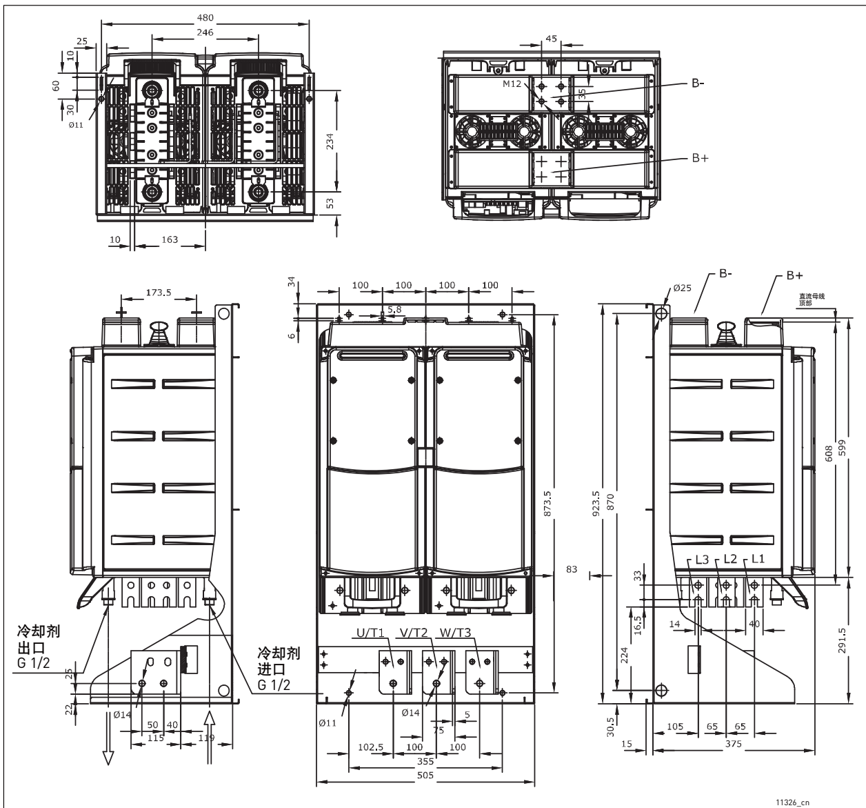
图 18. 带安装支架的 VACON® 水冷交流变频器，CH63
