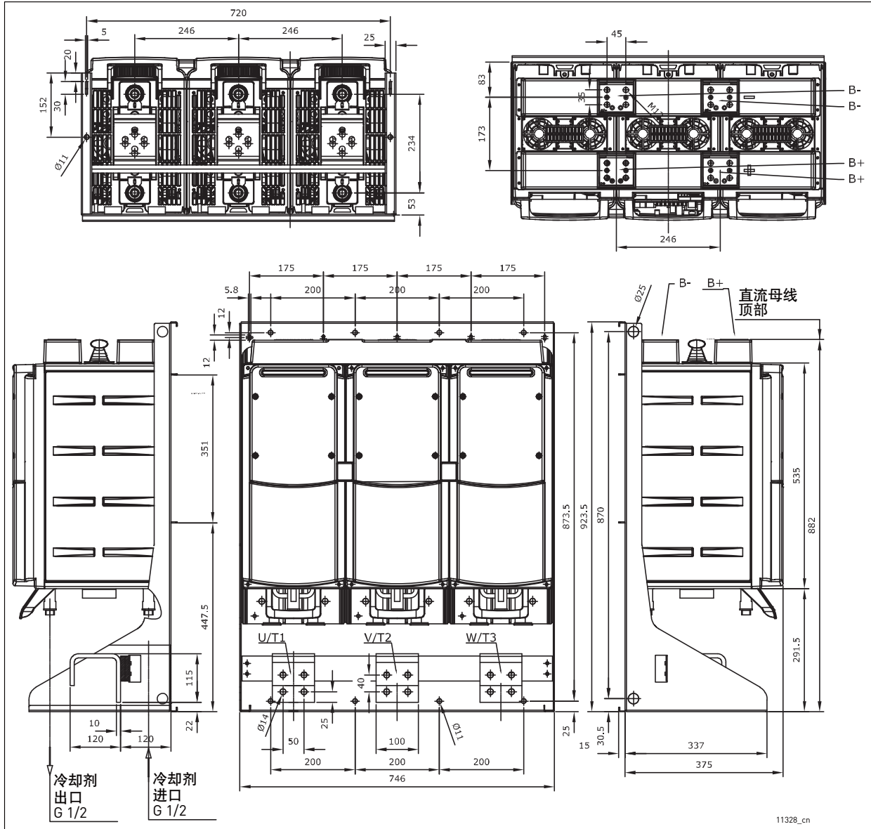
图 20. VACON ® NX 水冷逆变器尺寸，CH64，IP00
