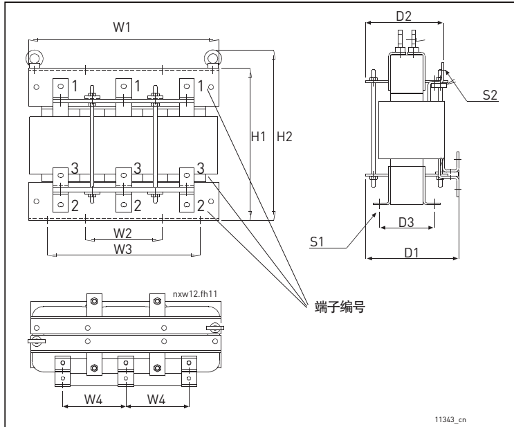
图 35. VACON® NX 水冷变频器的输入电抗器示例。尺寸 261 A...1150 A
