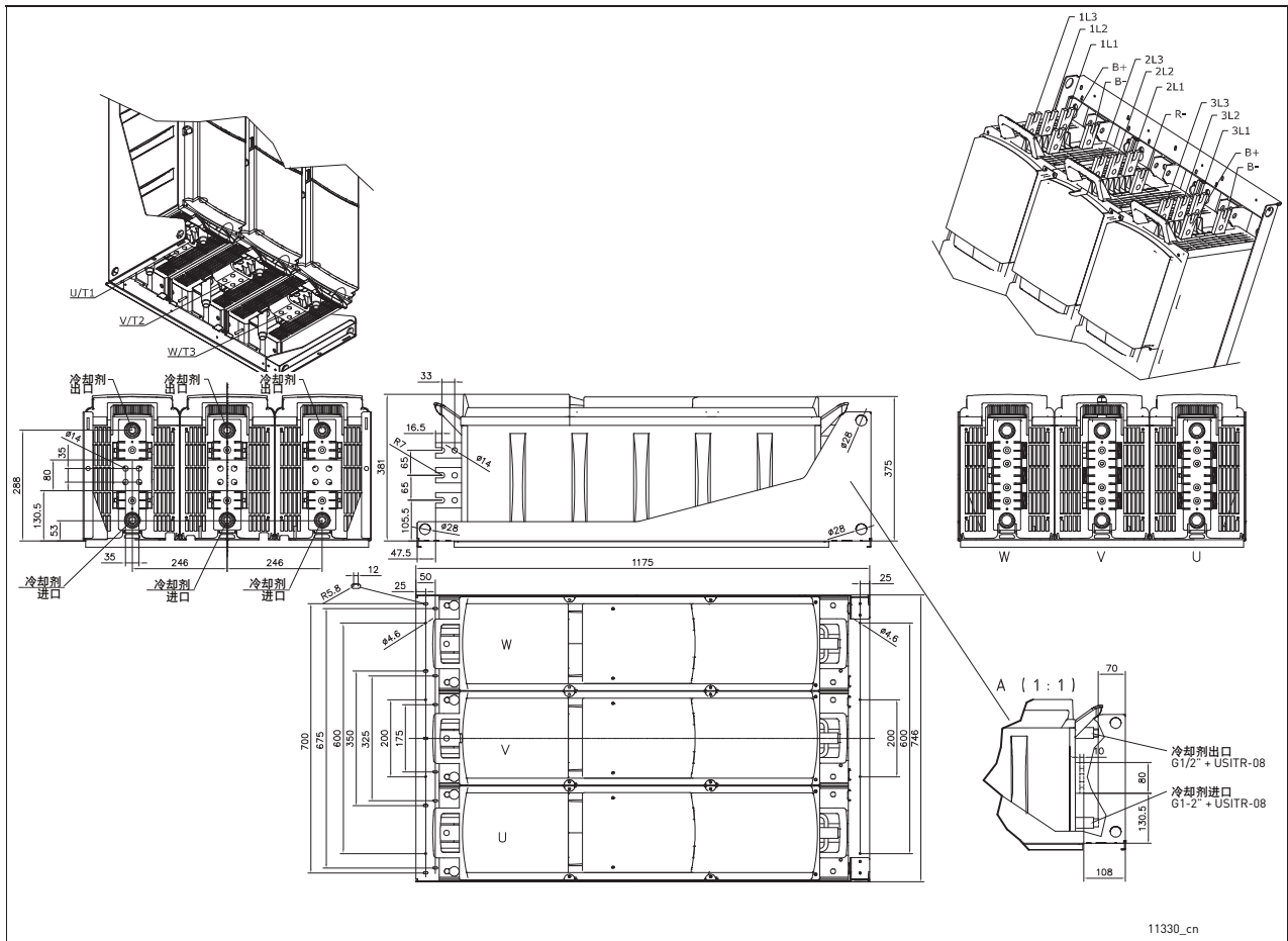
图 22. 带有内部制动斩波器的 VACON® NX 水冷交流变频器 ( 6 脉冲 ) 尺寸, CH74, IP00
