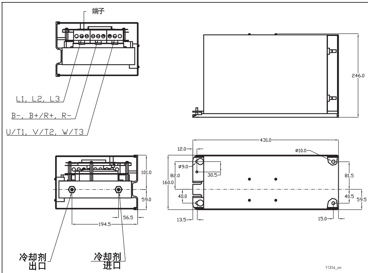
图 6. VACON® NX 水冷变频器尺寸, CH3
