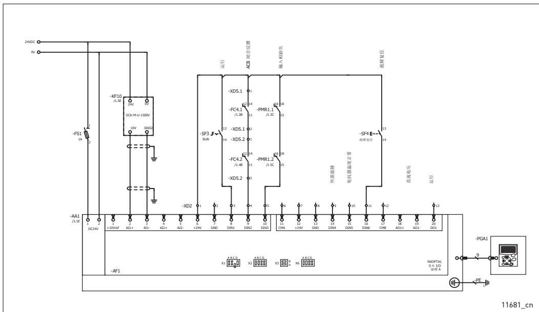
图 99. 控制接线图，OPTA1。
