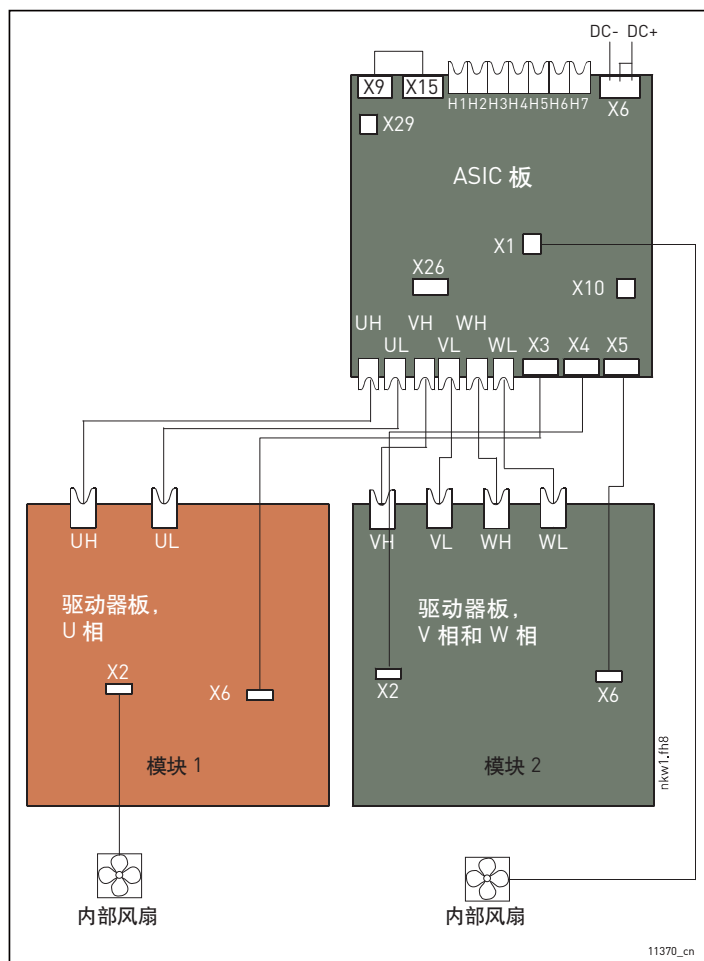
图 53. ASIC 和驱动板 (CH63) 之间的端子和连接
