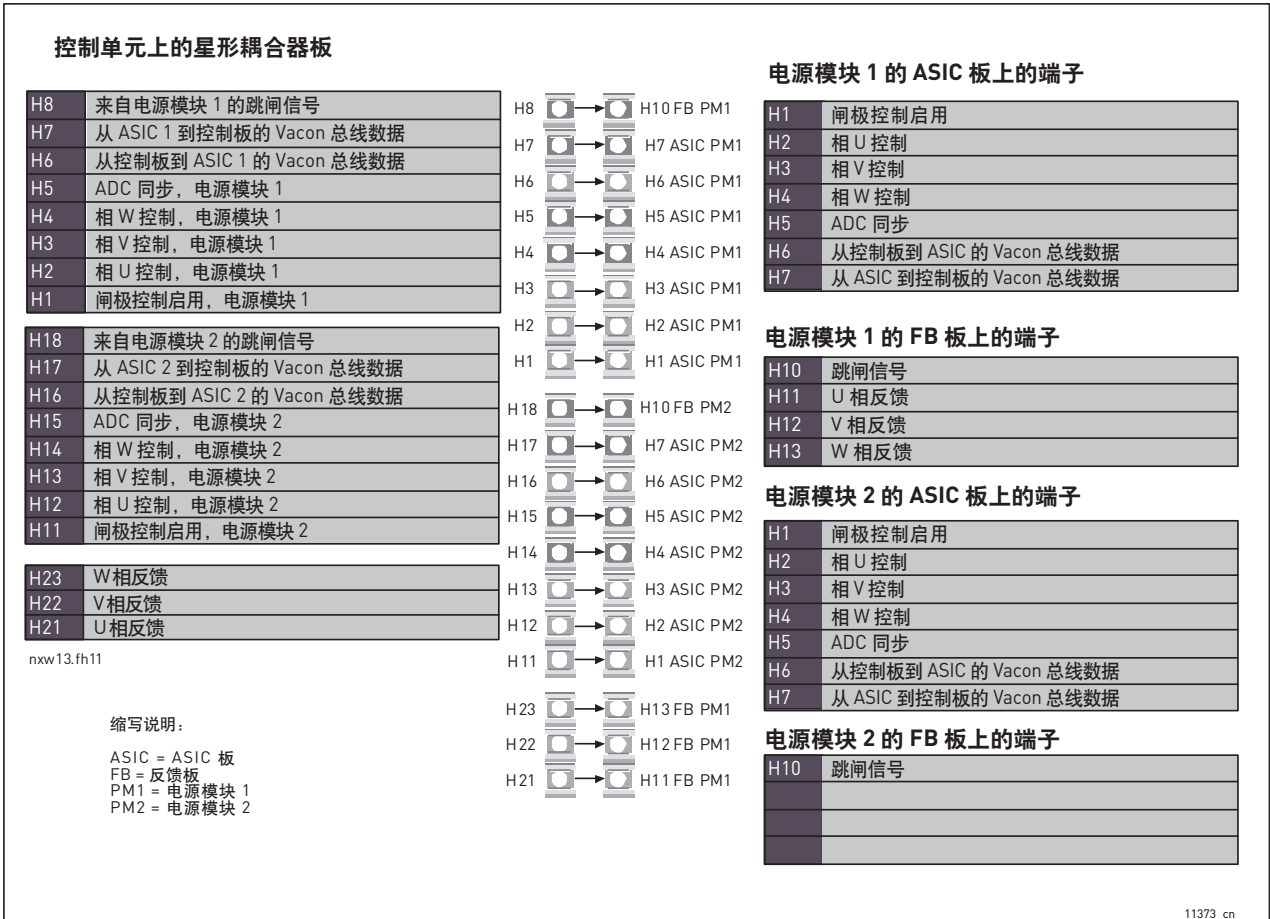
图 59. 星形耦合器板、ASIC 板和反馈板 (CH64 和 CH74) 之间的端子和连接
