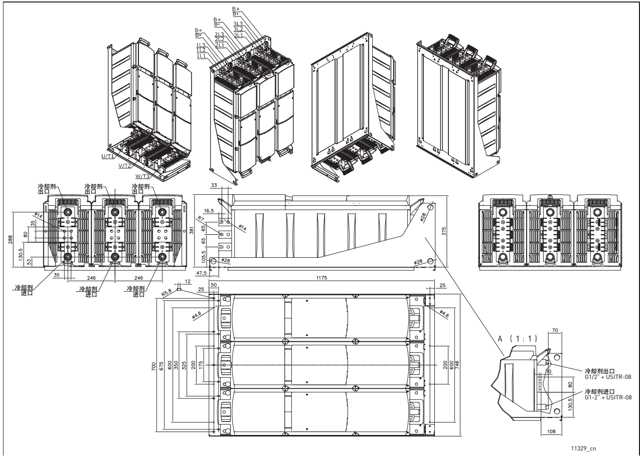
图 21. VACON® NX 水冷交流变频器（6 脉冲）尺寸，CH74，IP00
