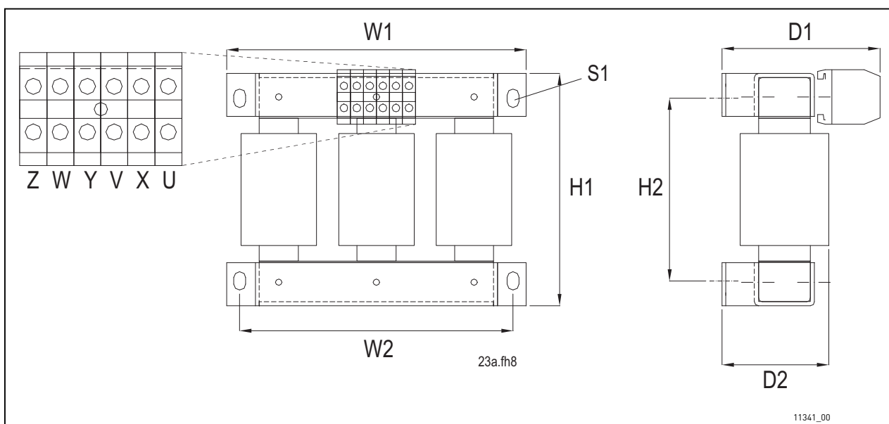
图 33. VACON® NX 水冷变频器的输入电抗器示例。最大尺寸 62 A
