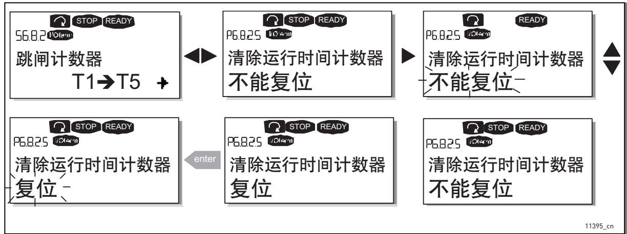
图 81. 计数器重置
