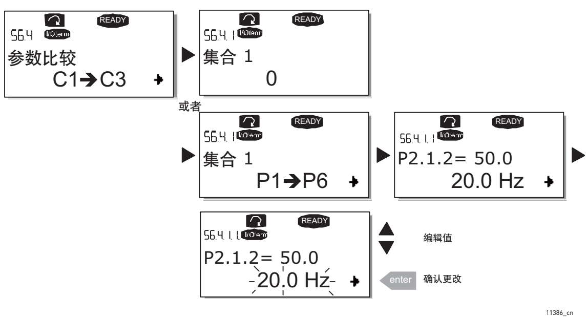
图 72. 参数比较
