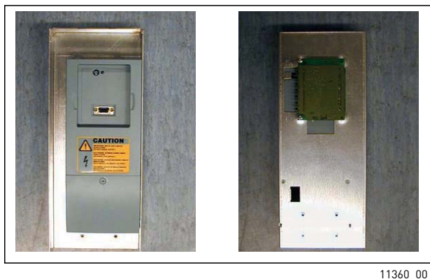
图 51. 安装在安装盒内的控制单元；左：正面；右：背面
