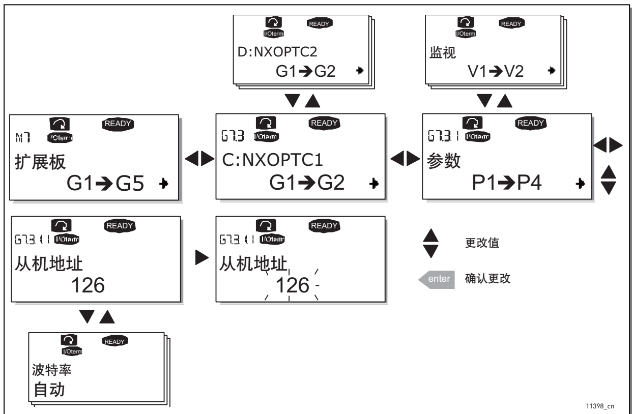
图 84. 扩展板信息菜单
