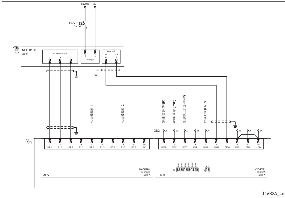
图 100. 控制接线图，OPTBH，OPTB1
