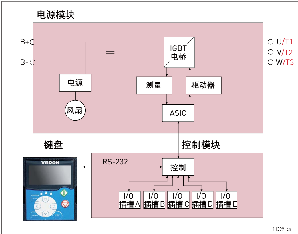
图 86. 有源前端模块示意图
