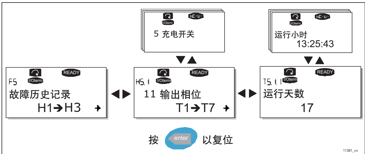
图 67. 故障历史记录菜单
