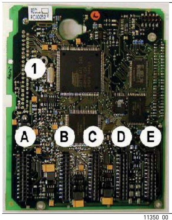
图 41. VACON® NX 控制板
