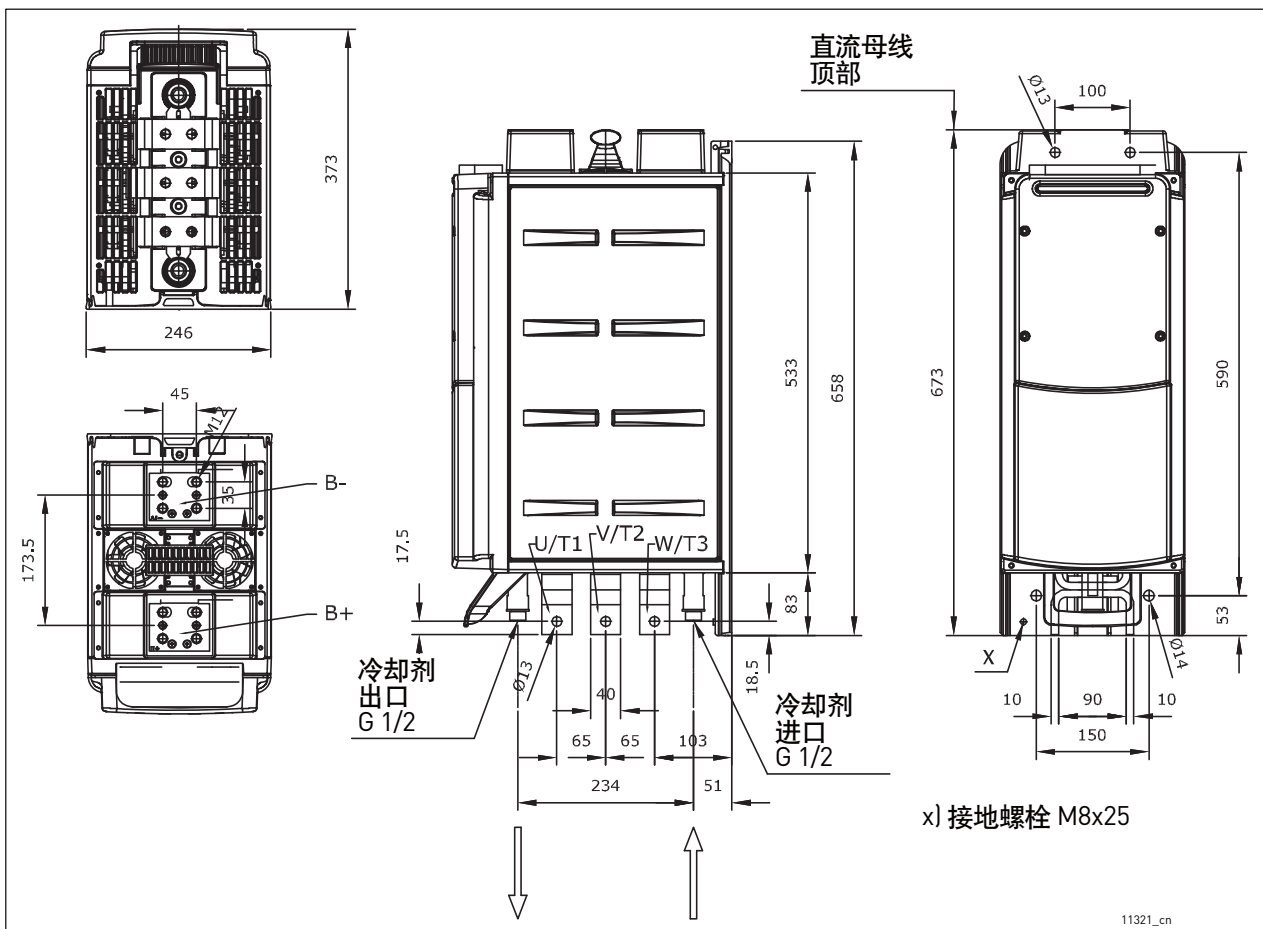
图 13. VACON® 水冷逆变器，CH62
