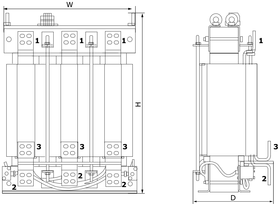
图 105. FLU-CHK-1030-6-DL 电抗器示例
