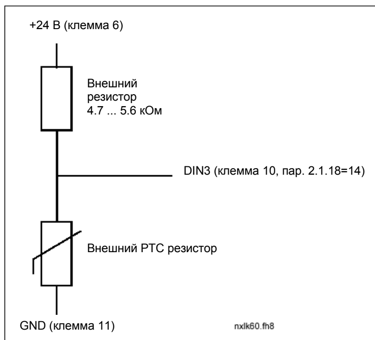
Рис. 6-27. Подключение термистора двигателя PTC
