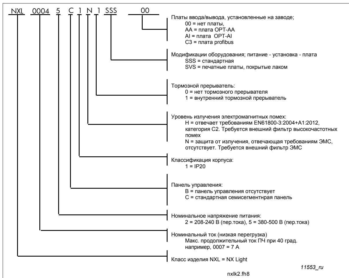
Рис. 3-1. Расшифровка кода условного обозначения Vacon NXL для типоразмеров MF2 и MF3
