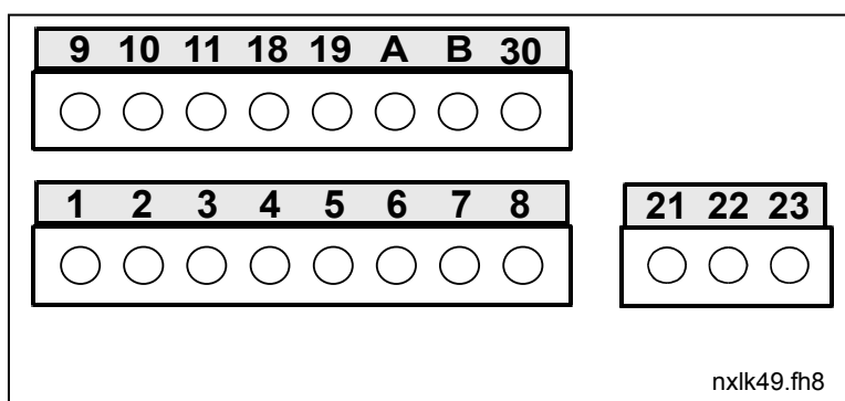
Рис. 6-22. Клеммы управления, MF4 – MF6
