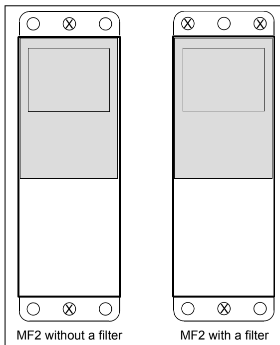
Рис. 5-2. Установка преобразователя NXL, MF2
