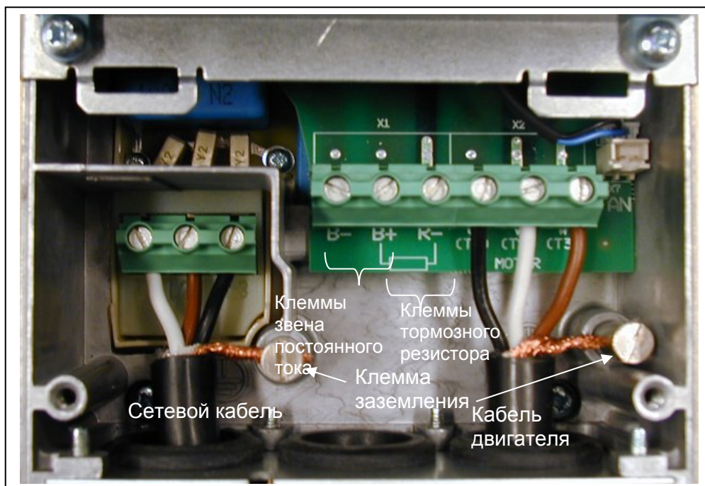
Рис. 6-14. Подключение кабелей в Vacon NXL, MF4
