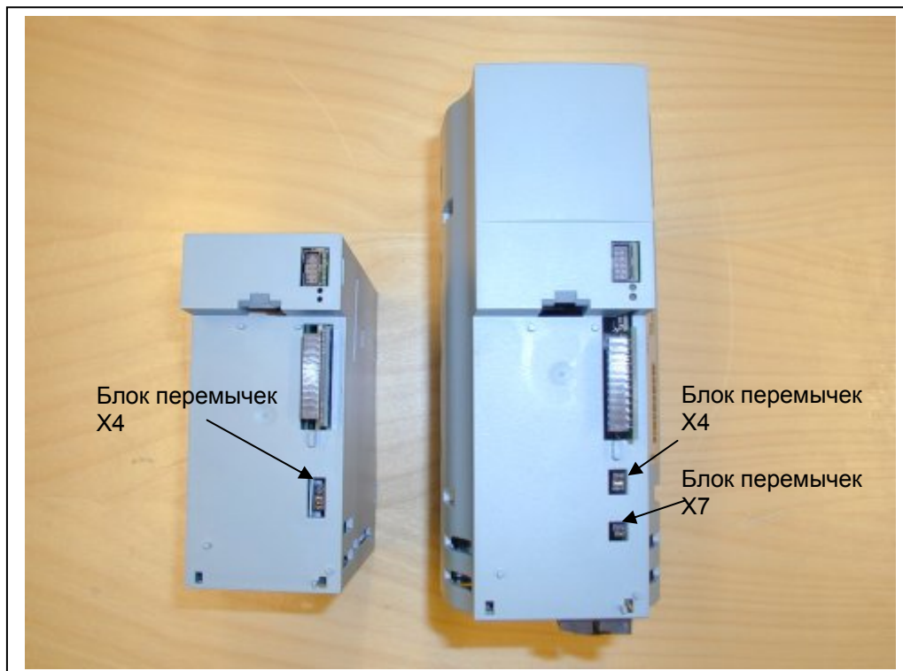
Рис. 6-25. Расположение блоков переключателей в MF2 (слева) и MF3 (справа)
