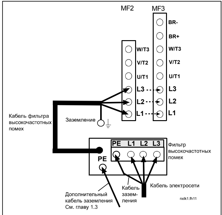
Рис. 6-11. Подключение кабелей при установке фильтра радиочастотных помех в Vacon NXL
