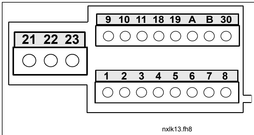
Рис. 6-21. Клеммы управления, MF2 – MF3
