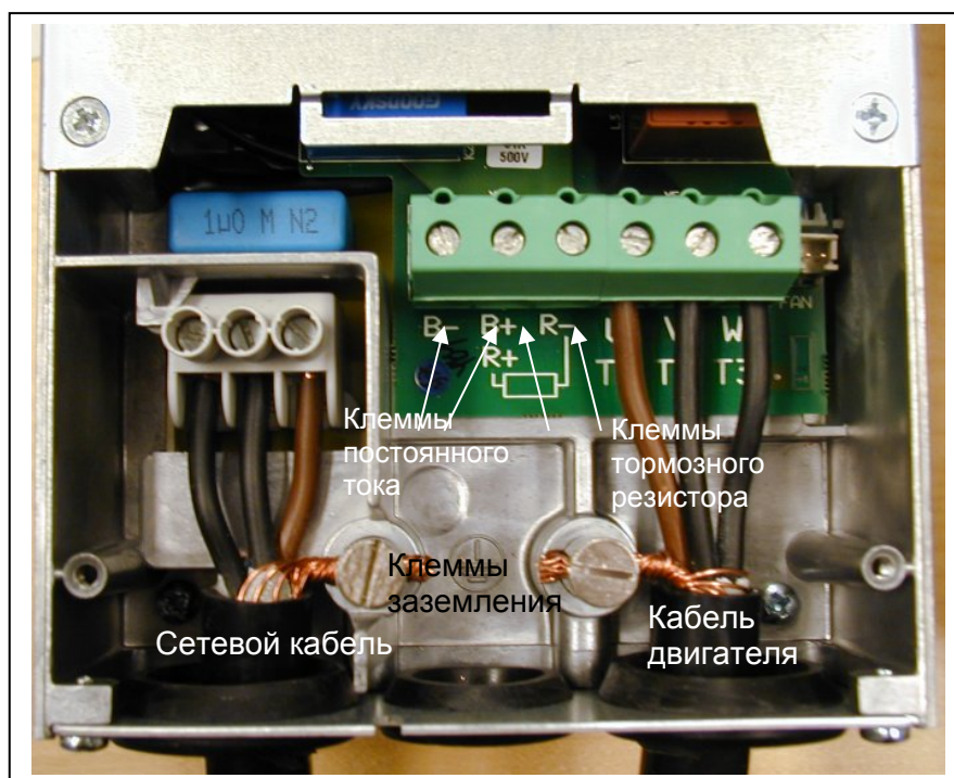
Рис. 6-17. Подключение кабелей в Vacon NXL, MF5
