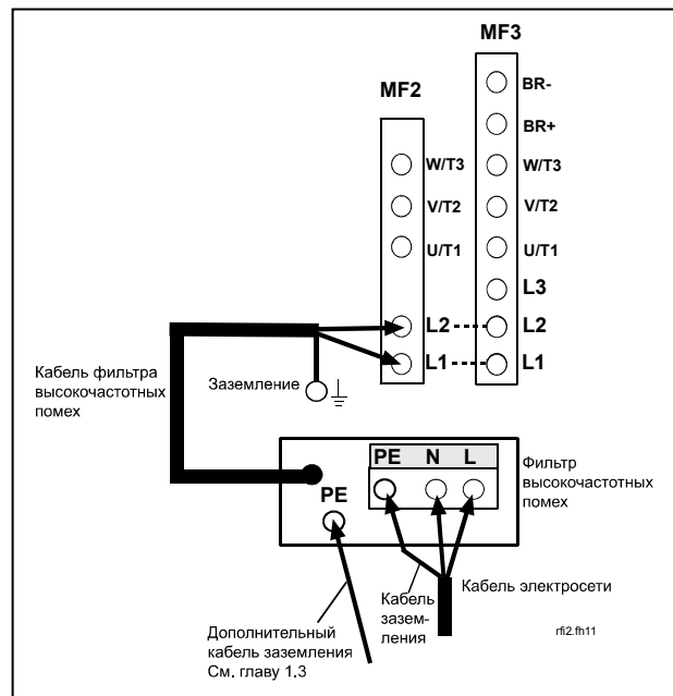
Рис. 6-12. Подключение кабеля фильтра радиопомех в MF2 и MF3, 208...240V, 1-фазное напряжение. Фильтр типа RFI-0013-2-1
