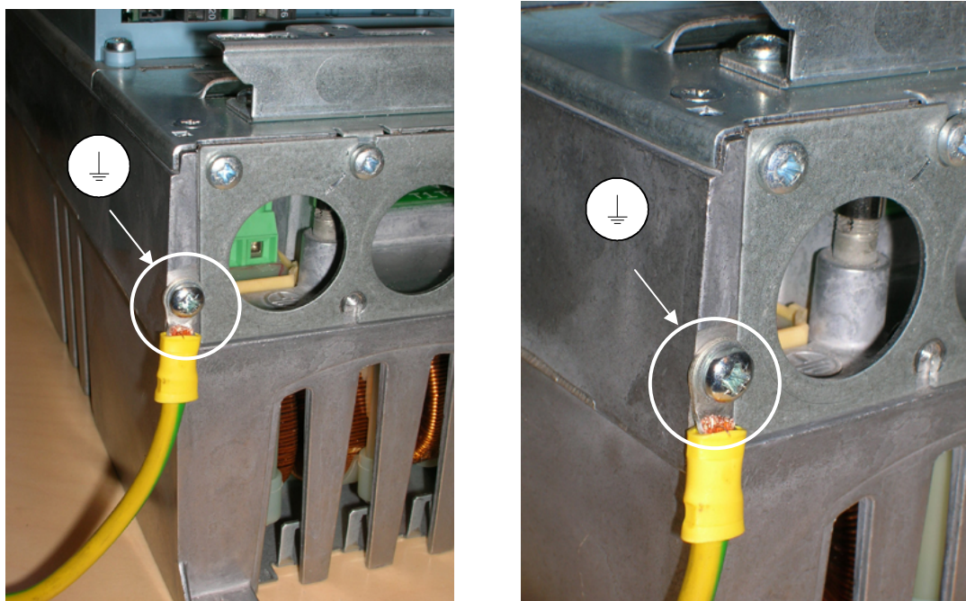
Рис. 6-15. Подключение дополнительного кабеля заземления, MF4. См. главу 1.3
