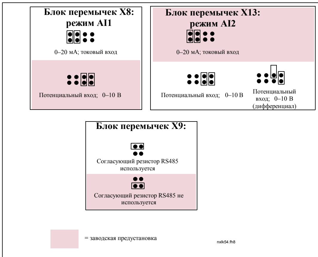
Рис. 6-24. Положения перемычек для Vacon NXL, MF4 – MF6
