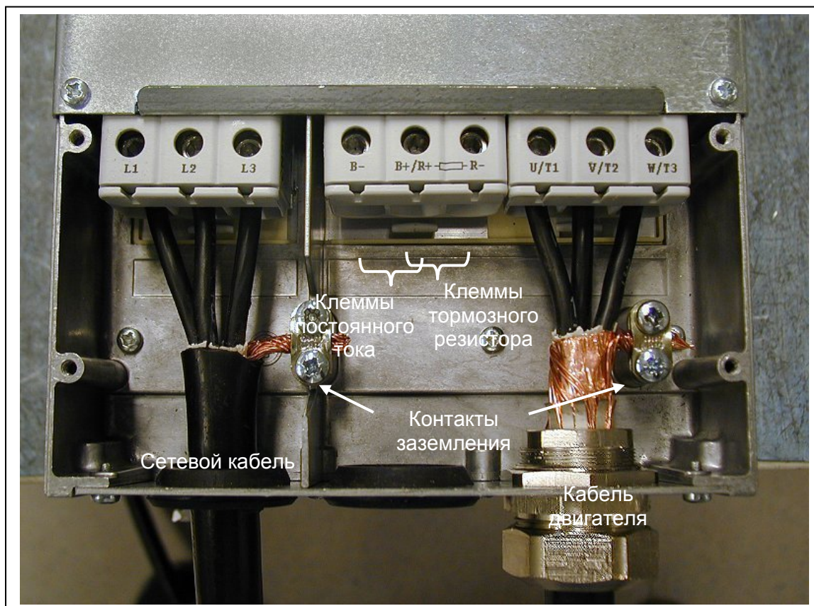
Рис. 6-19. Подключение кабелей в Vacon NXL, MF6
