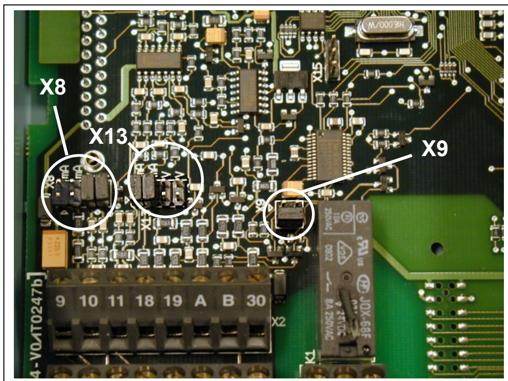
Рис. 6-26. Расположение блоков переключателей в плате управления MF4 – MF6
