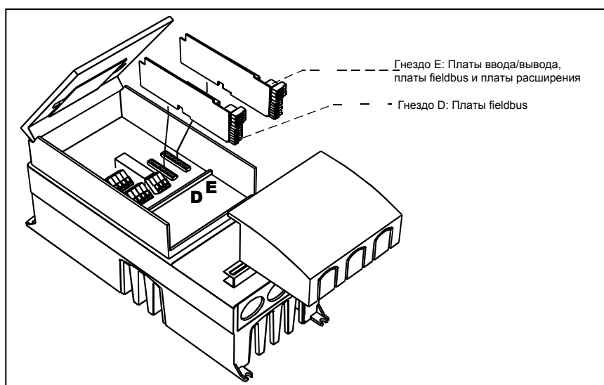
Рис. 6-20. Дополнительные гнезда разъемов плат D и E в блоках MF4 – MF6
