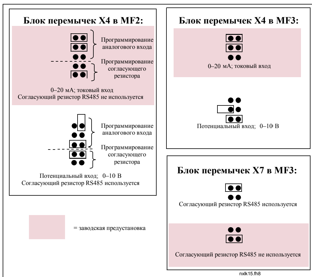
Рис. 6-23. Положения перемычек для Vacon NXL, MF2 и MF3
