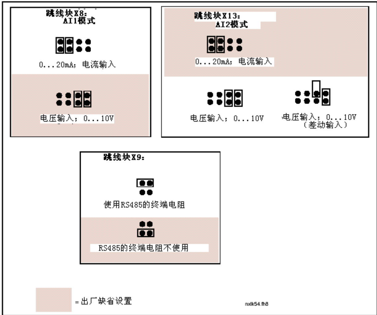
图 6-24. Vacon NXL 变频器的跳线选择, MF4-MF6
