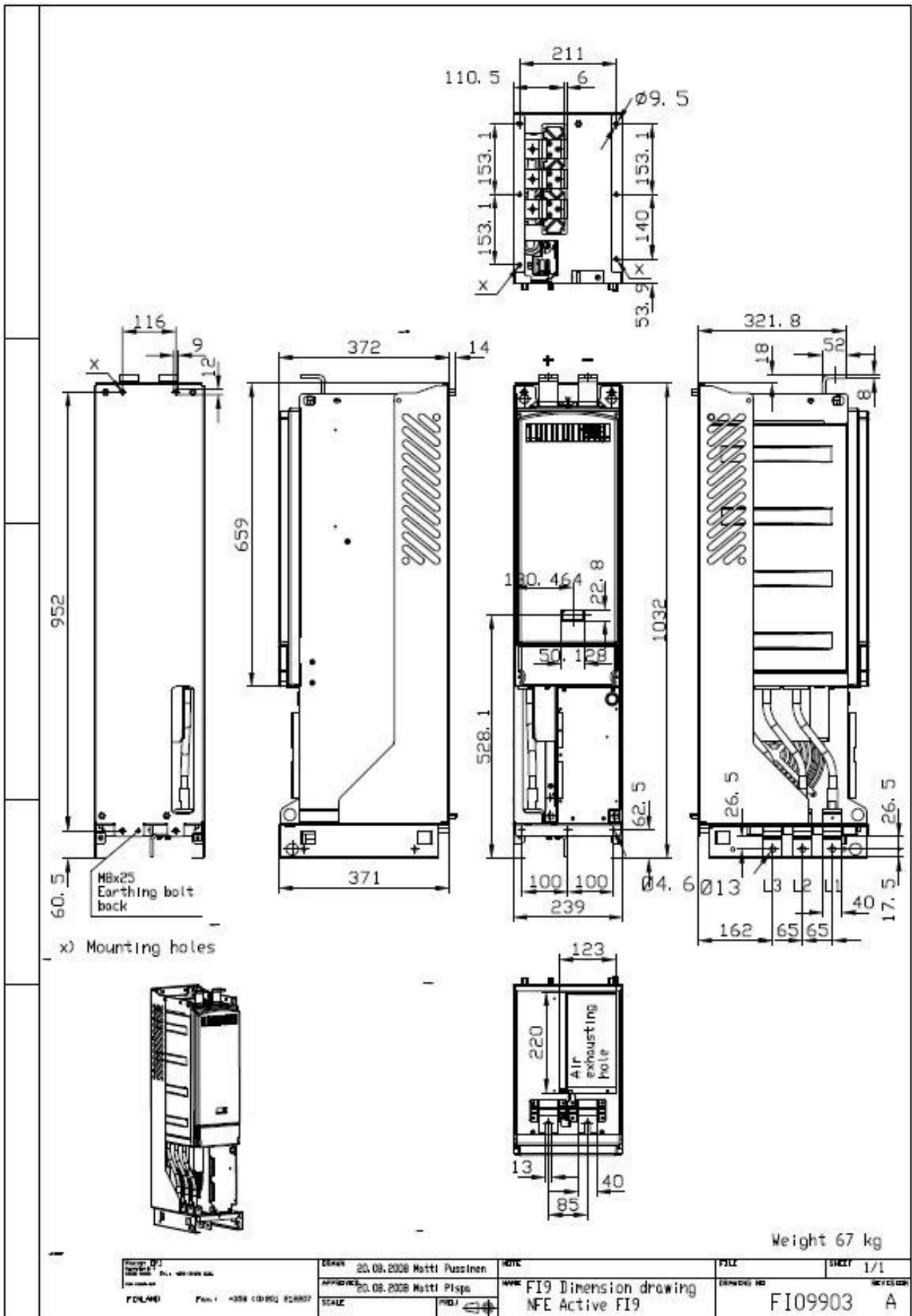
Appendix 7-4. F19 Dimensions
