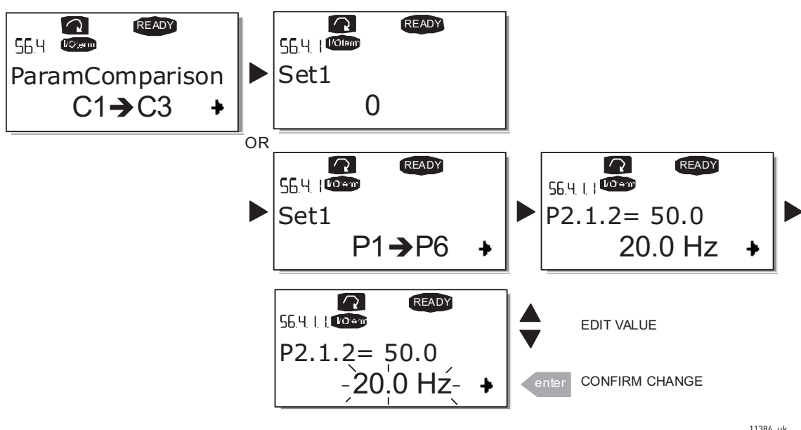
Figure 72. Parameter comparison
