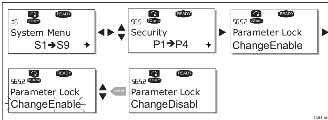
Figure 74. Parameter locking
