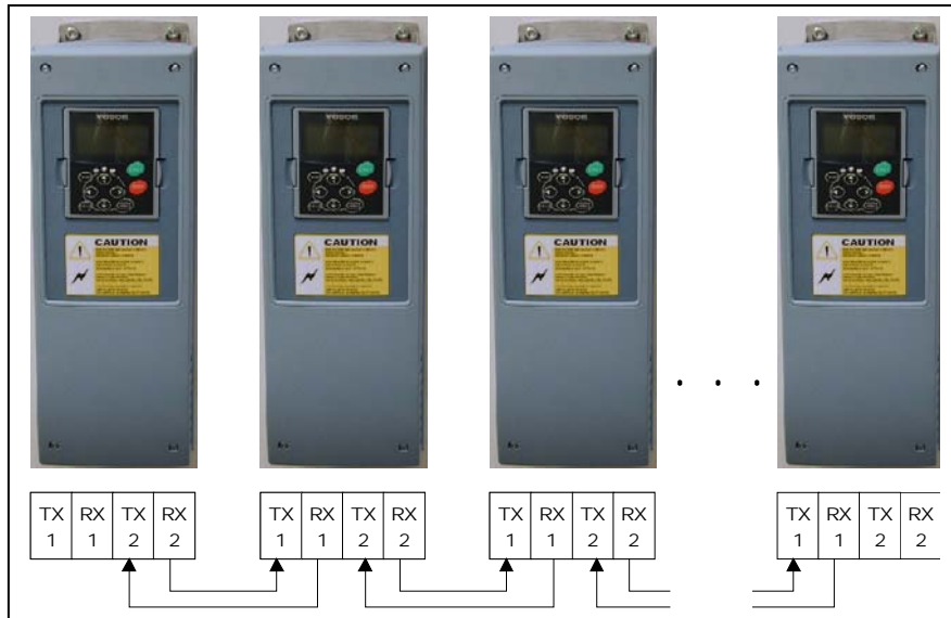
图7-4. 系统总线与NXOPTD1 板物理连接
