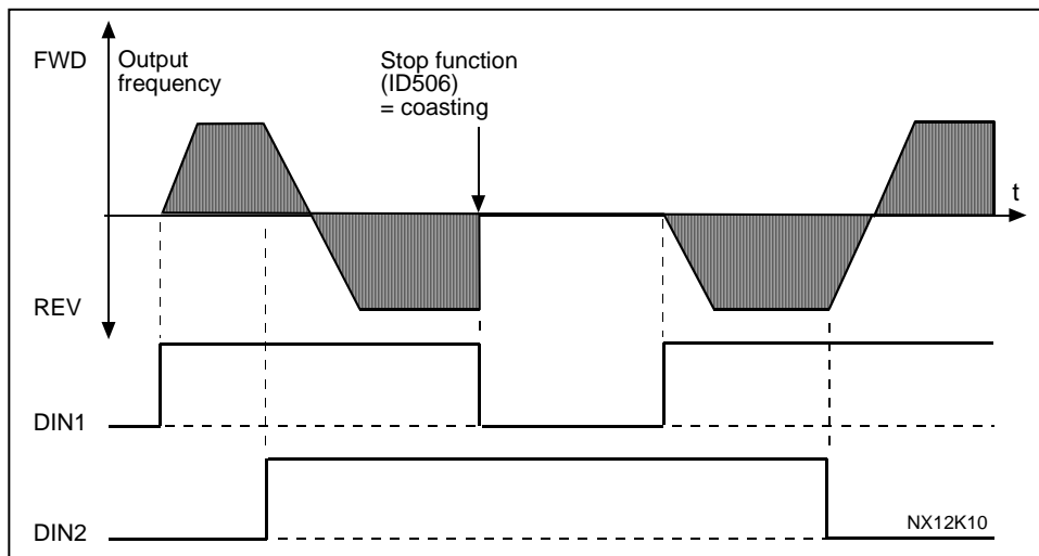
图6-4. 启动、停车、反向
