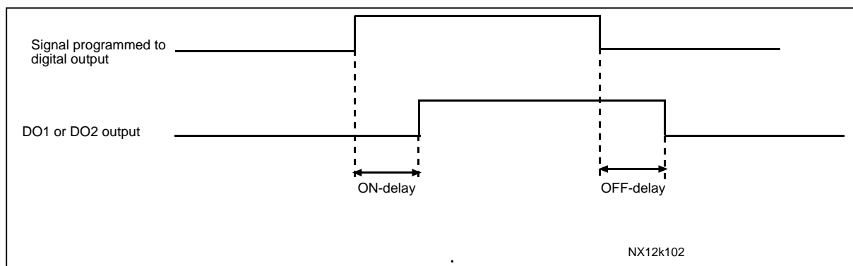
图6-21. 数字输出信号 1 和数字输出信号 2，接通/断开延时
