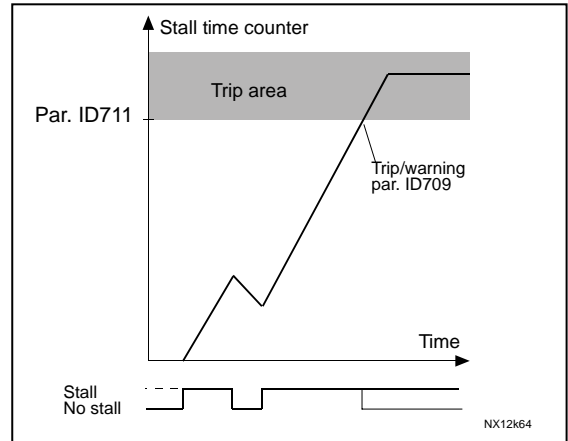
图6-32. 失速时间计时
