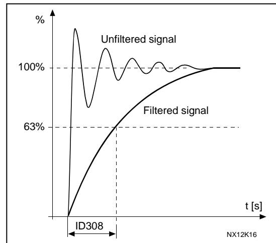
图 6-7. 模拟输出信号滤波
