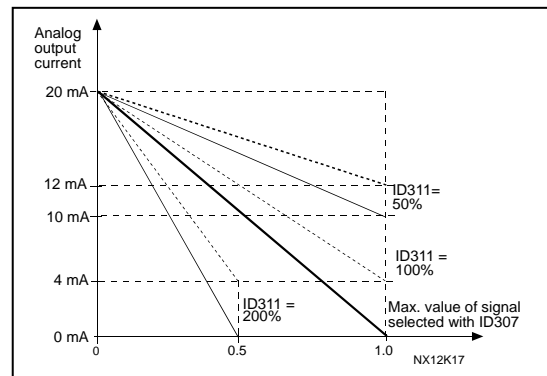
图 6-8. 模拟输出信号倒置
