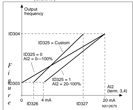
图6-12. 模拟输入 2 比例
