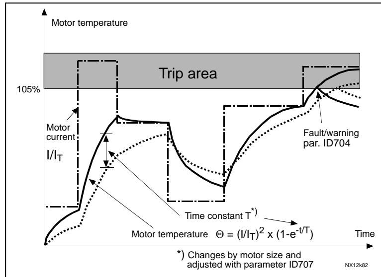
图6-30. 电机温度计算
