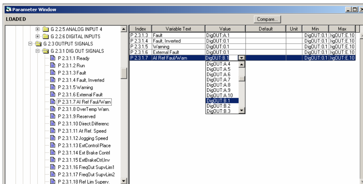
图 4-1. NCDrive 程序设计工具：输入地址编码
