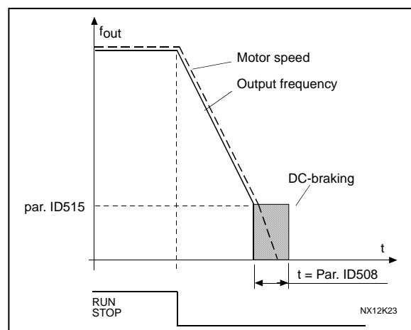
图6-25. 斜坡制动模式下的直流制动时间
