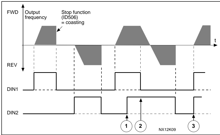
图6-3. 正向启动/反向启动
