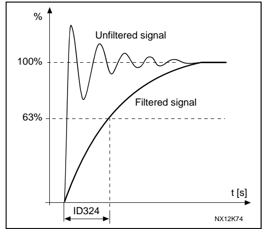
图6-11. 模拟输入信号 1 信号滤波
