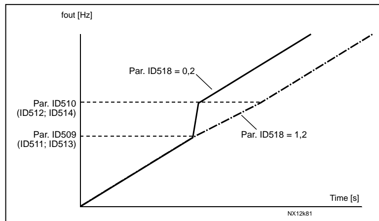
图6-27. 禁止频率限制范围之间的斜坡速度比例
