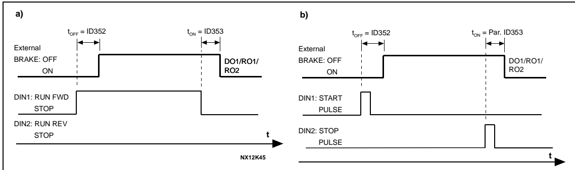
图6-13. 外部制动控制:
