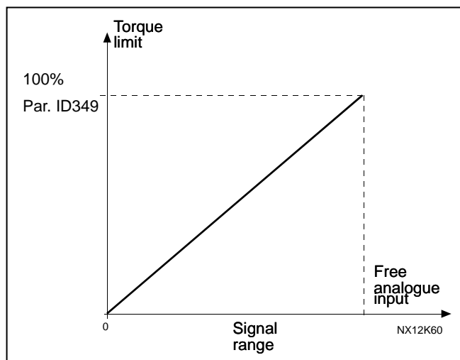
图 6-20. 降低转矩监视限制
