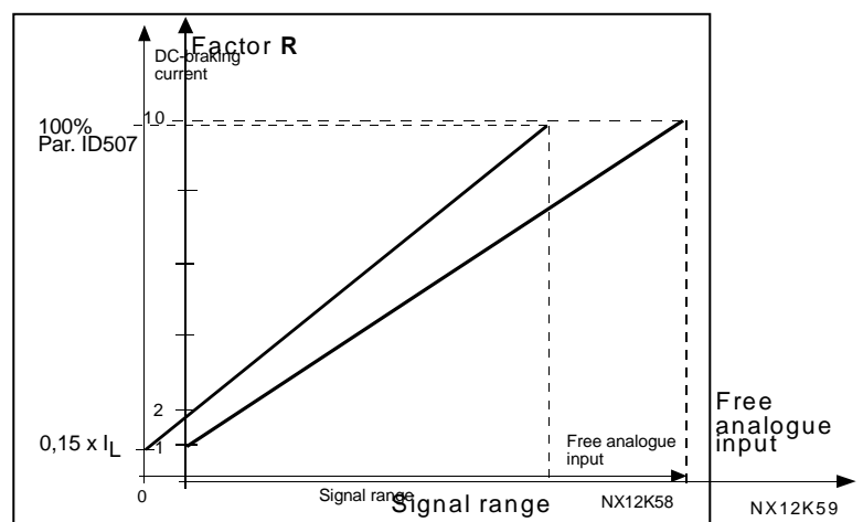
图 6-18. 直流制动电流比例
