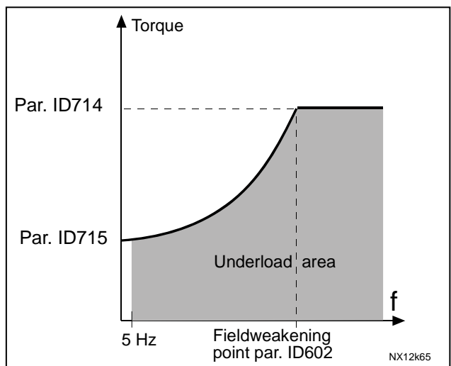
图6-33. 最小负载设置
