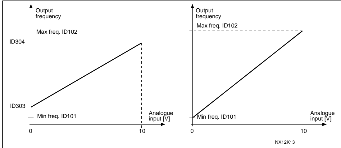
图6-6. 左: 参考值有定标; 右: 没有比例(参数 ID303 = 0)。
