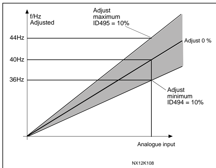
图6-22. 输入调整例子
