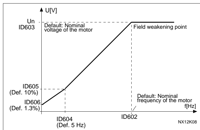
图6-2. 可设计的U/f曲线
