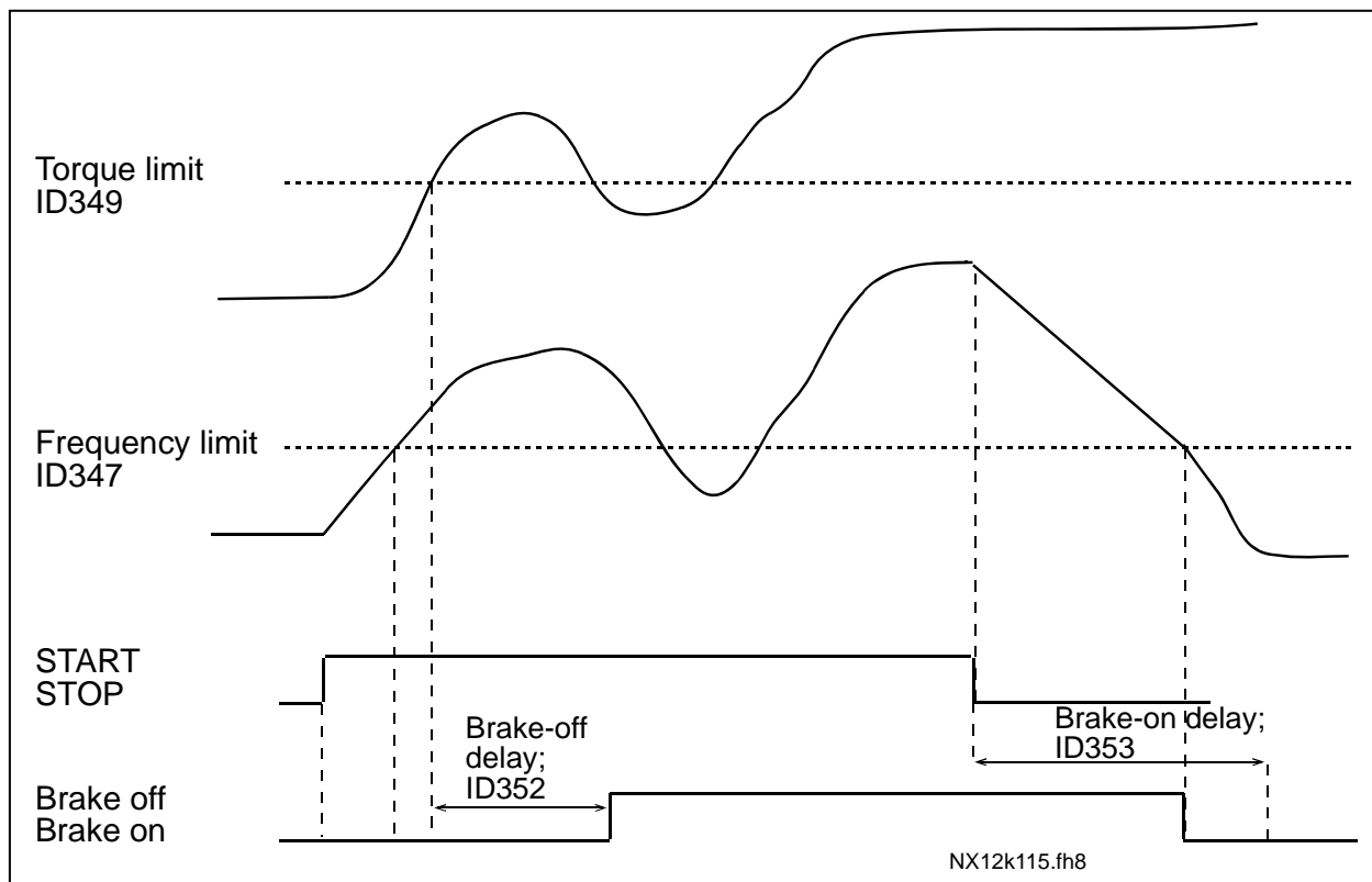
图7-1. 制动控制附加限制
