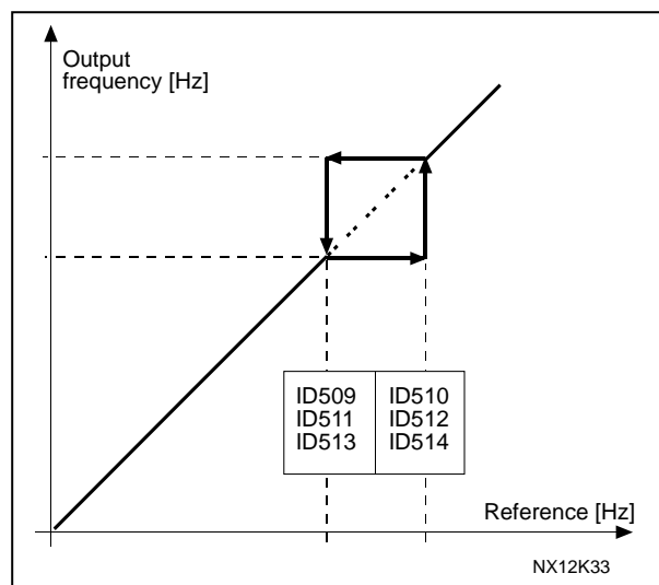
图6-26. 禁止频率范围设置例子
