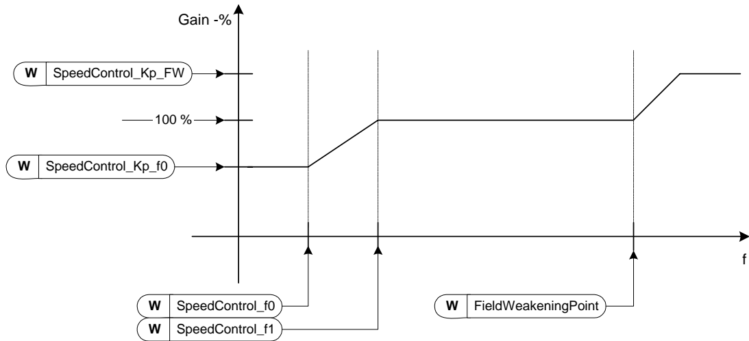
图6-36速度控制器自适应增益
