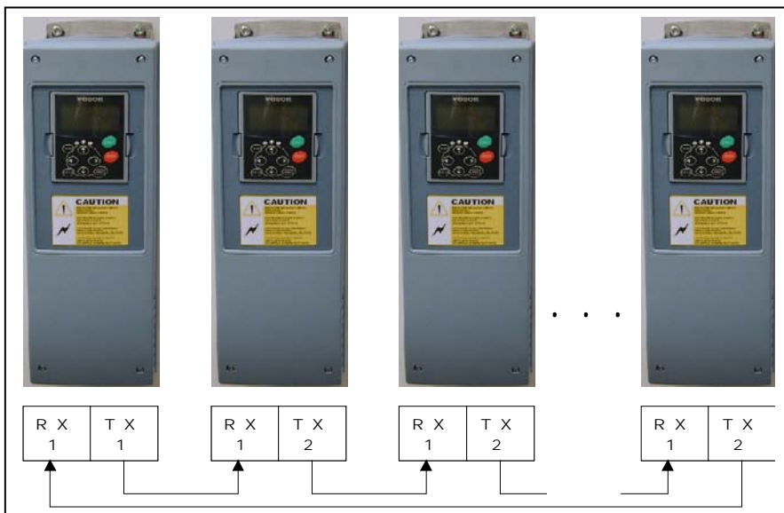
图7-3. 系统总线与NXOPTD2 板物理连接
