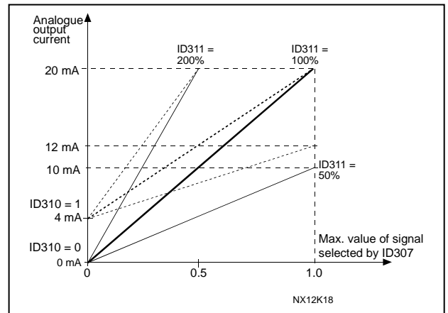
图6-9. 模拟输出信号标定
