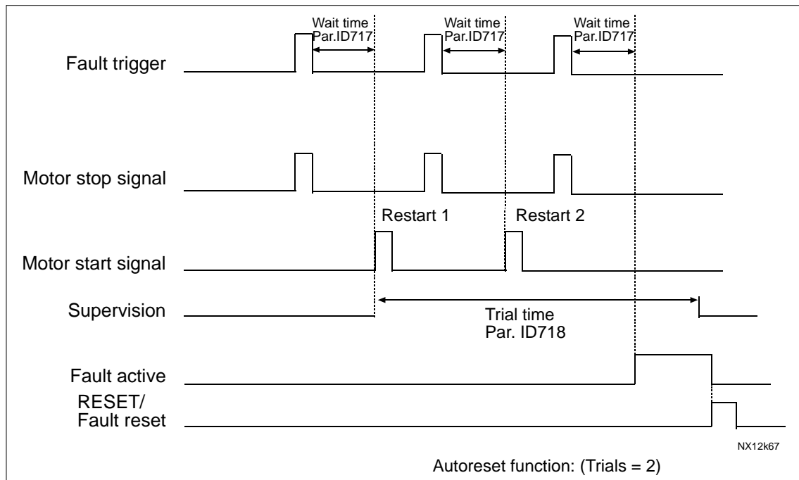
图6-35. 自动重启例子
