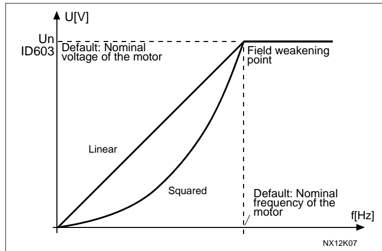
图6-1. 电机电压的线性和二次变化
