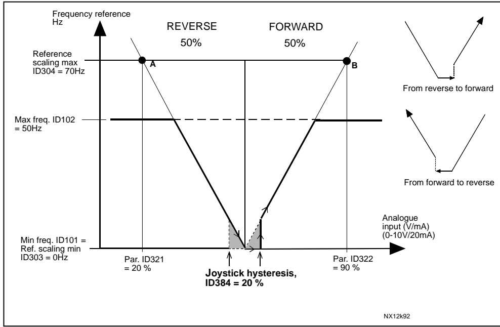
图 6-15. 手柄滞后例子, 例子中, 参数 ID385(睡眠限制)的值等于 0
