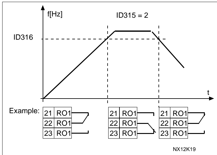
图6-10. 输出频率监控
