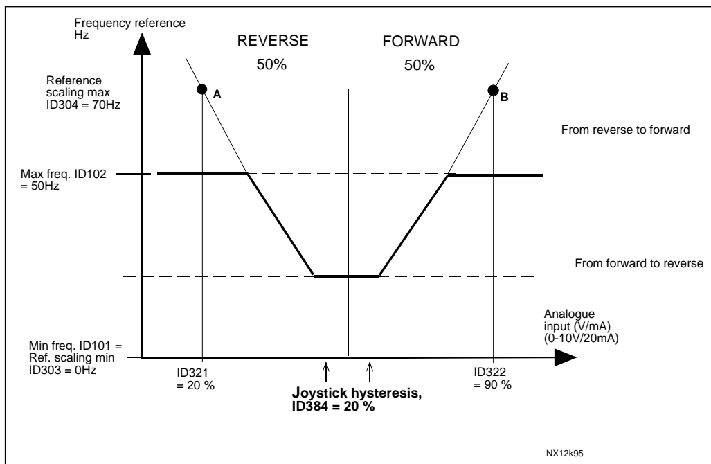
图6-17. 35Hz 最小频率手柄滞后
