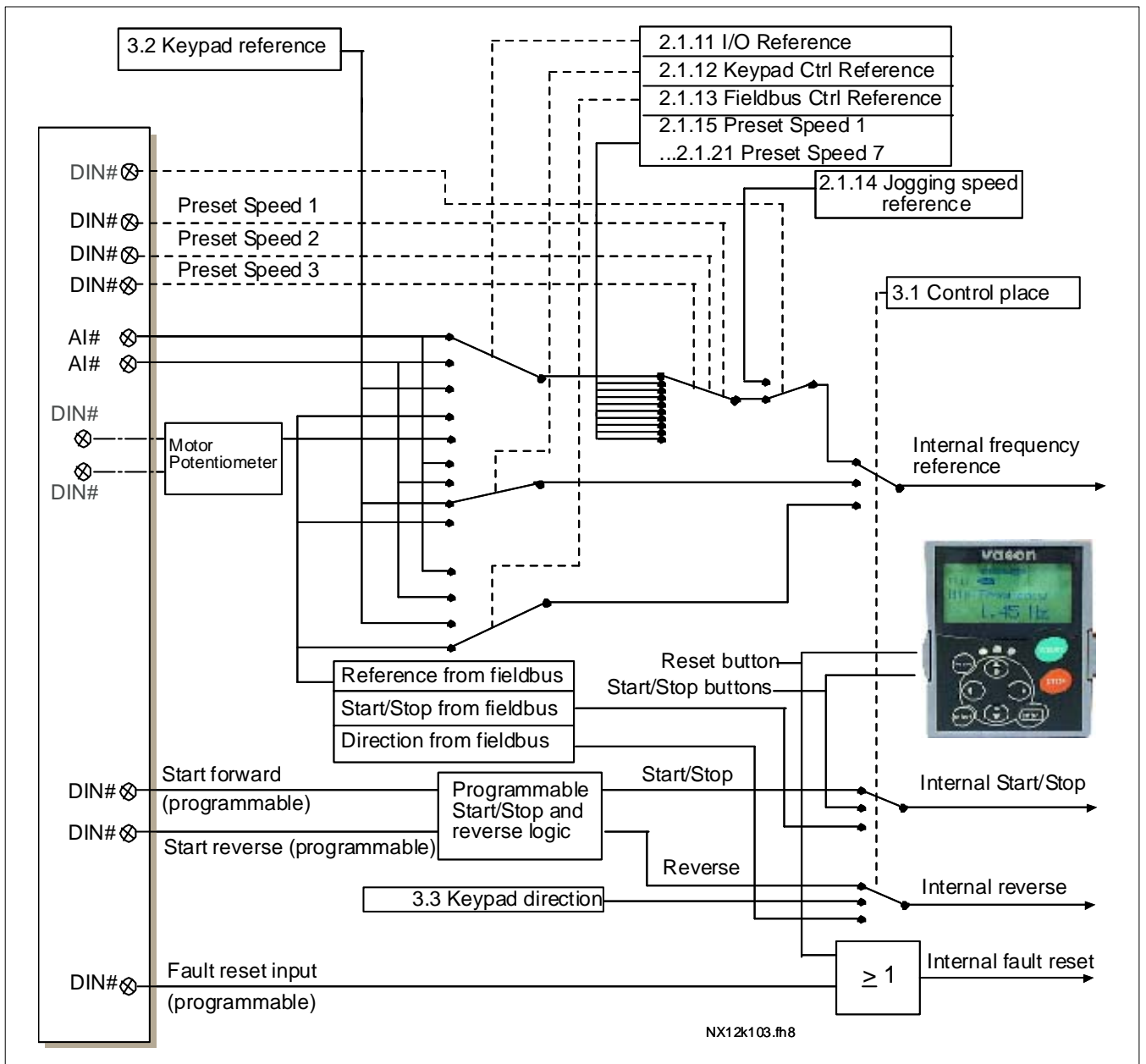
图3-1. 船舶行业应用宏中的控制信号逻辑
