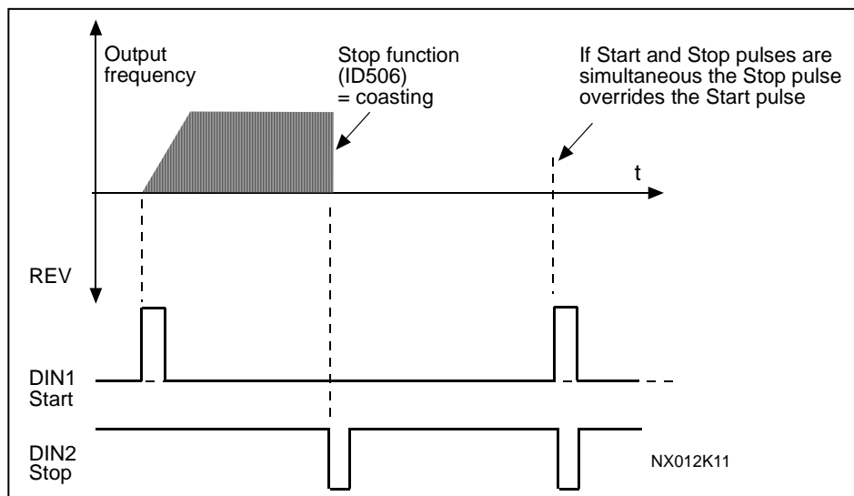
图6-5. 启动脉冲/停车脉冲
