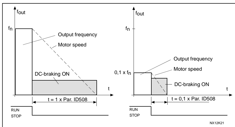
图6-24. 惯性停机模式下的直流制动时间
