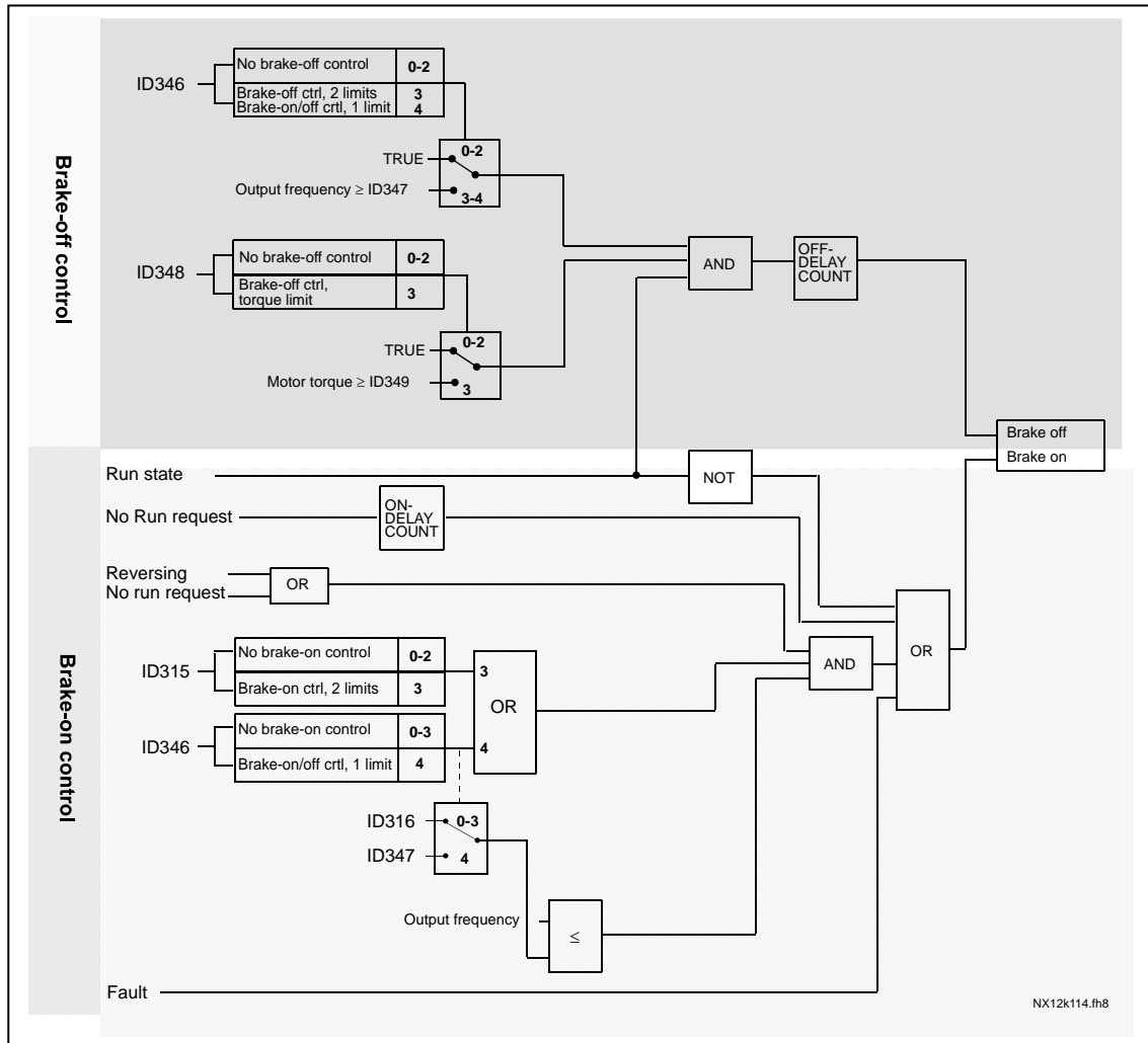
图 7-2. 制动控制逻辑
