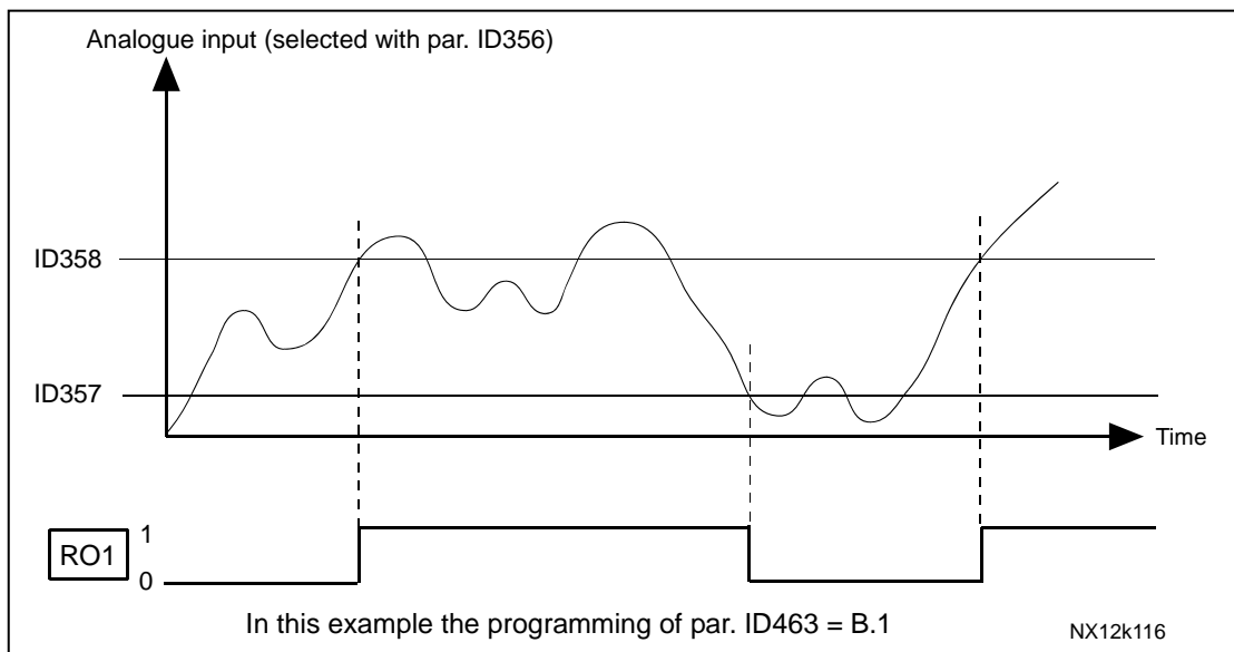
图6-14. On/Off 控制举例
