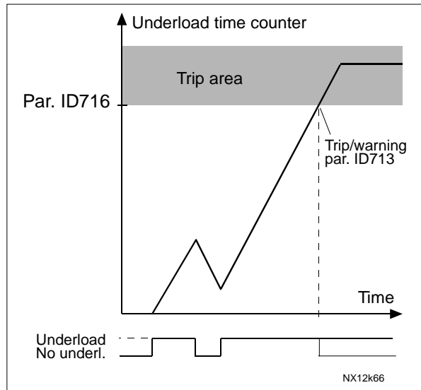
图 6-34. 欠载时间计时器功能
