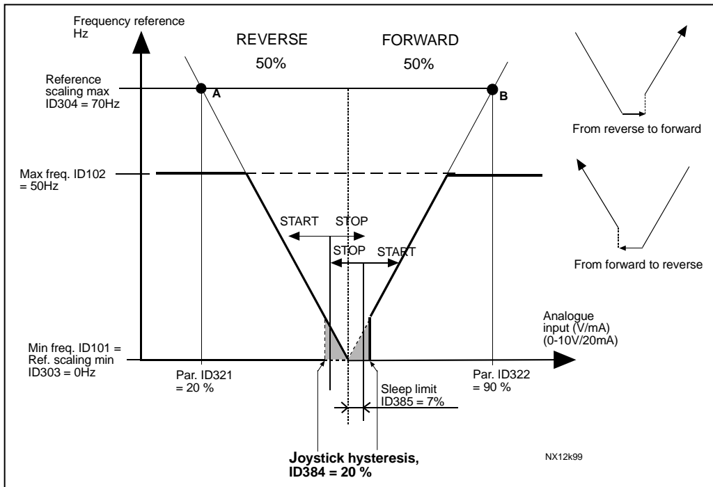
图 6-16. 睡眠限制功能例子
