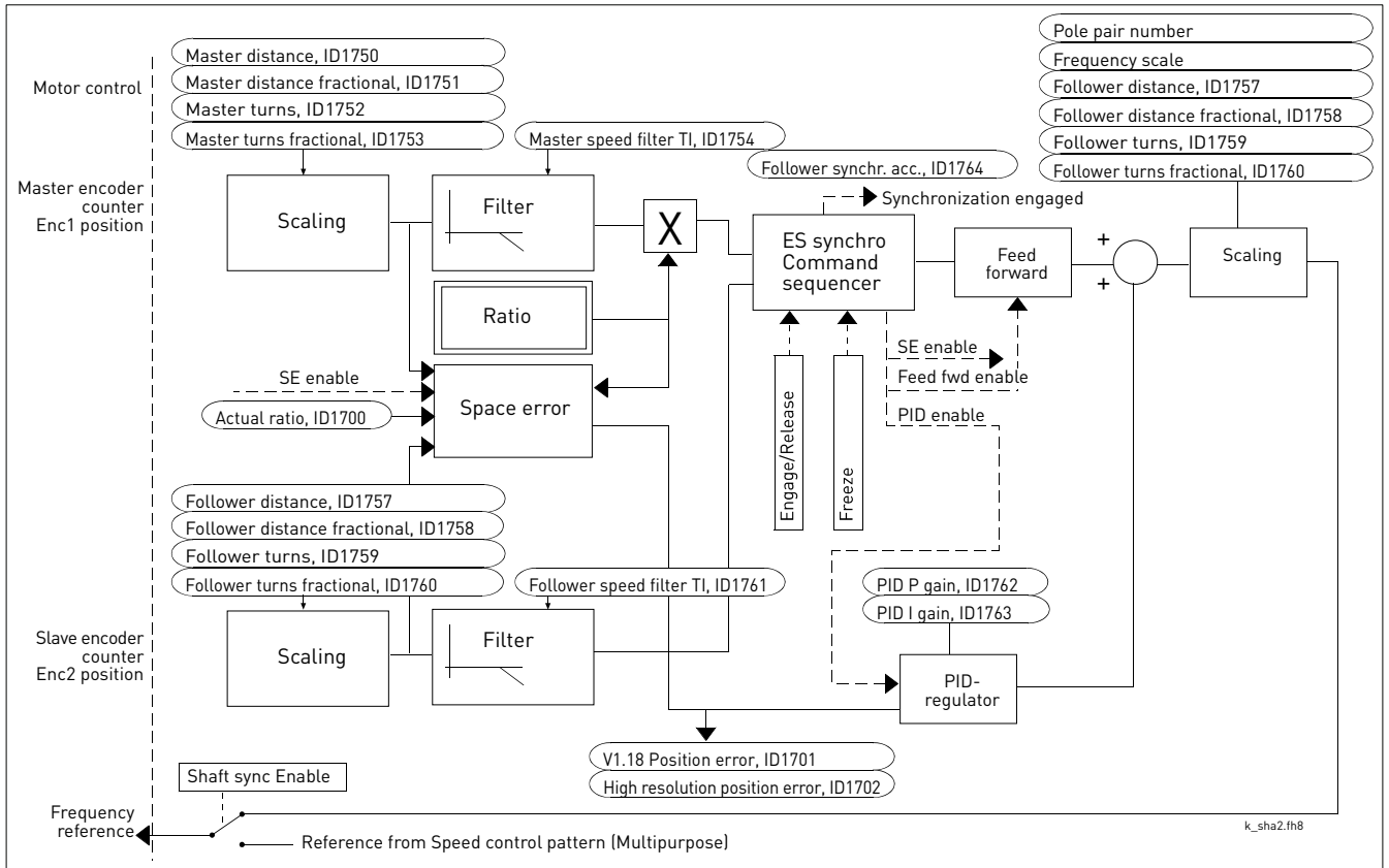
图 29. 轴同步应用, 功能块图
