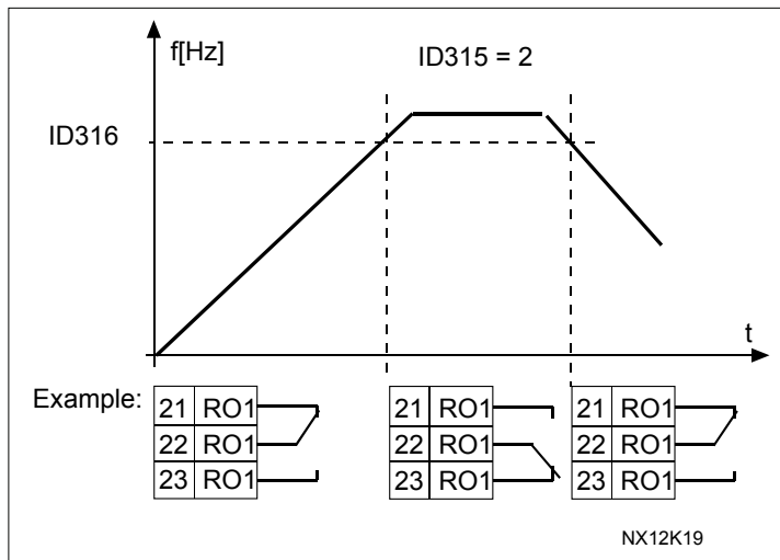
图 11. 输出频率监控
