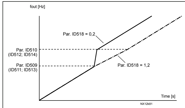
图 22. 在禁用频率段的斜坡速度定标
