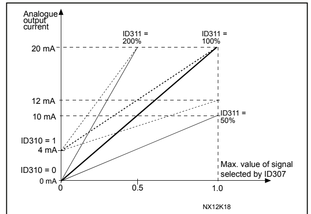
图 10. 模拟输出定标
