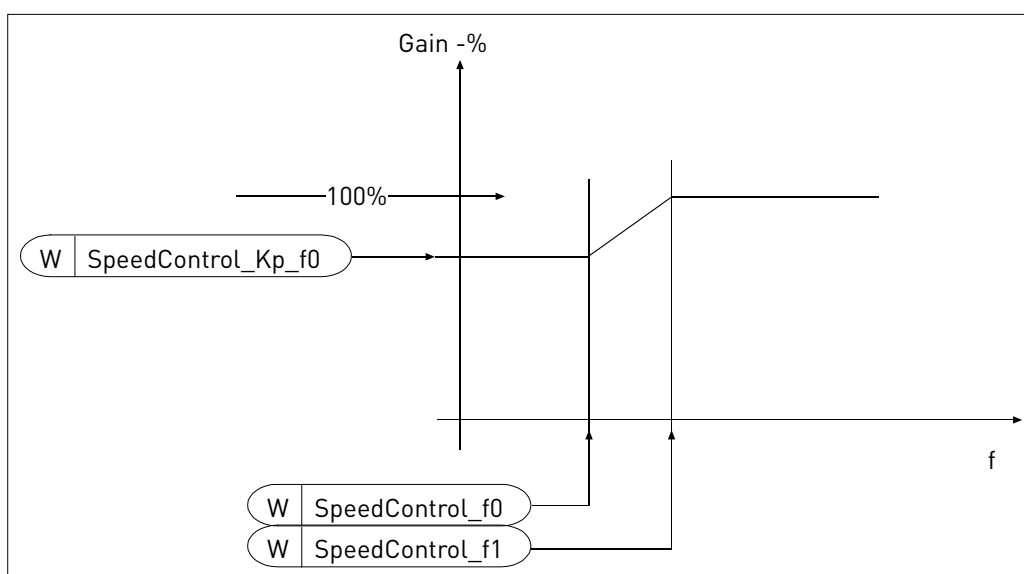
图 28. 低速速度调节器增益表
