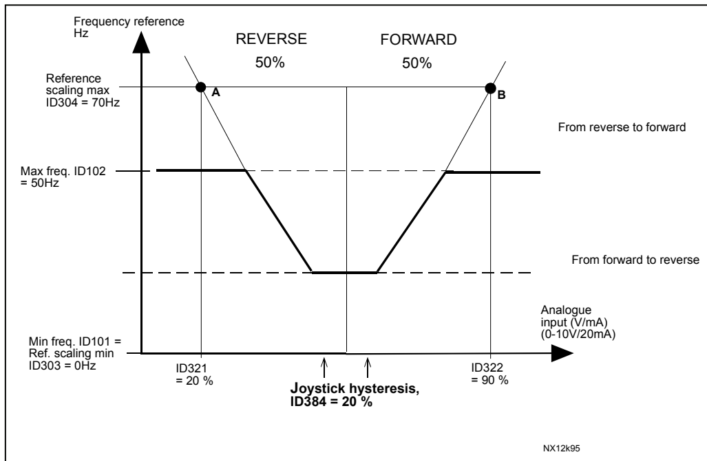
图 16.最小频率在 35Hz 操纵杆滞环
