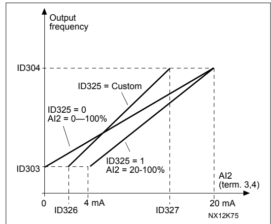
图13. 模拟输入 AI2 定标
