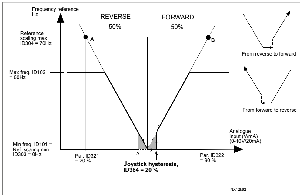
图 15. 一个操纵杆延时的例子。在这个例子中，ID385(休眠限制)的值为 0
