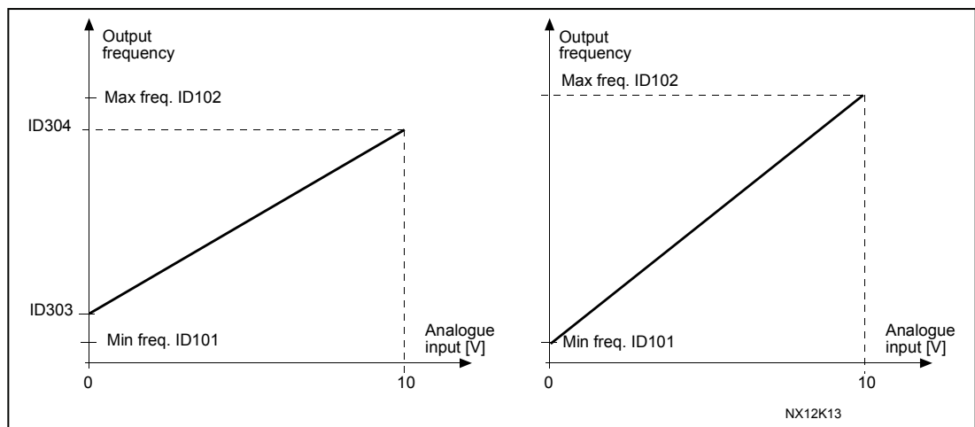
图 7. 左: 参考值定标
