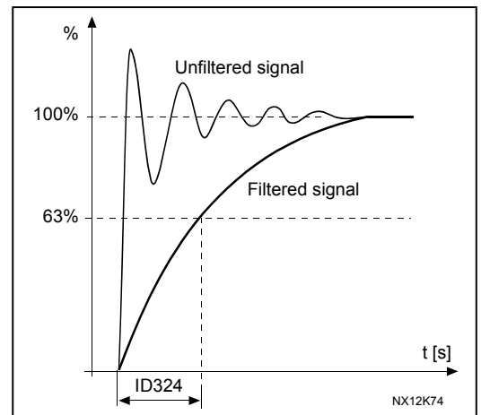
图 12. AI1 信号滤波
