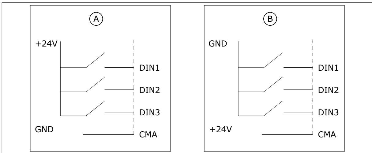
图 25: 正/负逻辑
