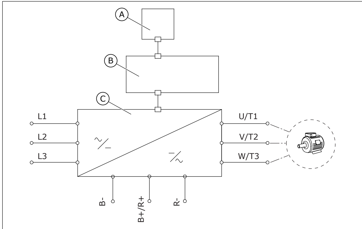
图 19: 主要连接图
