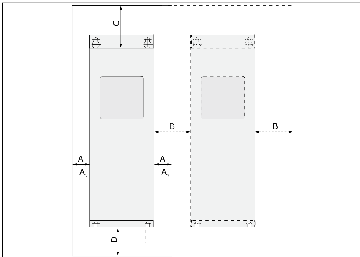
图 16: 安装空间
