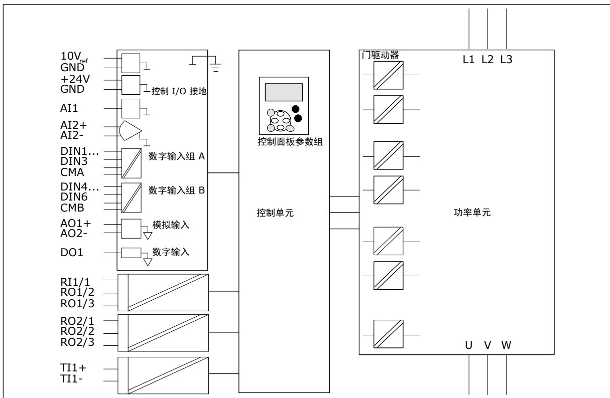
图 31: 电隔离屏障
