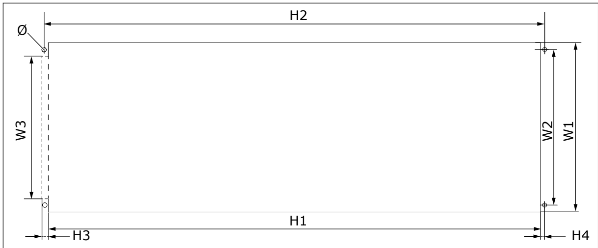
图 10: 使用法兰时的开口和变频器轮廓尺寸, FR4 至 FR6
