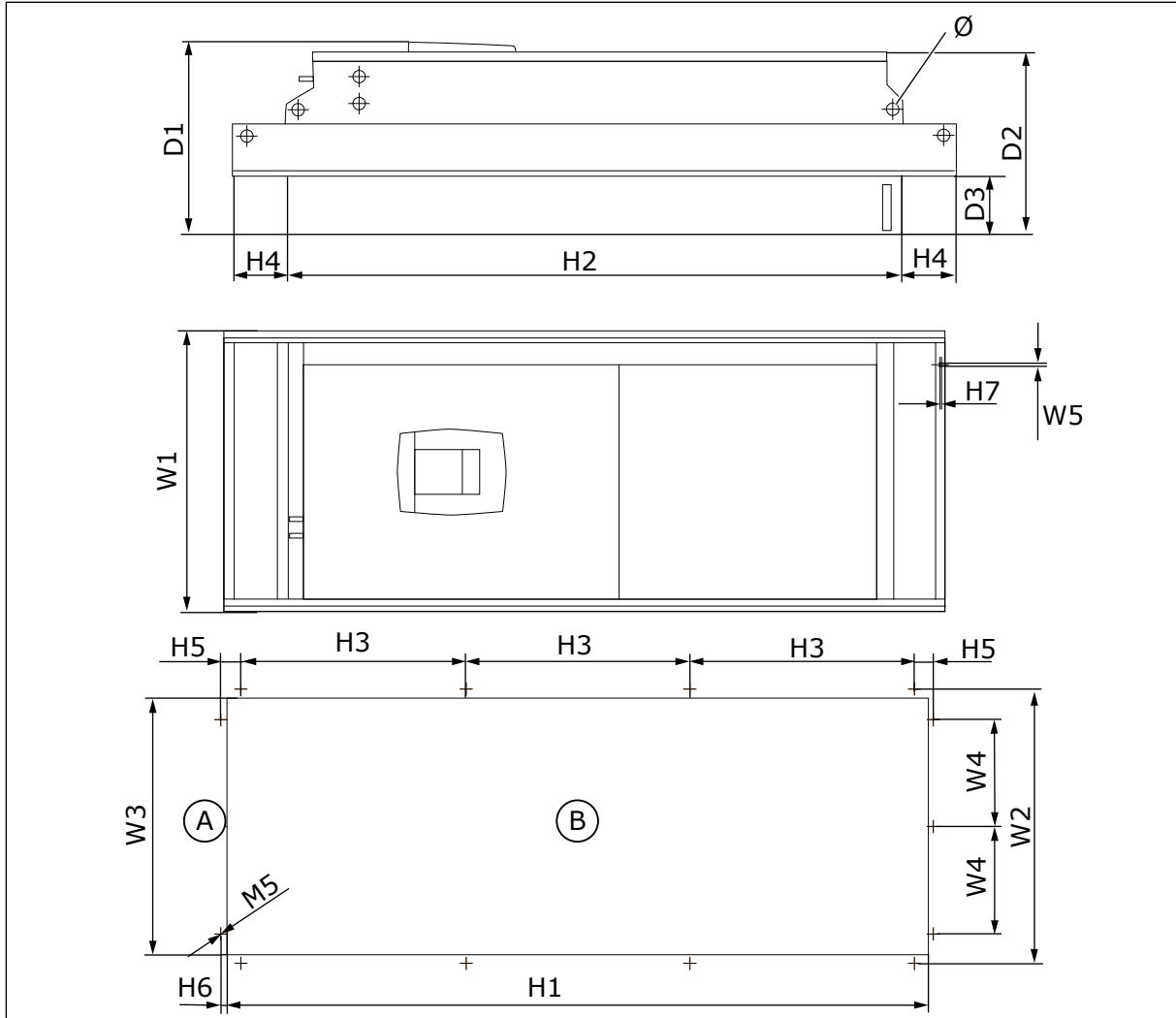
图 14: NXS 和 NXP 交流变频器的尺寸, F9
