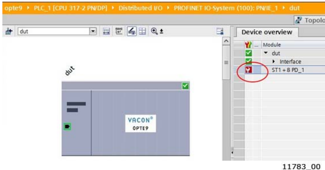
Figure 42. Siemens TIA portal - Alarm indicator
