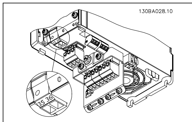
Forbindelse til 24 V back-up-forsyning.
