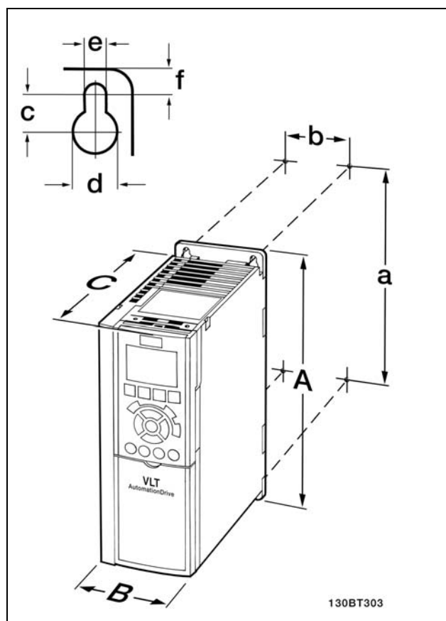
FC 300 IP20 - se den medfølgende tabel for mekaniske dimensioner.
