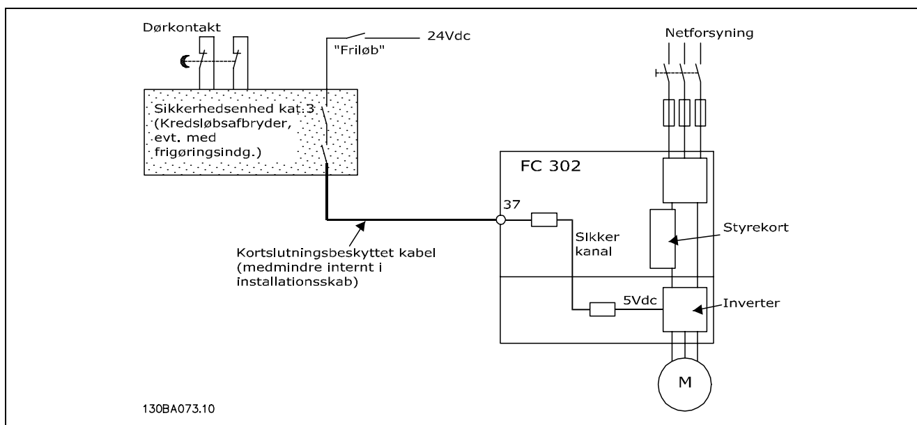
Illustration af disse vigtige elementer i installationen for at opnå standsningskategori 0 (EN 60204-1) med sikkerhedskategori 3 (EN 954-1).
