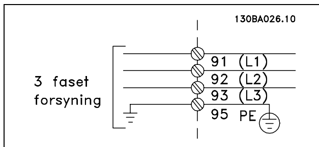
Klemmer til net og jording.
