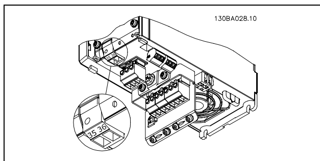
Tilslutning til 24 V back-up-forsyning.
