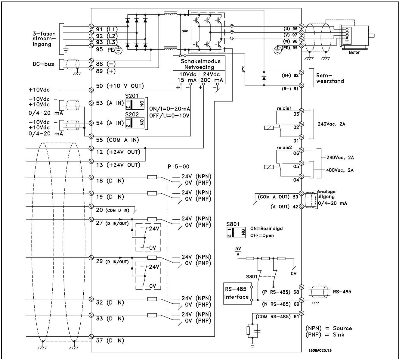
Schema met alle elektrische klemmen. Klem 37 maakt geen onderdeel uit van de FC 301.
