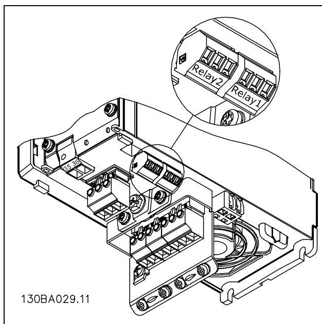
Klemmen voor aansluiten relais.
