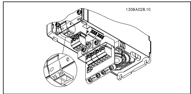
Aansluiting op 24V-reservevoeding.
