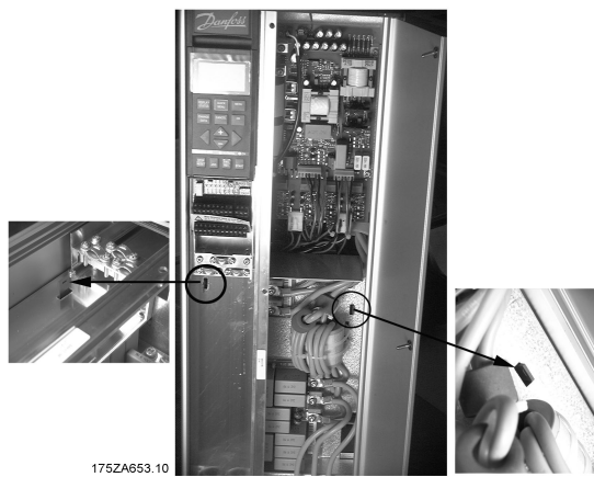
Compact IP 20/NEMA 1 VLT 5011 - 5016 200 - 240 V VLT 5027 - 5032 380 - 500 V VLT 5027 - 5032 525 - 600 V
