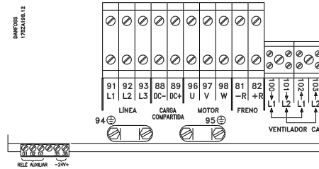
Fig. 8 IP 54 Compacto 5016 - 5062 380 - 500 V 5008 - 5027 200 - 240 V
