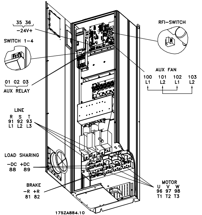
Compact IP 00 con sconnessione e fusibili VLT 5202-5302 380-500 V
