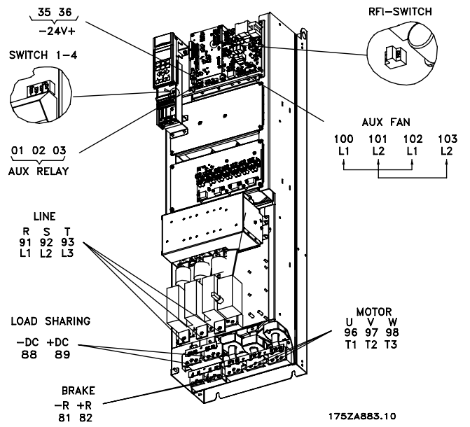
Compact IP 00 con sconnessione e fusibili VLT 5202-5302 380-500 V
