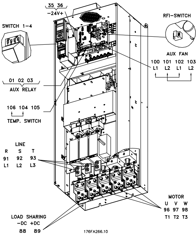
Pozice zemních svorek, IP 00
