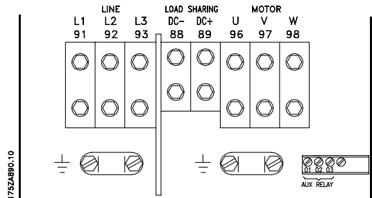
Krytí IP 54/NEMA 12, provedení kompaktní VLT 8102-8122, 380-480 V
