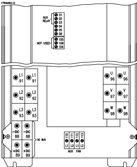
IP 00/šasi a IP 20/NEMA 1 VLT 8200-8300, 525-600 V
