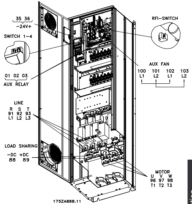
IP 54/NEMA 12, IP 21/NEMA 1 с разъединителем и сетевым предохранителем VLT 8152-8352, 380-480 B
