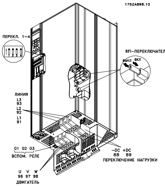
Compact IP 20/NEMA 1 VLT 8102-8122, 380-480 В
