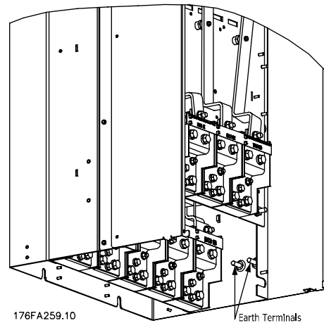
Расположение клемм заземления, IP 00
