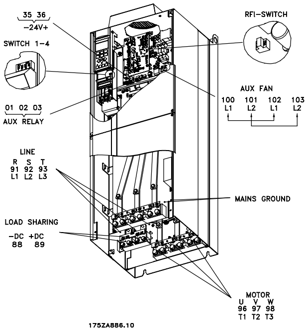
IP 00/Шасси VLT 8152-8352, 380-480 B
