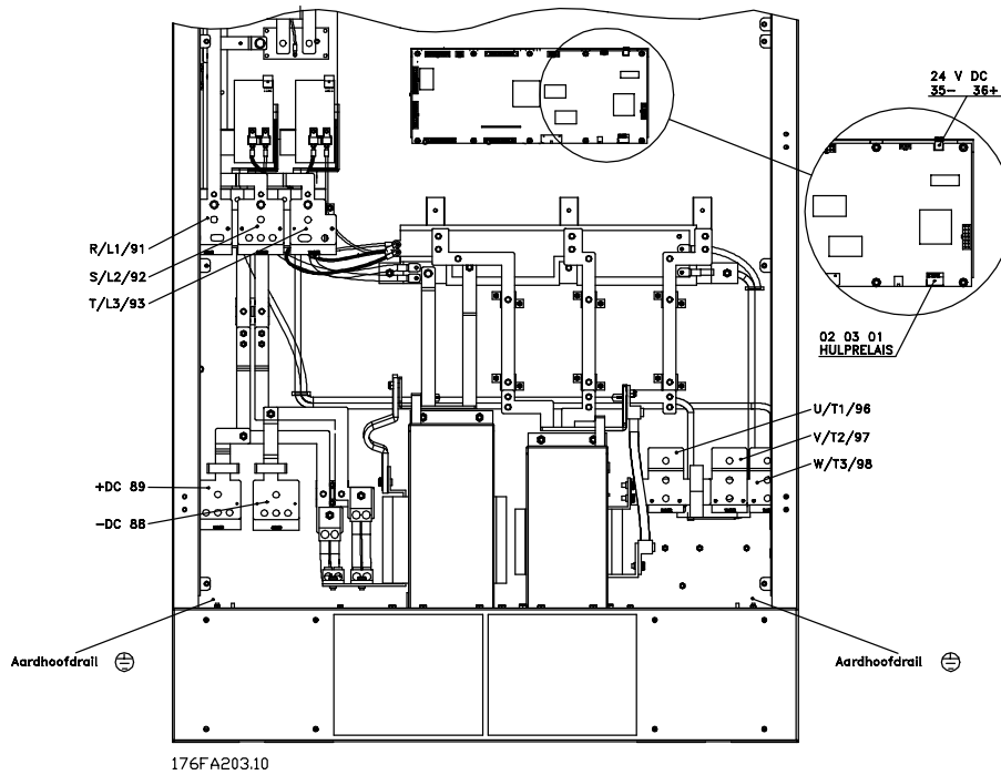
Compact IP 00/Chassis, IP 20/NEMA 1, en IP 54/NEMA 12 VLT 8450-8600 380-480 V zonder uitschakelaars en netzekeringen
