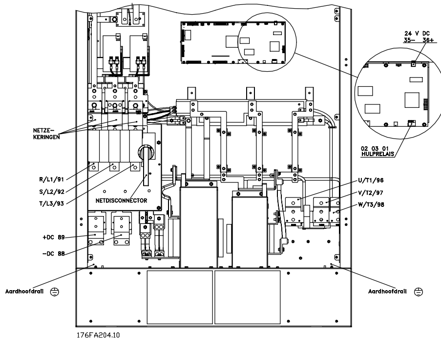
Compact IP 00/Chassis, IP 20/NEMA 1, en IP 54/NEMA 12 VLT 8450-8600 380-480 V met uitschakelaars en hoofdzekeringen
