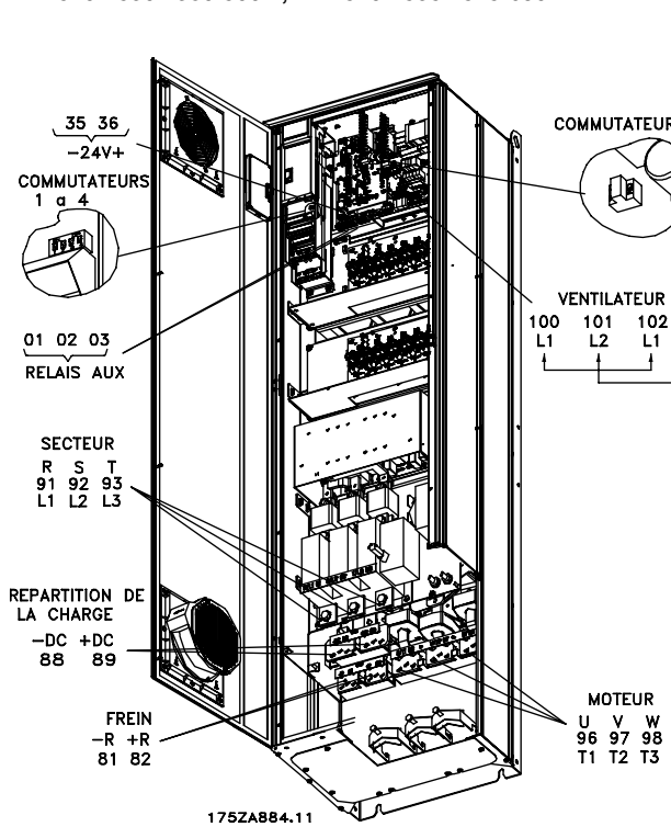
Compact IP21/IP54 avec rupteur et fusible VLT 5202-5302 380-500 V, VLT 5202-5352 525-690 V
