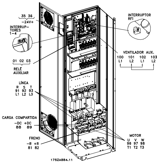
Compact IP 21/IP54 con sistema de desconexión y fusible VLT 5202-5302 380-500 V, VLT 5202-5352 525-690 V
