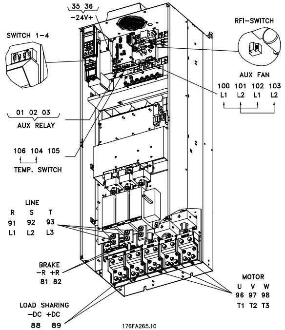
Krytí IP 00 s odpojováním a pojistkou, provedení kompaktní VLT 5352-5552 380-500 V
