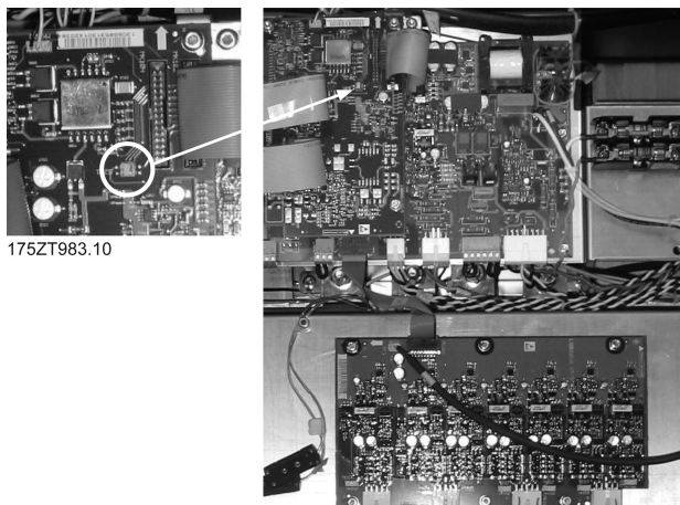
Krytí IP 54, provedení kompaktní VLT 5072-5102 380-500 V
