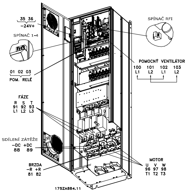
Krytí IP 21/IP54 s odpojováním a pojistkou, provedení kompaktní
