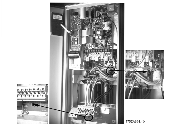
Krytí IP 54, provedení kompaktní VLT 5008-5011 200-240 V VLT 5016-5027 380-500 V
