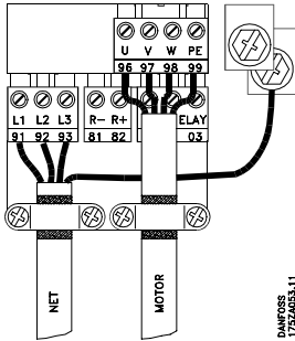
Obr. 5 Provedení kniha, krytí IP 20 5001 - 5011 380 - 500 V 5001 - 5006 200 - 240 V
