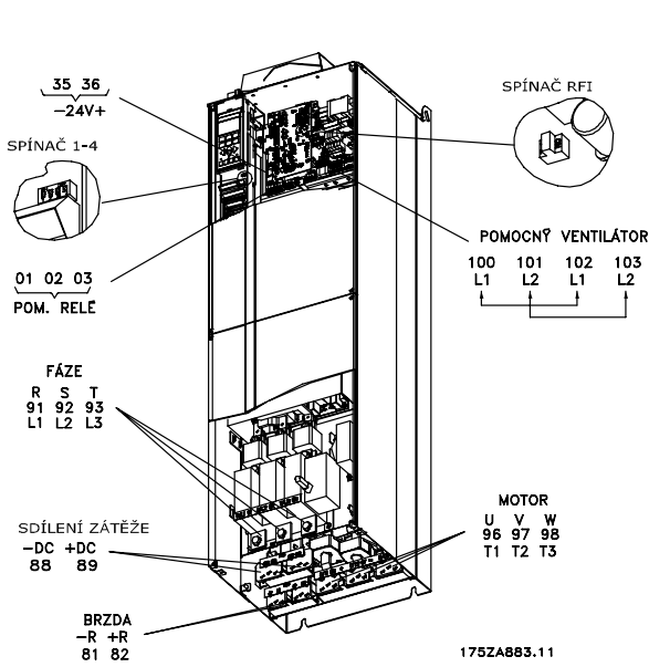
Krytí IP 00 s odpojováním a pojistkou, provedení kompaktní VLT 5202-5302 380-500 V, VLT 5202-5352 525-690 V
