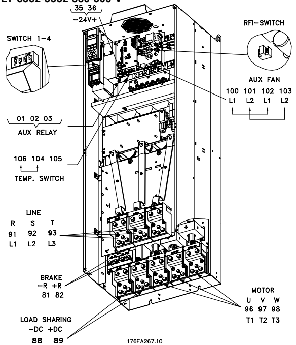
Krytí IP 00 bez odpojování a pojistky, provedení kompaktní VLT 5352-5552 380-500 V
